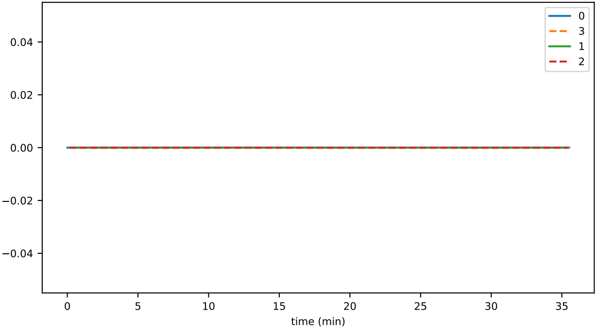
SmartContractService:SystemContractMethodCall_FREEZE_UNFREEZE_total
