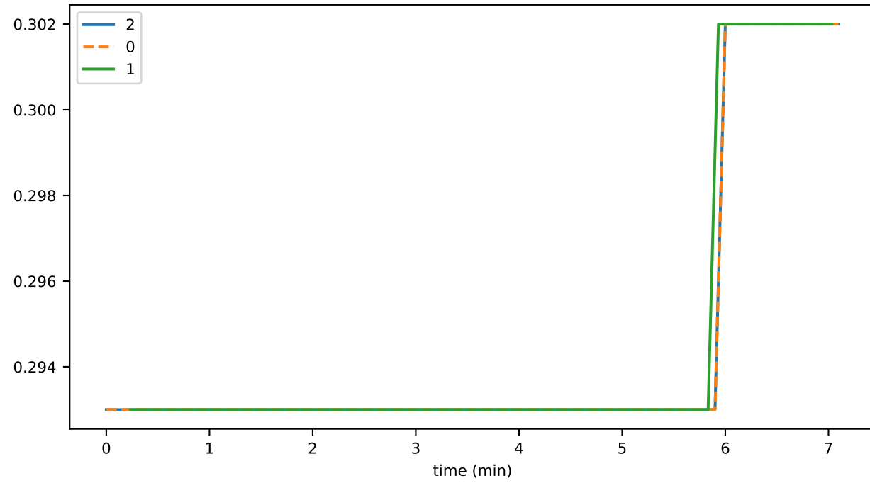
preHandleMicros
