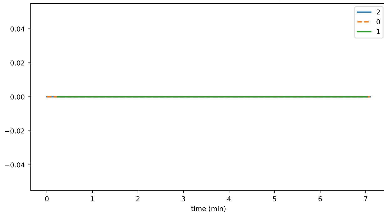
createTransactionRecordThrottledTxns
