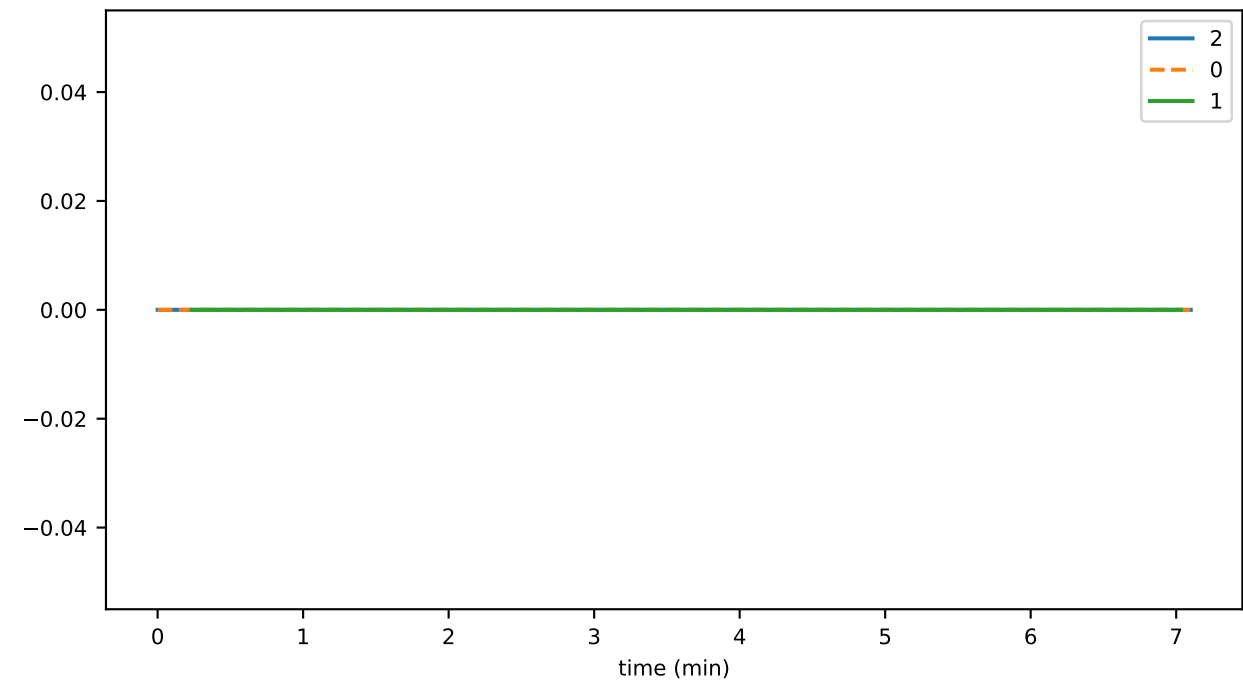
tokenUpdateThrottledTxns
