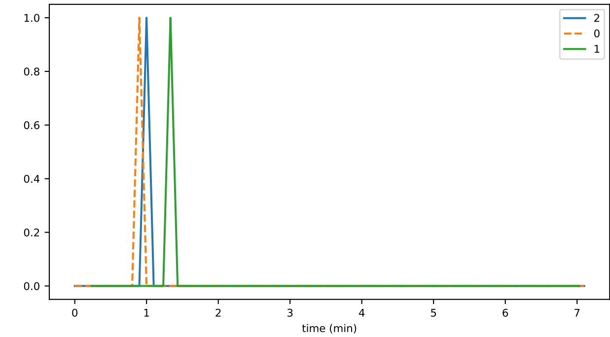
PlatSigEnqueueTime
