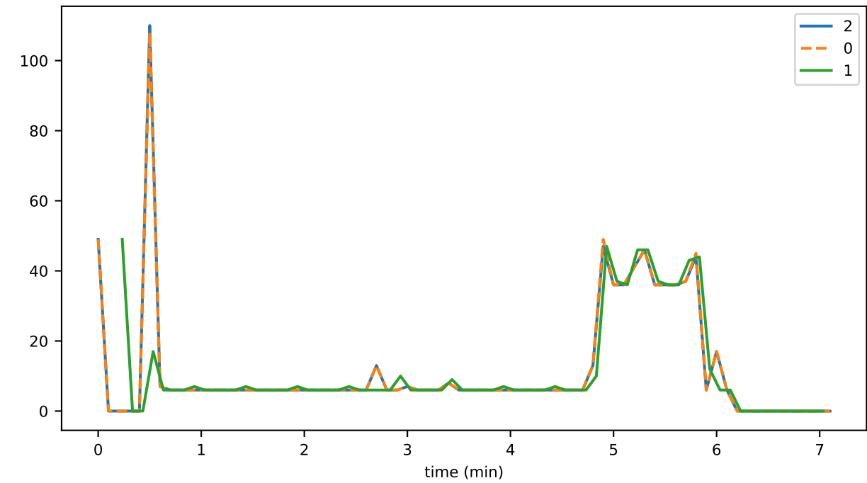
dupEv_per_sec
