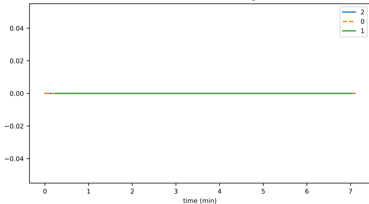
tokenGetNftInfosDurationAvg
