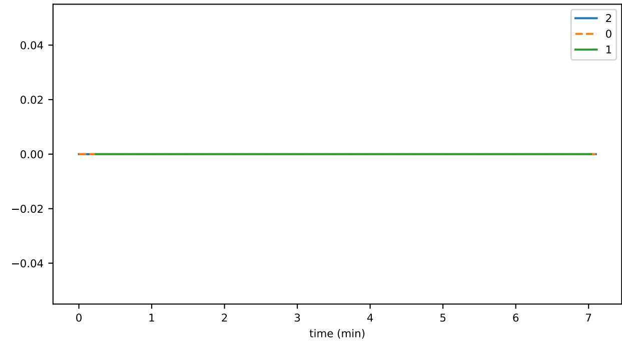
dupEv_per_sec
