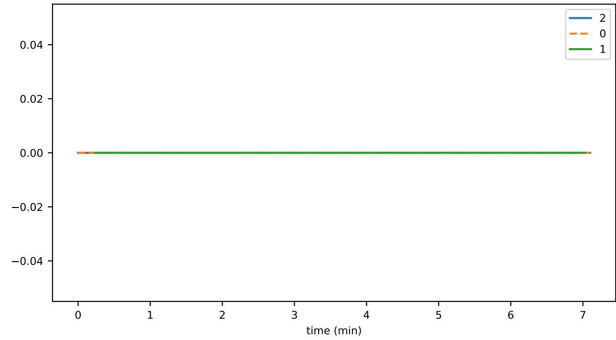
tokenGrantKycToAccountDurationMax
