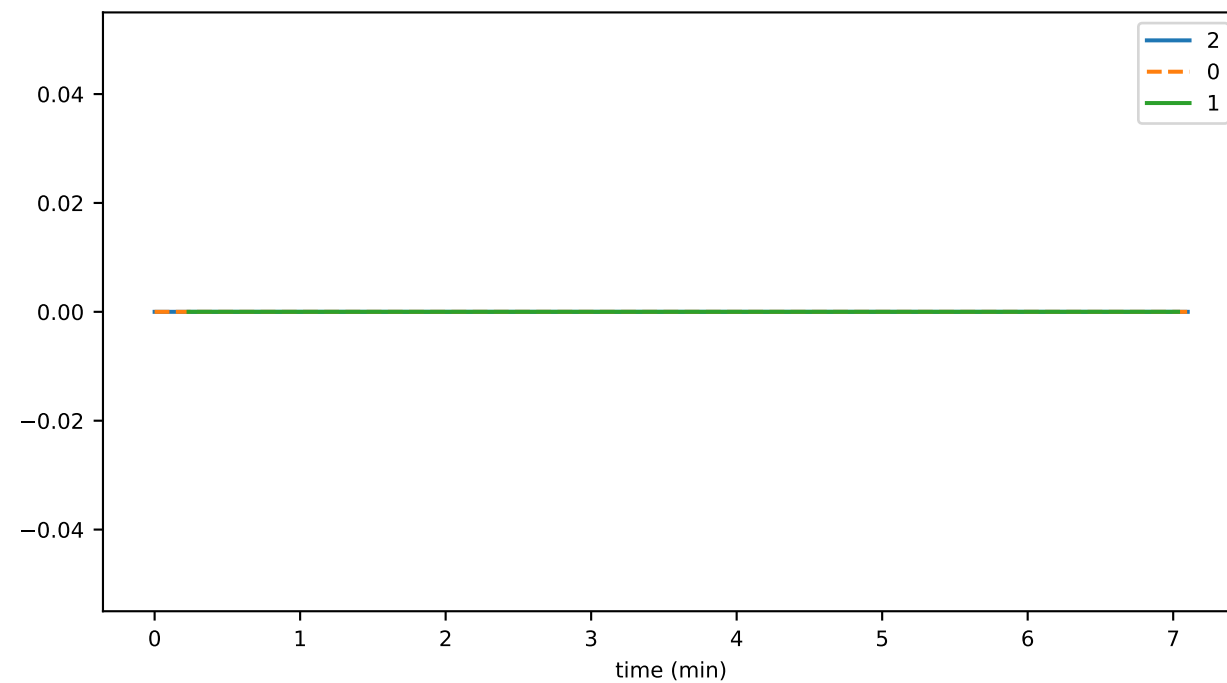
tokenMintThrottledTxns
