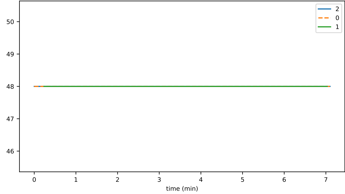
proc
