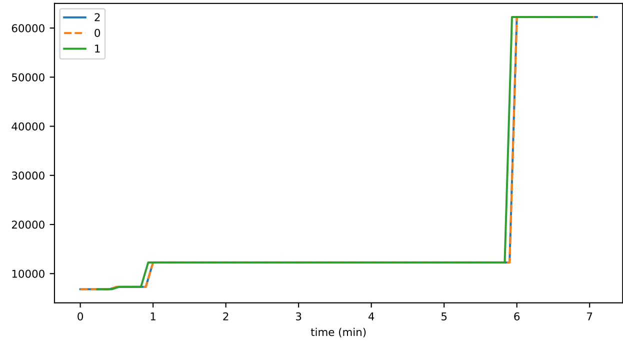
proc
