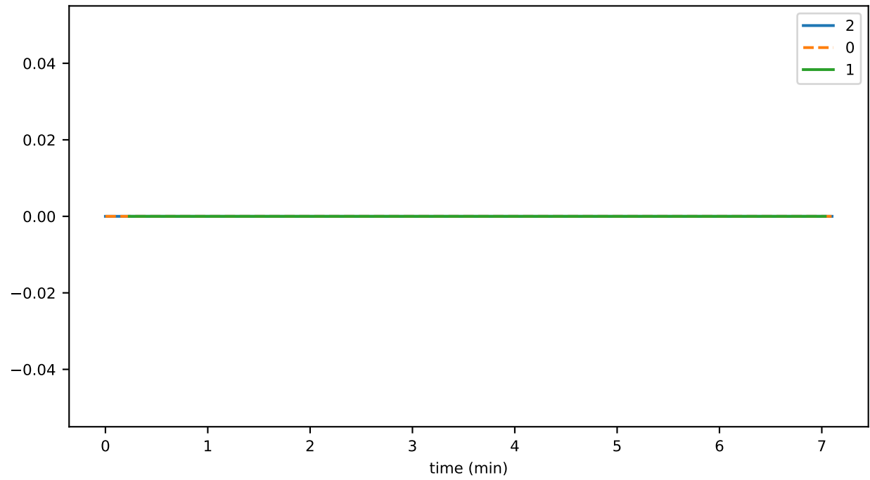
doNotSyncFairSelector
