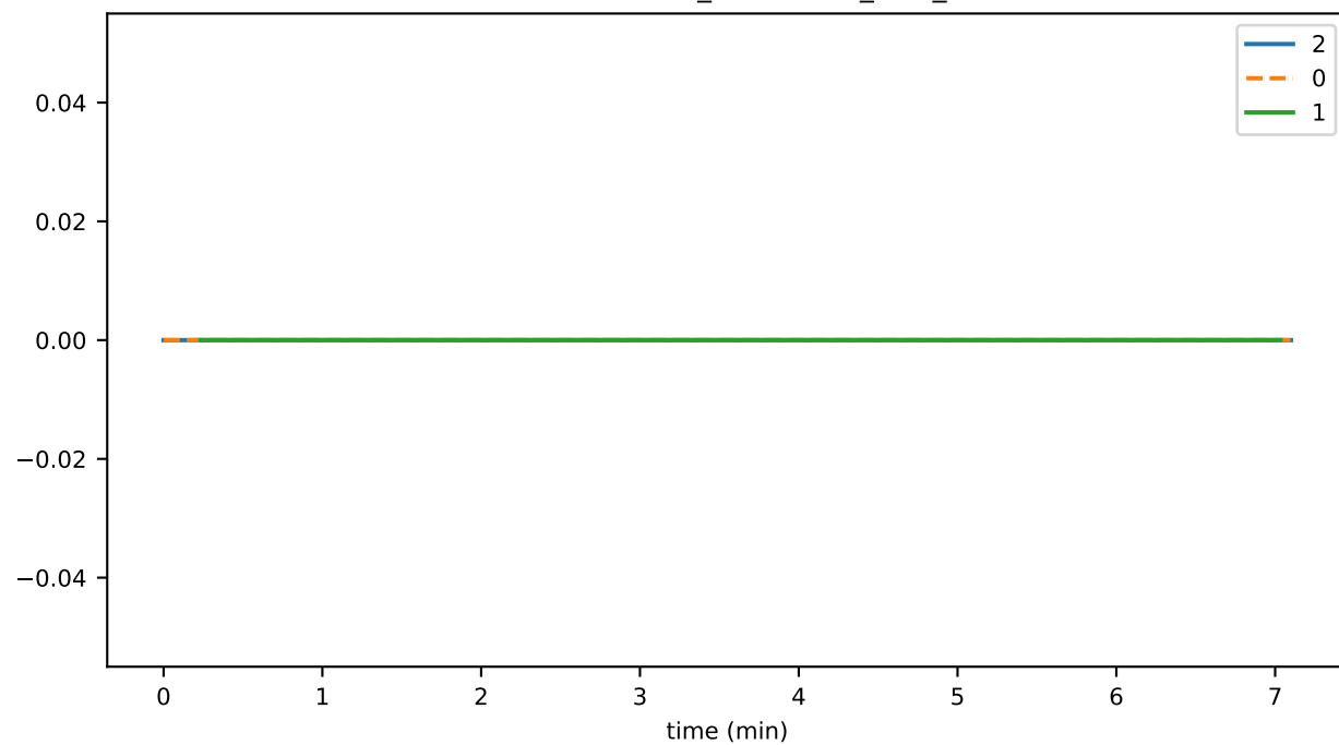
TransactionHandler_unhandled_task_count
