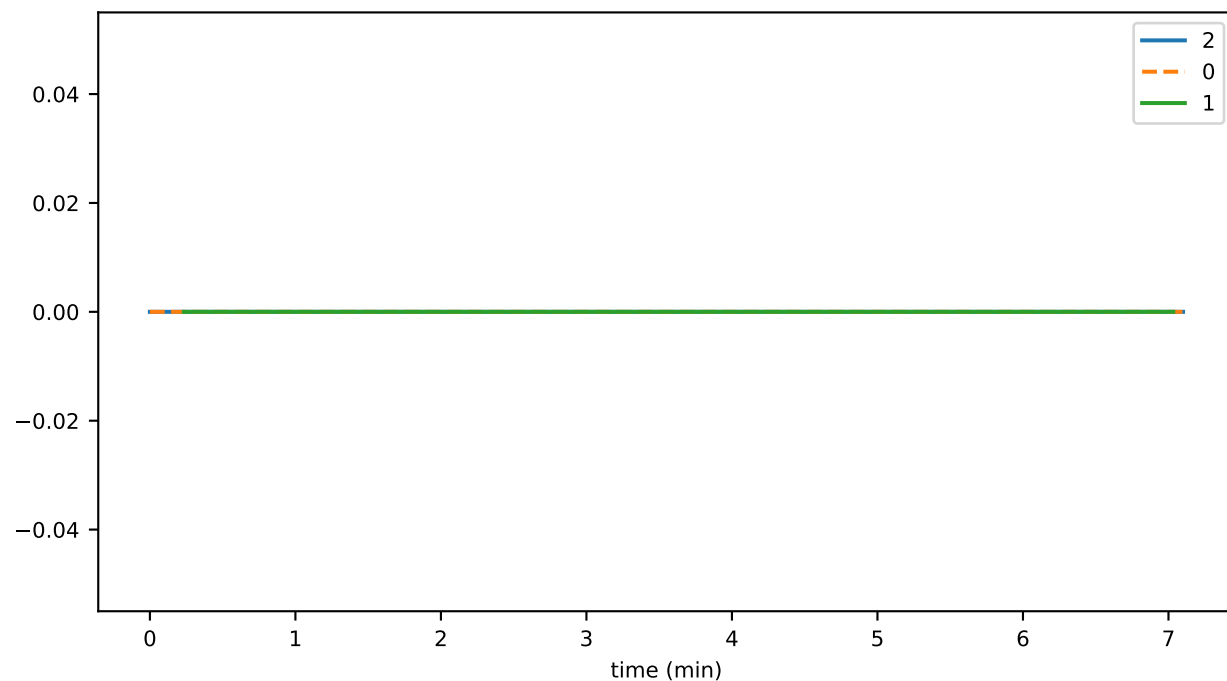
transactionGetFastRecordThrottledTxns
