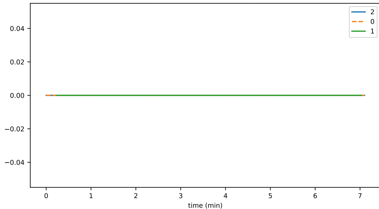
getVersionInfoThrottledTxns
