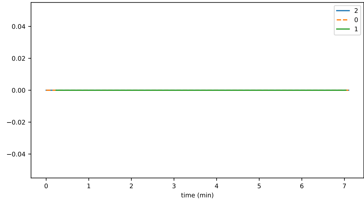
issCount
