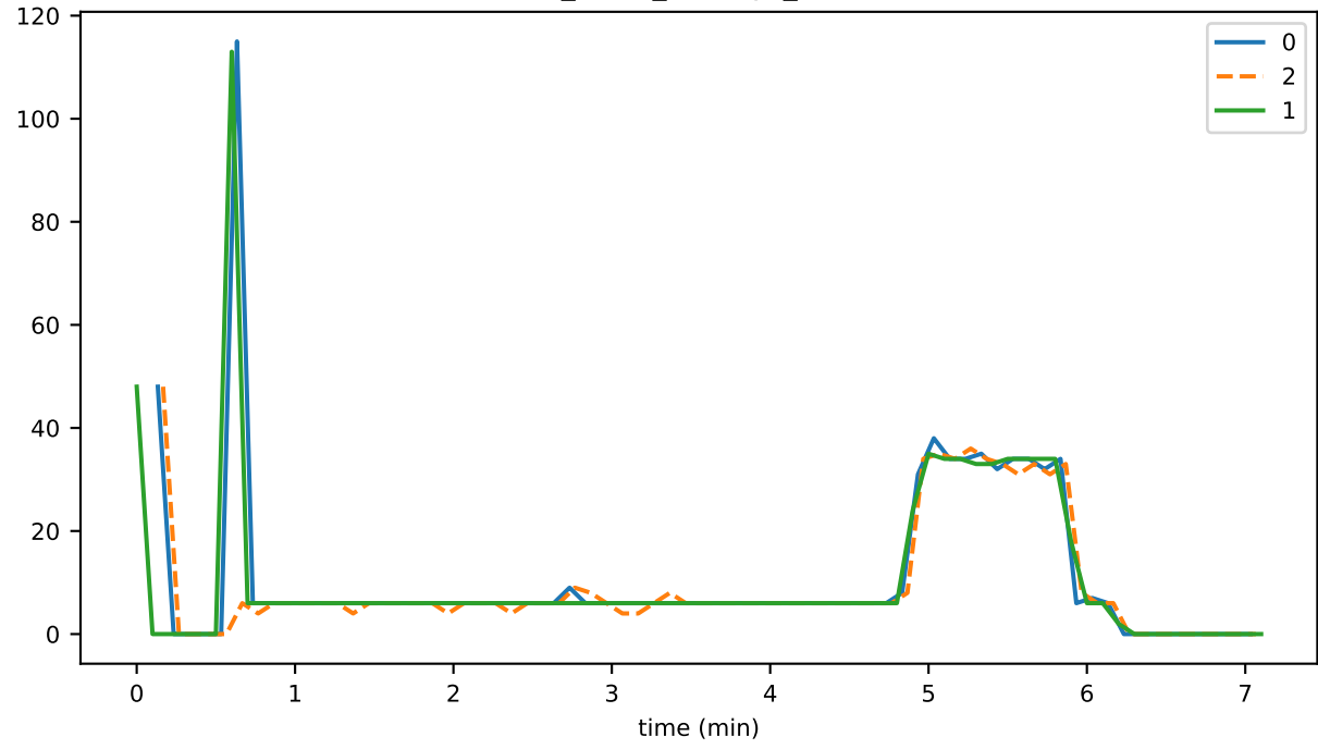
dupEv_per_sec
