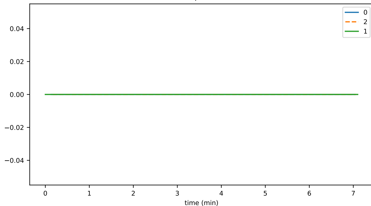
tokenAssociateToAccountDurationMax
