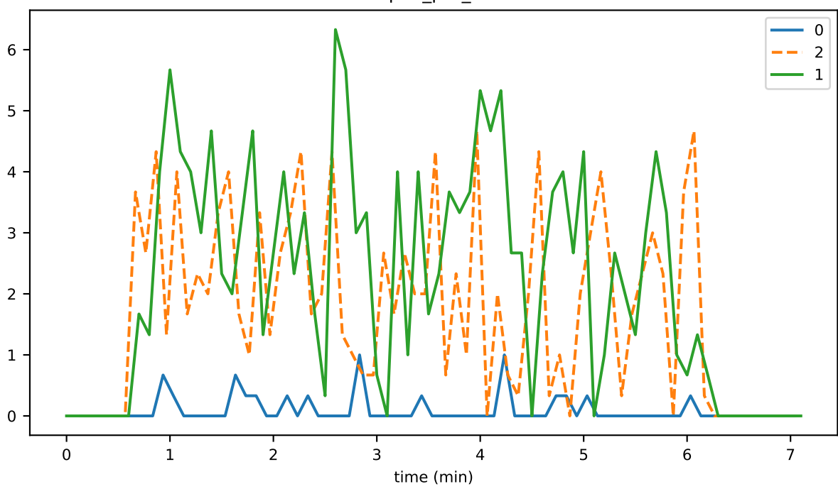
dupEv_per_sec
