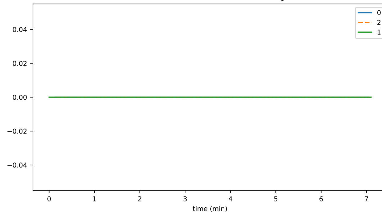
tokenAssociateToAccountThrottledTxns
