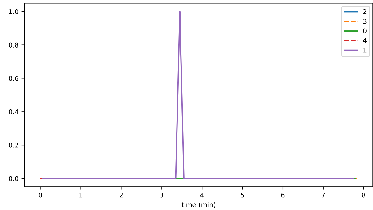
IssDetector_unhandled_task_count
