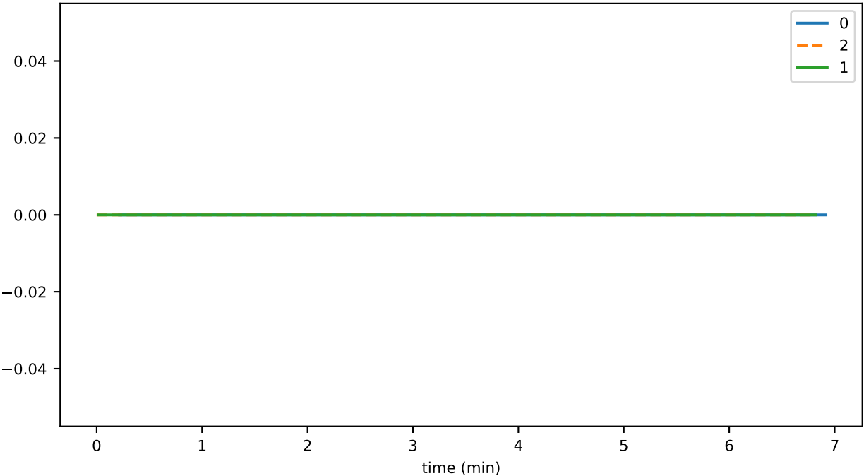
SmartContractService:SystemContractMethodCall_TOKEN_QUERY_total
