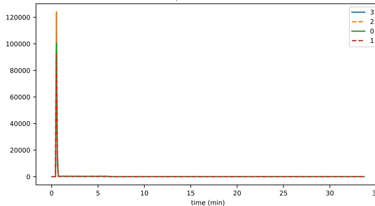
preHandleMicros
