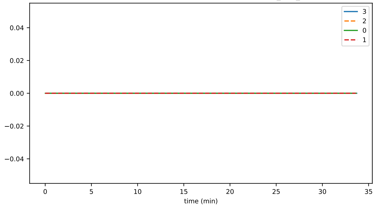
SmartContractService:SystemContractMethodCall_HTS_total
