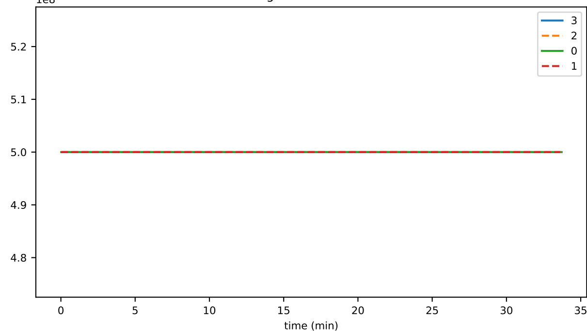
storageSlotsMaxNumber
