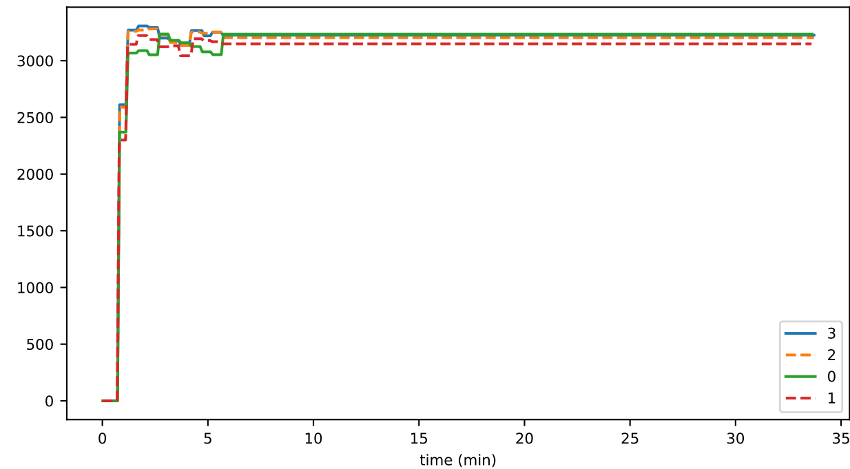
writeStateToDisk
