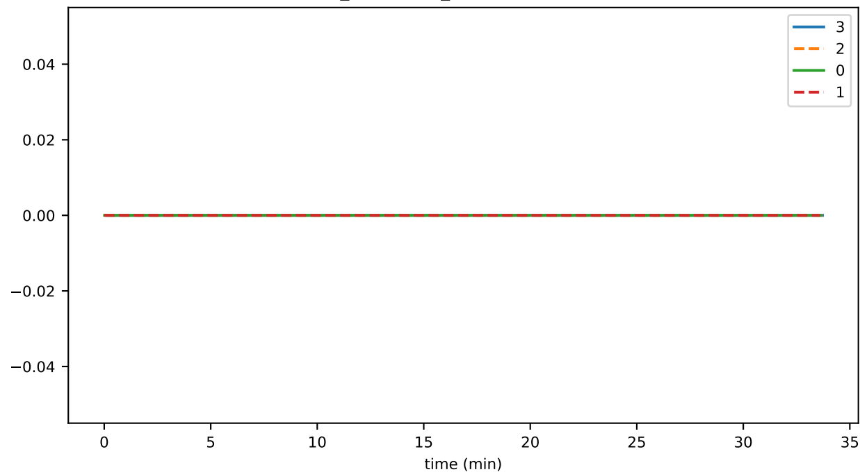
conn_connClose_internalError
