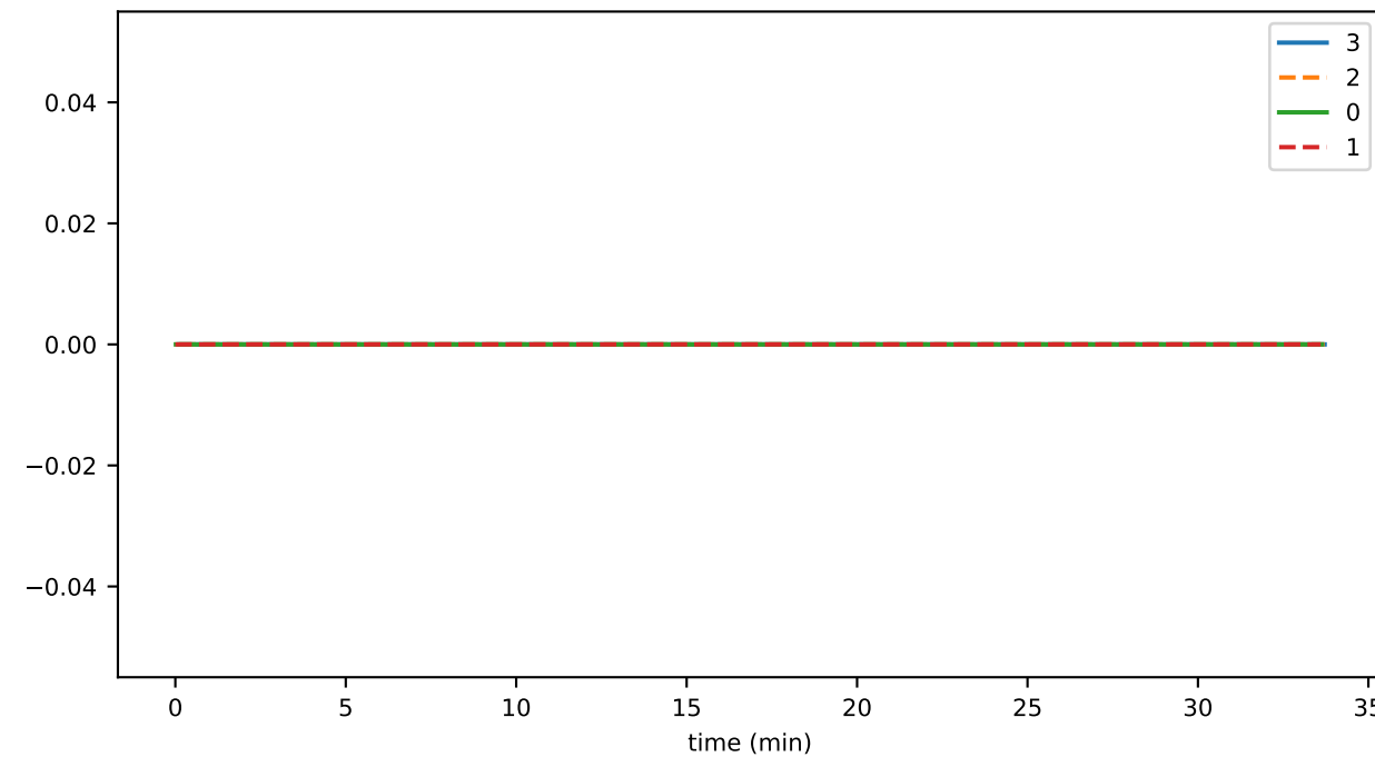
DigSubWrkItmTime
