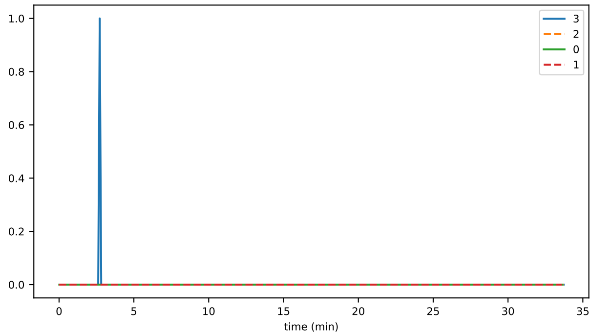
syncRoundLag
