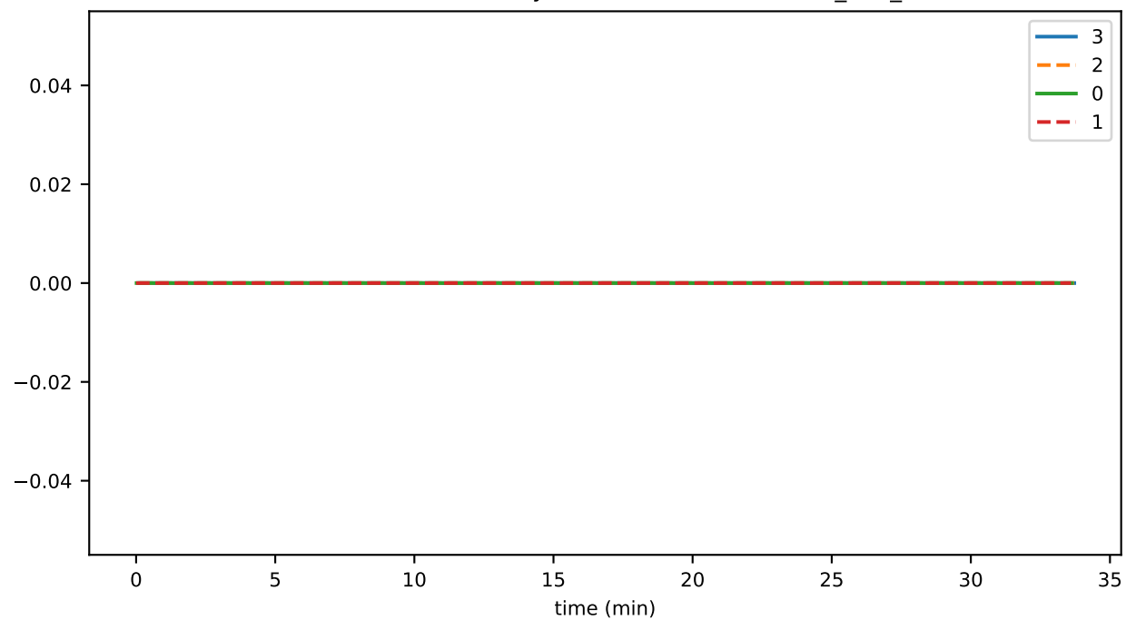
SmartContractService:SystemContractMethodCall_KYC_total
