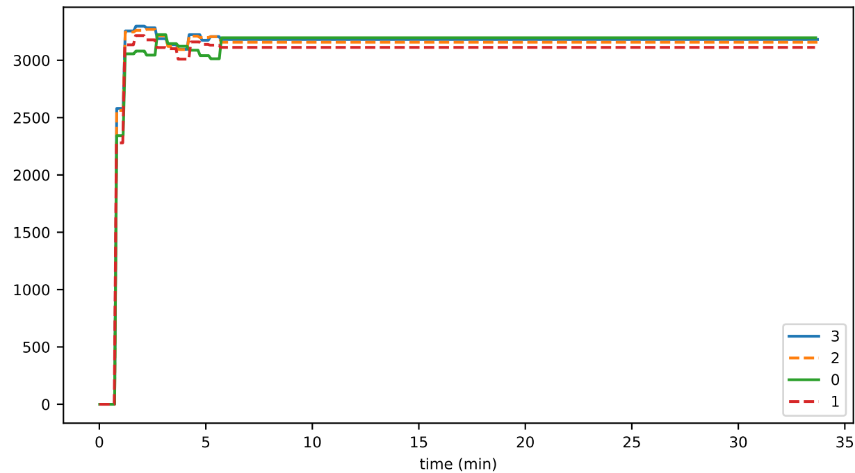
writeMerkleRootToDisk
