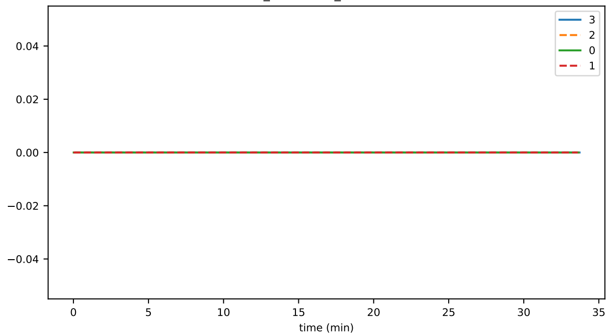
conn_connClose_internalError
