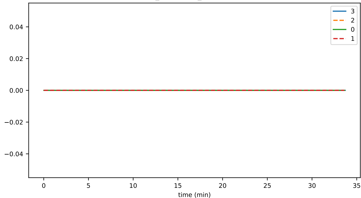
conn_connClose_configUpdate
