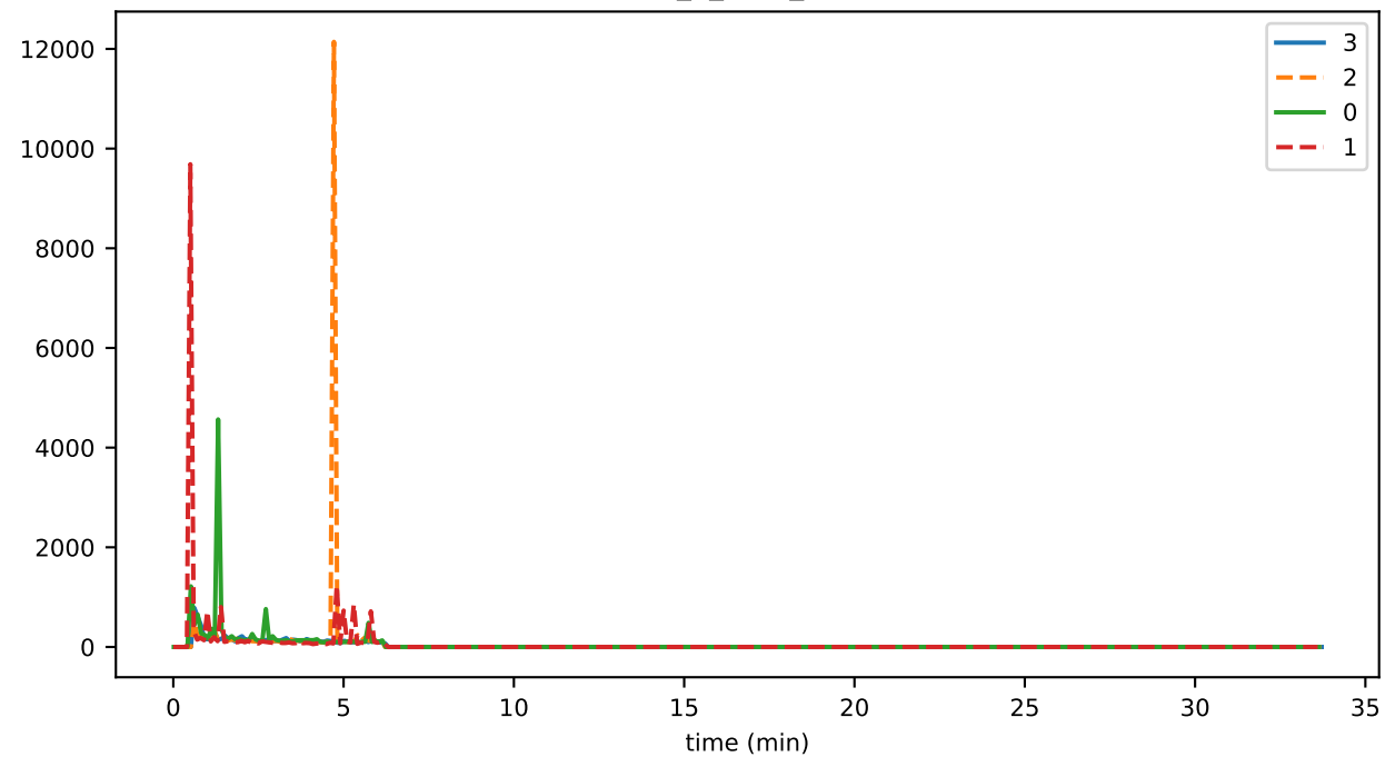
eventDelay_6_pces_runtimeMAX
