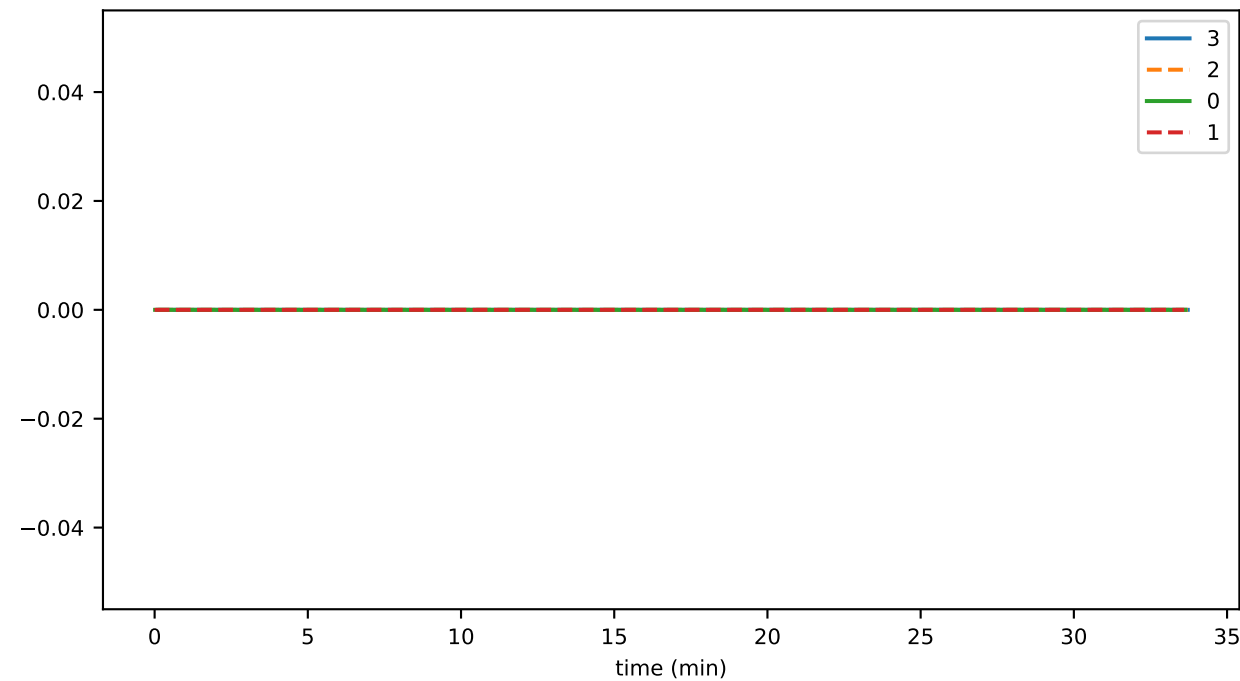
hapiBalanceQueryLimitsPercentUsed
