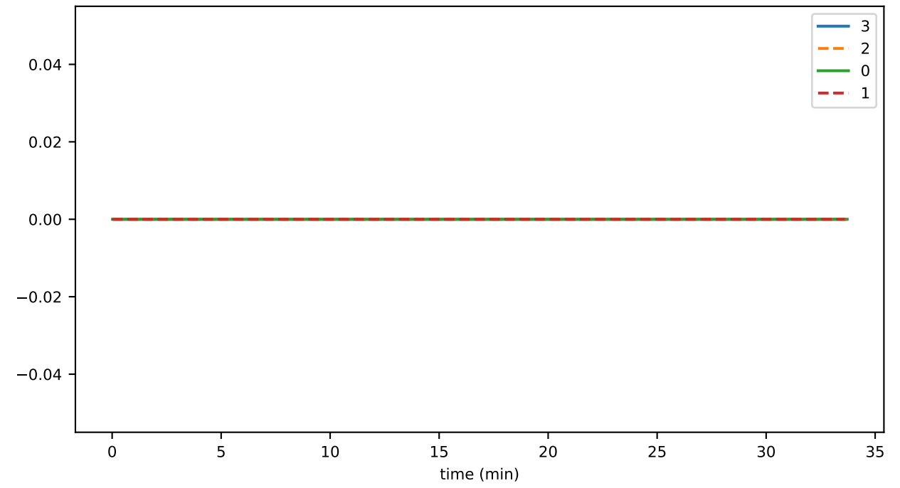
secC2RC
