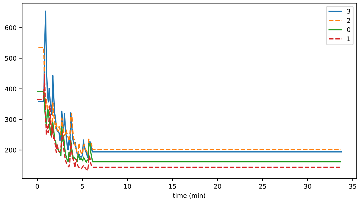
StateHasher_busy_fraction
