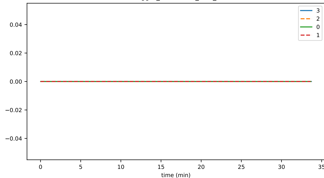
HashLogger_unhandled_task_count
