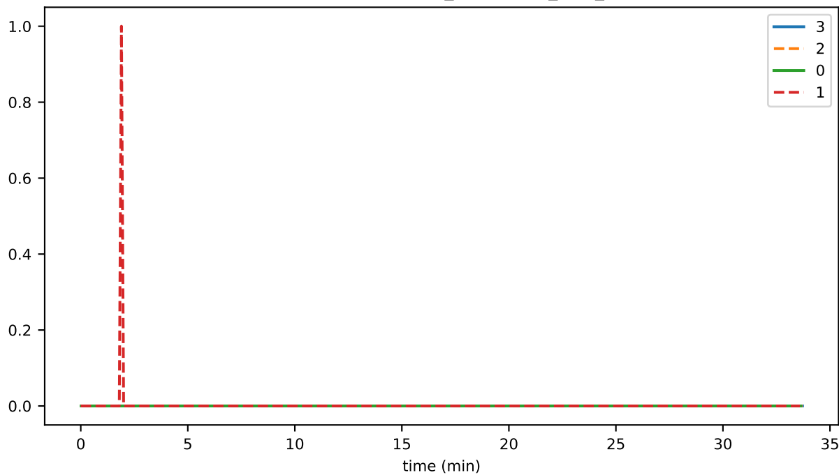
EventSignatureValidator_unhandled_task_count
