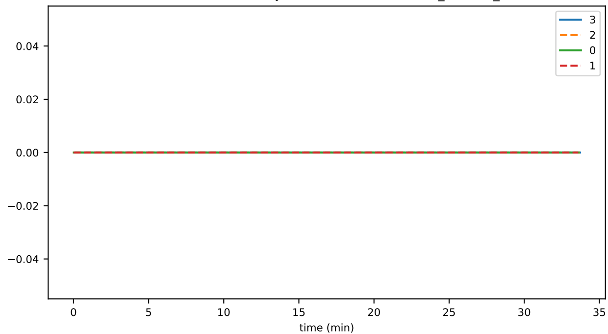
SmartContractService:SystemContractMethodCall_ERC721_total
