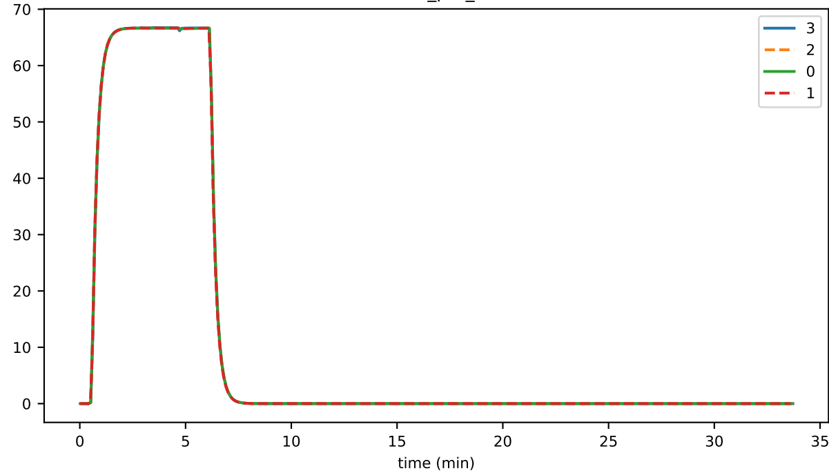
EventSignatureValidator_unhandled_task_count
