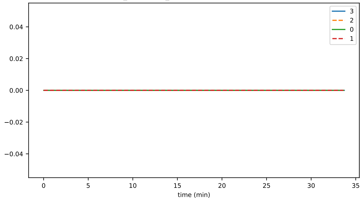
conn_connClose_tooManyEndStreamResponses
