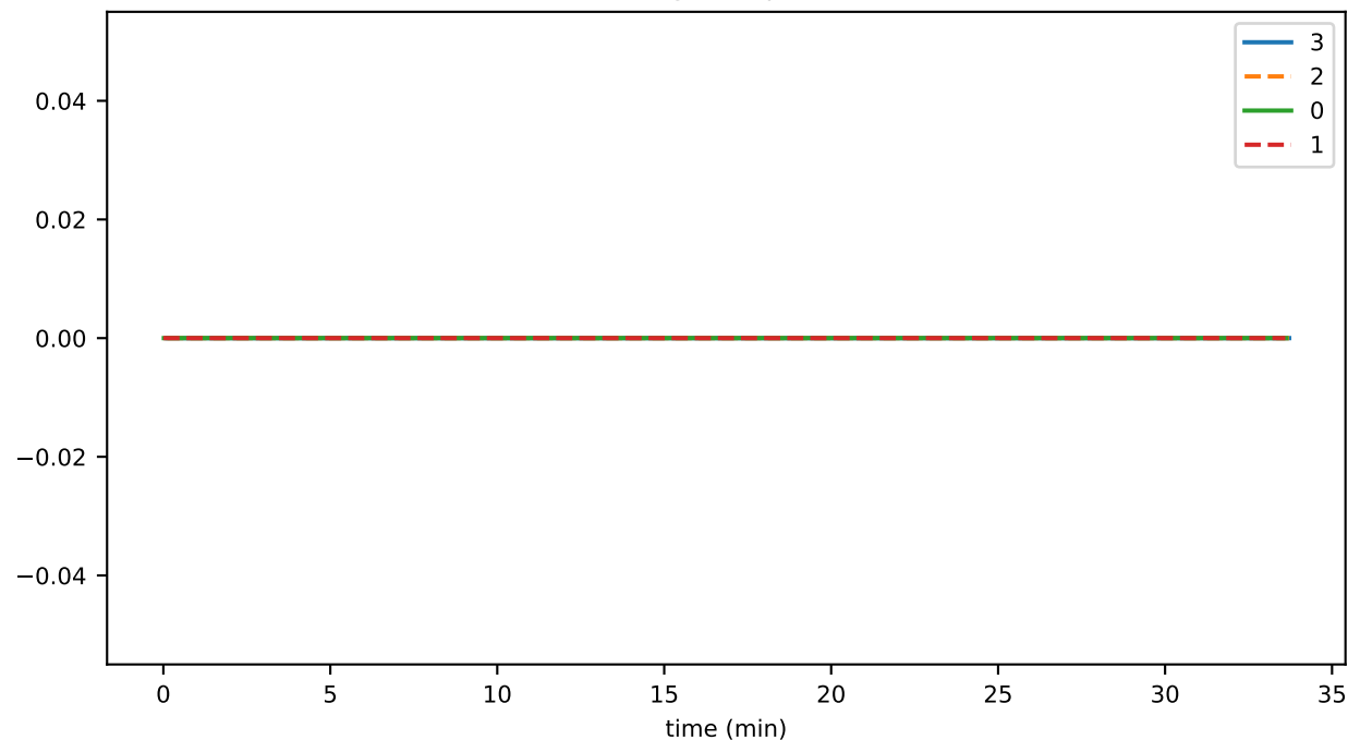
DigSpans_per_sec
