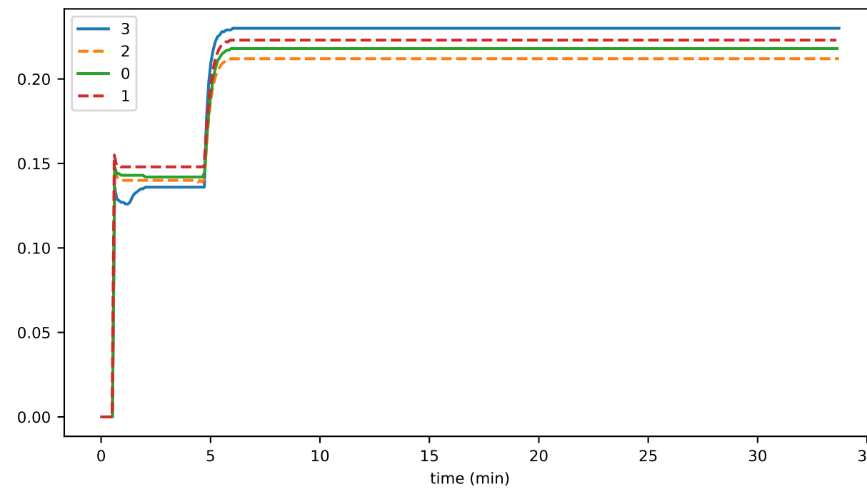
secR2F
