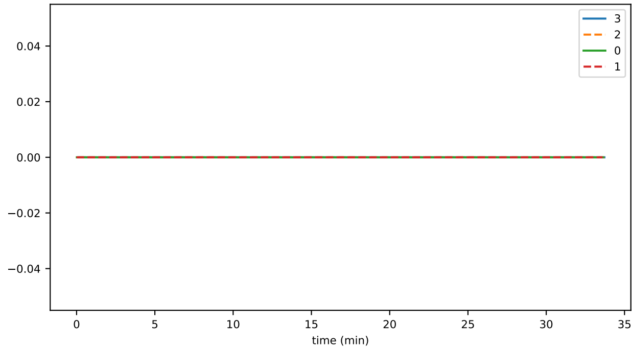
SmartContractService:SystemContractMethodCall_TOKEN_QUERY_total
