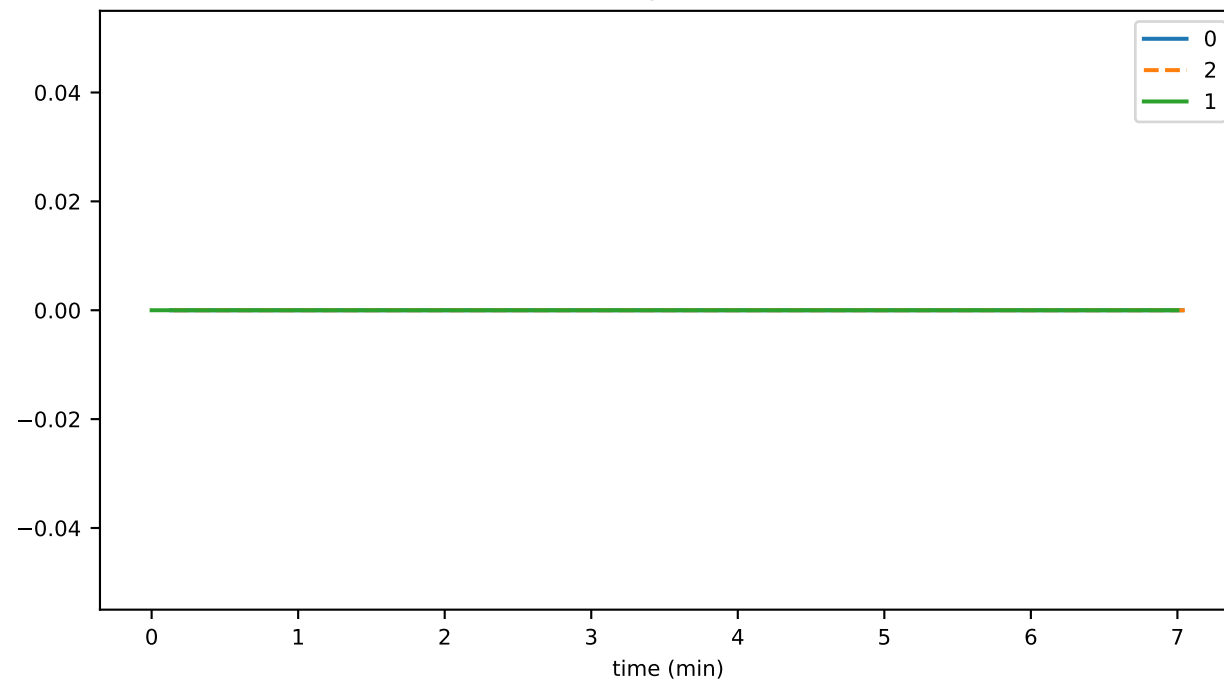
BranchReporter_unhandled_task_count
