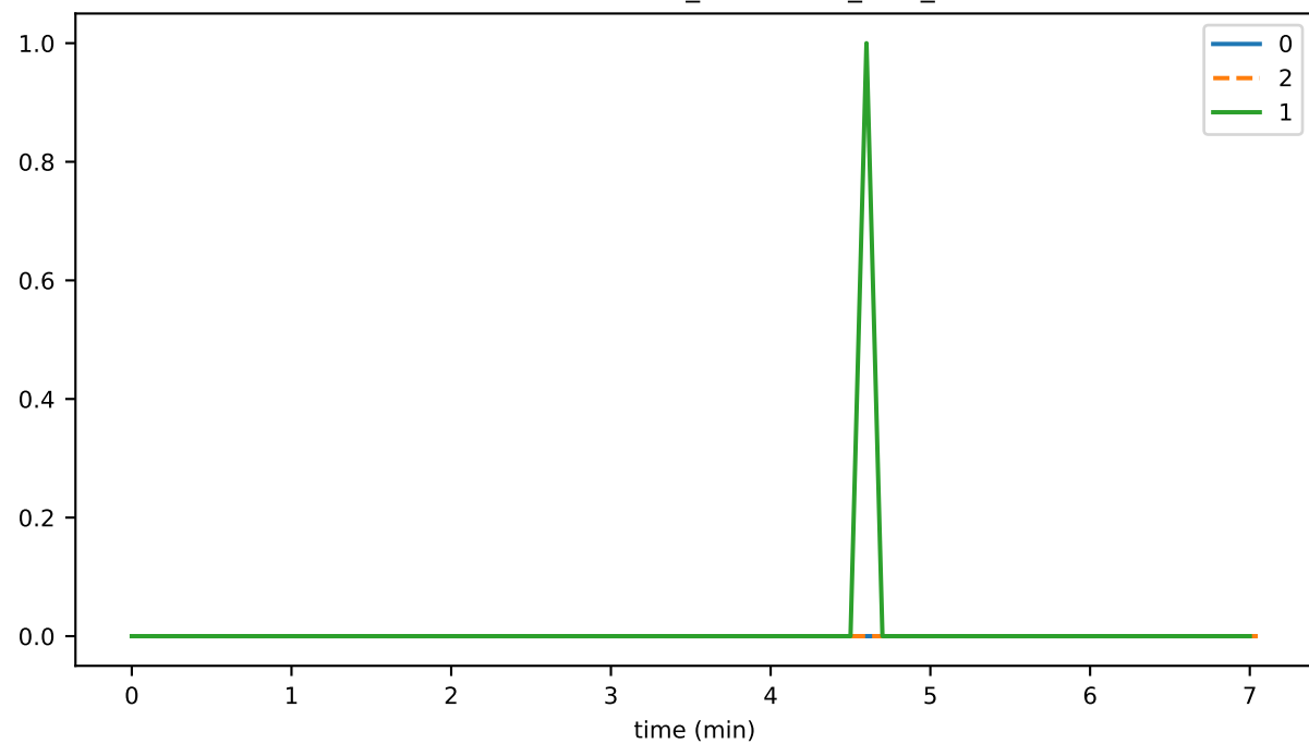
InternalEventValidator_unhandled_task_count
