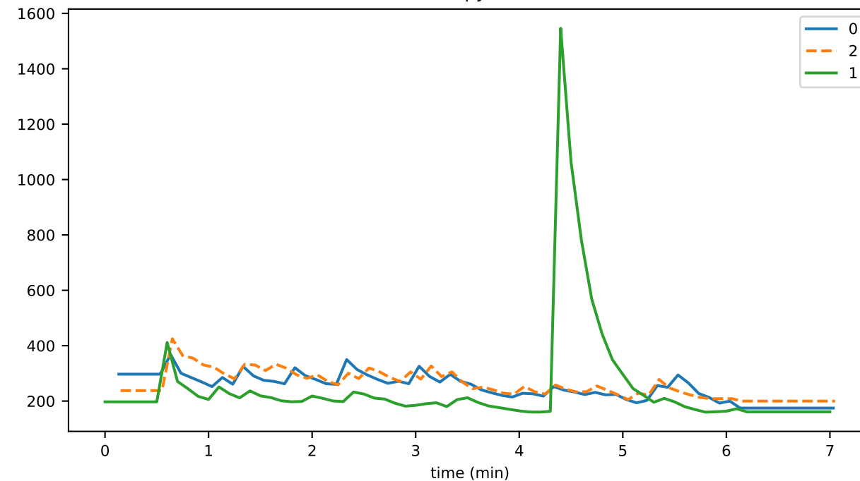
StateHasher_busy_fraction
