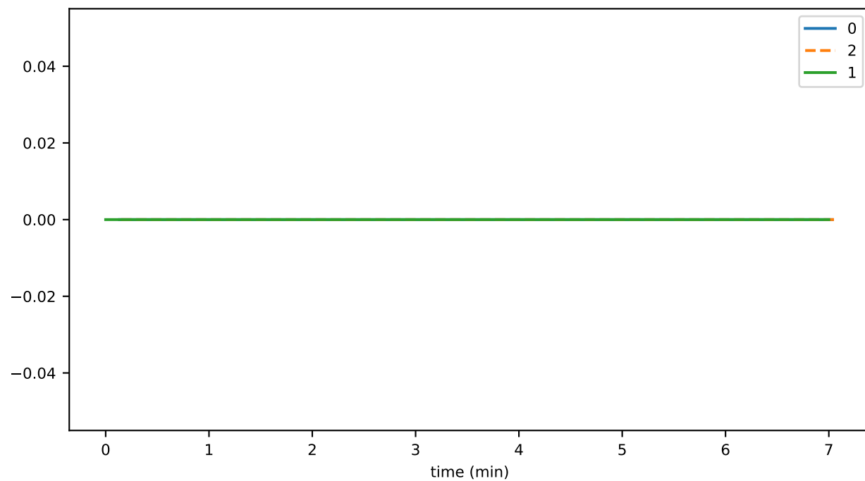
lambdaSStoreThrottledTxns
