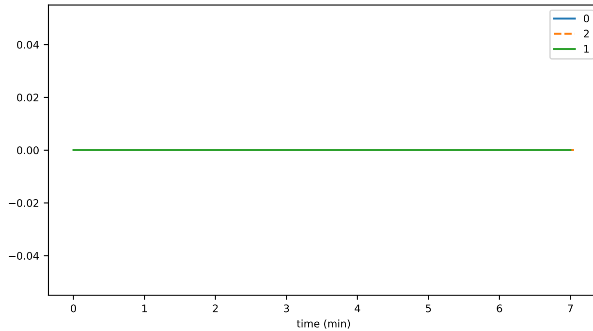
tokenUpdateNftsDurationMax
