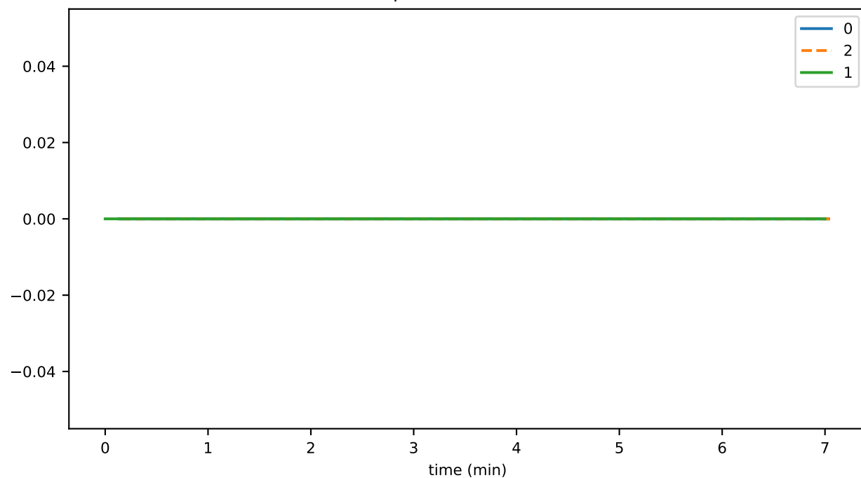
1e6 topicsMaxNumber
