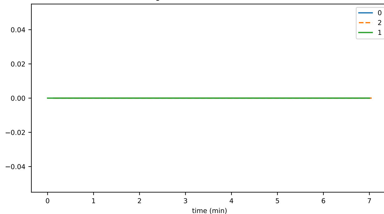
1e18 MaxSigBatchSz
