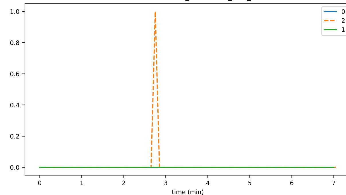
TtIDig
