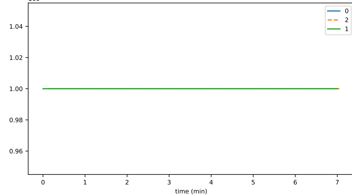
1e6 topicsMaxNumber
