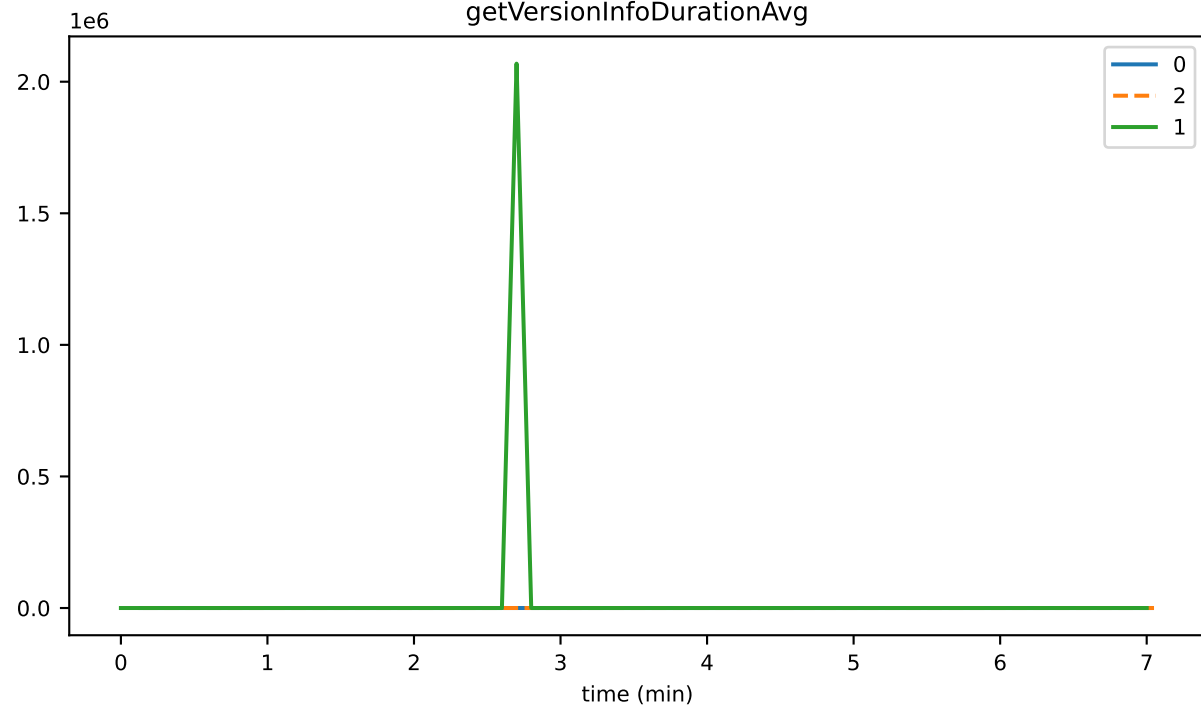
getVersionInfoDurationAvg
