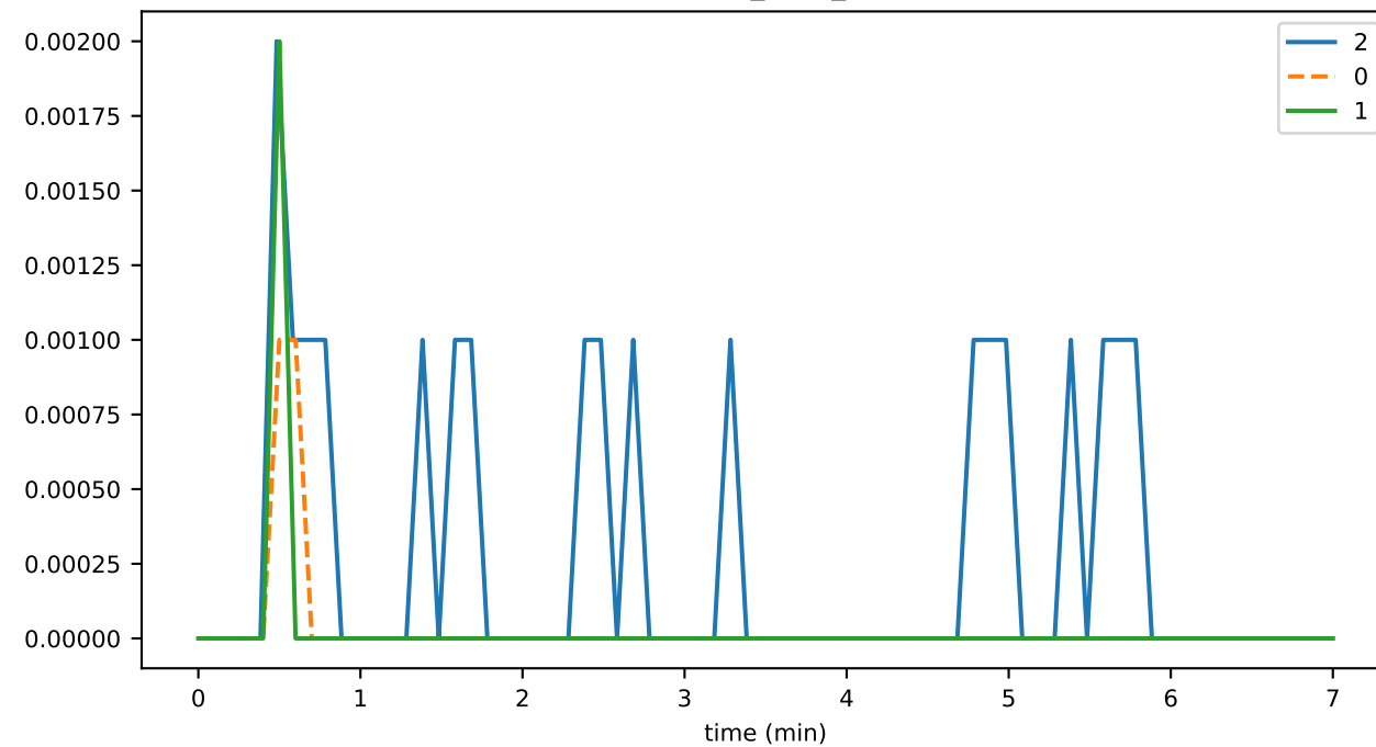
StateHasher_busy_fraction
