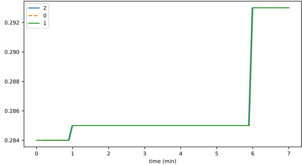
preHandleMicros
