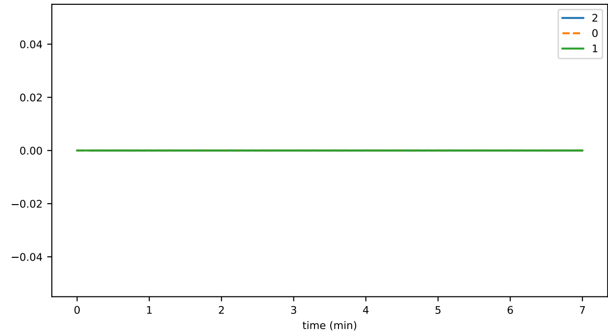
1e18 MaxSigBatchSz
