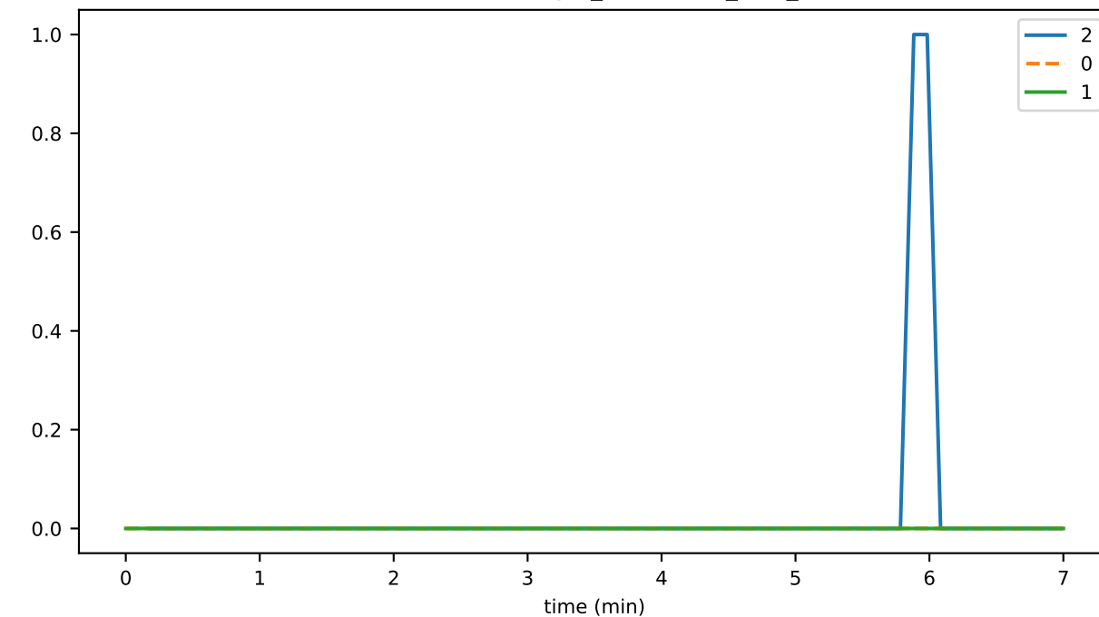
EventDeduplicator_unhandled_task_count
