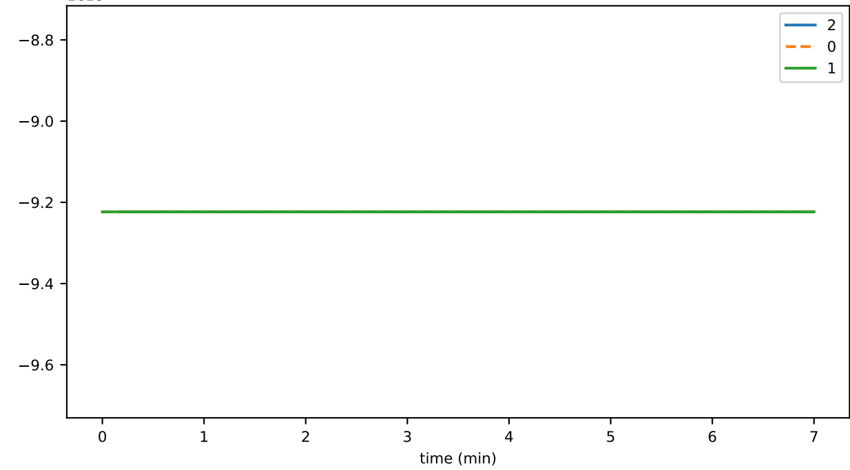
1e18 MaxSigBatchSz
