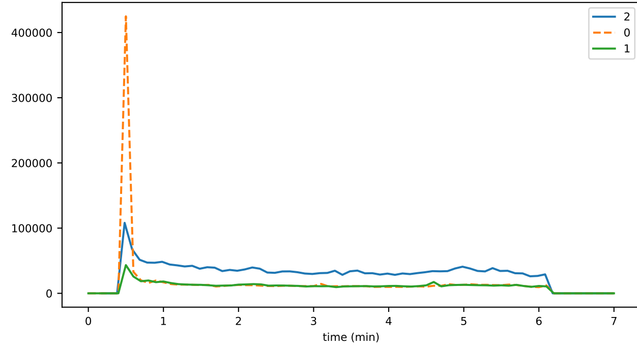
ping_ms_00
