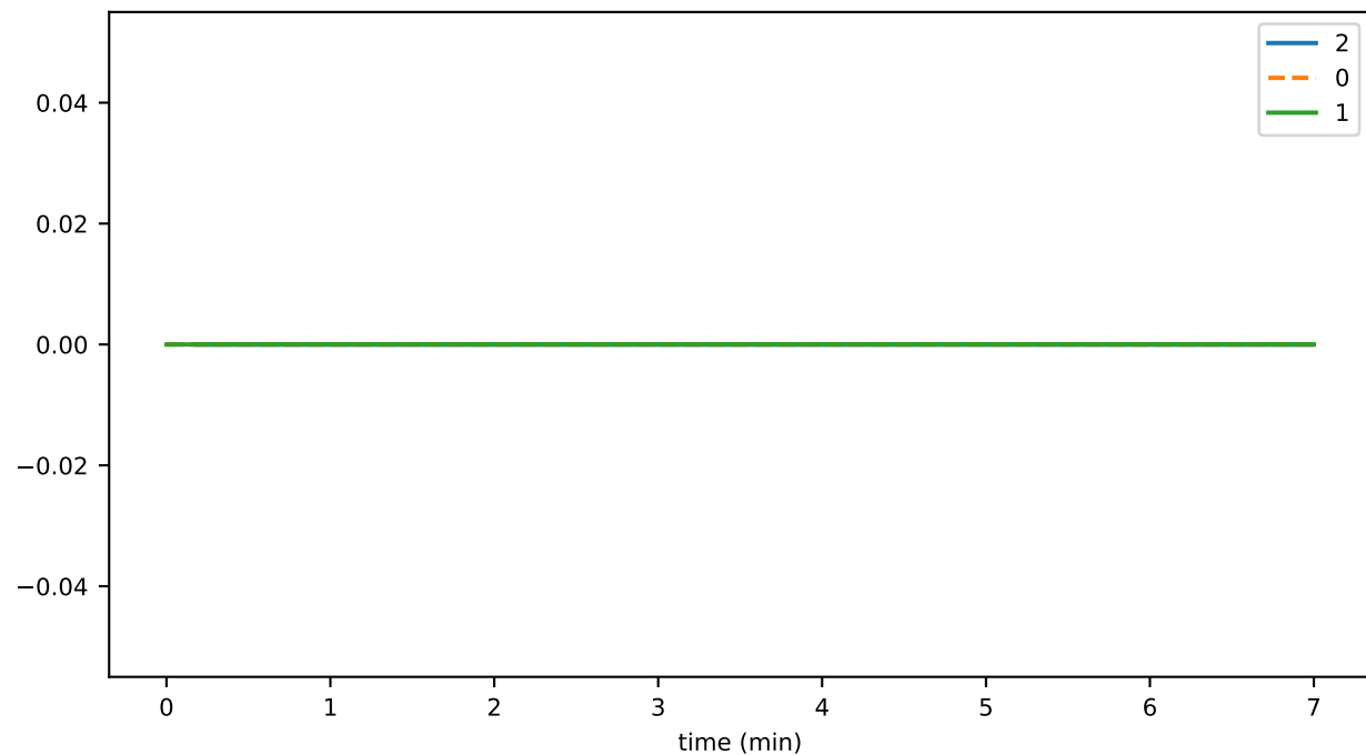
StateGarbageCollector_unhandled_task_count
