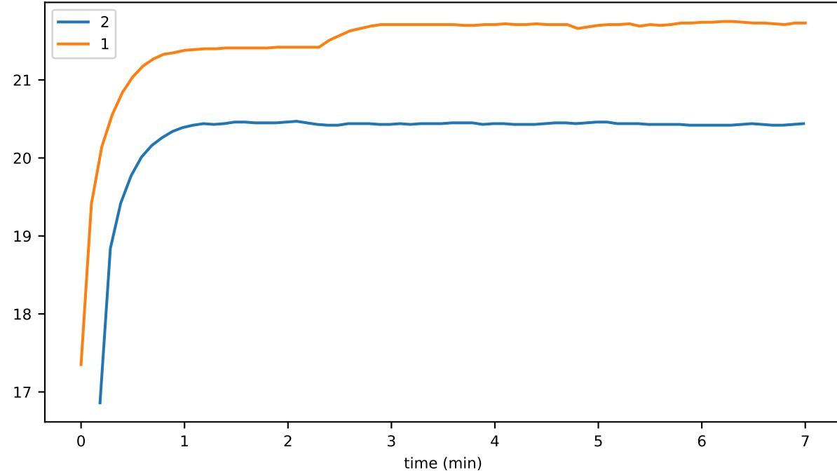
ping_ms_00
