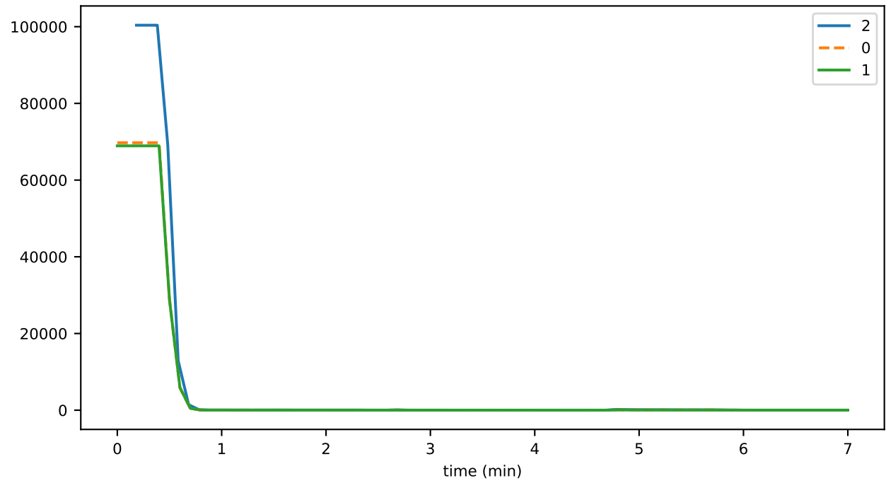
preHandleMicros
