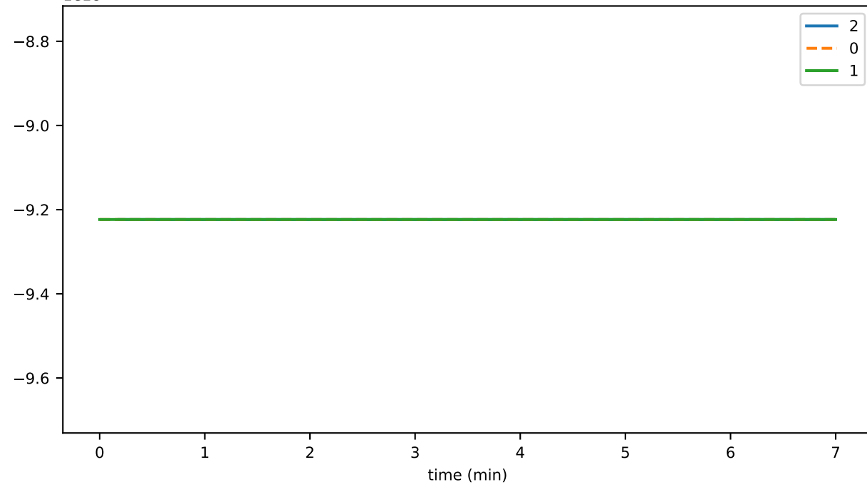
1e18 MaxDigBatchSz
