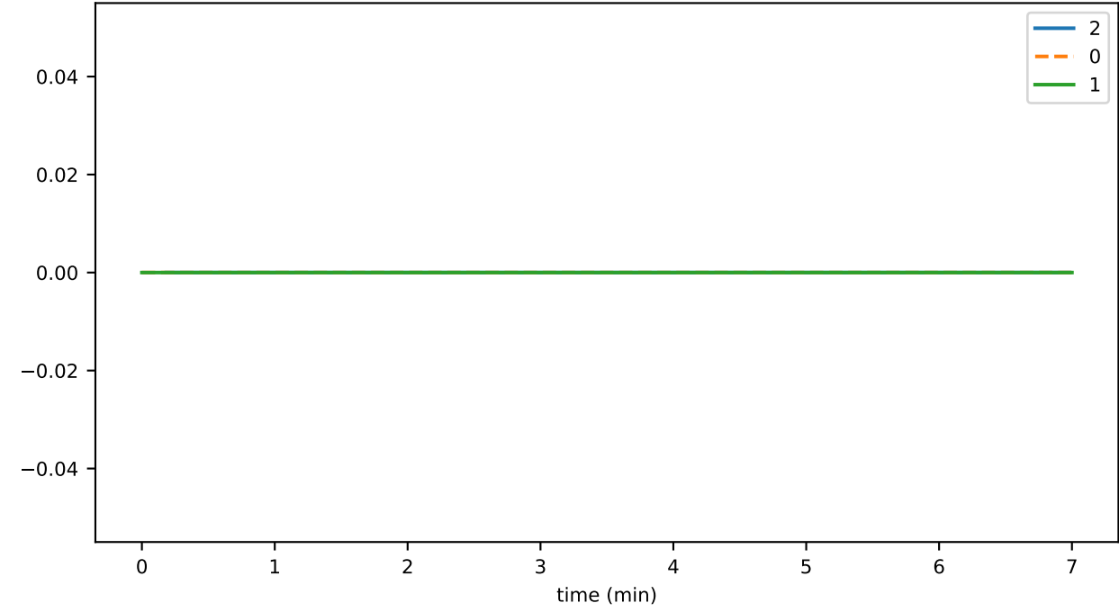
tokenPauseDurationMax
