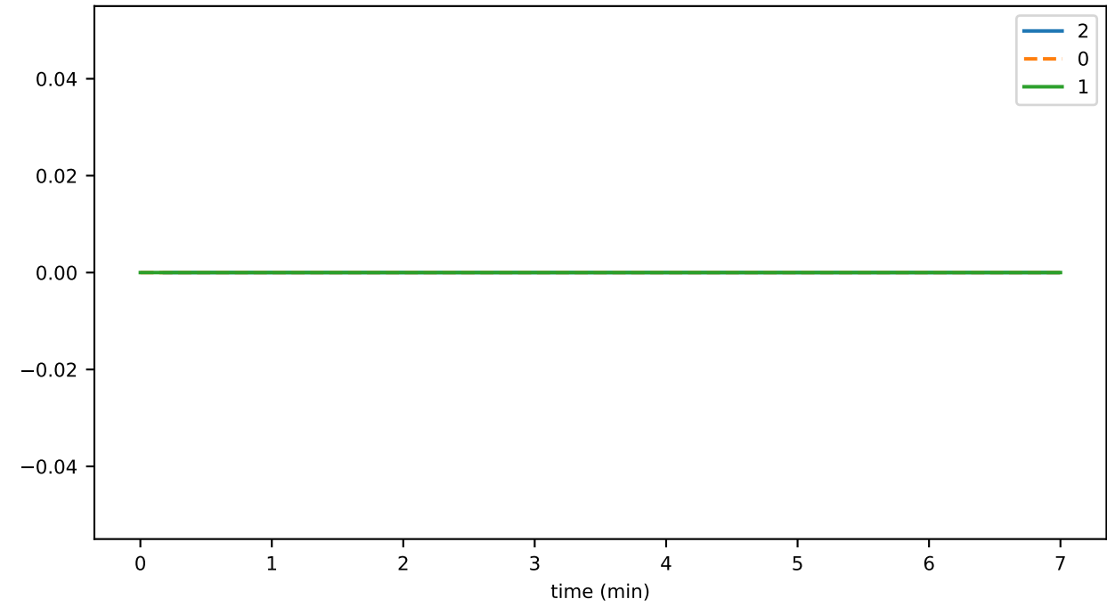
tokenPauseDurationMax
