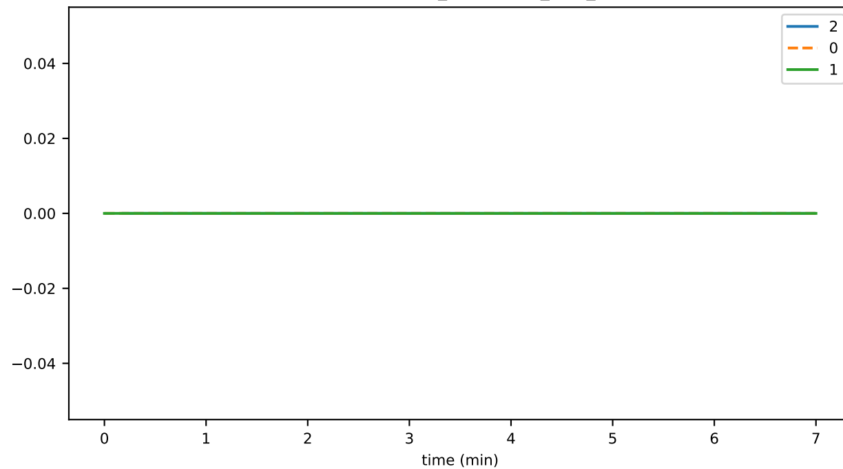
EventDeduplicator_unhandled_task_count
