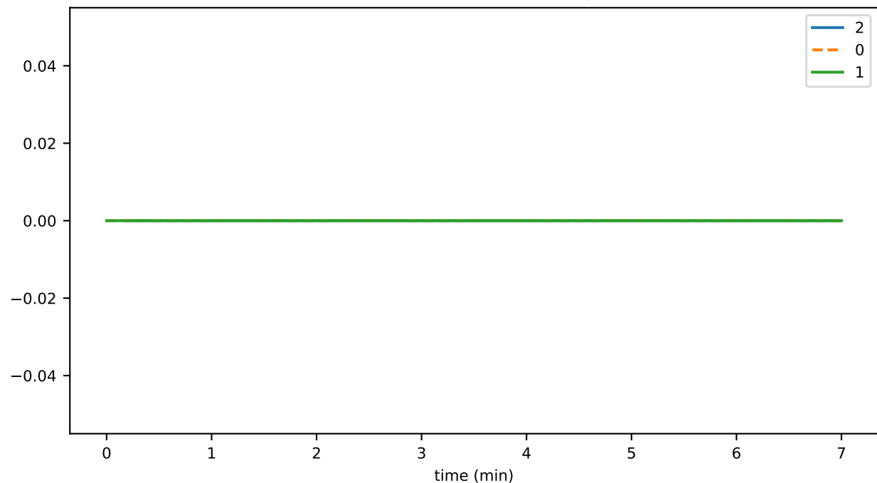
lambdaSStoreThrottledTxns
