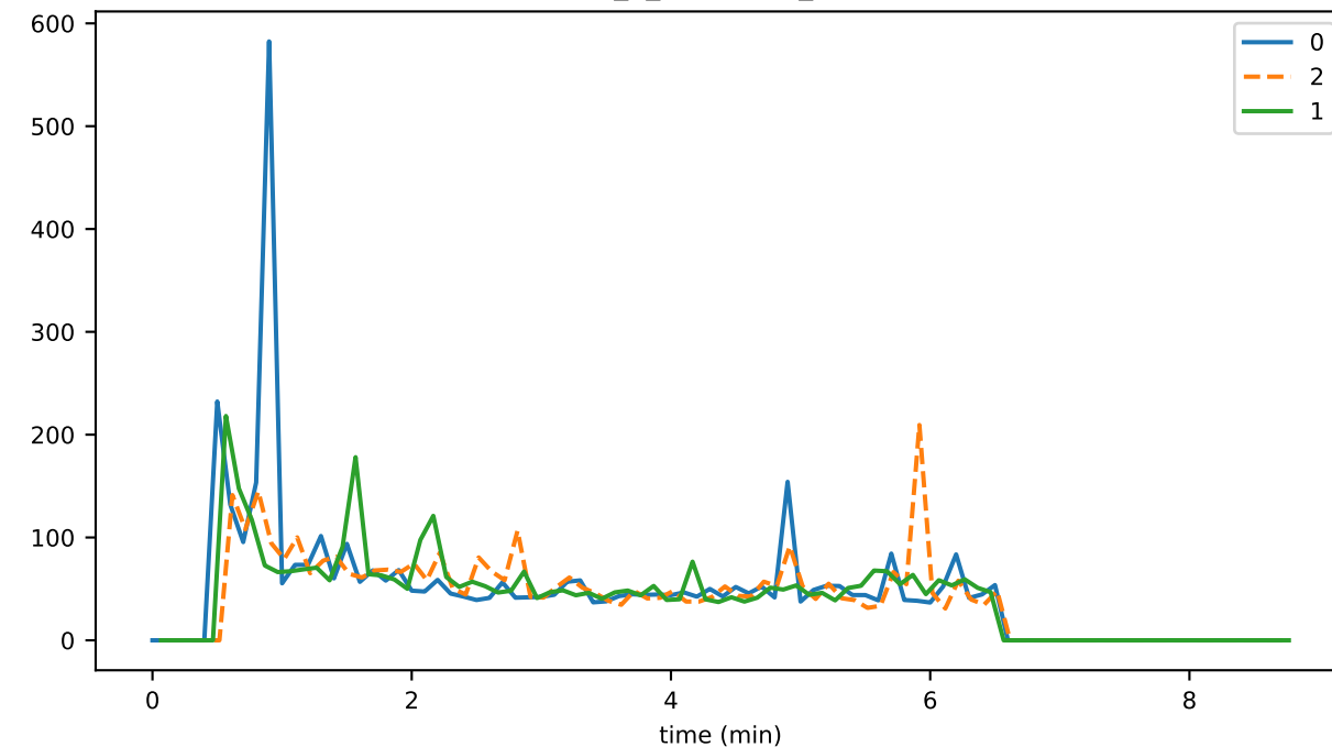
eventDelay_2_validation_runtimeMAX
