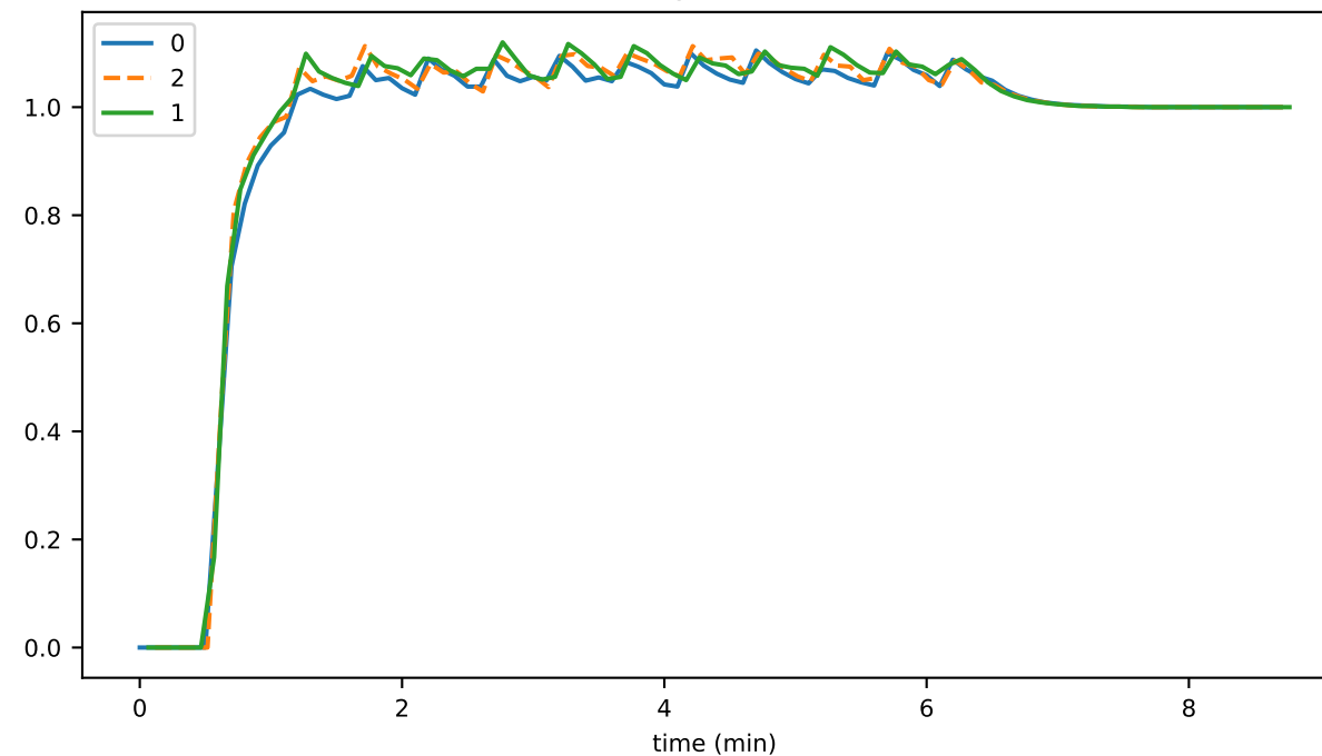
stateToDisk
