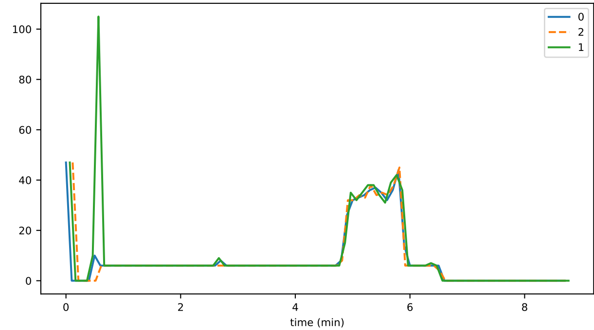
dupEv_per_sec
