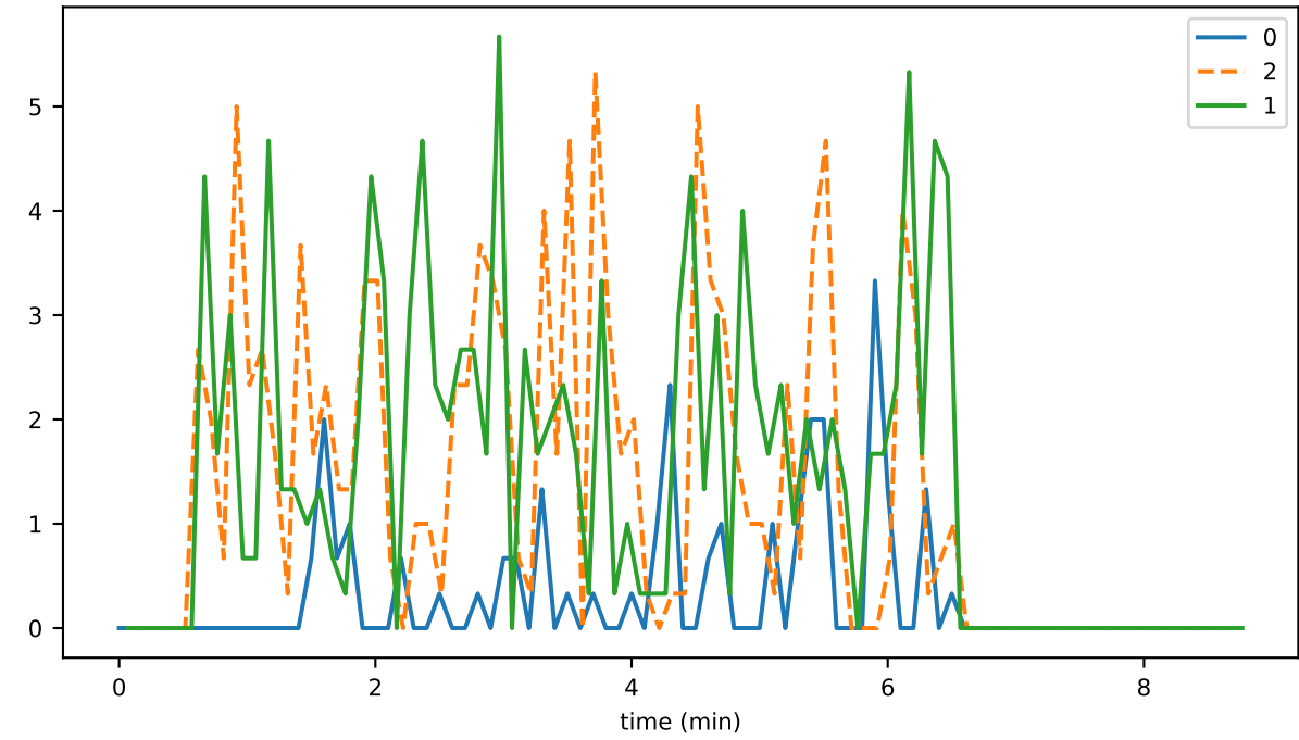
dupEv_per_sec
