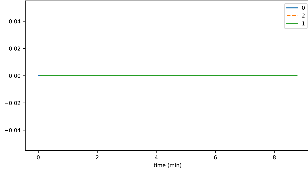
contractUpdateThrottledTxns
