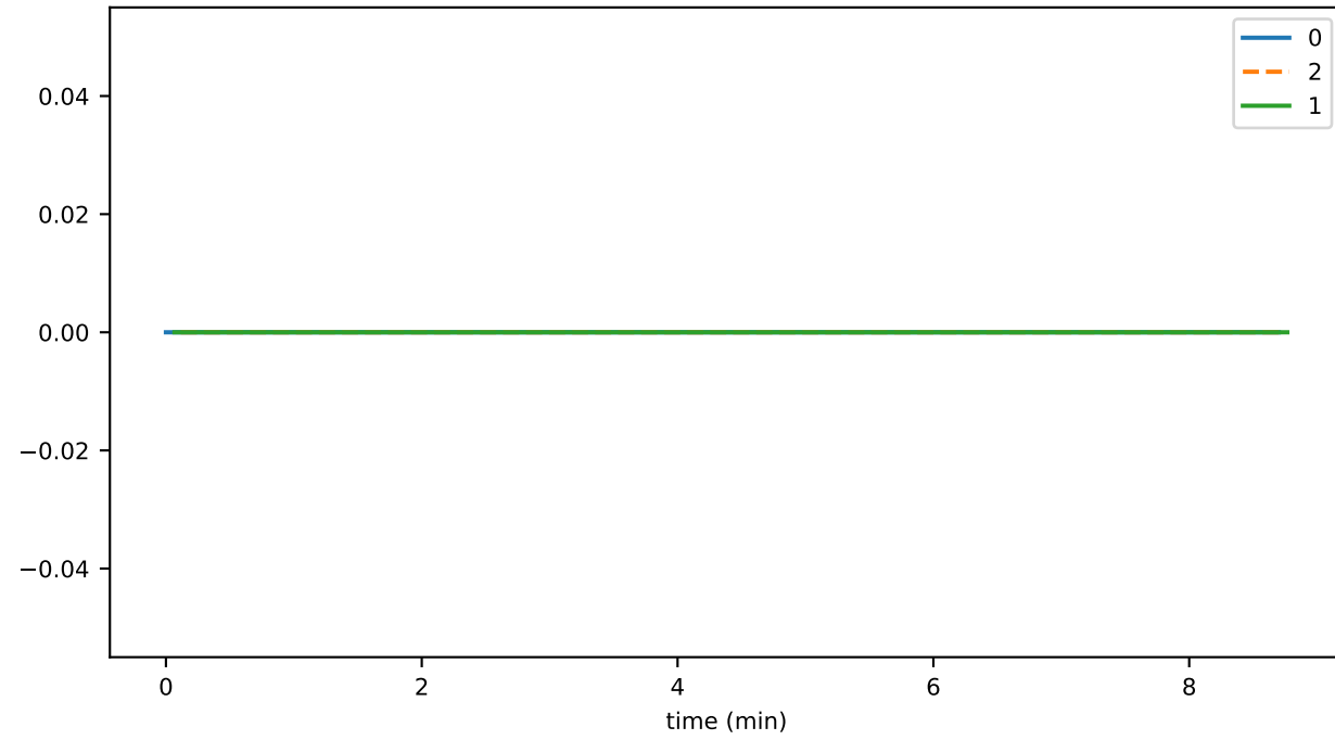
contractUpdateThrottledTxns
