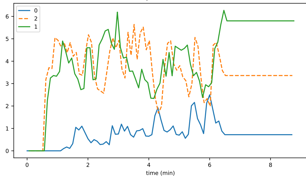
endsReconnectAsSender
