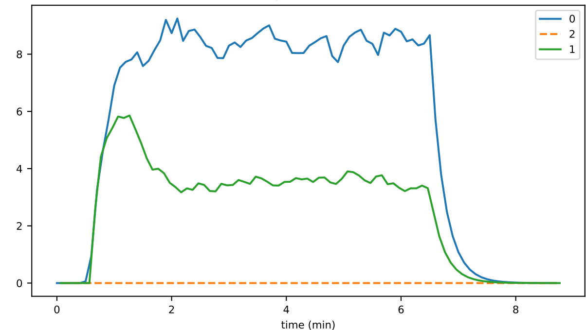
tokenAccountWipeDurationMax
