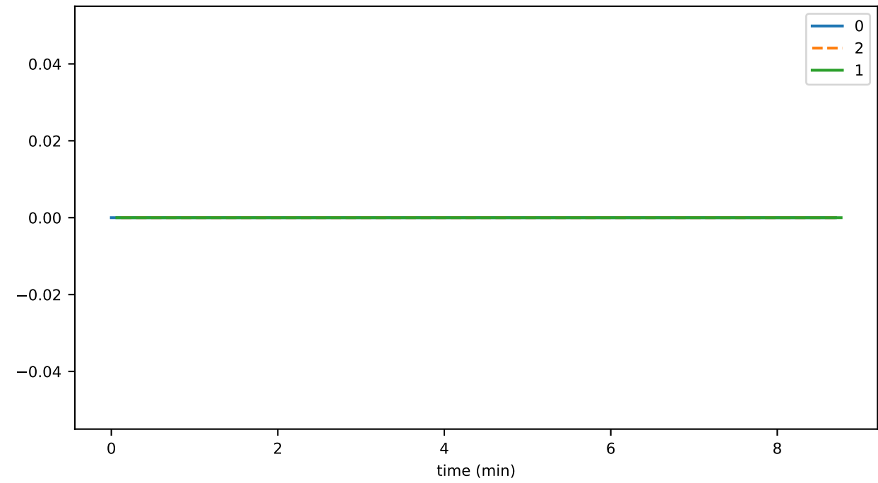
fileAppendDurationMax
