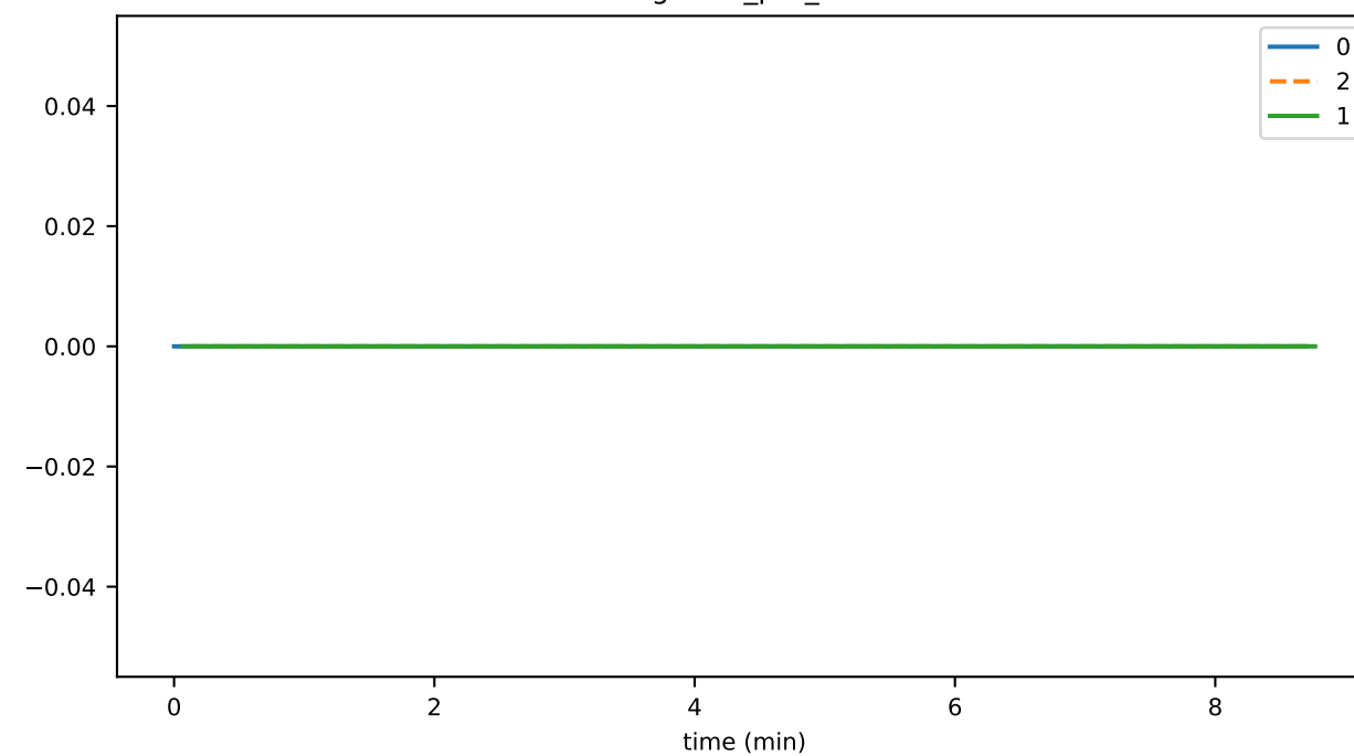
DigPulse_per_sec
