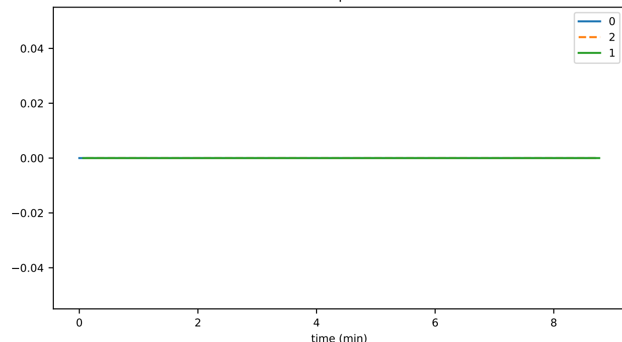
tokenAccountWipeThrottledTxns
