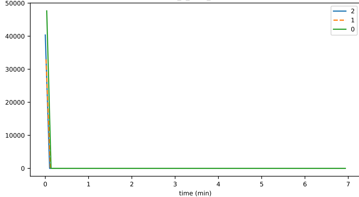
eventDelay_6_pces_storageMAX
