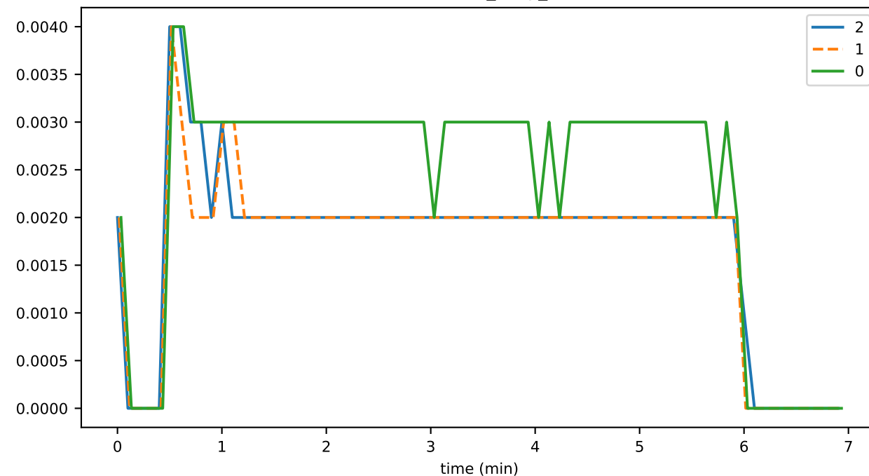
InternalEventValidator_unhandled_task_count
