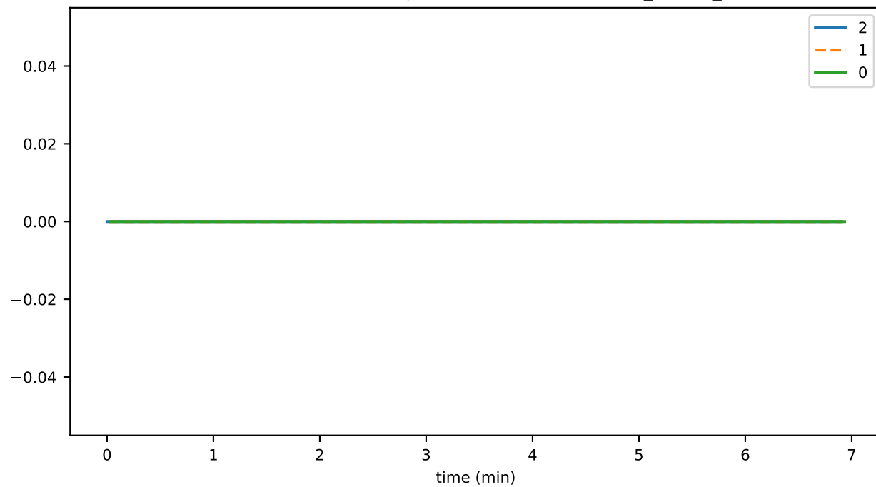
SmartContractService:SystemContractMethodCall_ERC721_total
