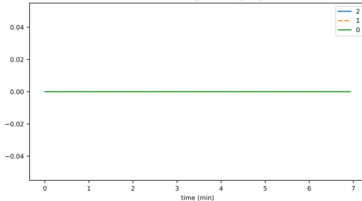
InternalEventValidator_unhandled_task_count
