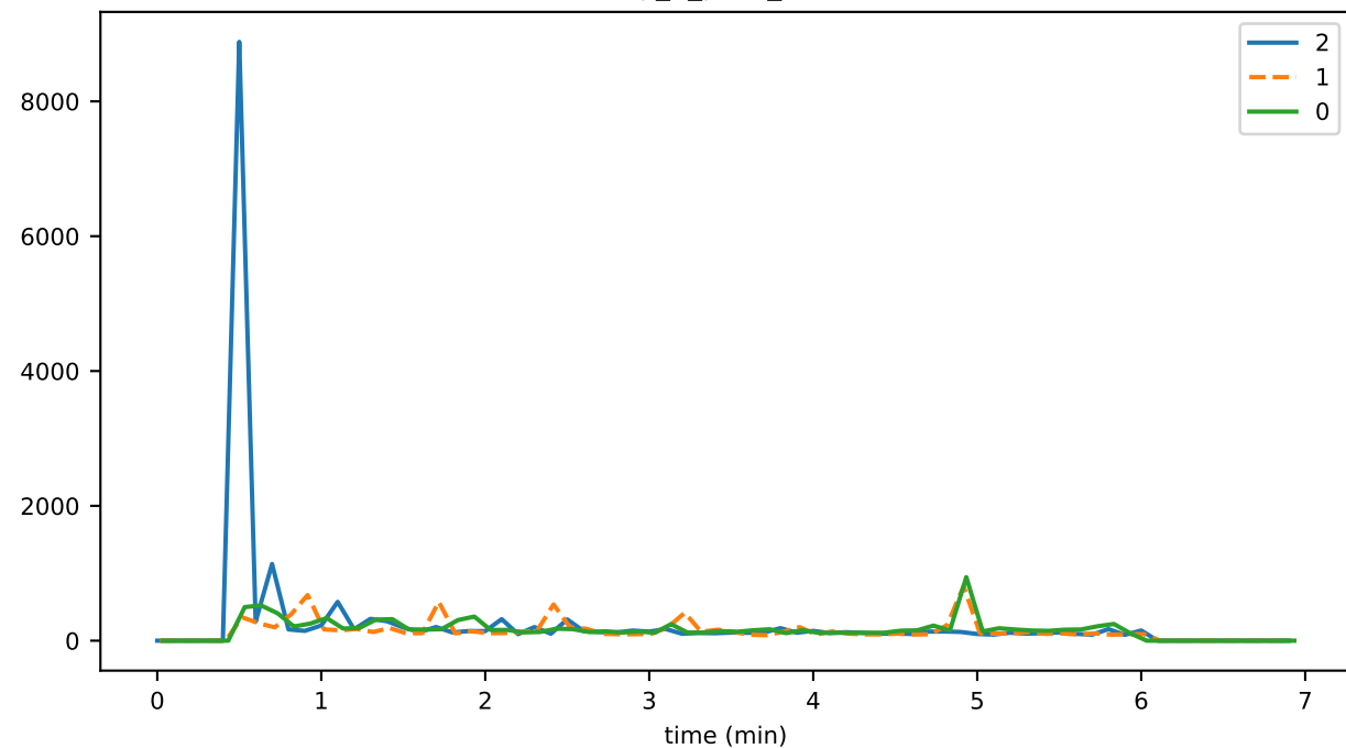
eventDelay_6_pces_storageMAX
