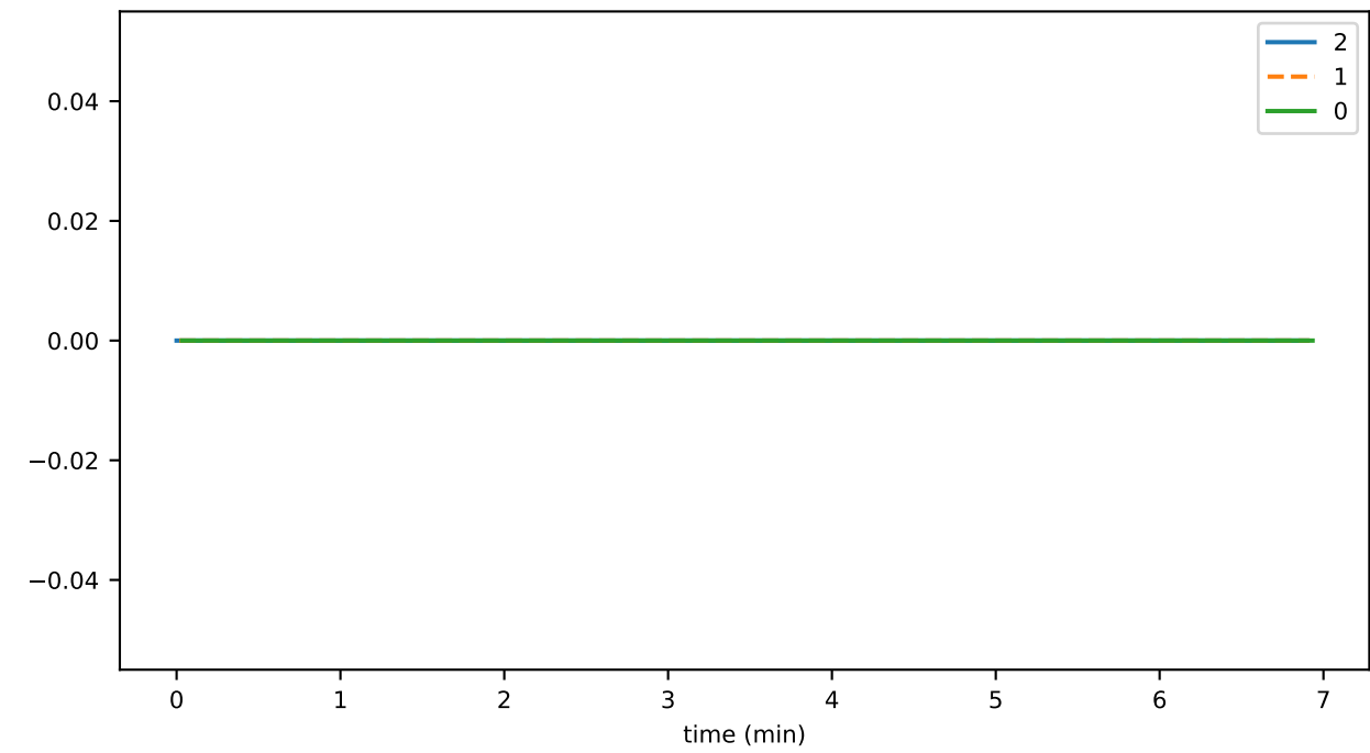
contractAutoRenewThrottledTxns
