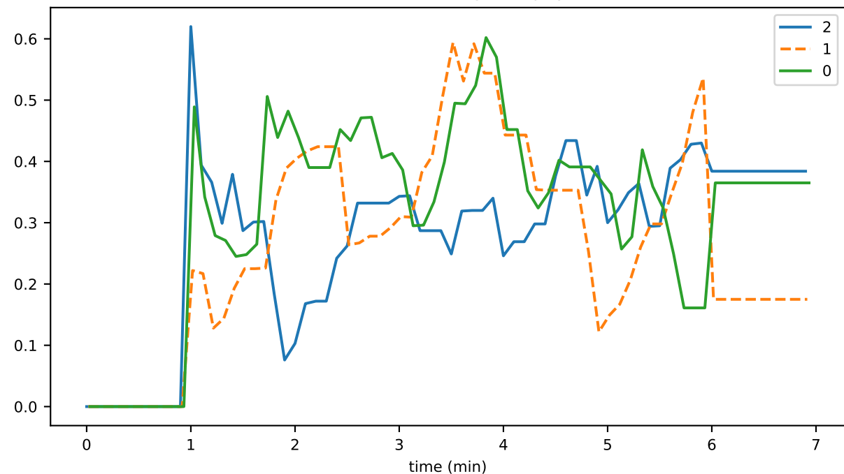
InlinePcesWriter_unhandled_task_count
