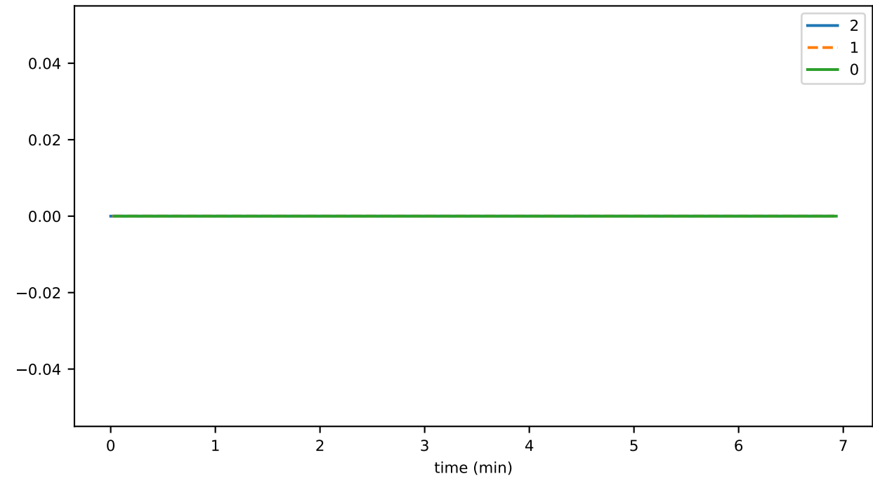
tokensPercentUsed
