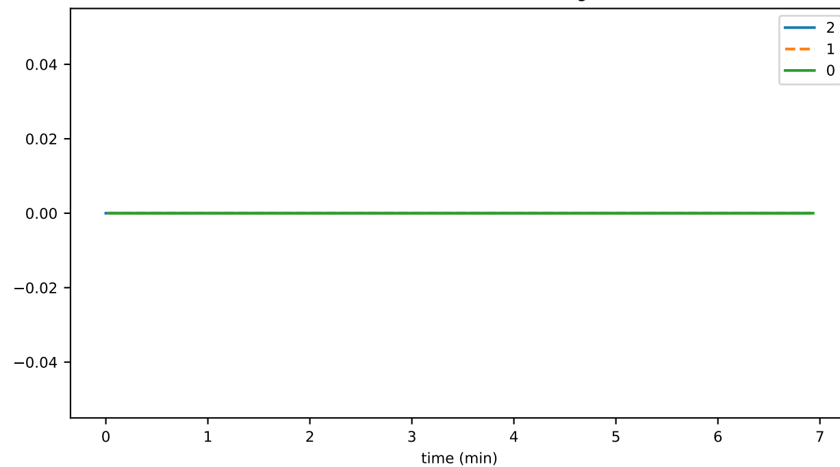
tokenGetNftInfosDurationAvg
