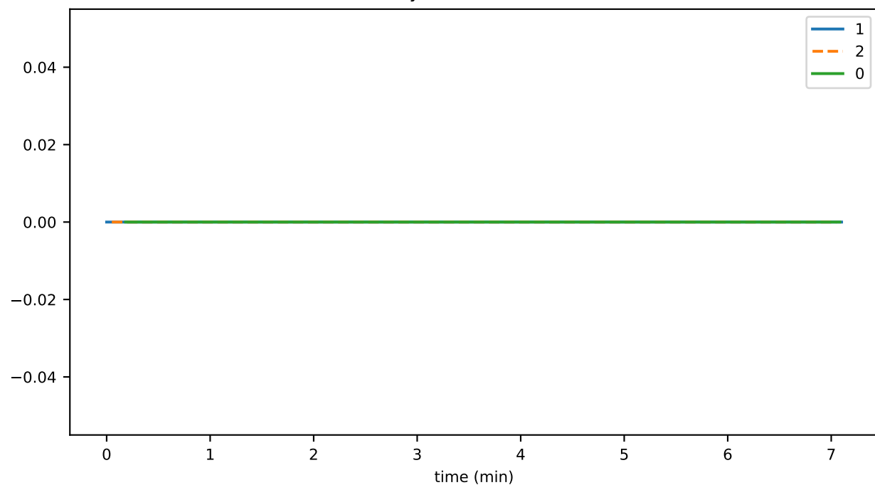
1e6 tokensMaxNumber
