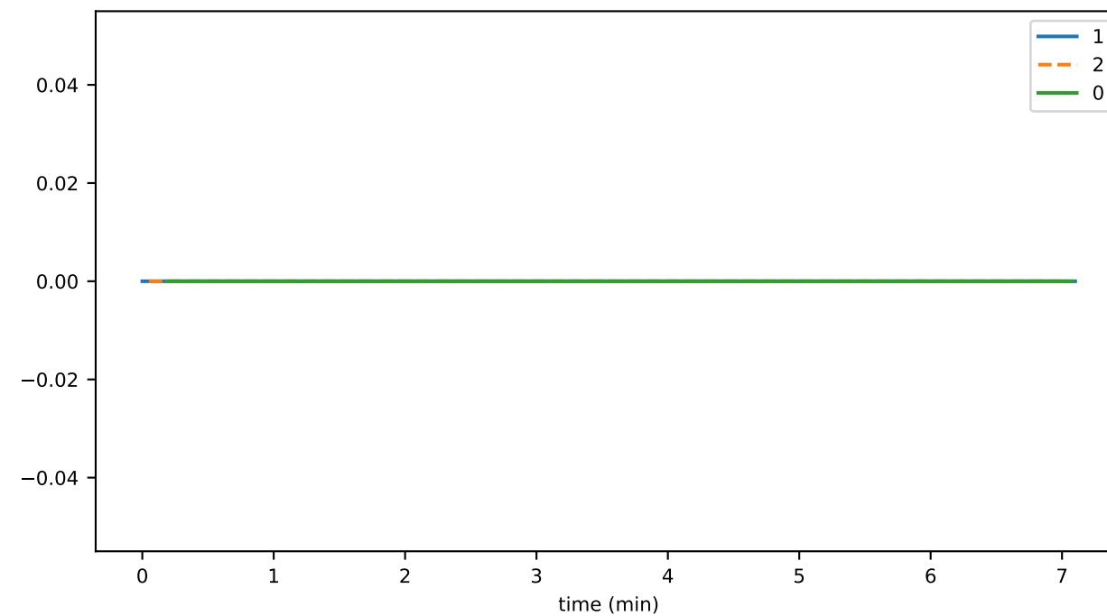
tokenGetInfoDurationMax
