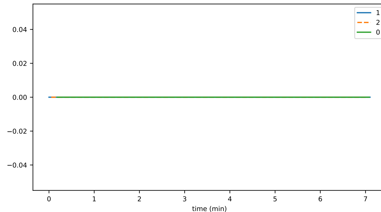
tokenGetInfoDurationMax
