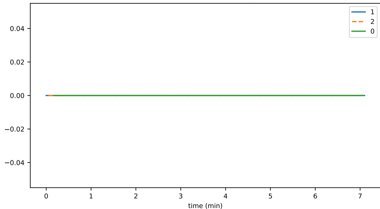
tokenRejectThrottledTxns
