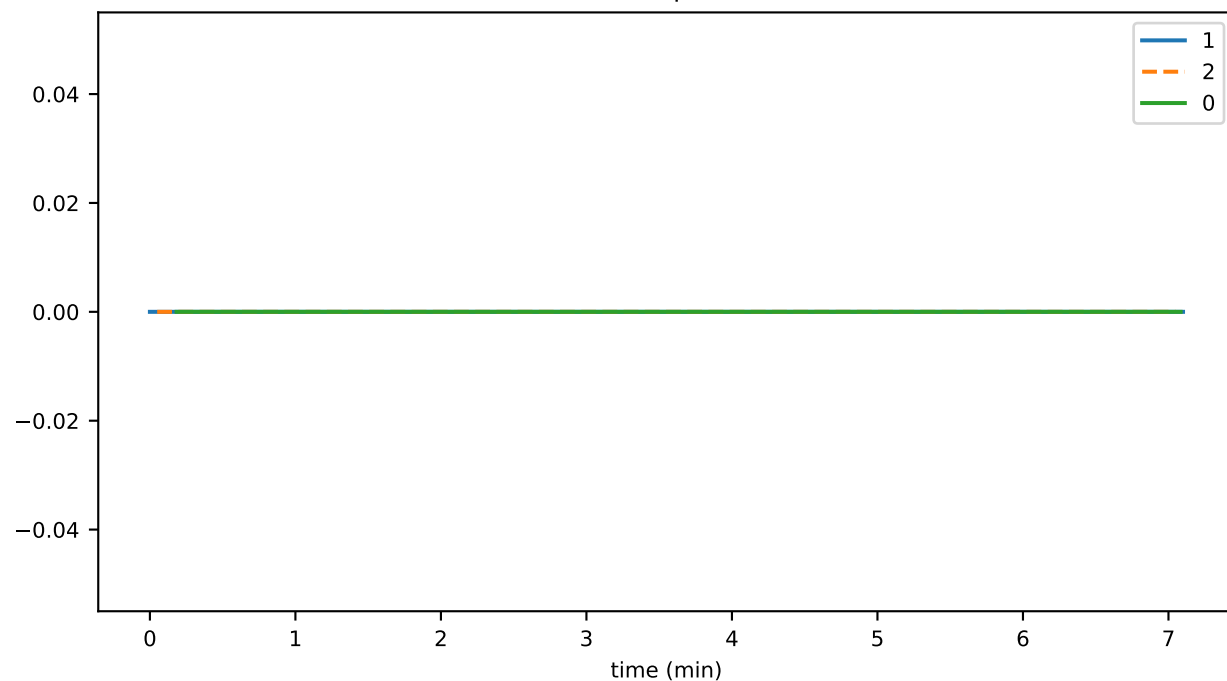
tokenFeeScheduleUpdateDurationMax
