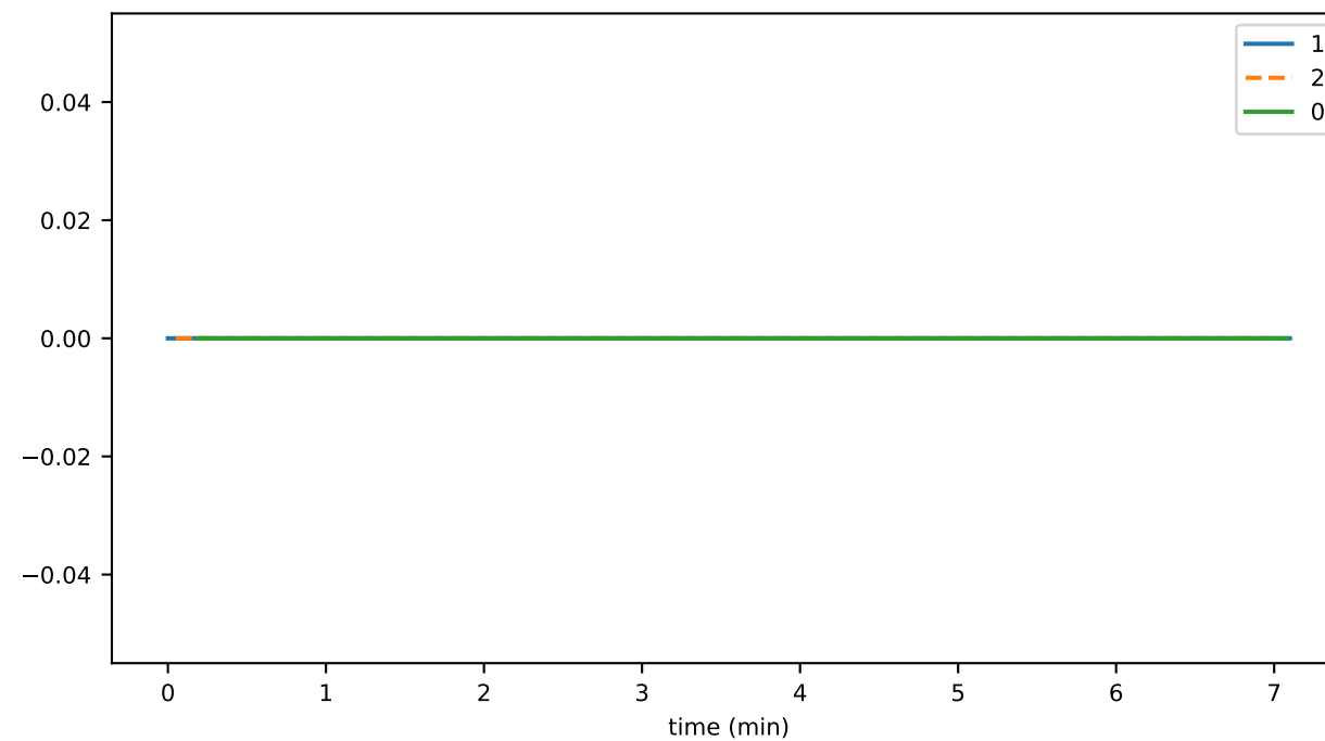
lambdaSStoreThrottledTxns
