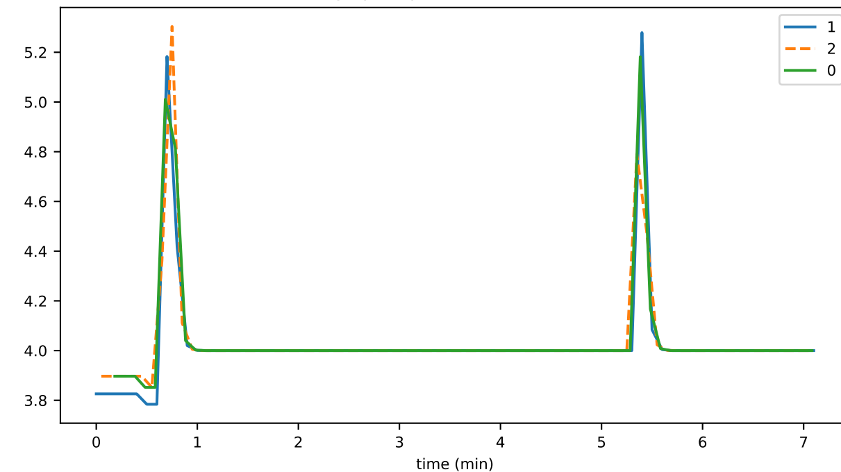
hapiBalanceQueryLimitsPercentUsed
