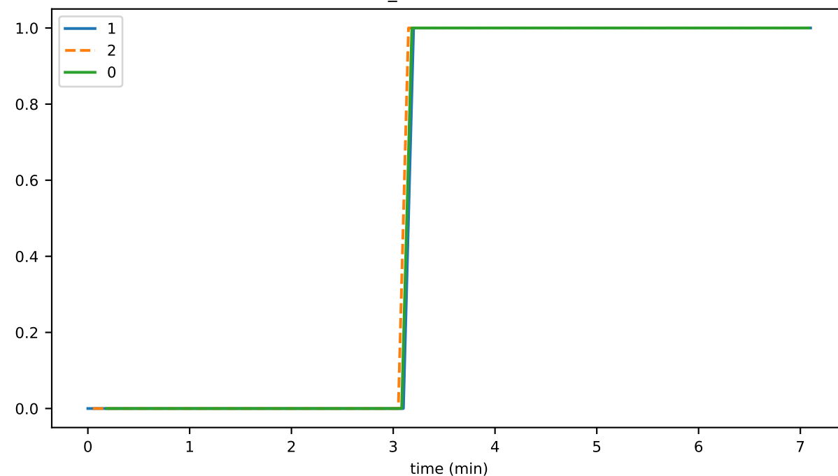
buffer_blockItemBytes
