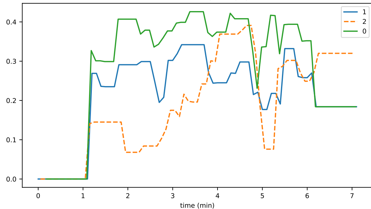
InlinePcesWriter_unhandled_task_count
