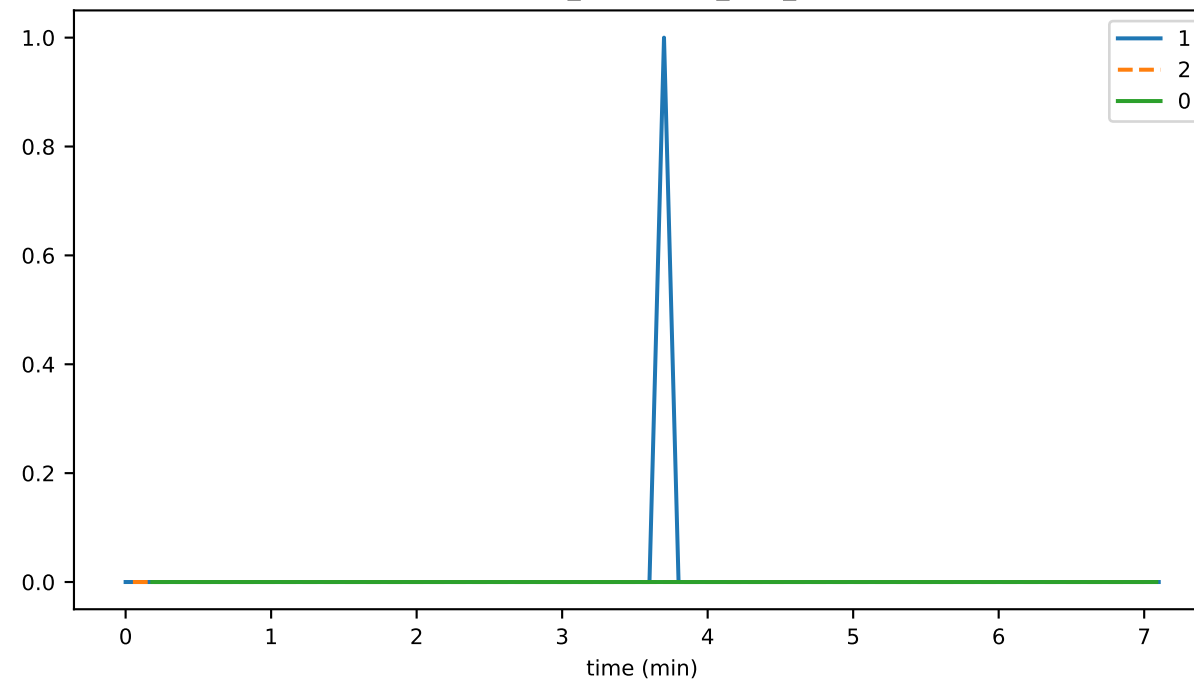
HashLogger_unhandled_task_count
