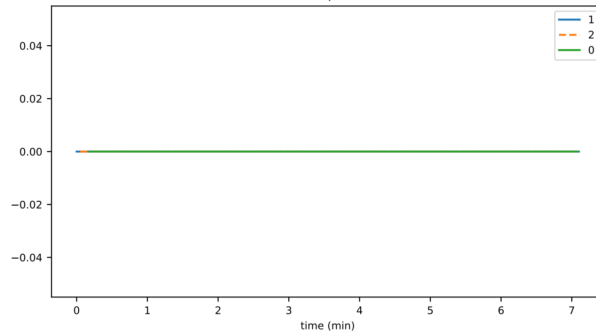
tokenFeeScheduleUpdateThrottledTxns
