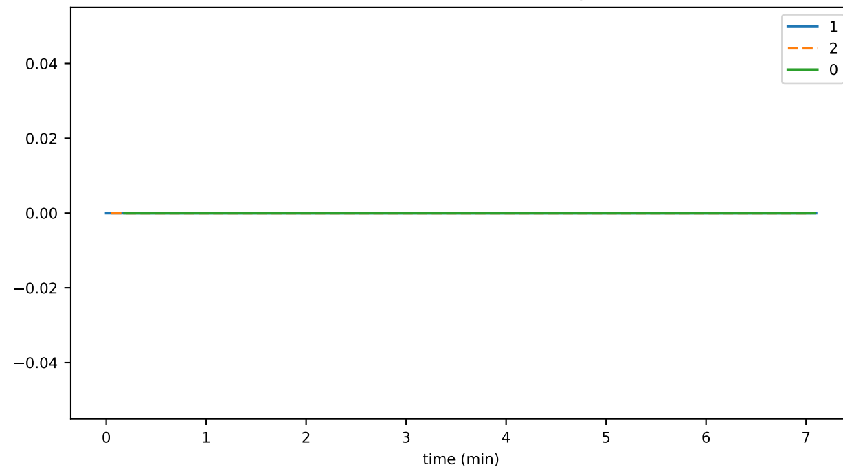
scheduleGetInfoThrottledTxns
