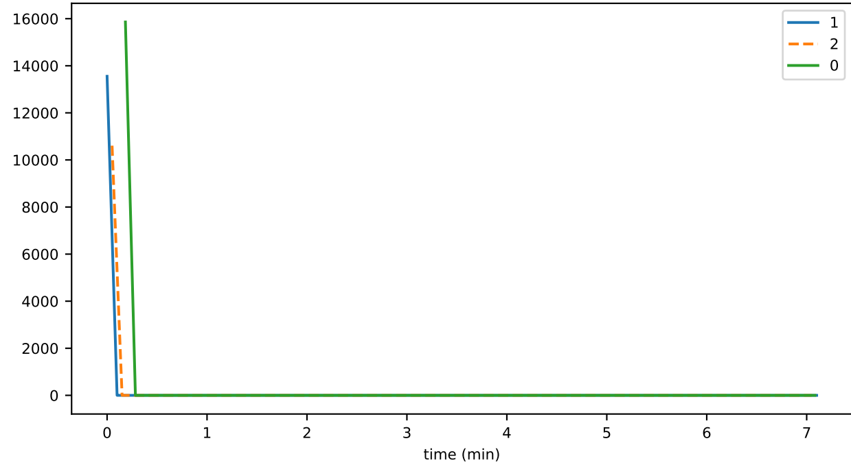
eventDelay_2_validation_gossipMAX
