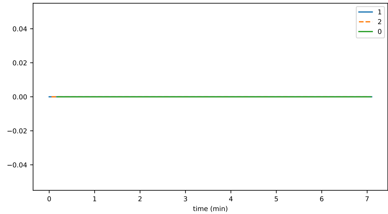
hintsPreprocessingVoteDurationMax
