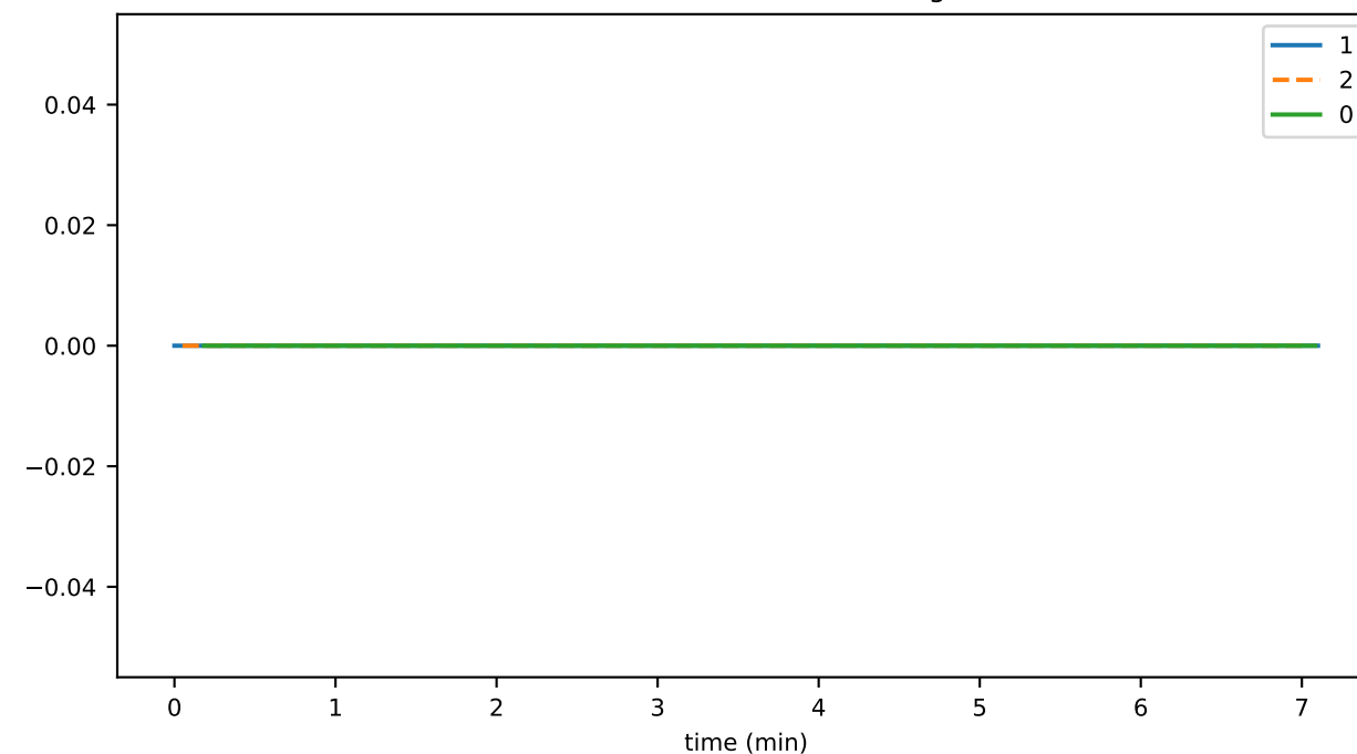
tokenGetNftInfosDurationAvg
