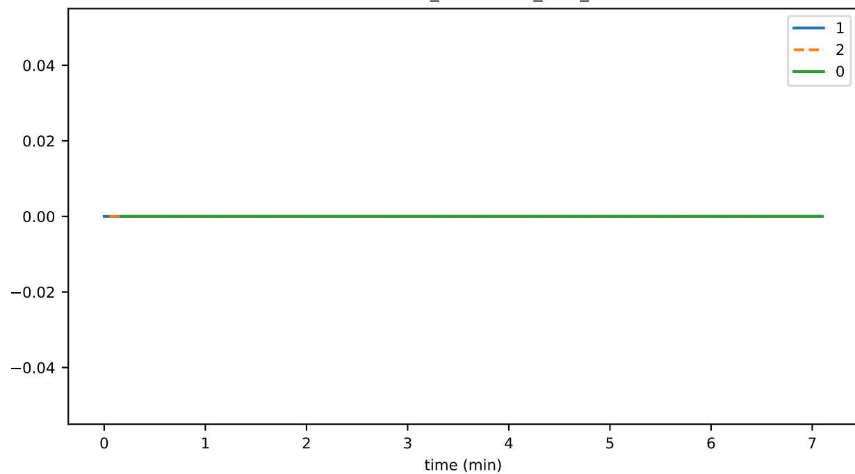
InlinePcesWriter_unhandled_task_count
