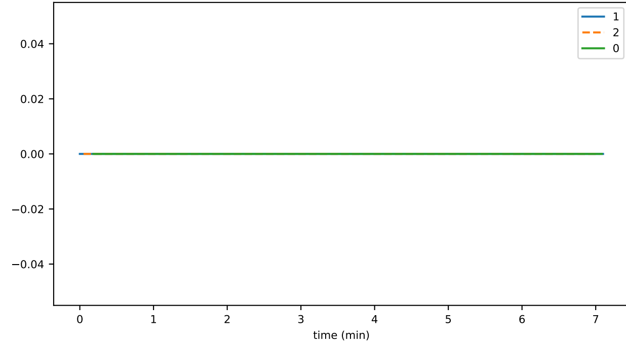
TransactionHandler_unhandled_task_count
