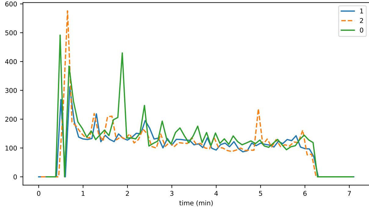
eventDelay_2_validation_gossipMAX
