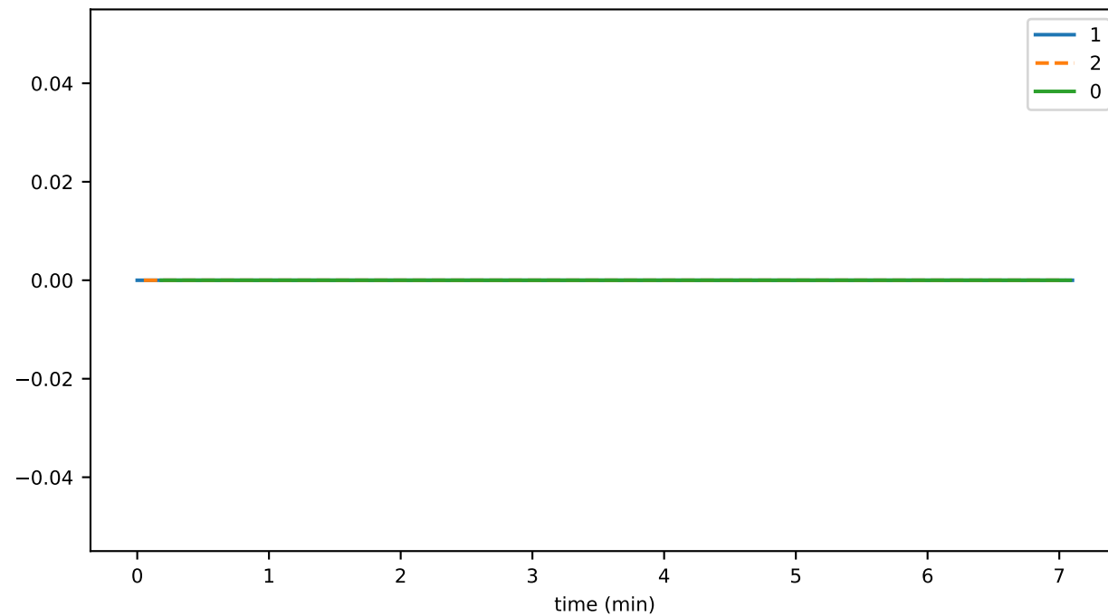
contractsUsed
