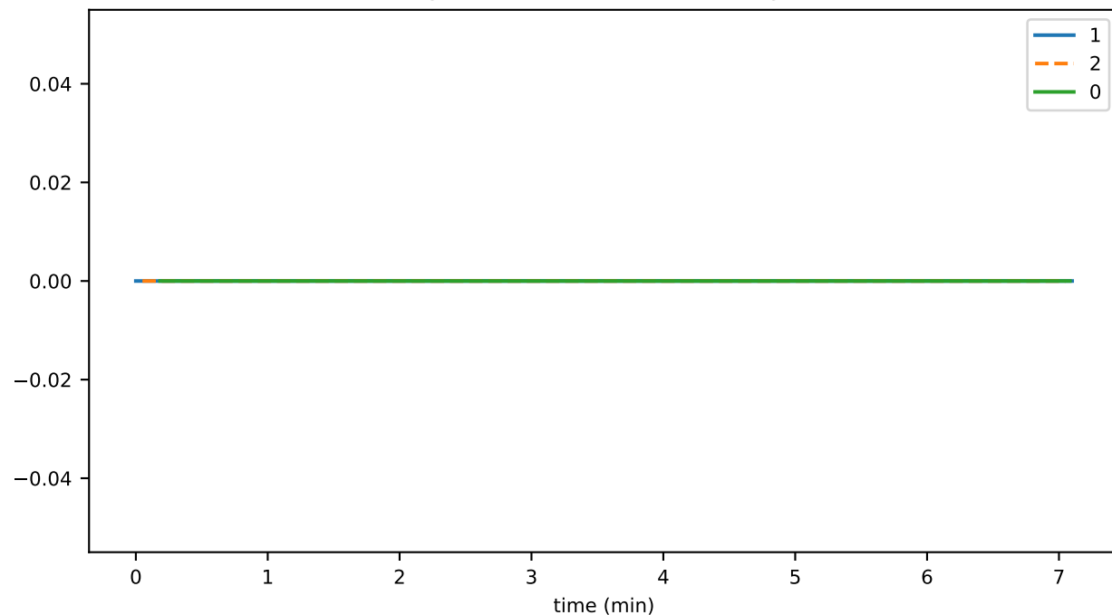
getAccountDetailsThrottledTxns
