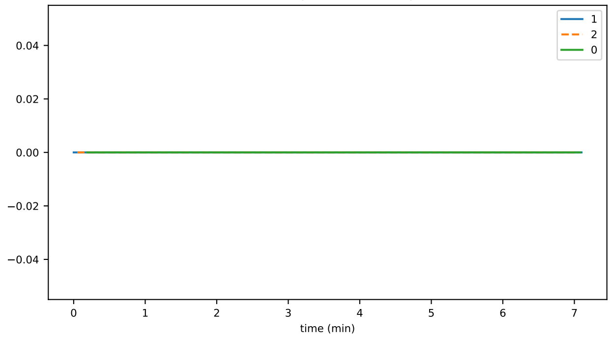
contractUpdateThrottledTxns
