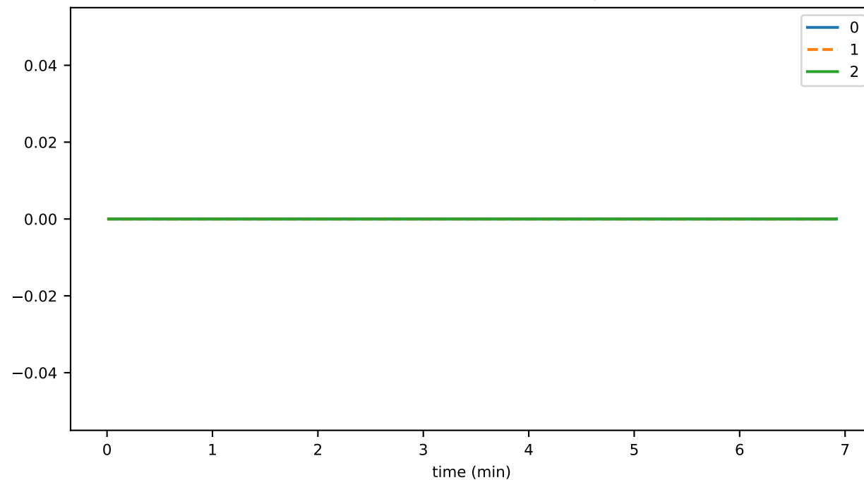
scheduleGetInfoThrottledTxns
