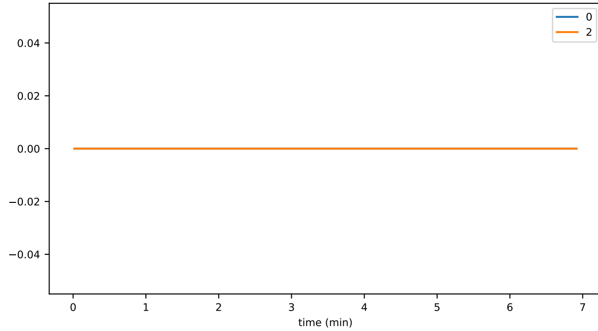
1e11 DiskspaceFree
