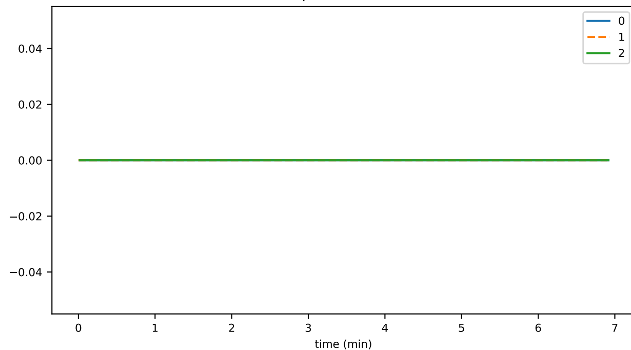
topicsPercentUsed
