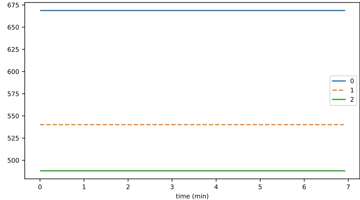
eventDelay_1_hashing_storage
