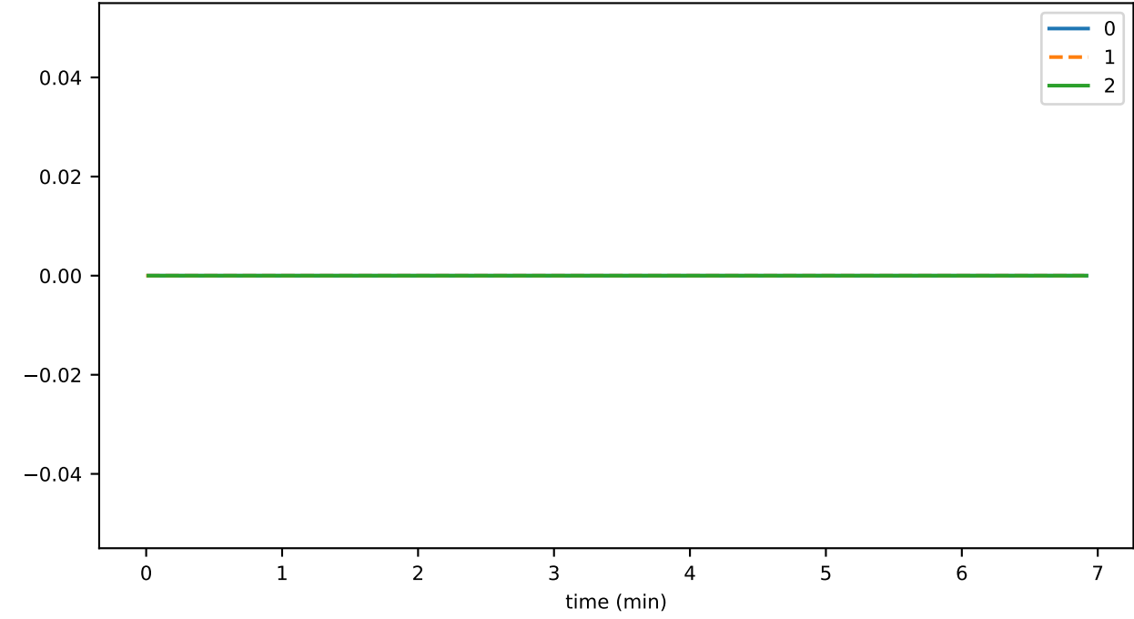
contractAutoRenewThrottledTxns
