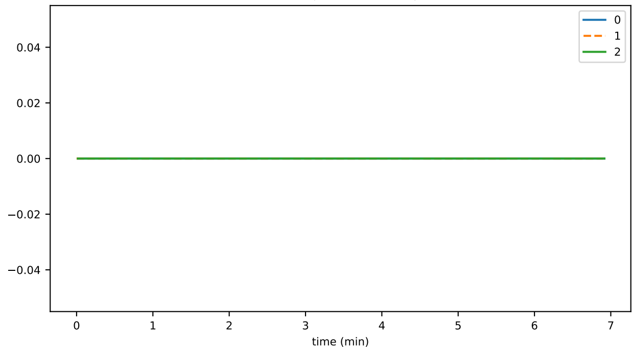
tokenRejectThrottledTxns
