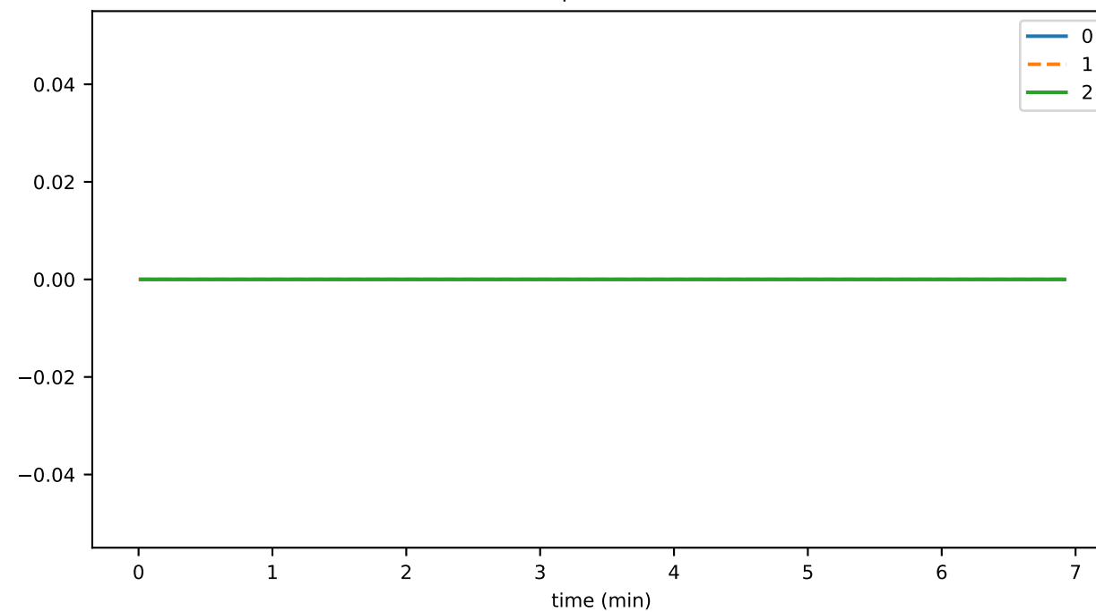
topicsUsed
