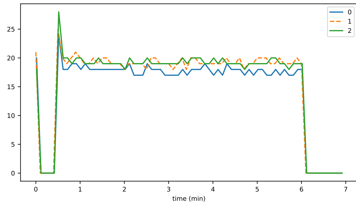
numReportFallenBehind
