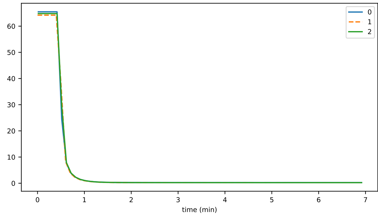
secC2RC
