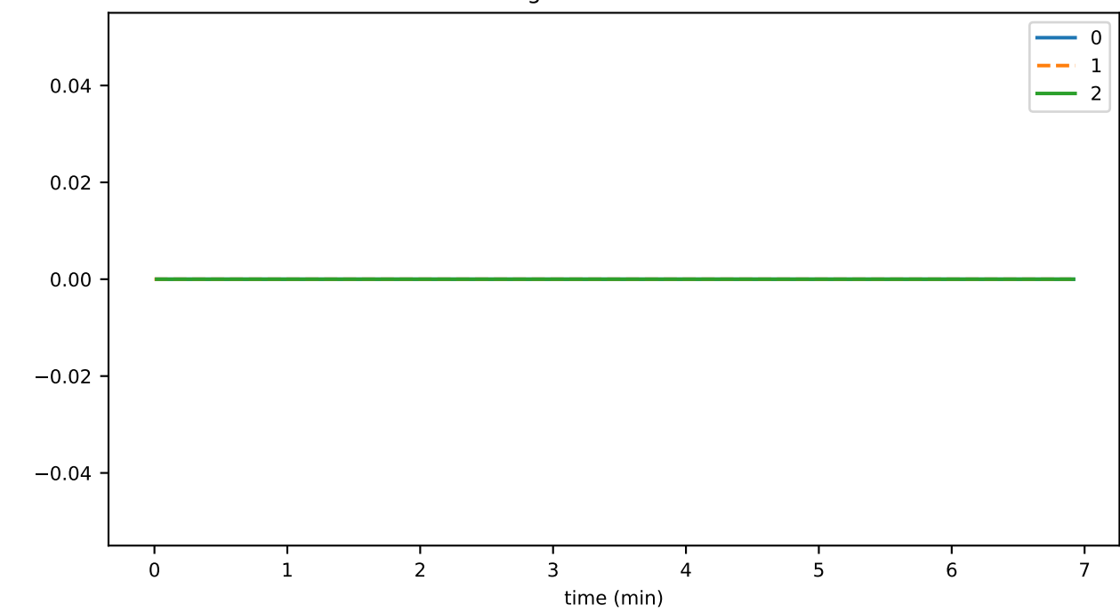
gasPerConsSec
