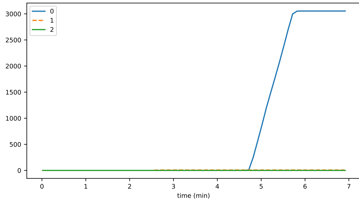
DeprTxnsRcv
