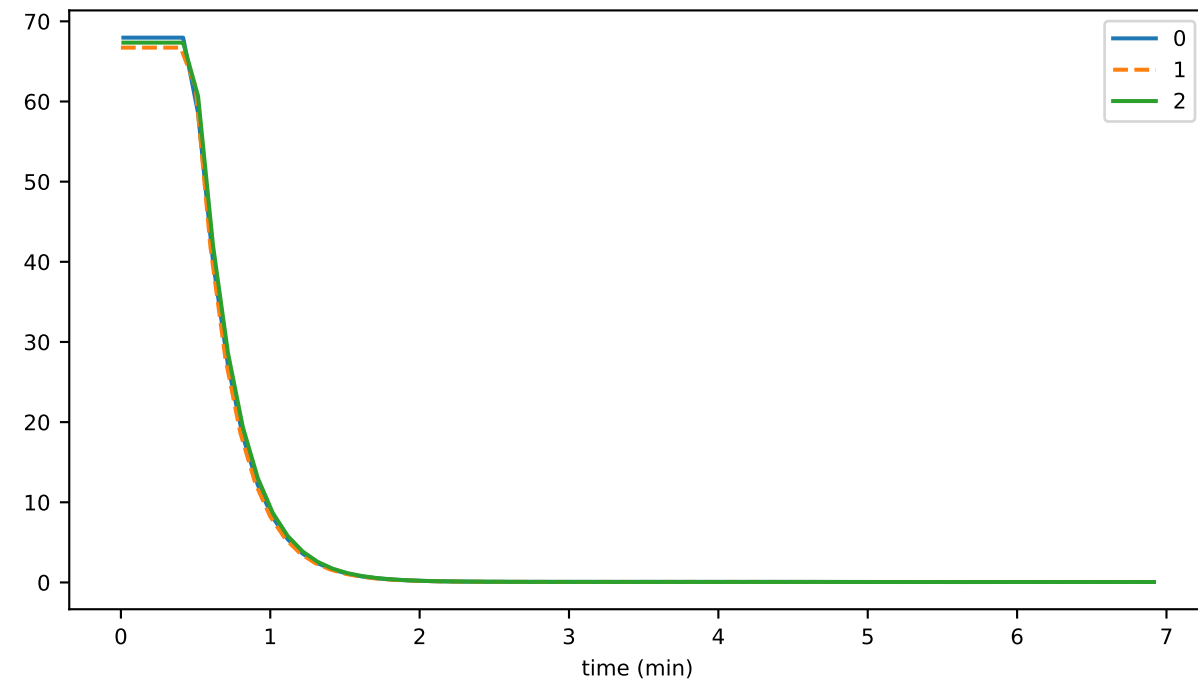
secC2R
