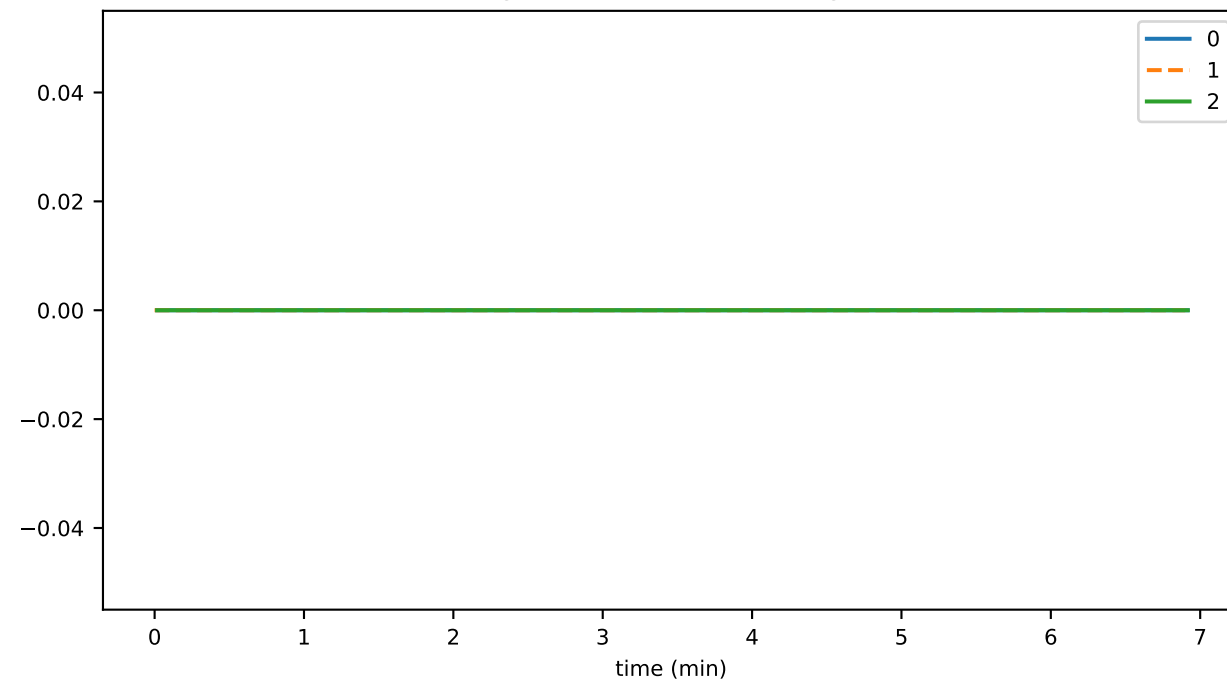
getVersionInfoThrottledTxns
