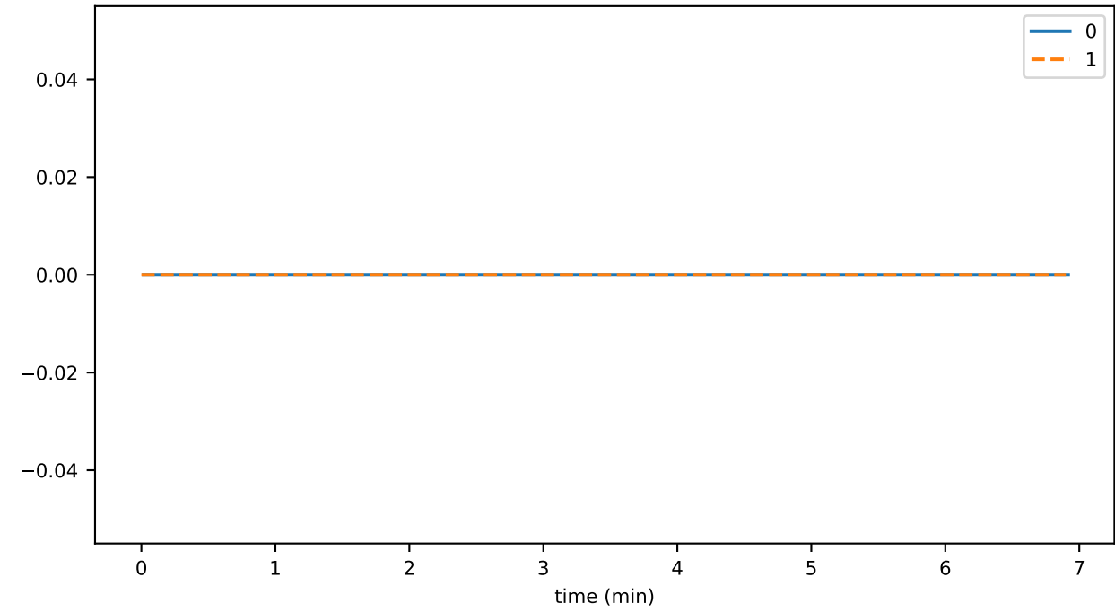
1e10 DiskspaceUsed
