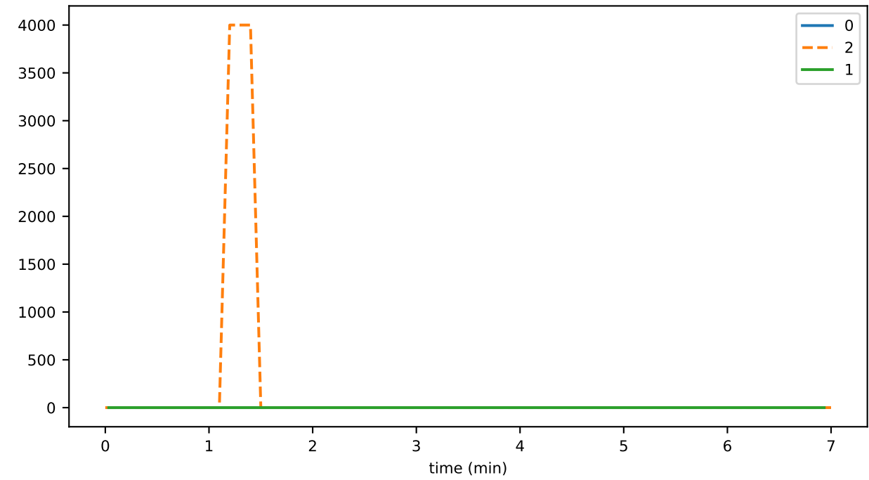
TransactionHandler_unhandled_task_count
