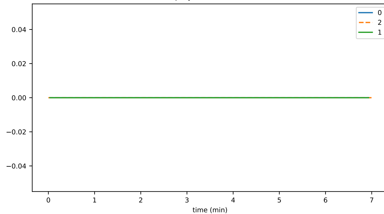
hapiBytesPercentUsed
