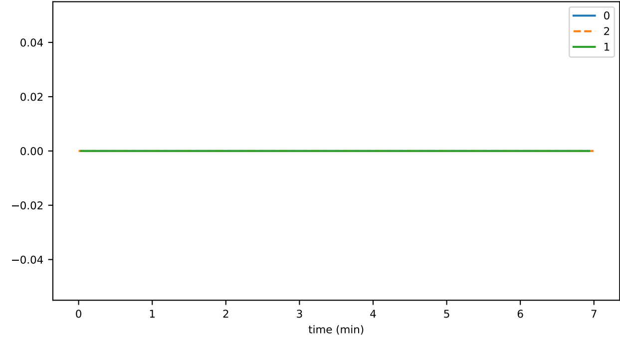
tokenMintThrottledTxns
