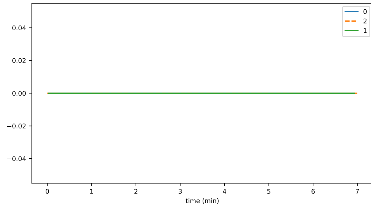
issCount
