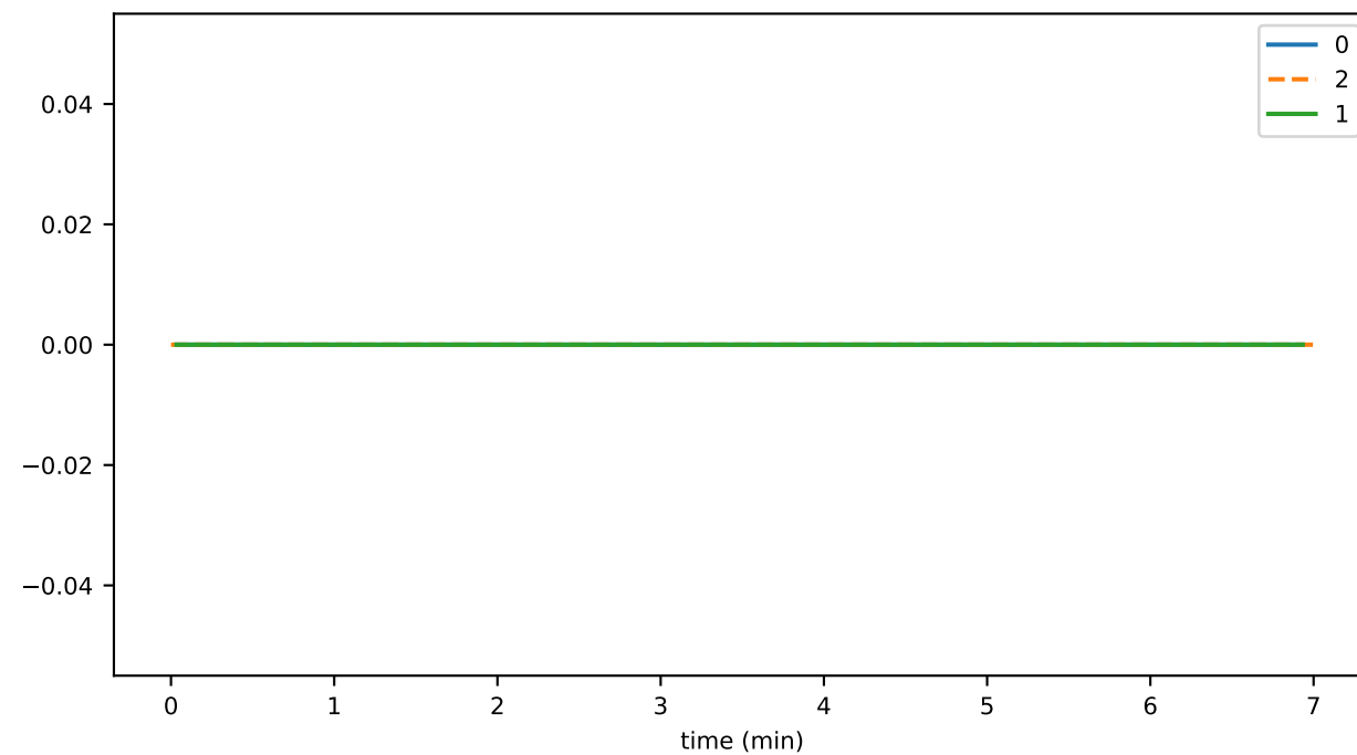
tokenGetNftInfosDurationMax
