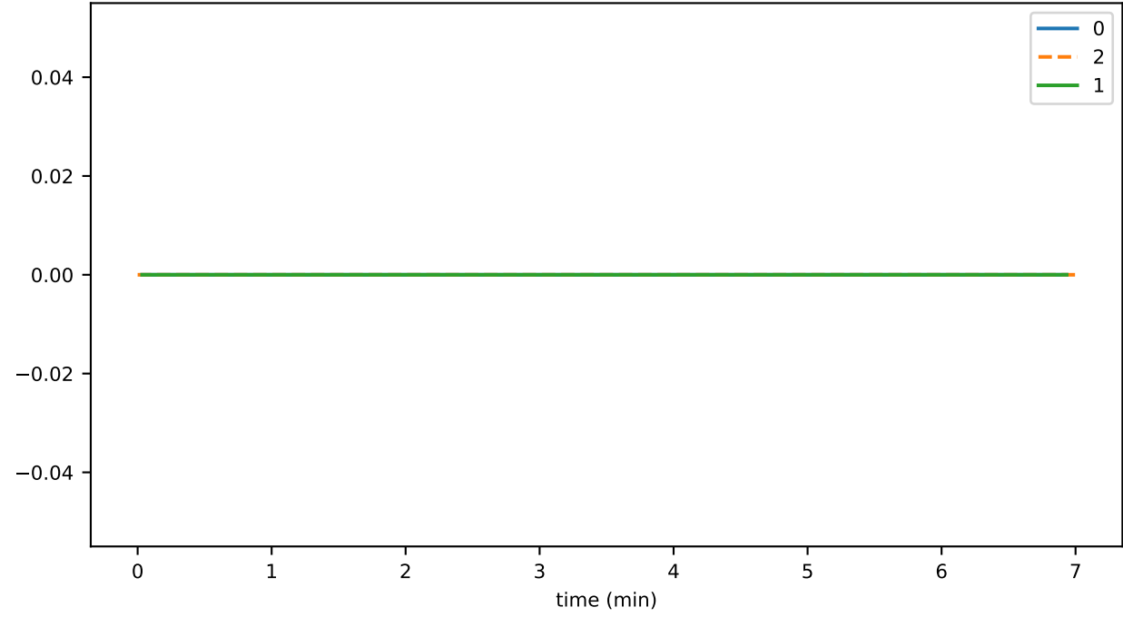
ParseErrBufUnderflowRcv
