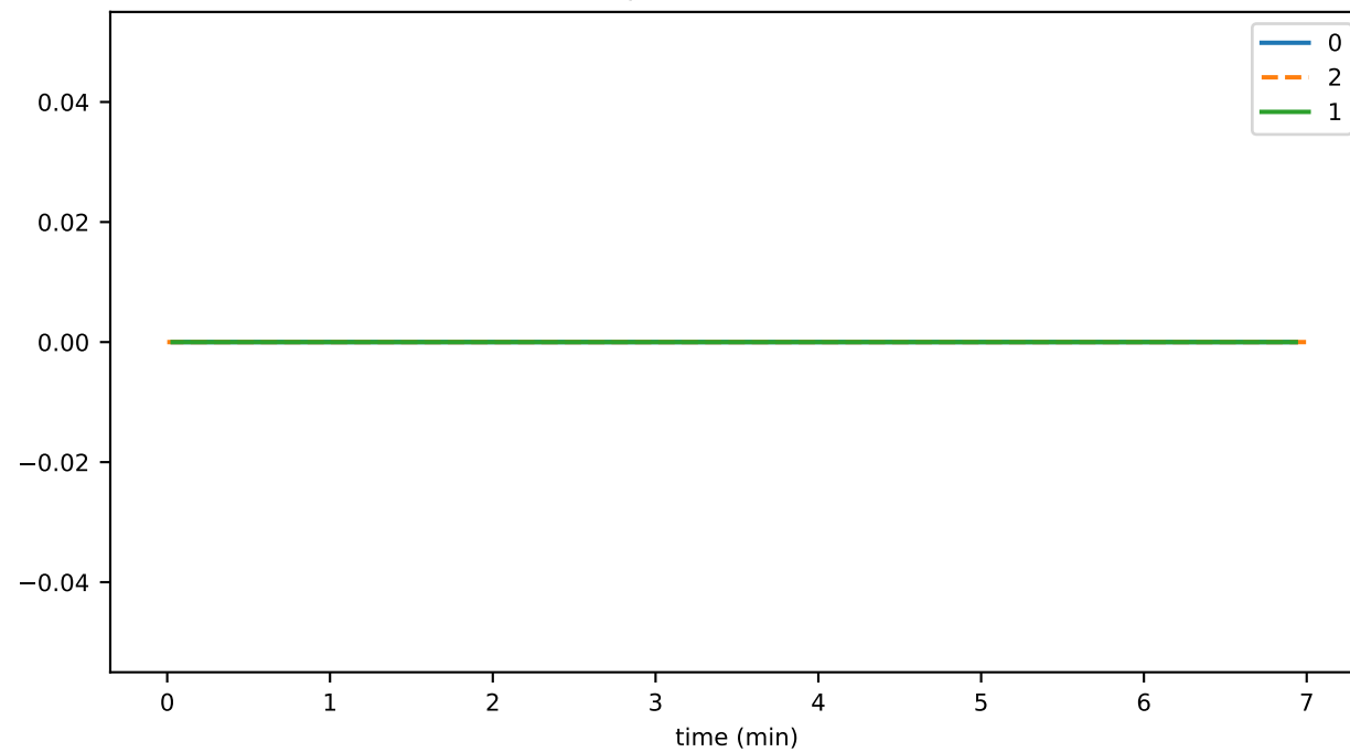
tokenUpdateThrottledTxns
