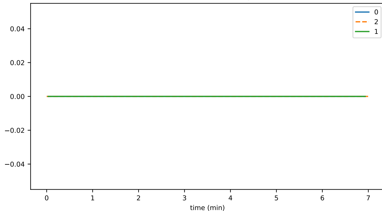
fileDeleteThrottledTxns
