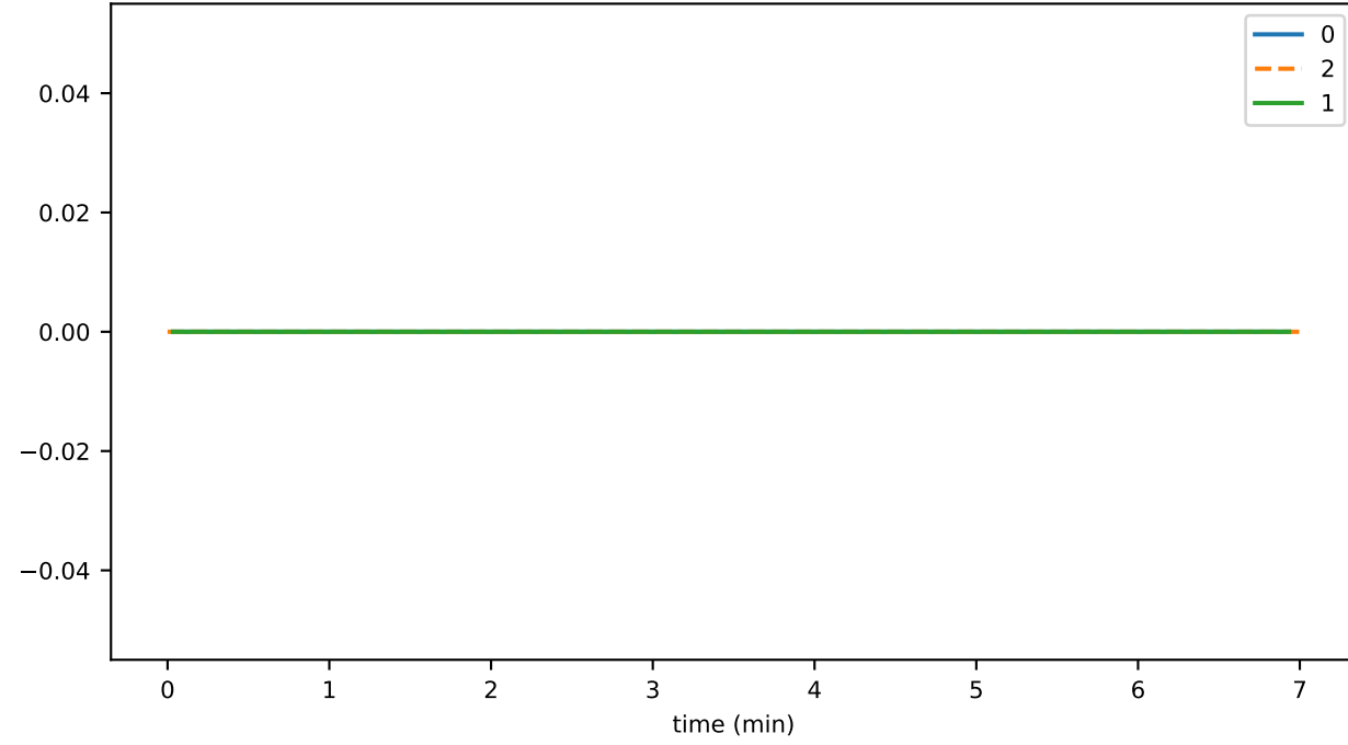
tokenPauseThrottledTxns
