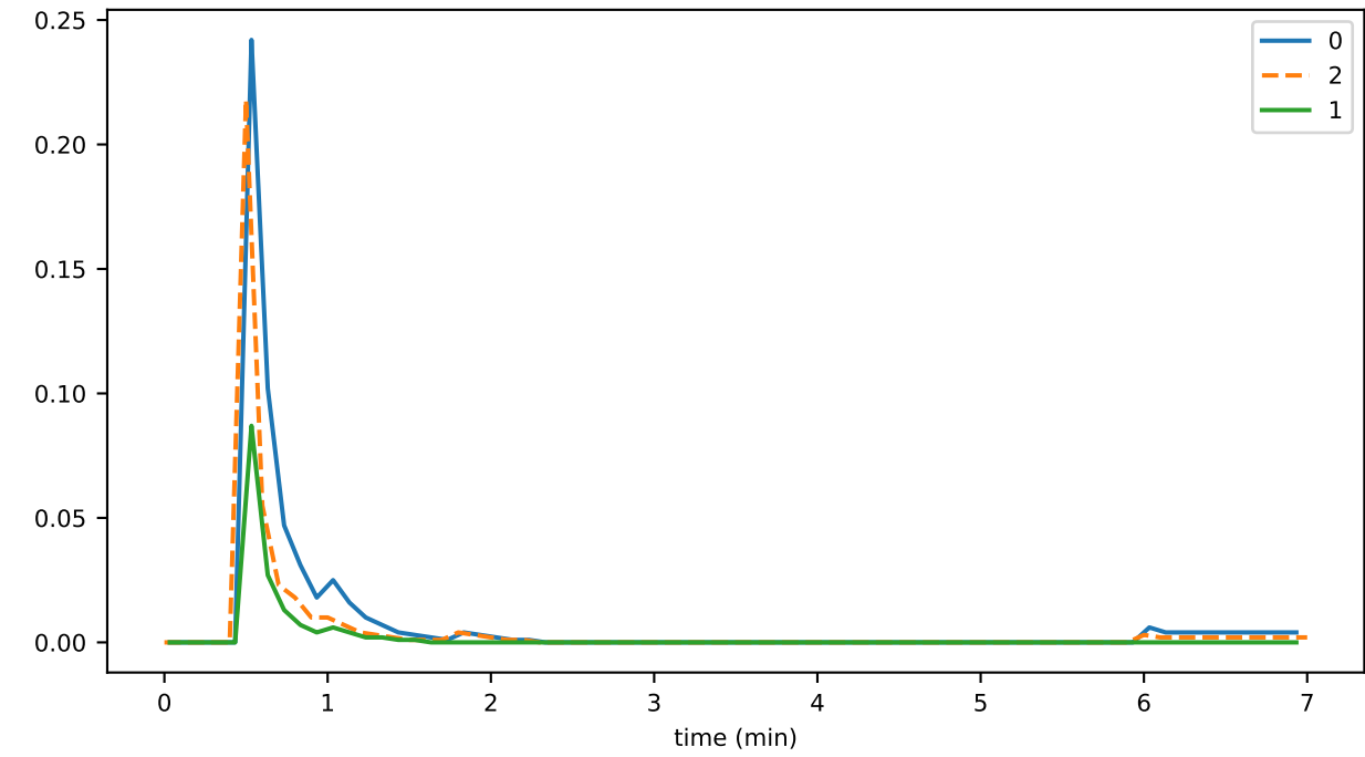
Sig_per_sec
