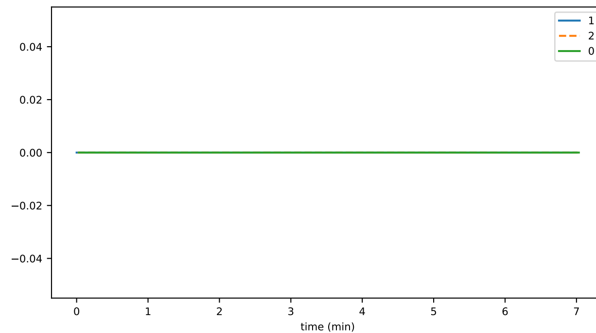
ParseErrOtherRcv
