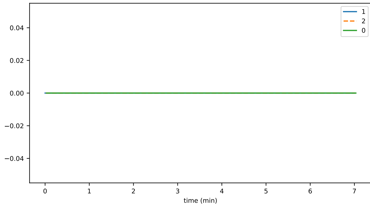
fileGetInfoDurationMax
