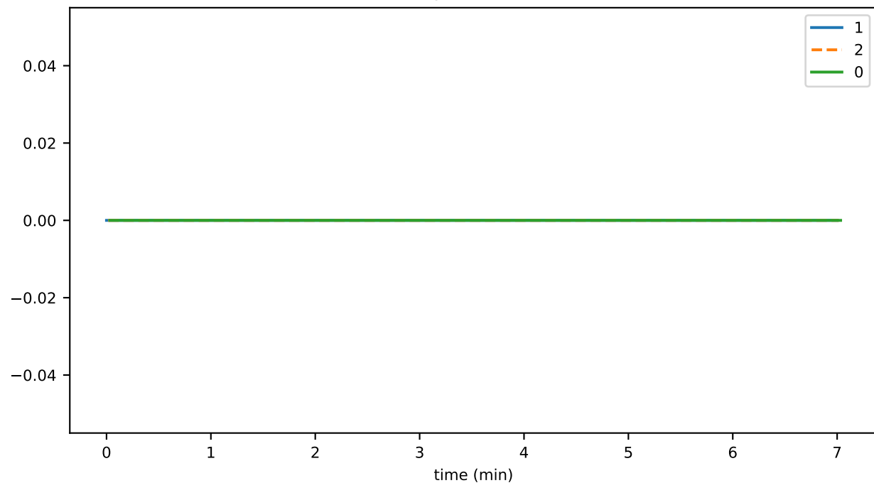
contractGetInfoDurationMax
