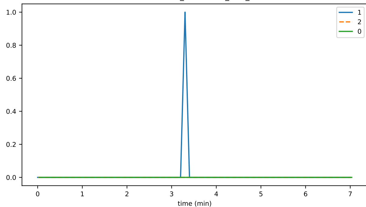
PlatSigEnqueueTime
