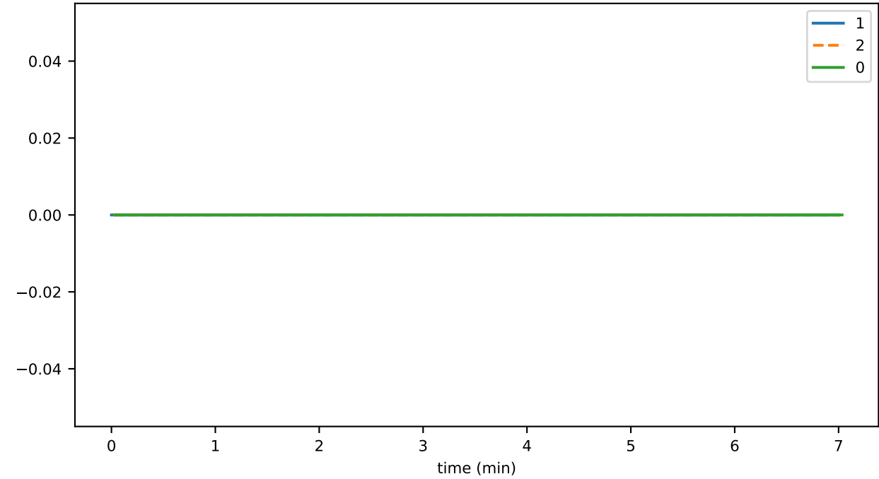
StateGarbageCollector_unhandled_task_count
