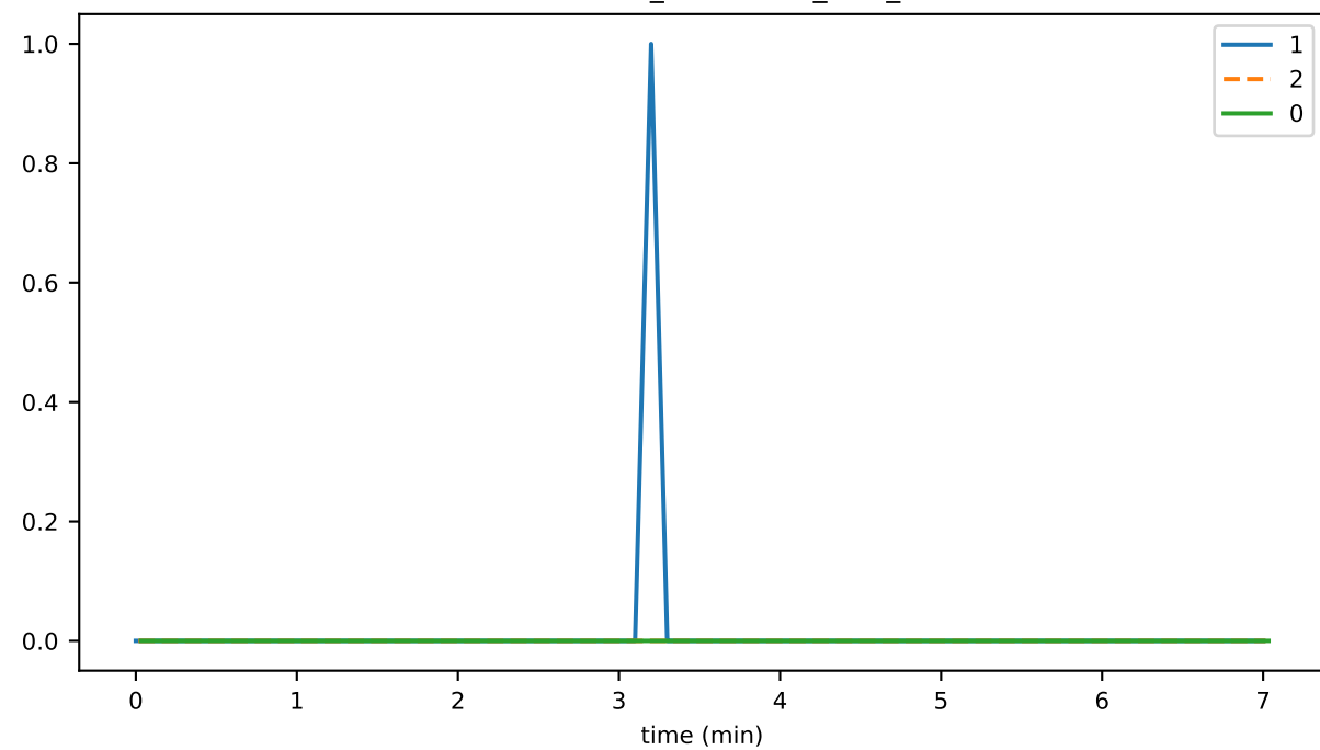
issCount
