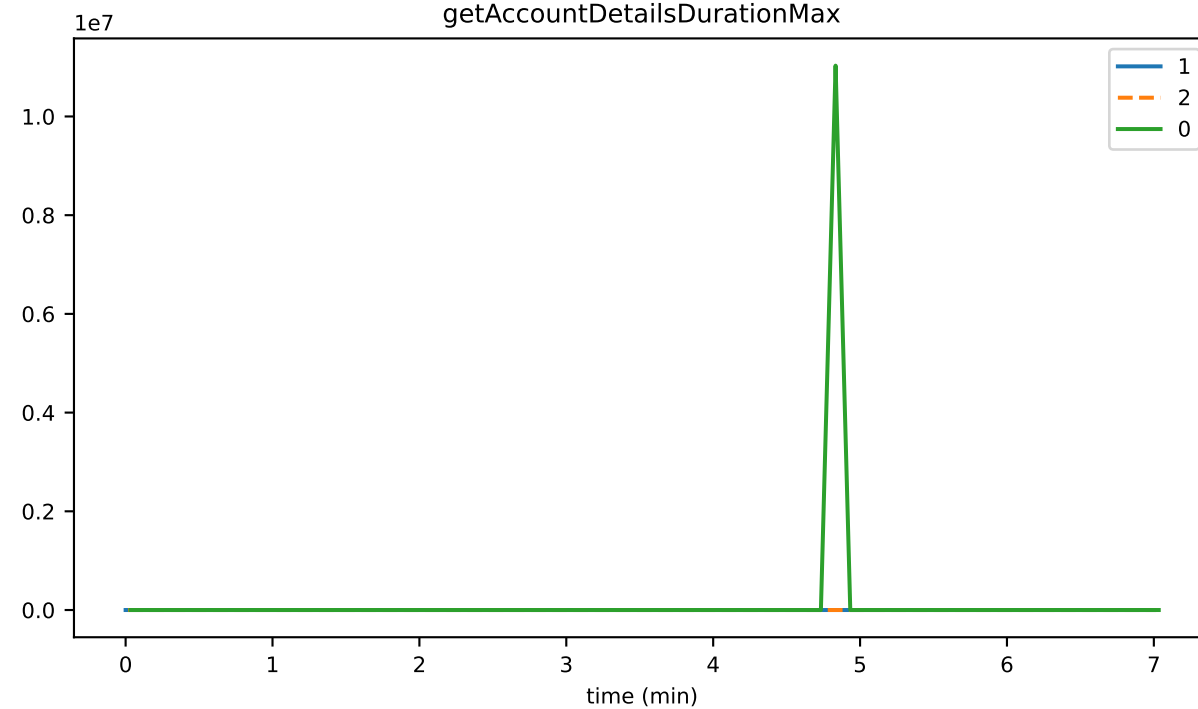
getAccountDetailsDurationMax
