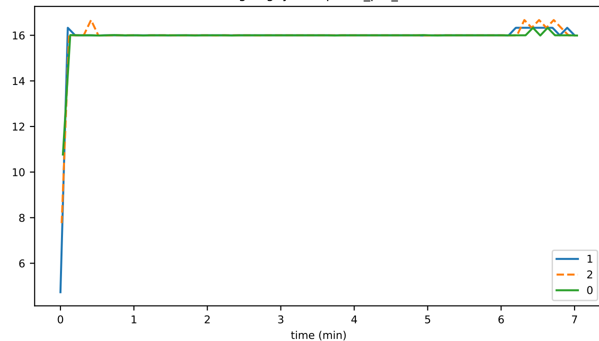
ParseErrBufUnderflowRcv
