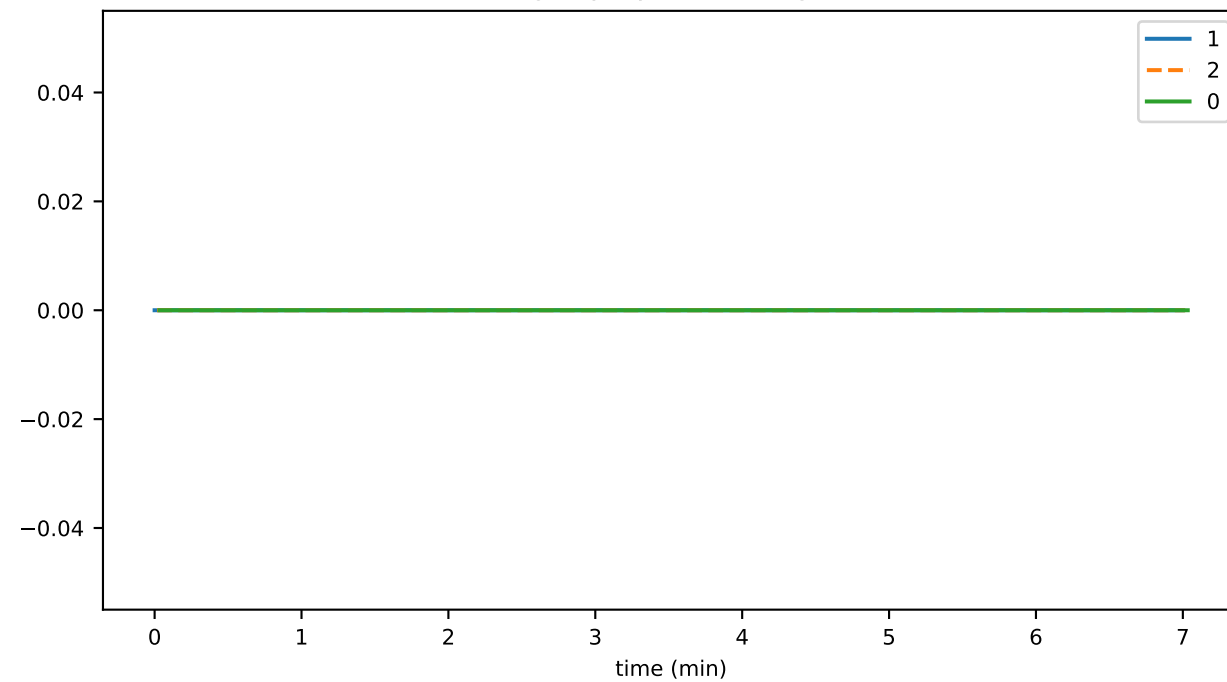
getByKeyThrottledTxns
