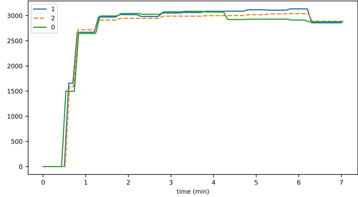
stateToDisk
