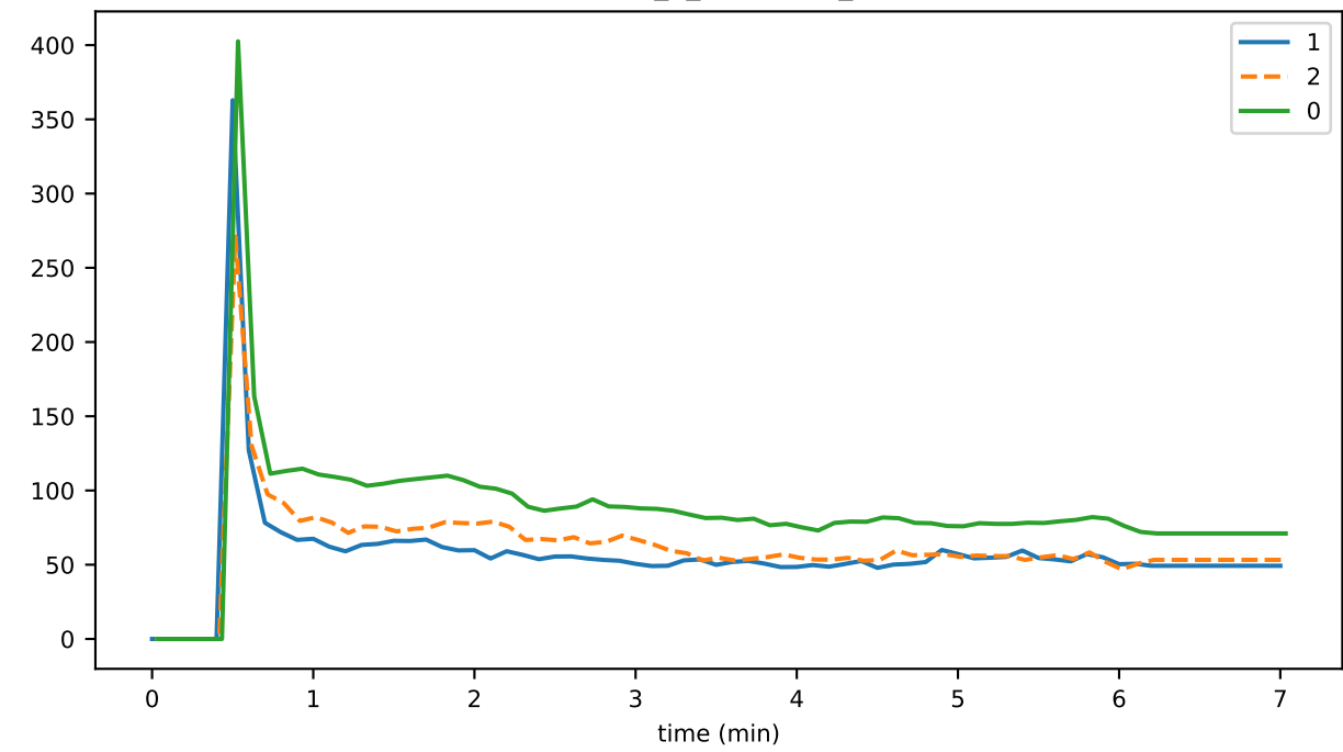
eventDelay_2_validation_gossip
