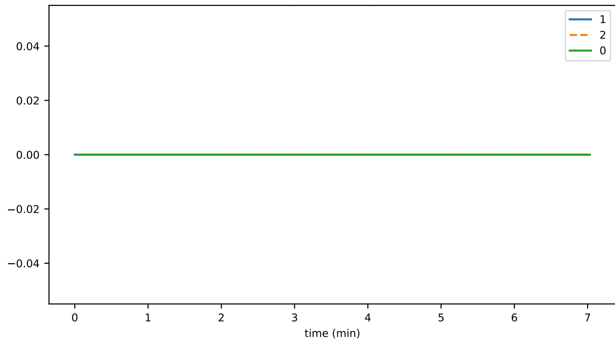
syncs_per_sec
