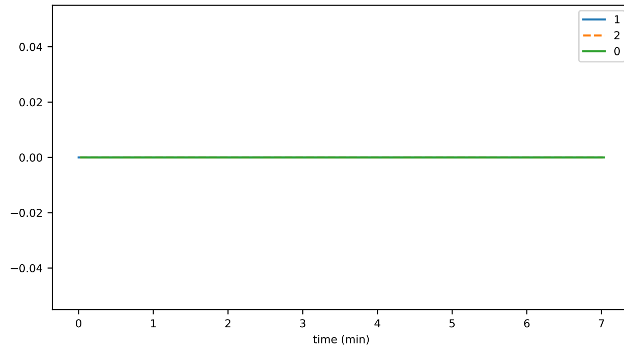
contractGetInfoThrottledTxns
