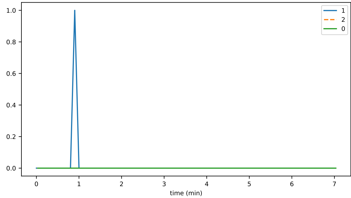
StateGarbageCollector_unhandled_task_count
