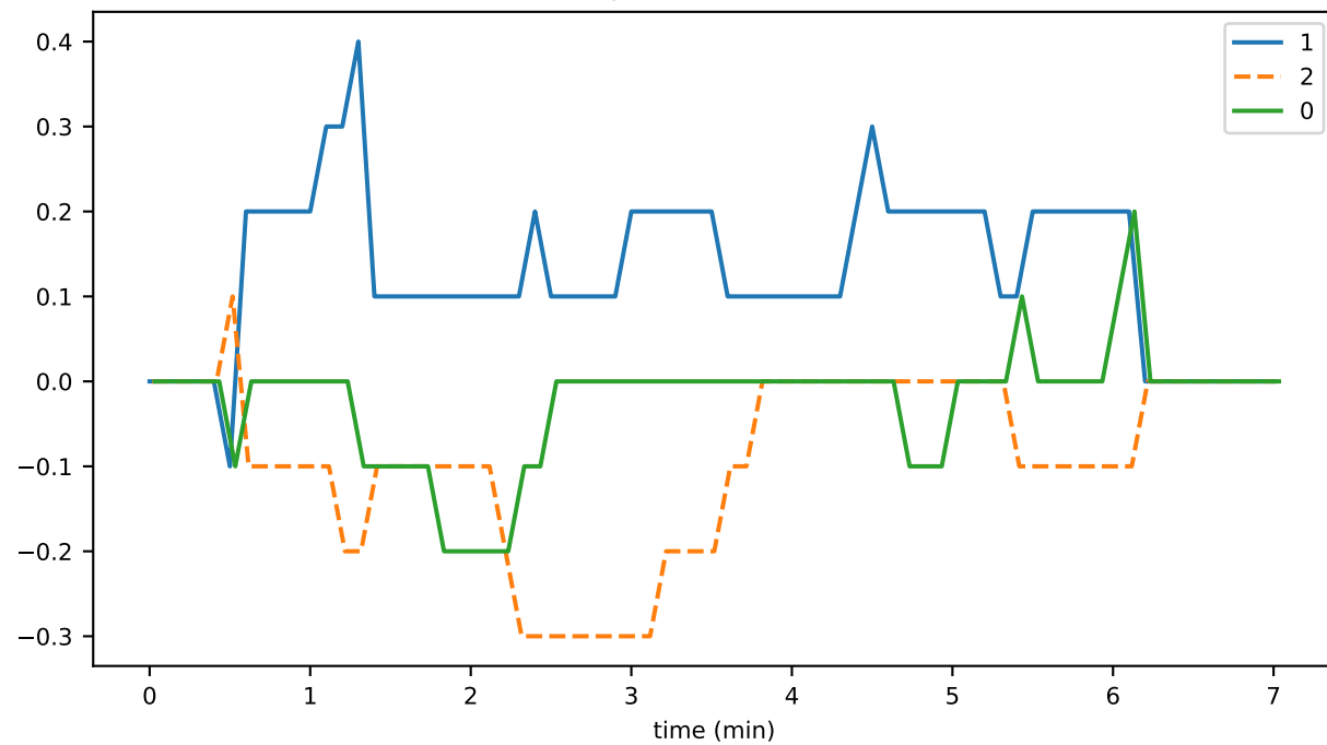
syncPermitsRevoked
