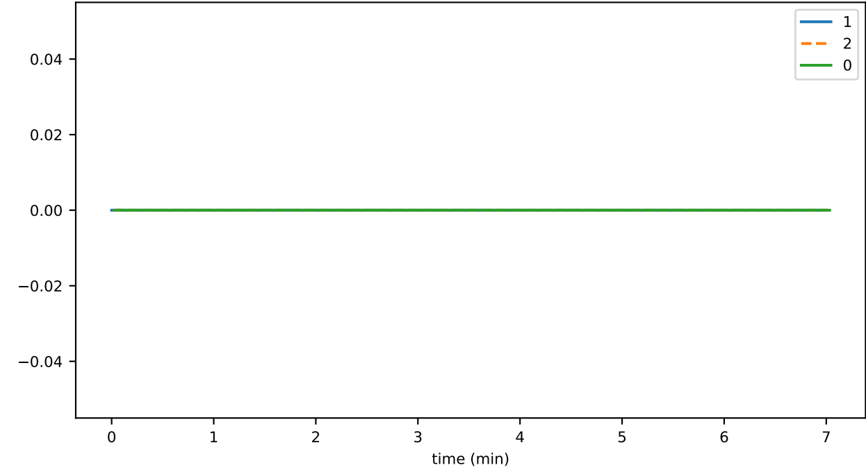
conn_connClose_unknown
