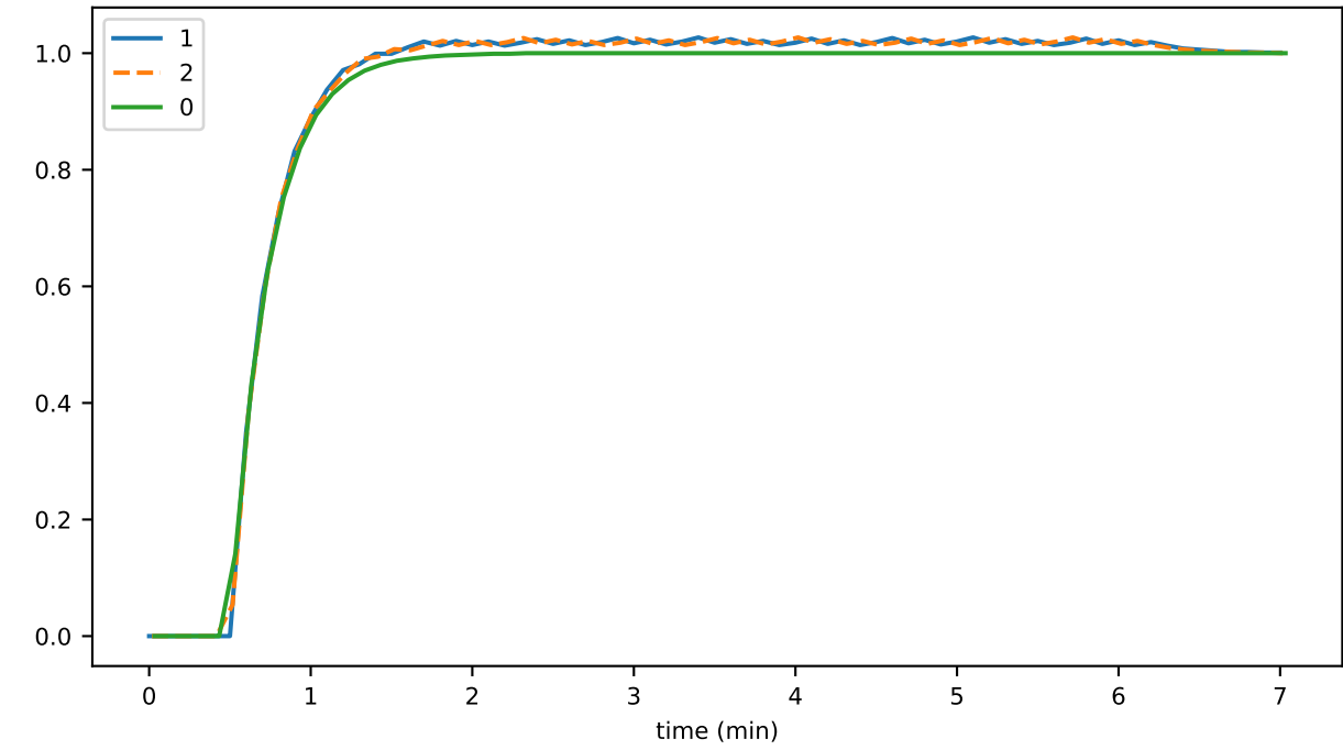
stateToDisk
