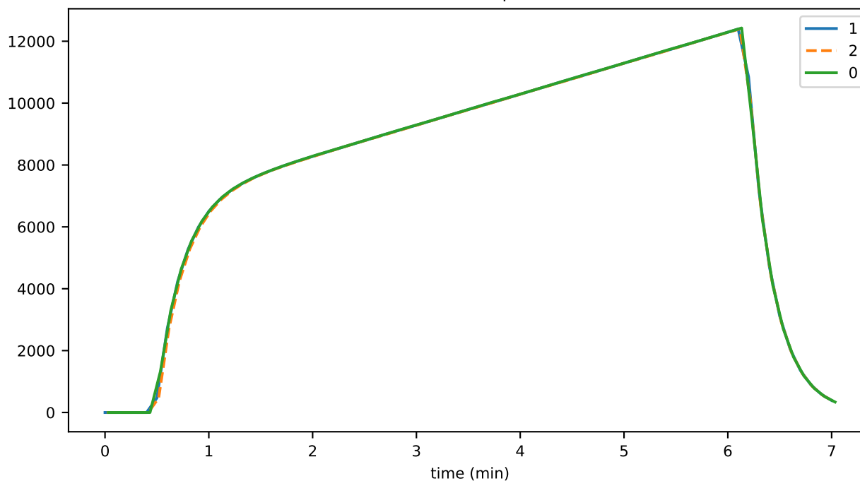
roundSup
