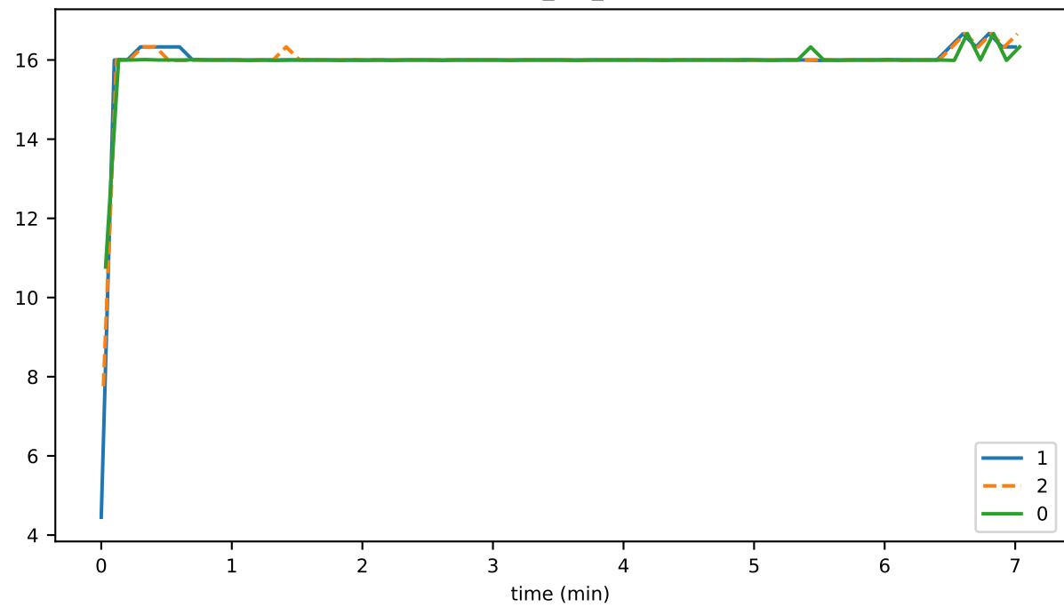
syncs_per_sec
