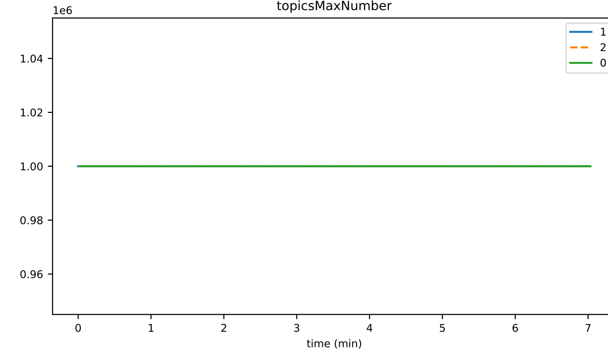
topicsMaxNumber
