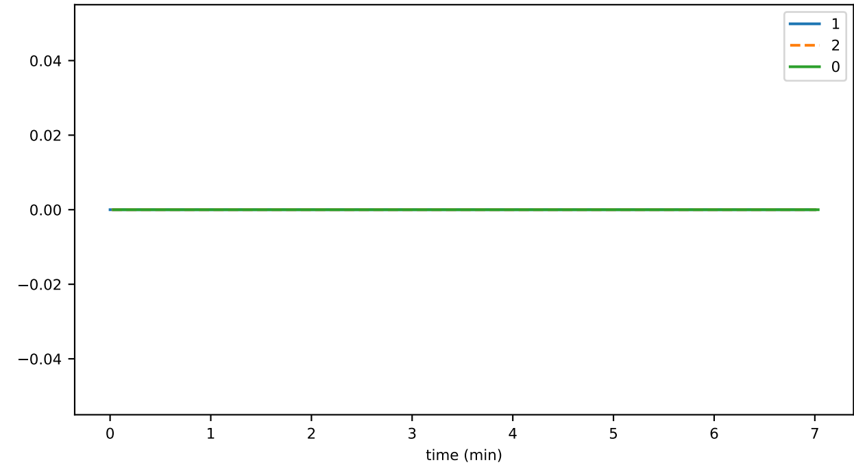
conn_connClose_unknown
