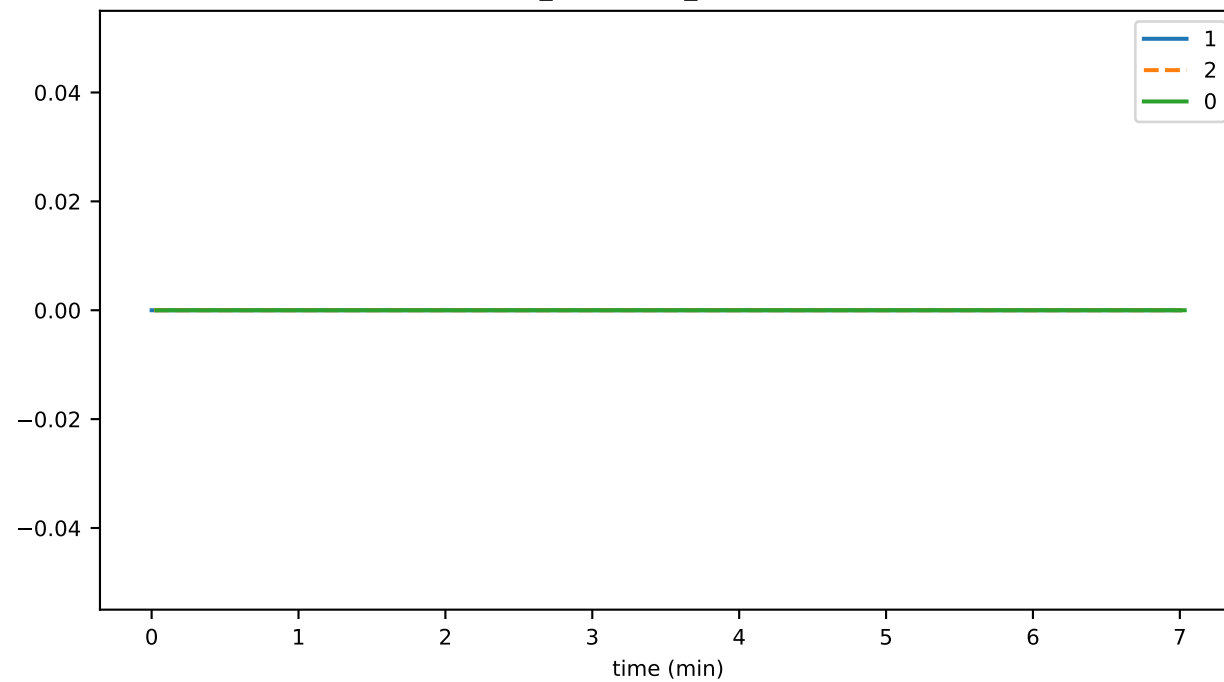
conn_connClose_periodicReset
