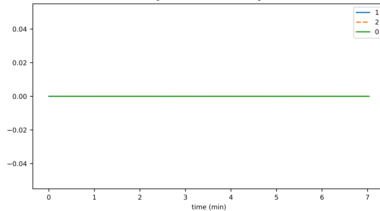
getVersionInfoDurationAvg
