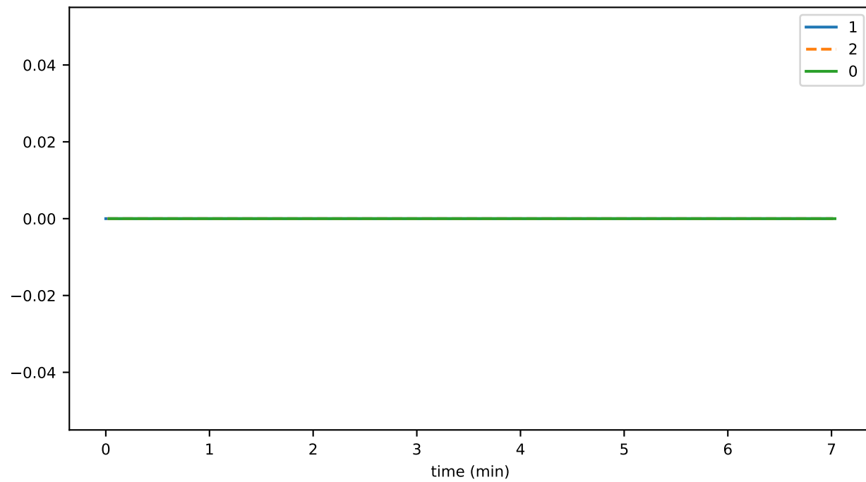
syncPermitsRevoked
