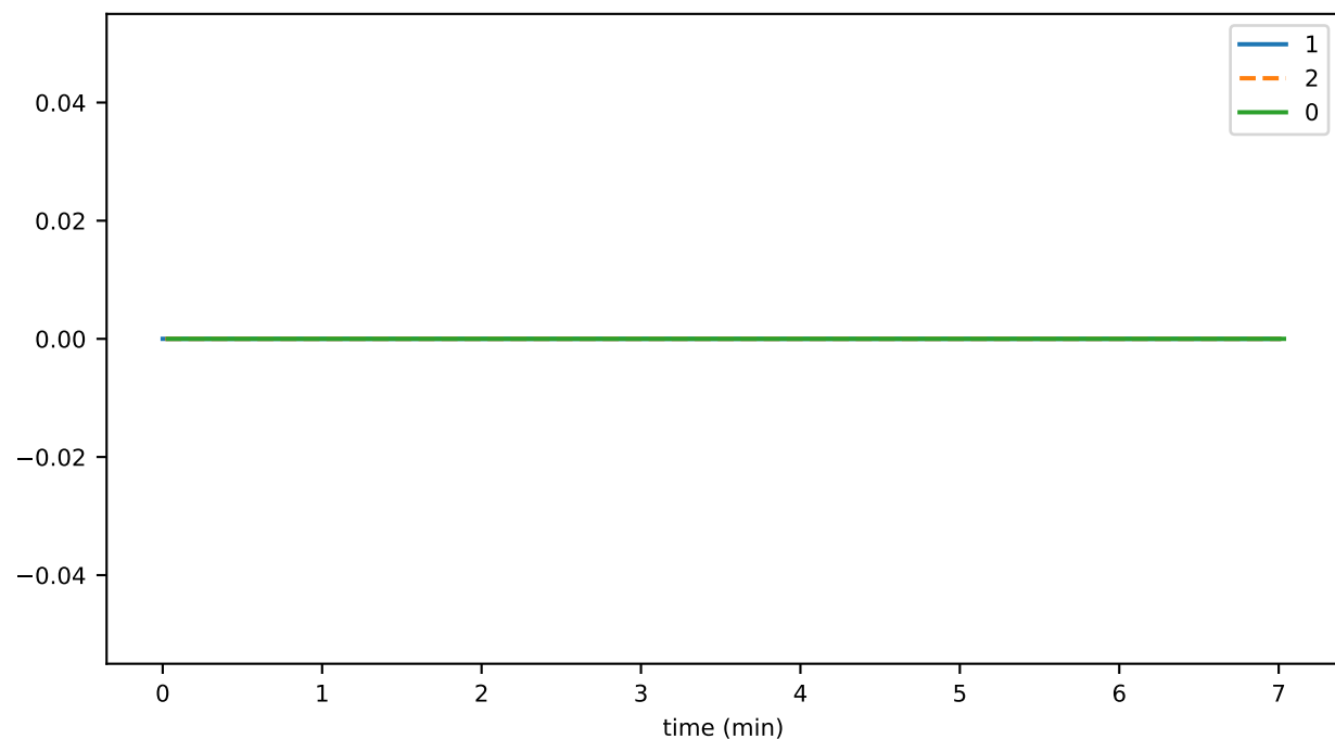
indicatorsWaitingForExpiry
