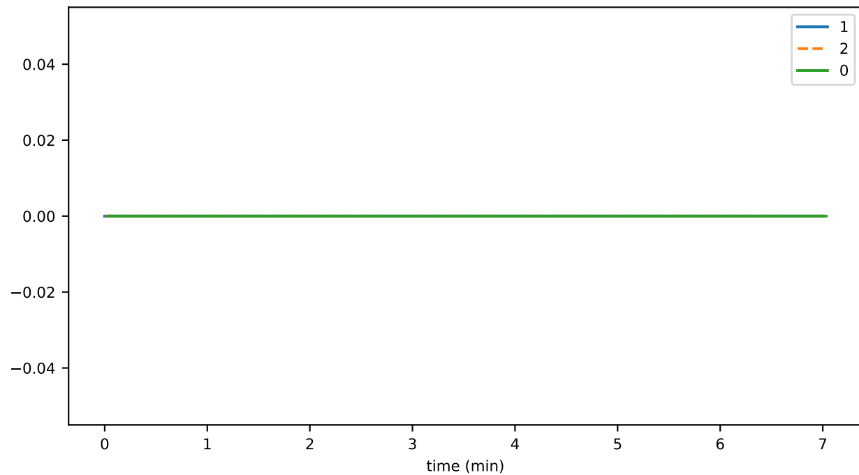
SigSubWrkltmTime
