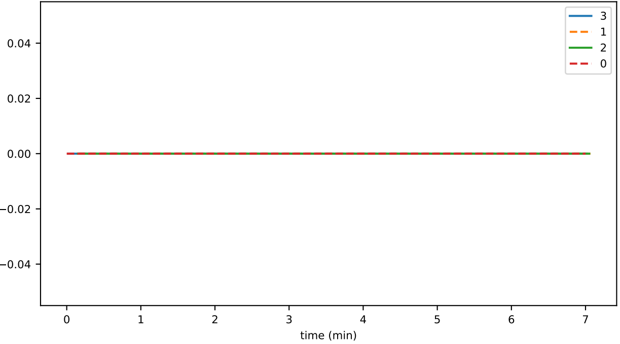
SmartContractService:SystemContractMethodCall_PROXY_total
