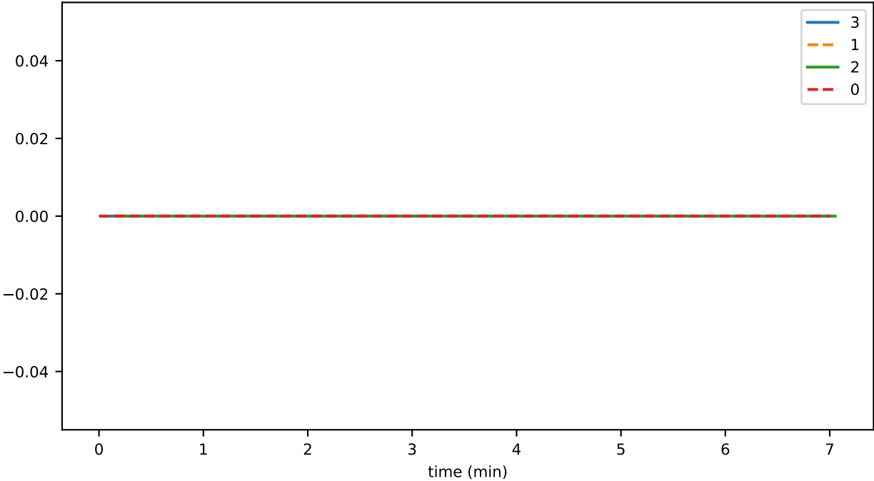
SmartContractService:SystemContractMethodCall_ALIASES_total
