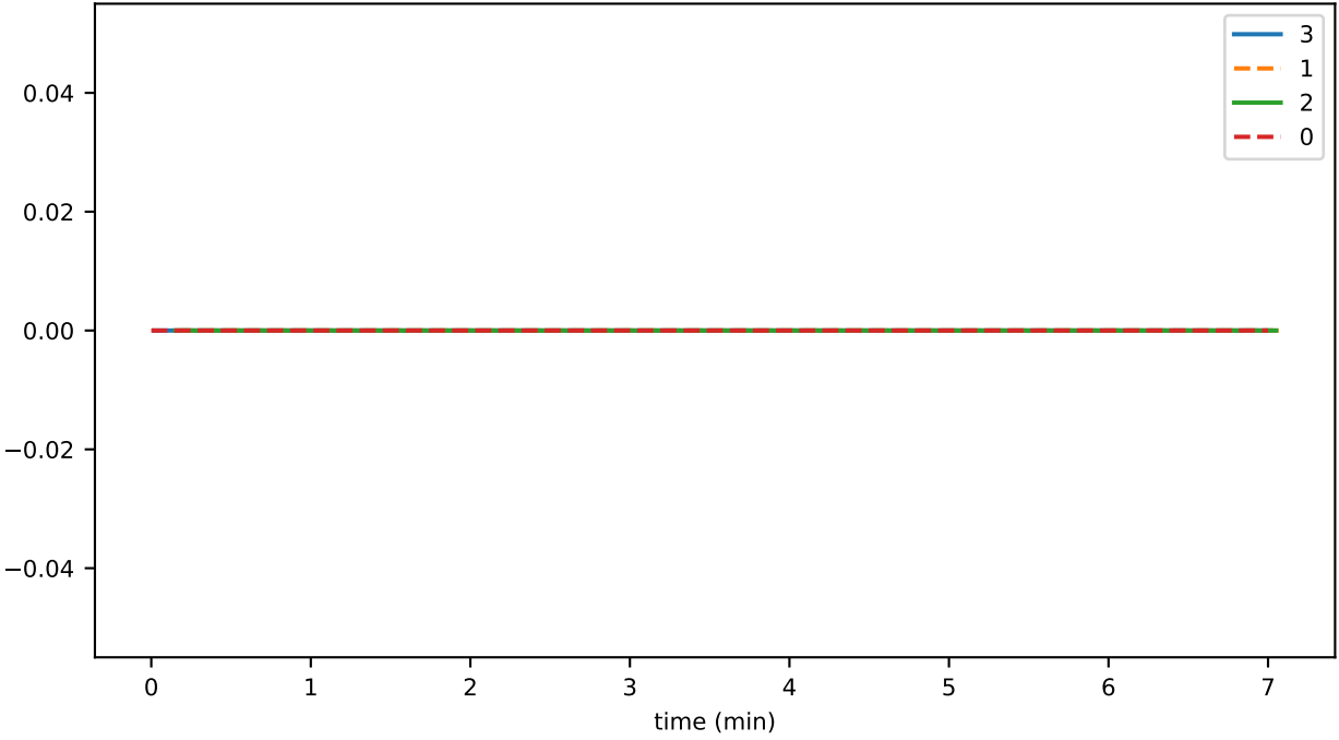
SmartContractService:SystemContractMethodCall_WIPE_total
