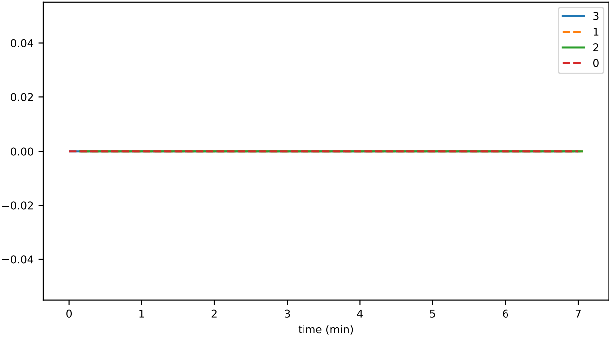
SmartContractService:SystemContractMethodCall_ERC20_total
