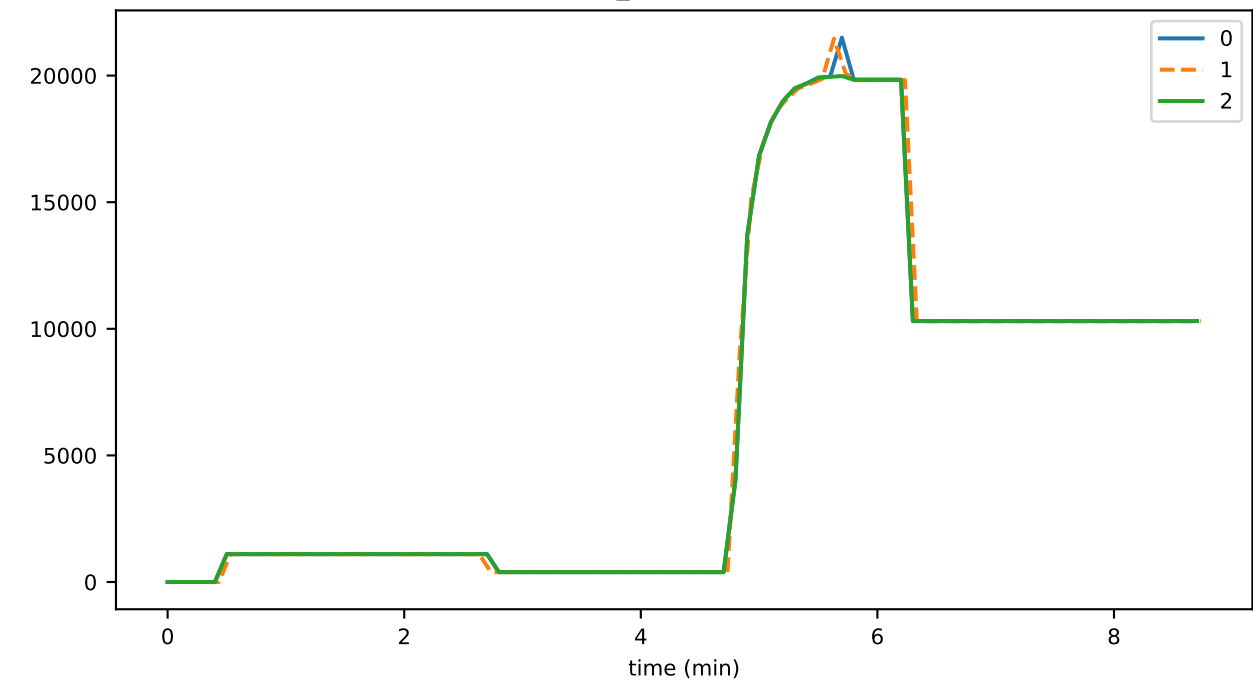
buffer_blockItemBytes
