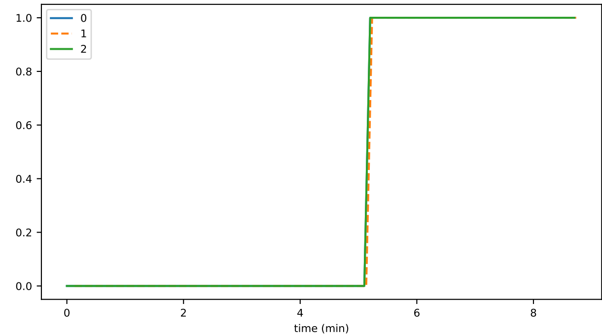
buffer_blockItemBytes
