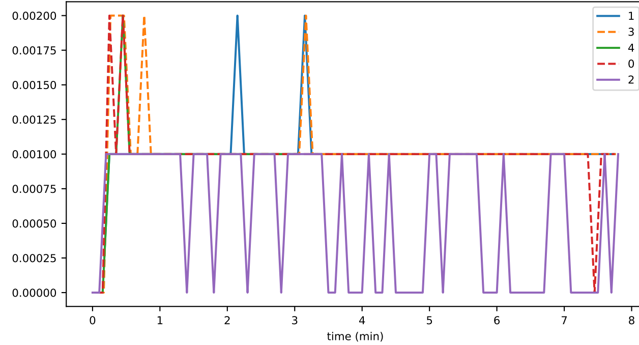
StateHasher_busy_fraction
