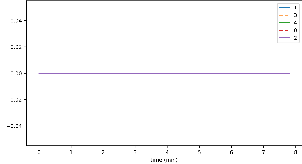
StateHasher_unhandled_task_count
