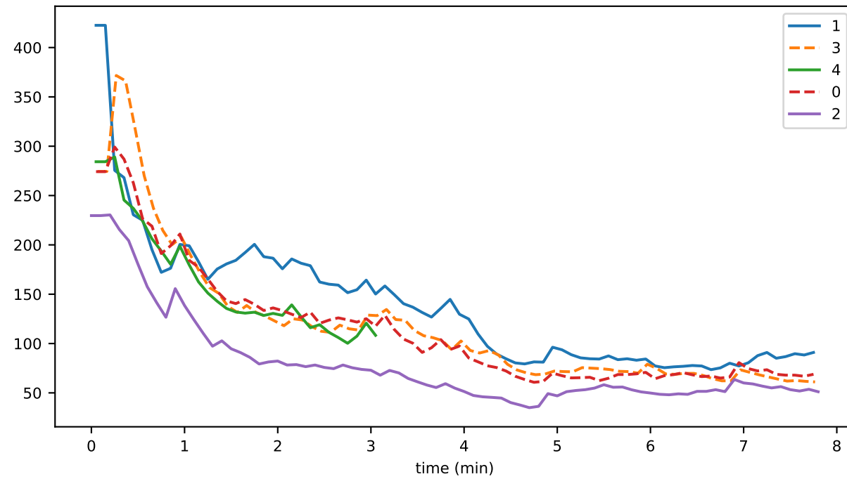
StateHasher_busy_fraction
