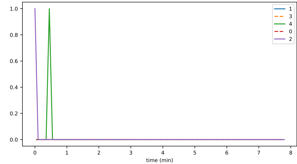
StateHasher_unhandled_task_count
