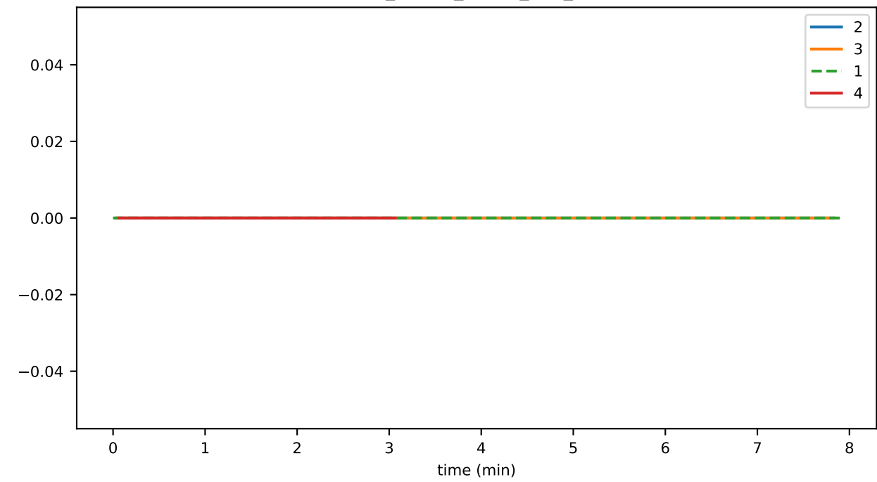
rpc_output_queue_size_00
