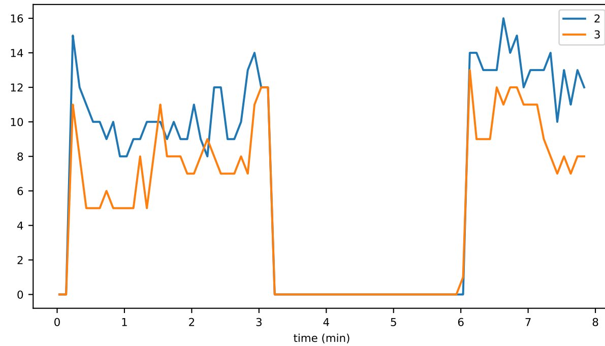
rpc_output_queue_poll_timeMAX
