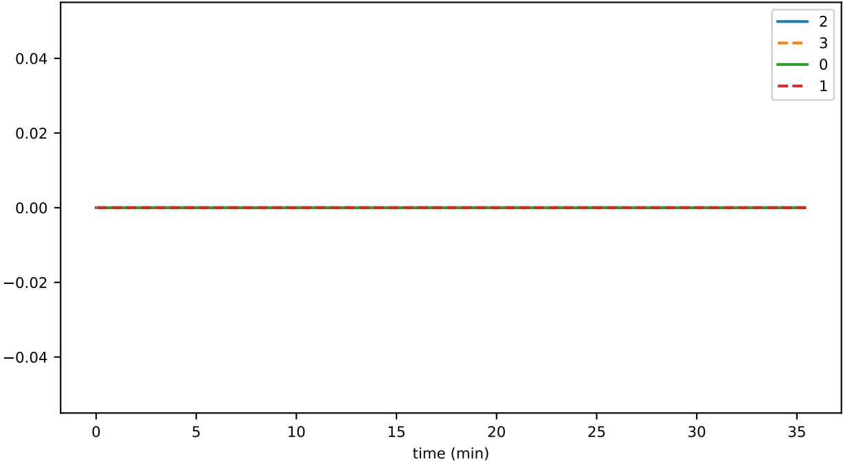
SmartContractService:SystemContractMethodCall_SCHEDULE_total
