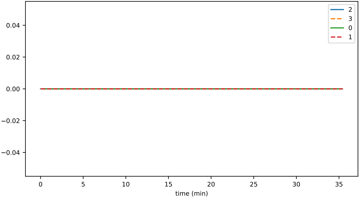
SmartContractService:SystemContractMethodCall_TOKEN_QUERY_failed
