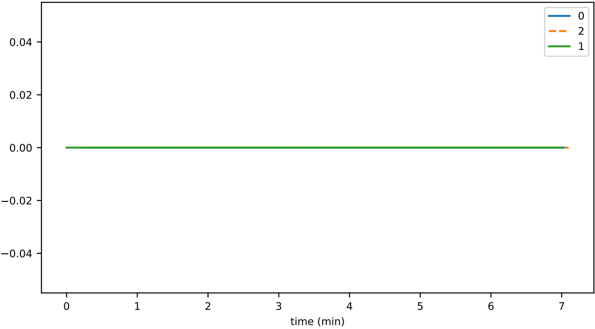
SmartContractService:SystemContractMethodCall_APPROVAL_total
