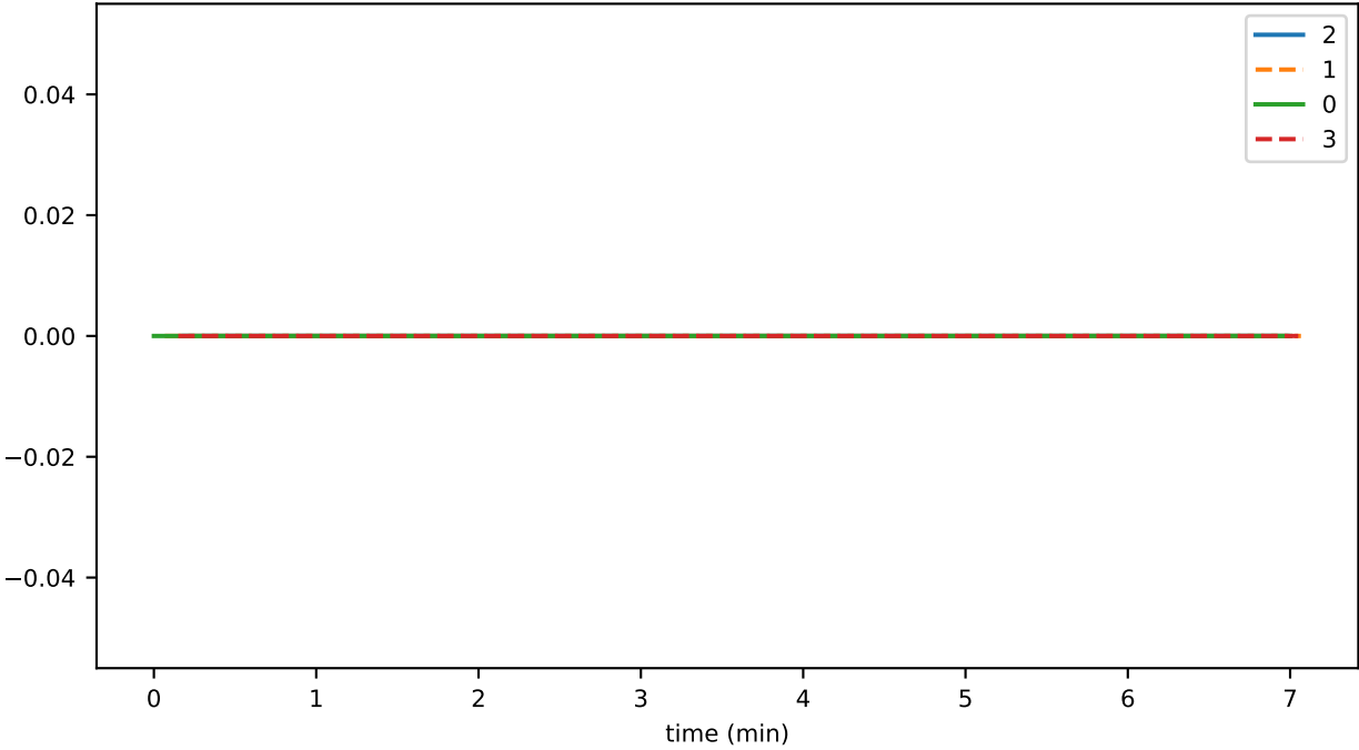
SmartContractService:SystemContractMethodCall_MINT_BURN_total
