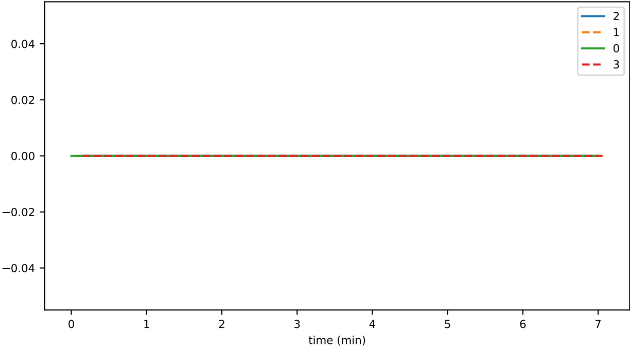
SmartContractService:SystemContractMethodCall_WIPE_total
