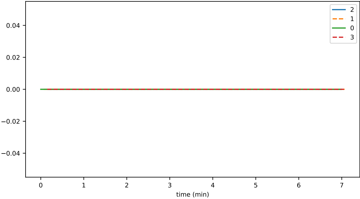
SmartContractService:SystemContractMethodCall_IS_AUTHORIZED_total
