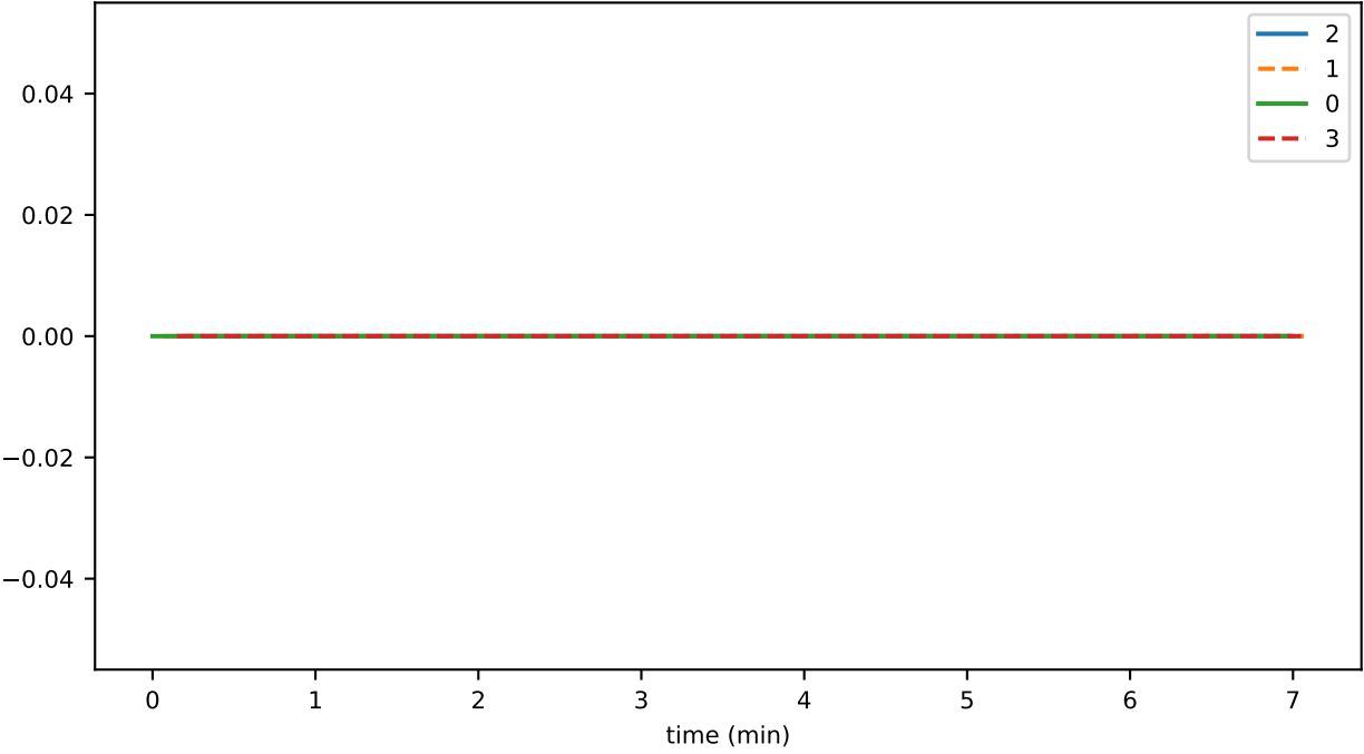
SmartContractService:SystemContractMethodCall_IS_AUTHORIZED_failed
