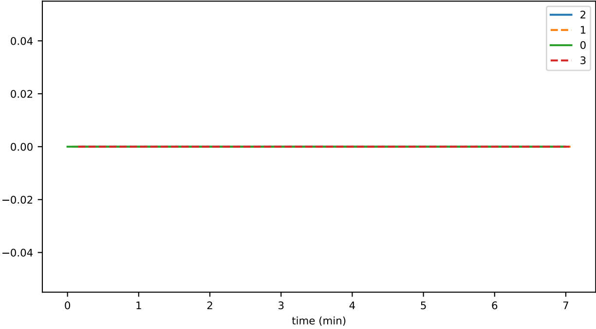
SmartContractService:SystemContractMethodCall_IS_AUTHORIZED_total
