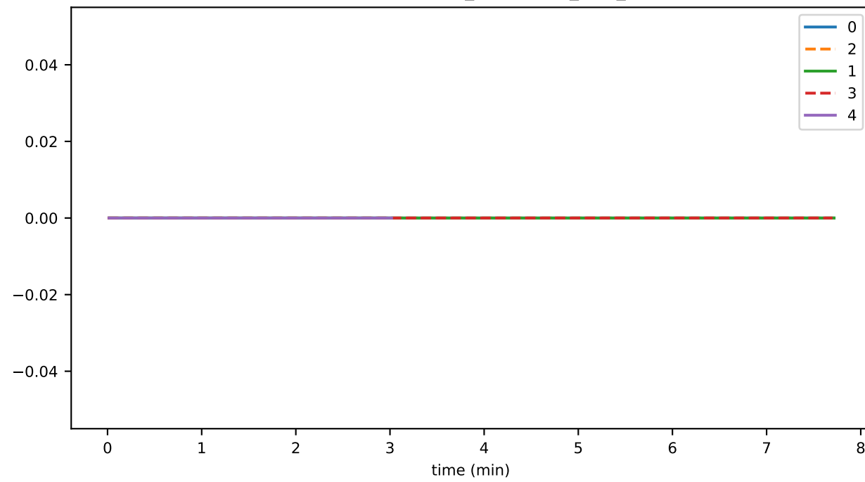
InternalEventValidator_unhandled_task_count
