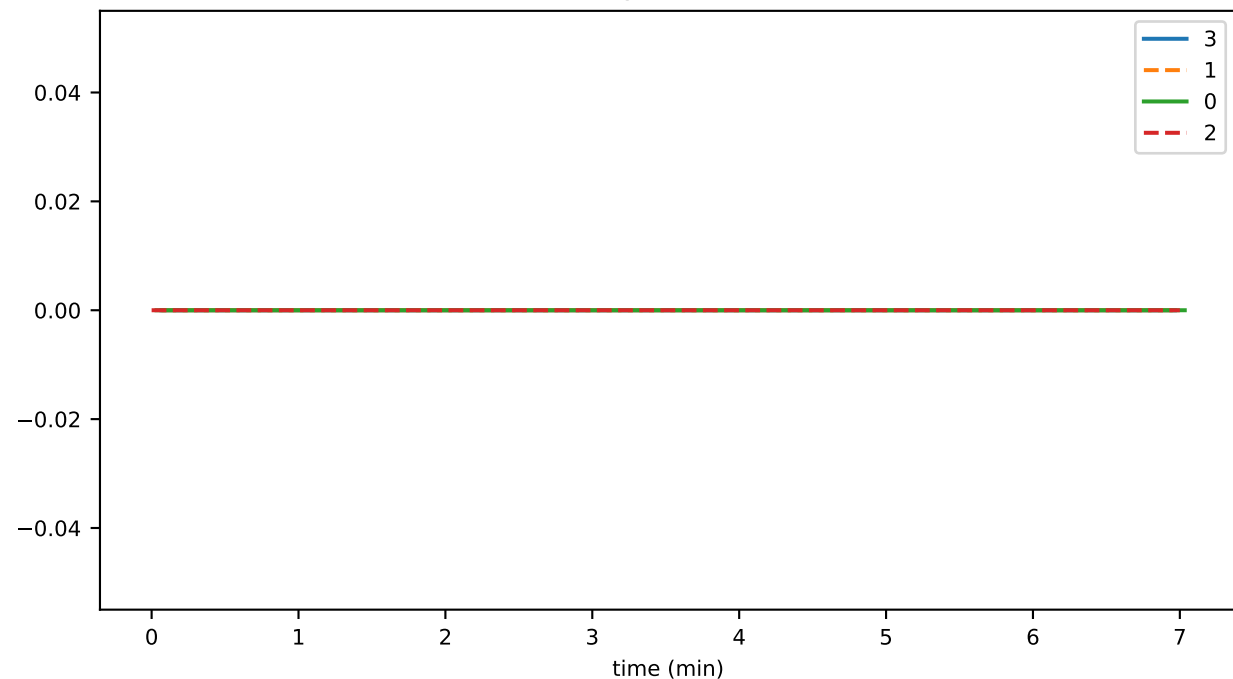
SigIntakeListSize
