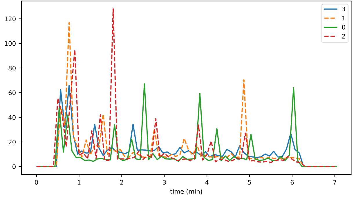
eventDelay_1_eventCreation_runtimeMAX
