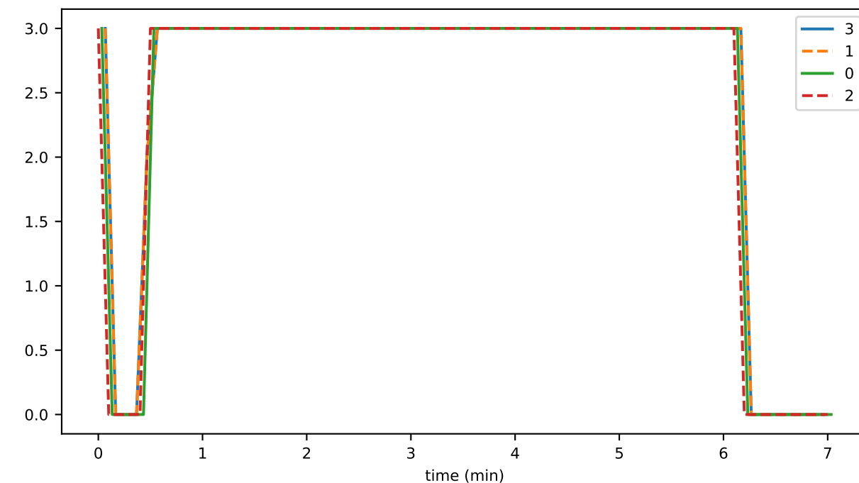
writeStateToDisk
