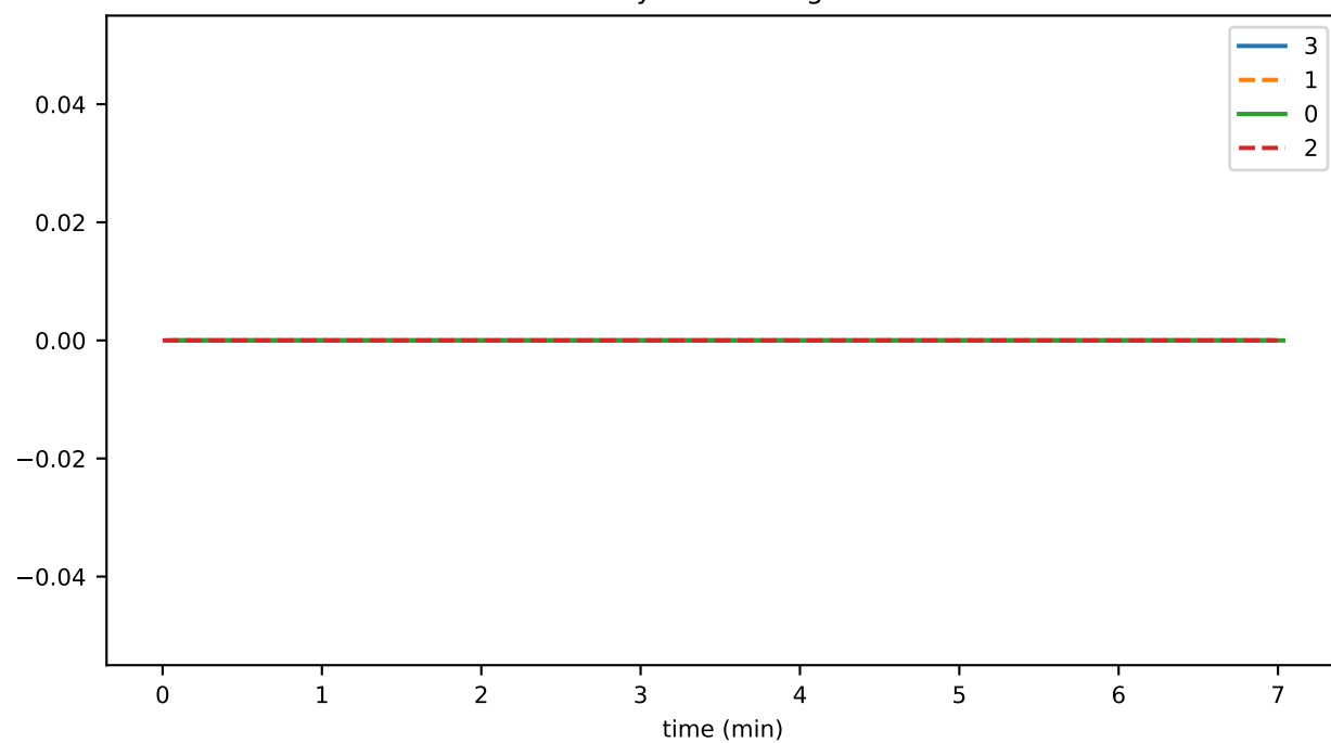
syncRoundLag
