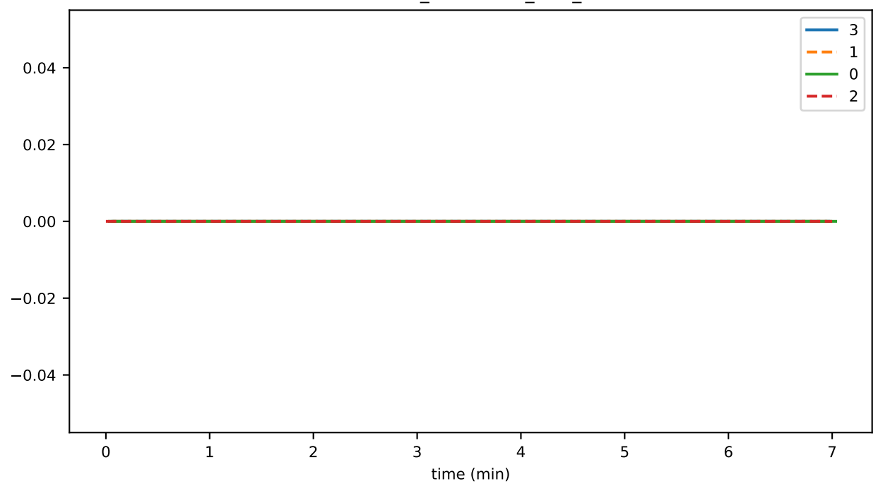
StateHasher_unhandled_task_count
