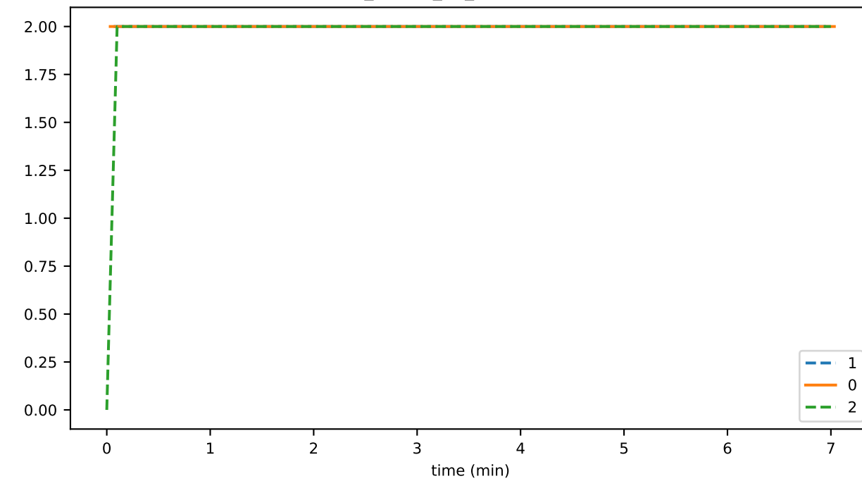
rpc_output_03_queueMaxSize
