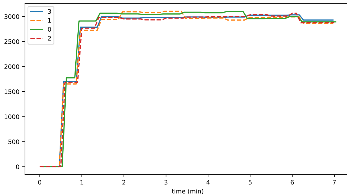
writeStateToDisk
