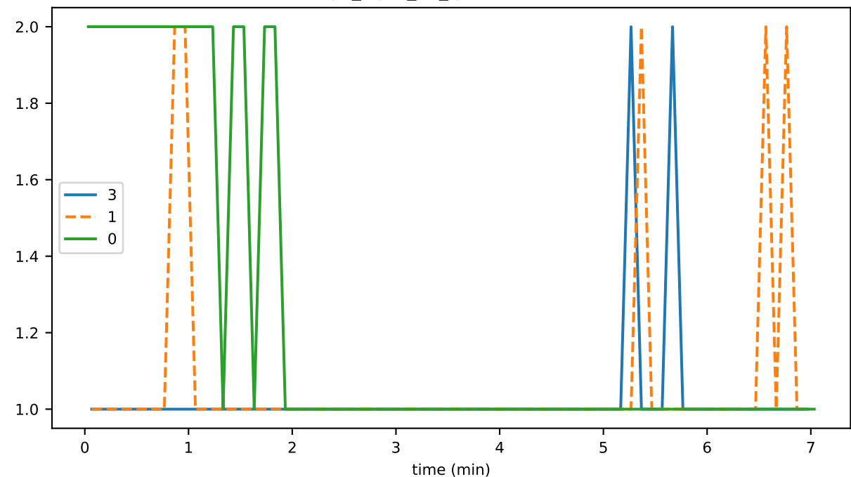
rpc_input_03_queueMaxSize
