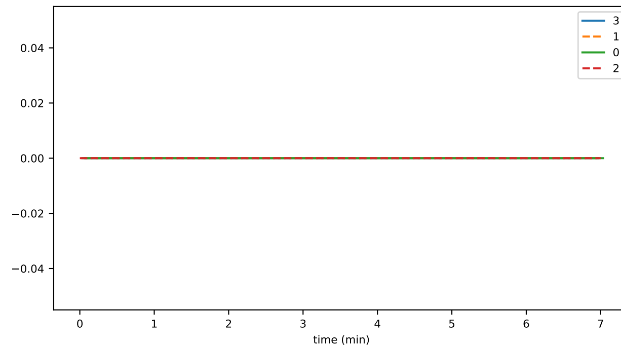
pcesAvgEventSize
