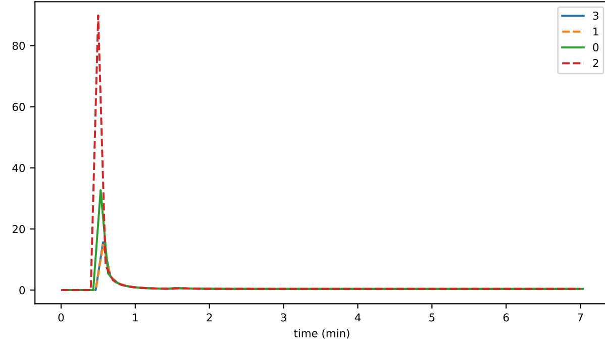
secC2RC
