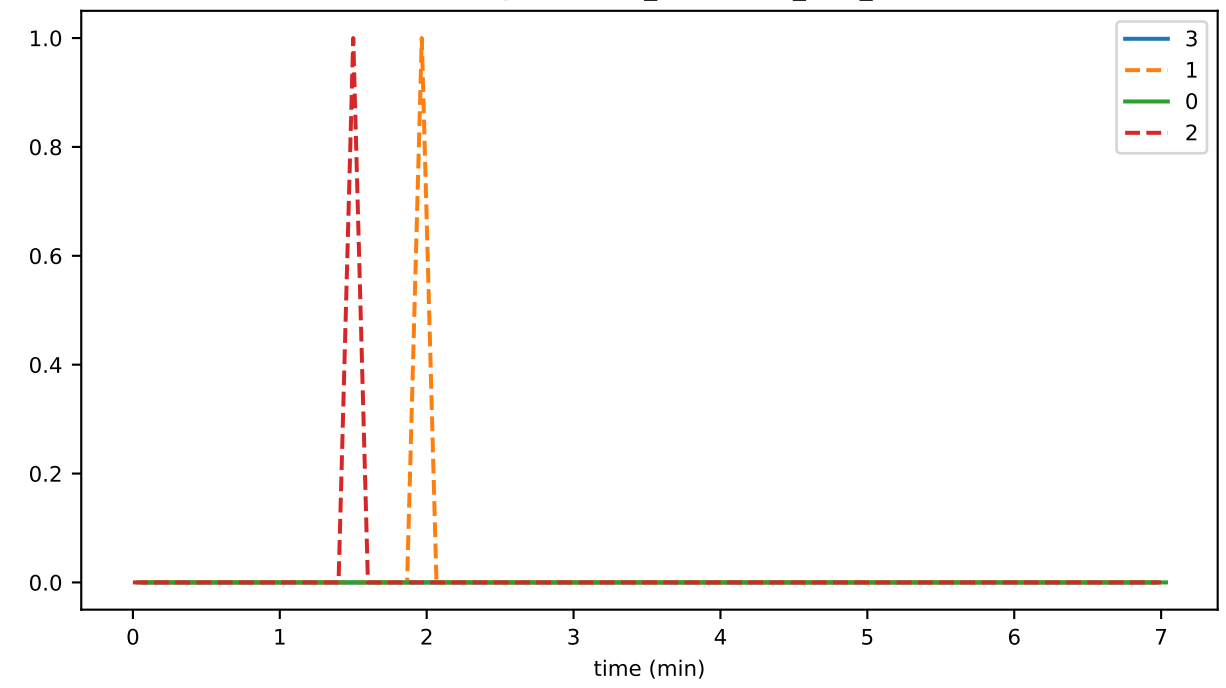
StateHasher_unhandled_task_count
