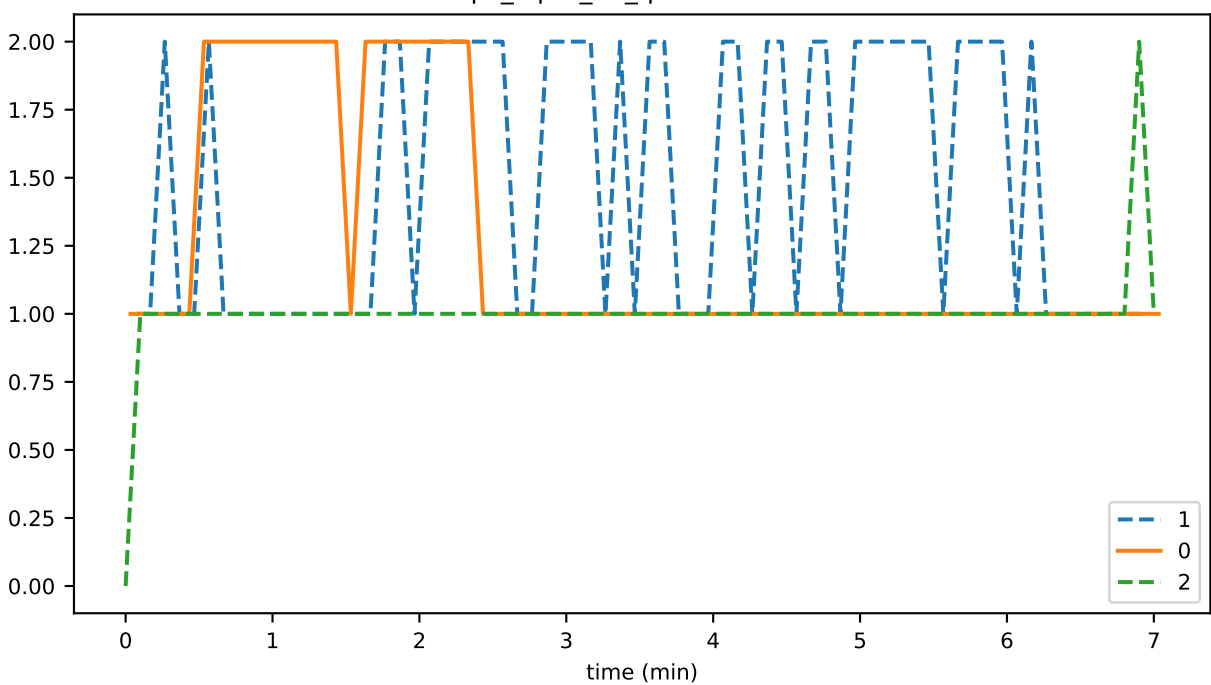
rpc_input_03_queueMaxSize
