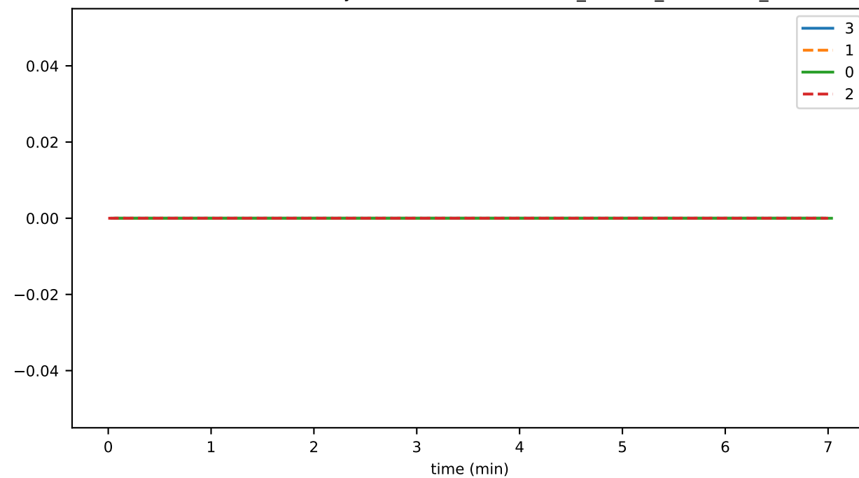
SmartContractService:SystemContractMethodCall_FREEZE_UNFREEZE_total
