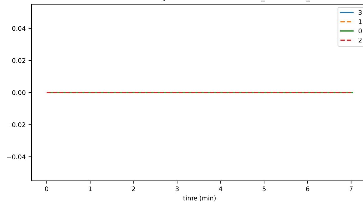
SmartContractService:SystemContractMethodCall_SCHEDULE_total
