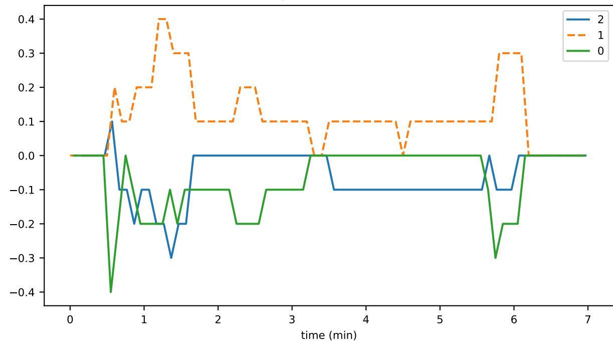
syncPermitsRevoked
