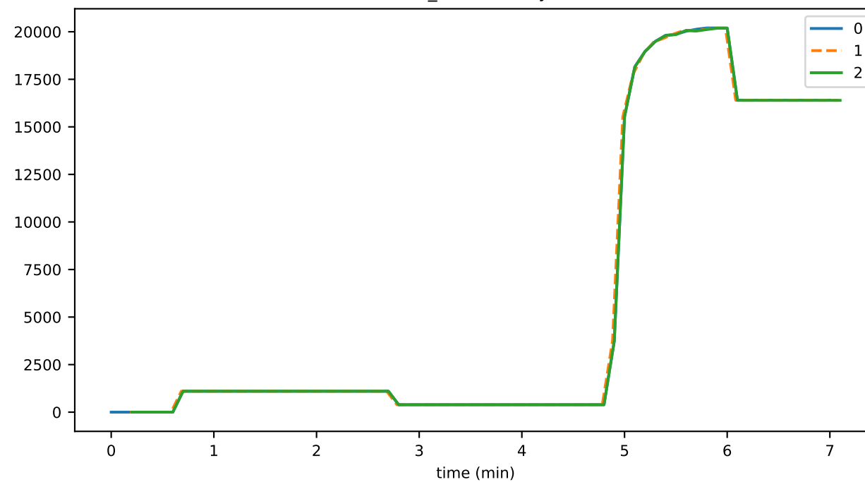
buffer_blockItemBytes
