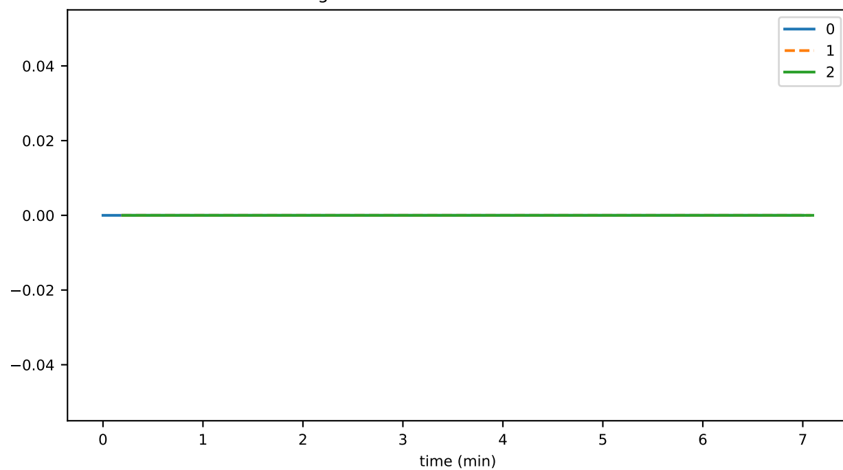
registeredNodeCreateThrottledTxns
