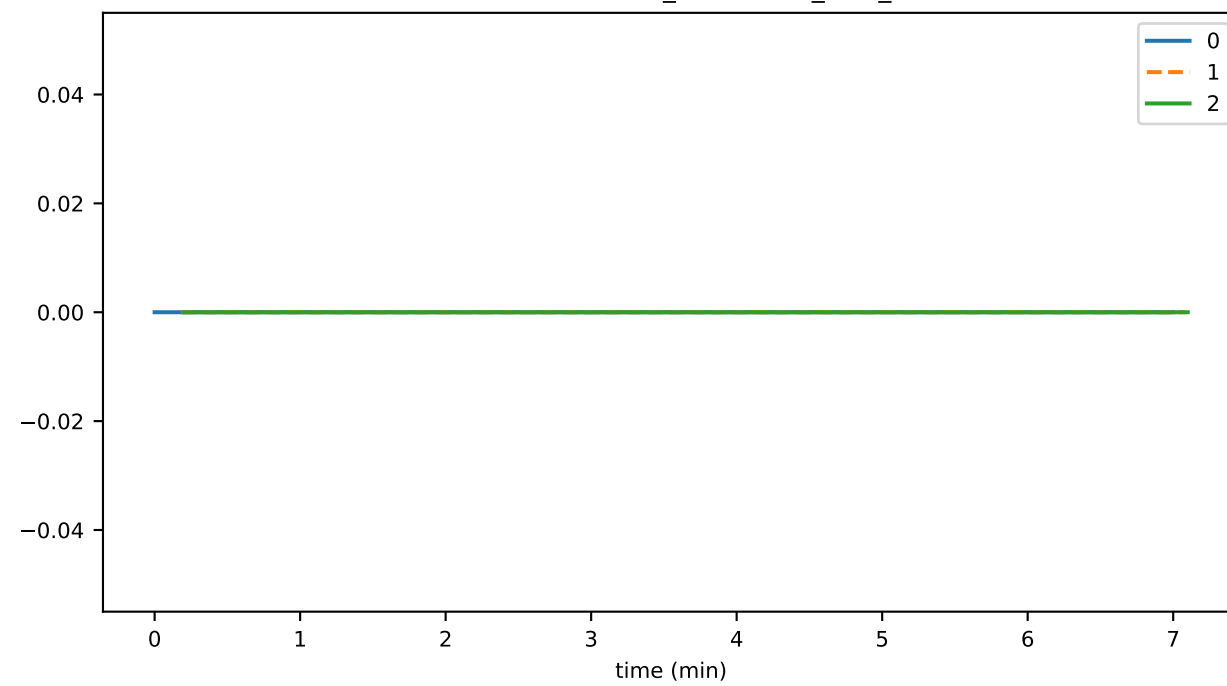
IssDetector_unhandled_task_count
