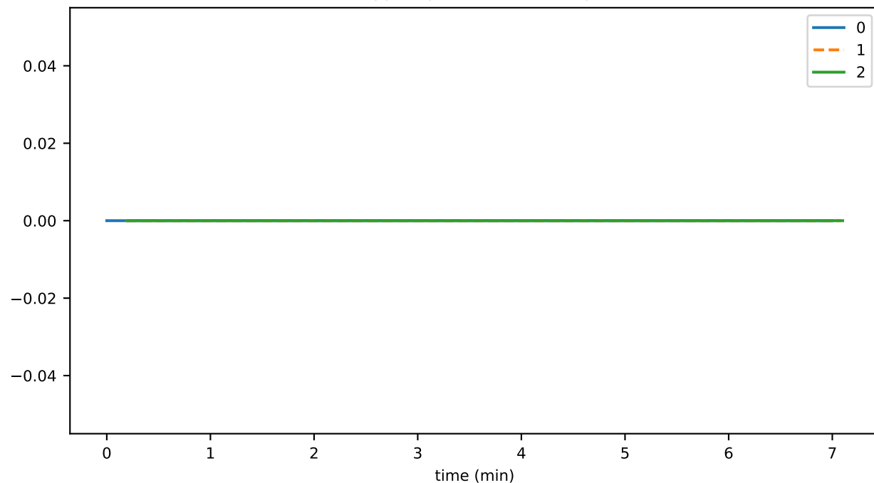
cryptoUpdateThrottledTxns
