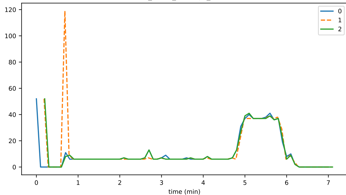
dupEv_per_sec
