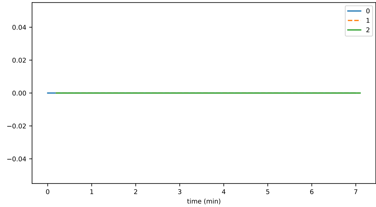
tokenGetAccountNftInfosThrottledTxns
