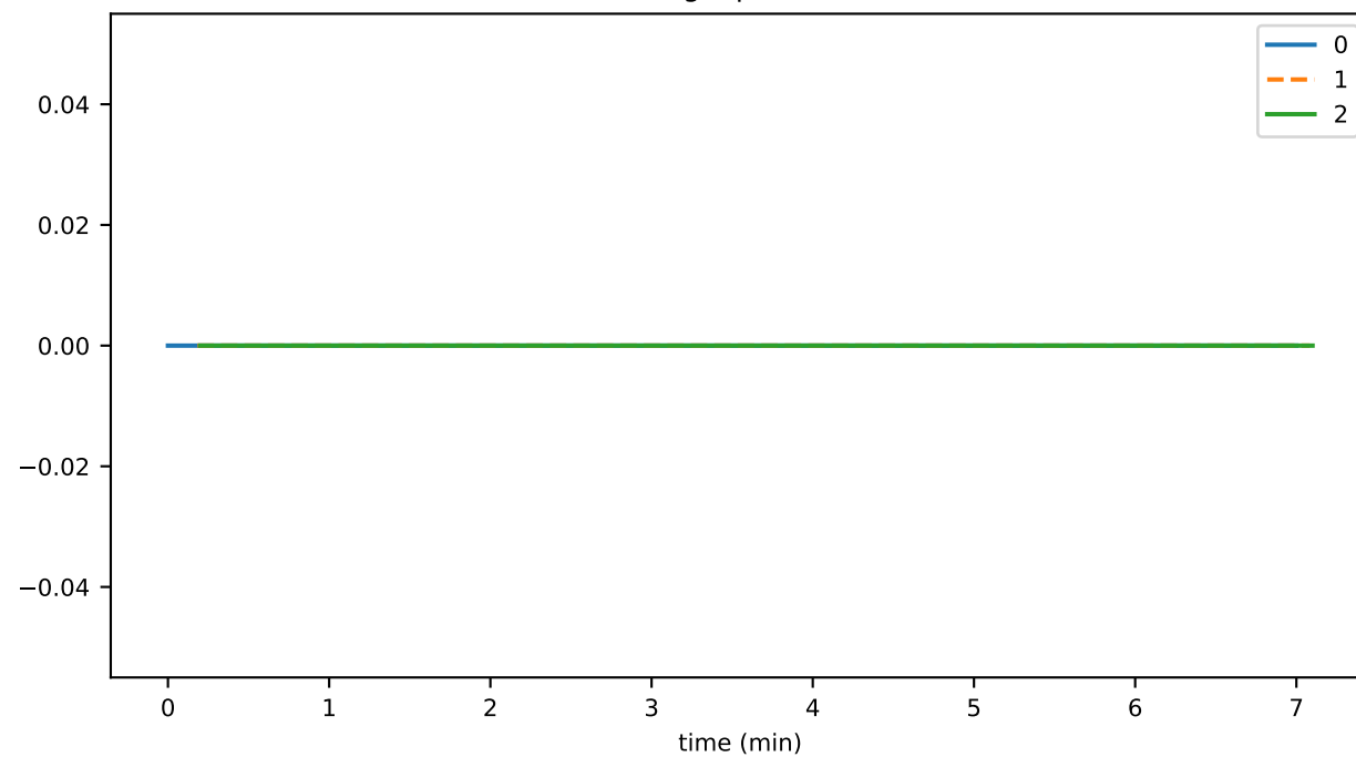
PlatSigExpandTime
