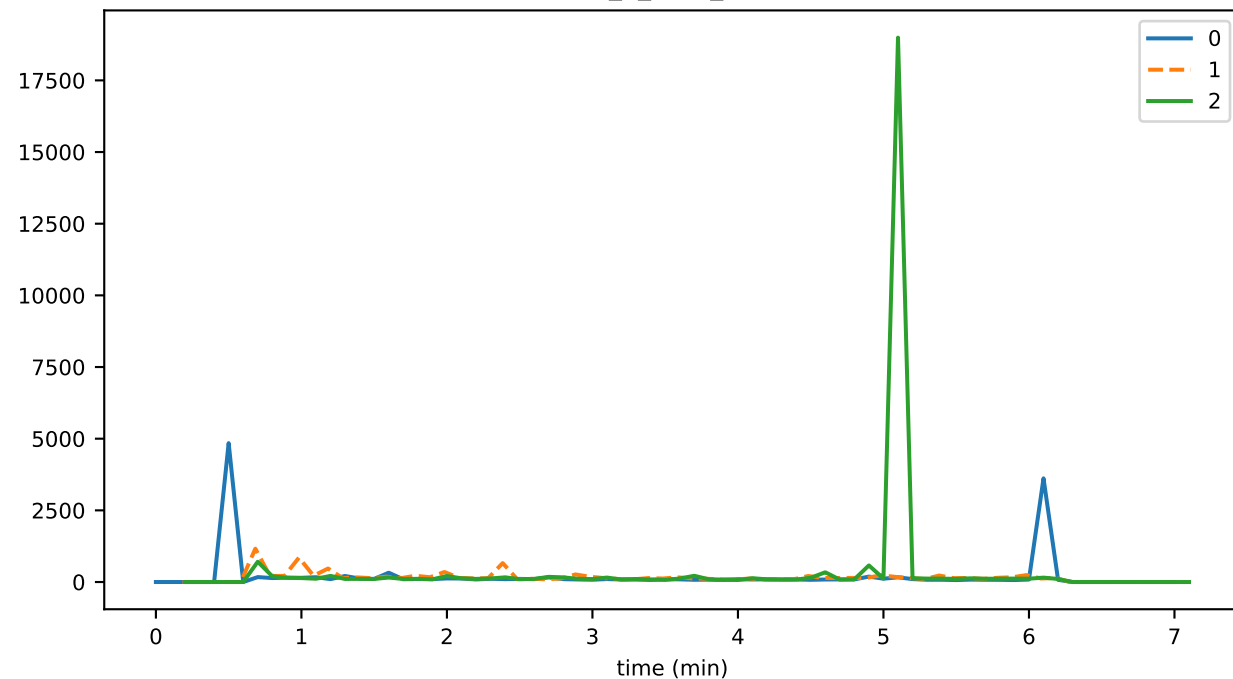
eventDelay_6_pces_runtimeMAX
