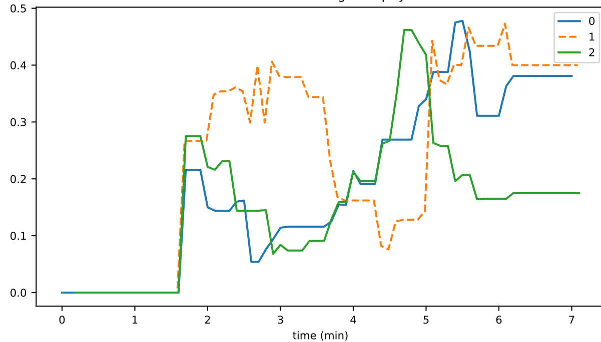
indicatorsWaitingForExpiry
