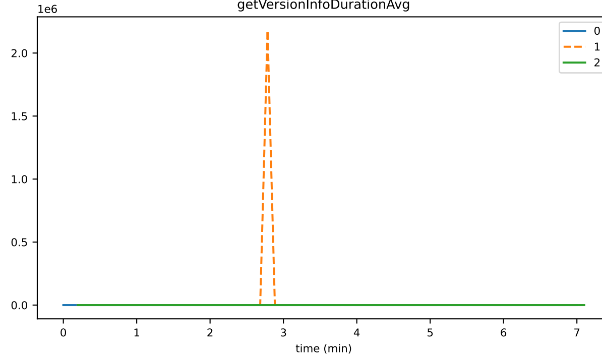
getVersionInfoDurationAvg
