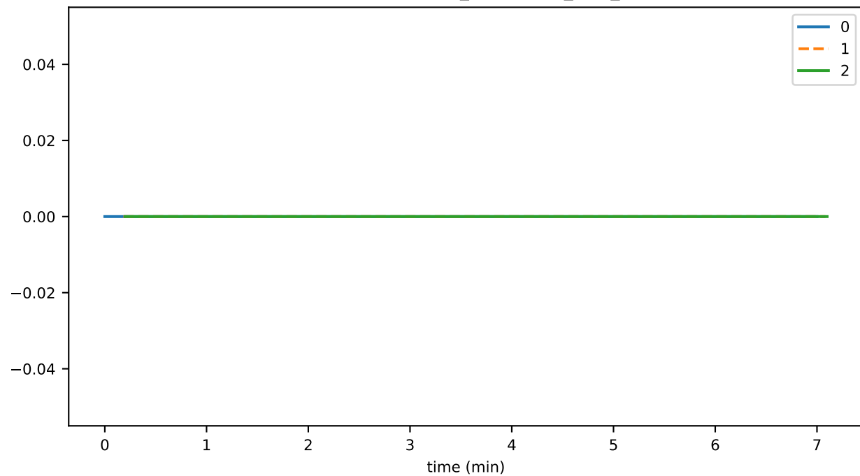
TransactionPrehandler_unhandled_task_count
