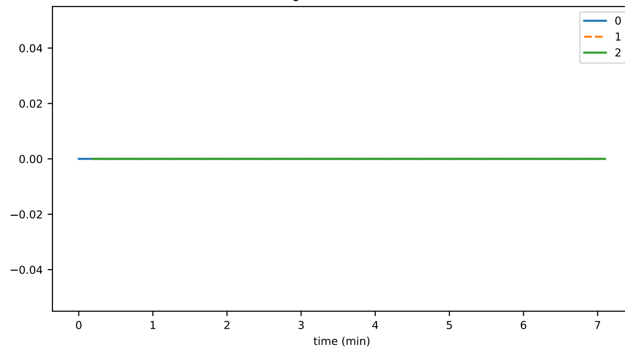
getAccountDetailsDurationMax
