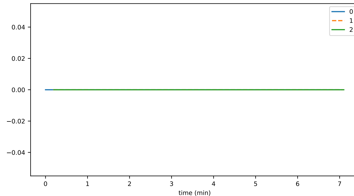
contractCallThrottledTxns
