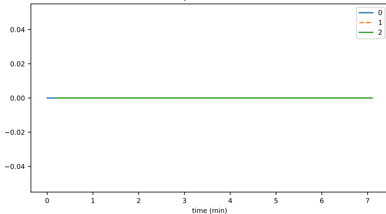
tokenGrantKycToAccountDurationMax
