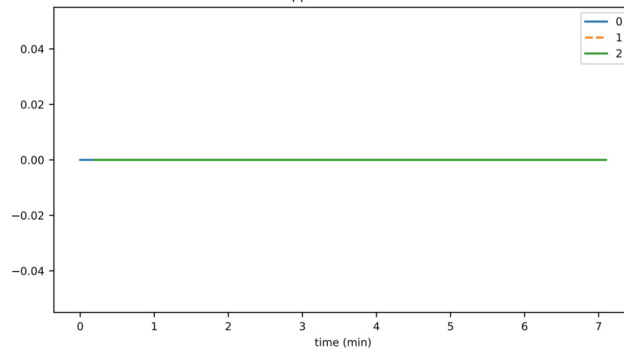
fileAppendThrottledTxns
