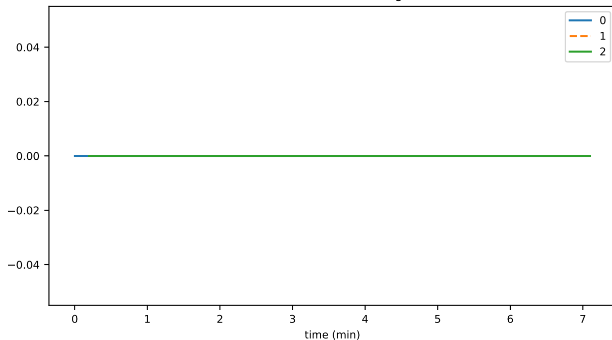
fileCreateThrottledTxns
