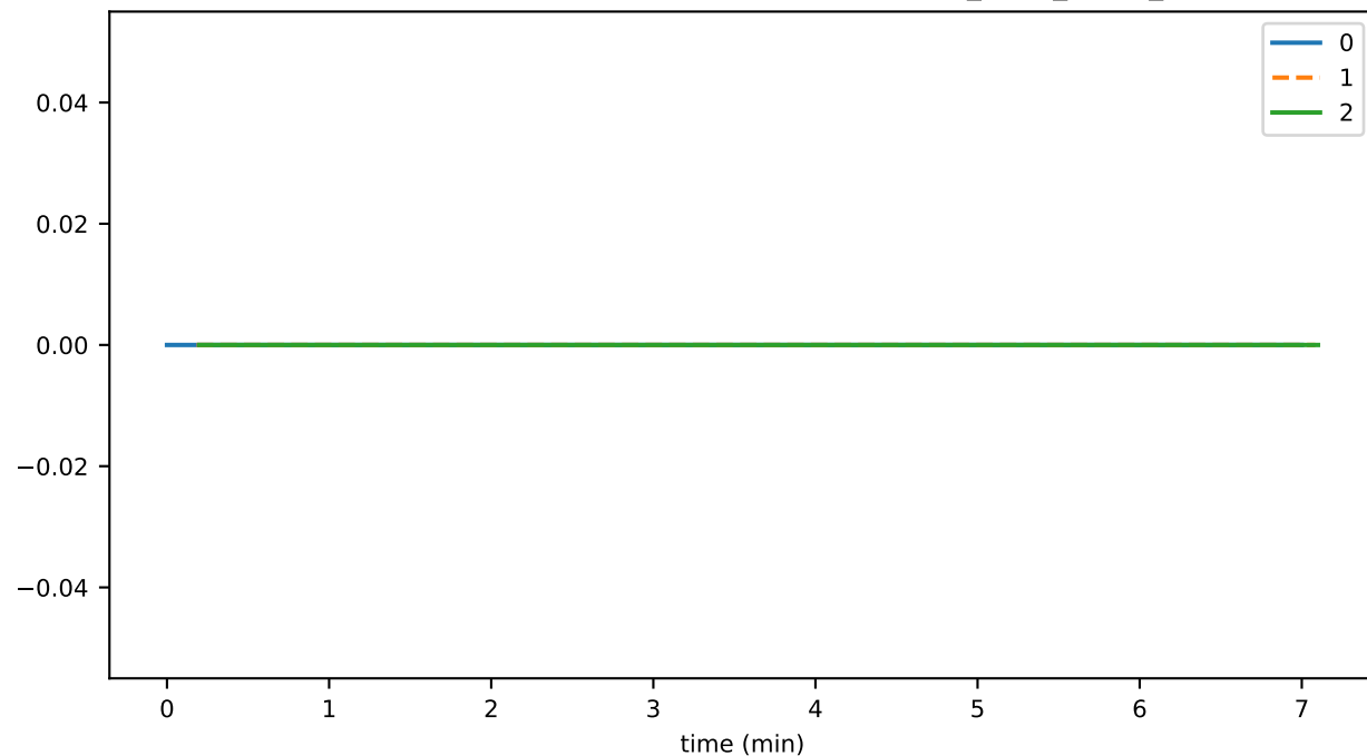
SmartContractService:SystemContractMethodCall_MINT_BURN_total
