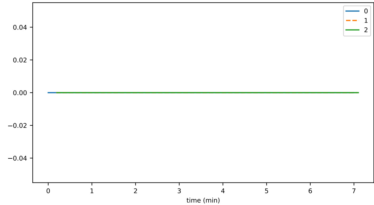
tokenFeeScheduleUpdateDurationAvg
