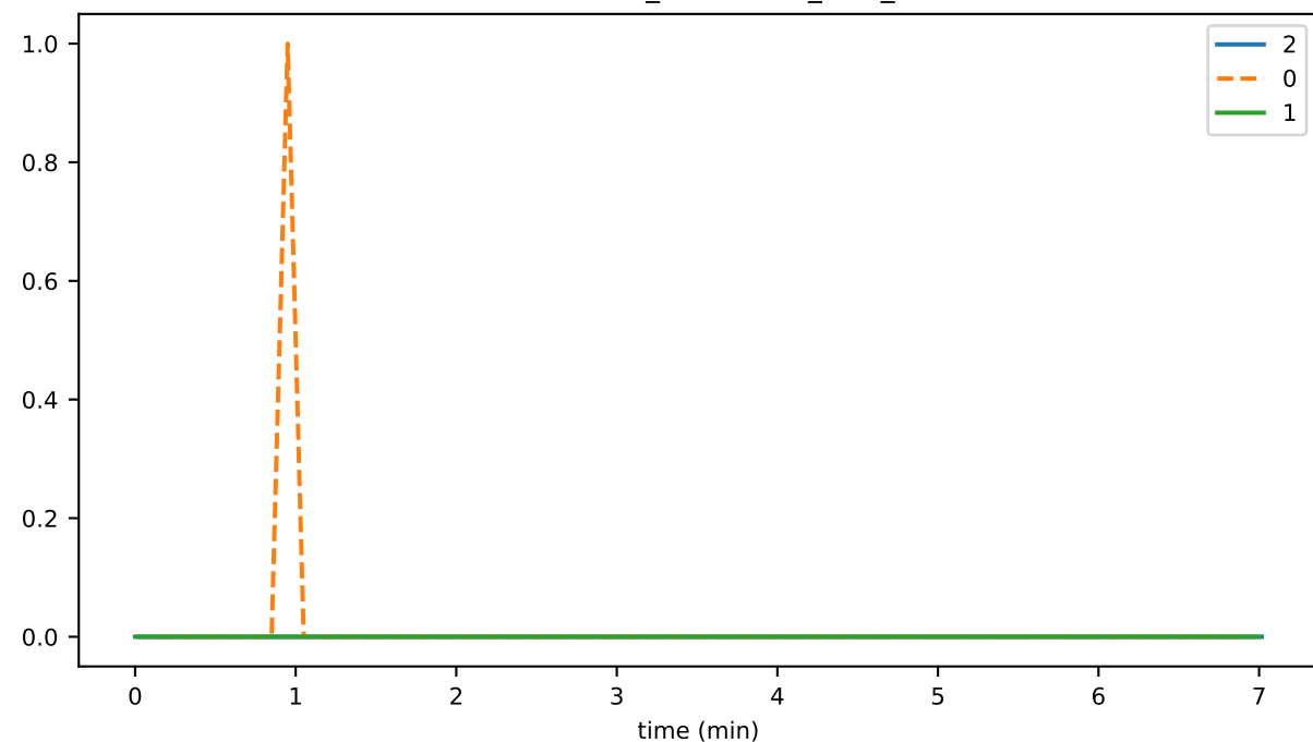
PlatSigEnqueueTime
