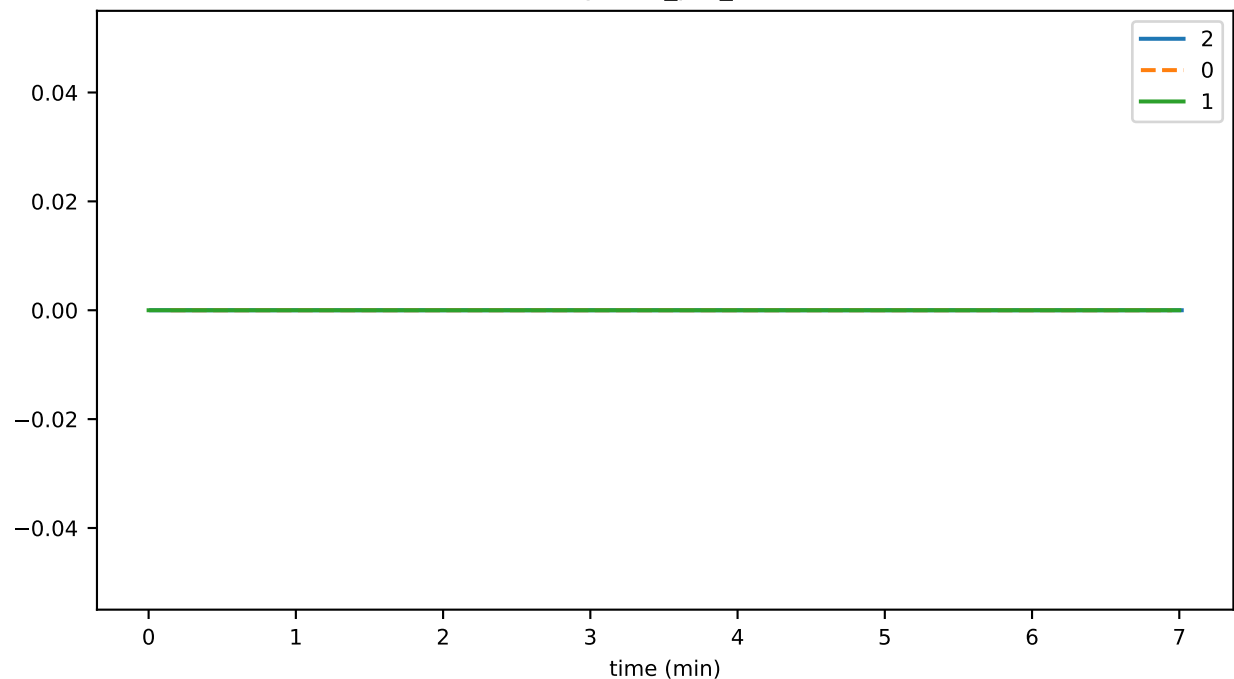
DigSliceSz
