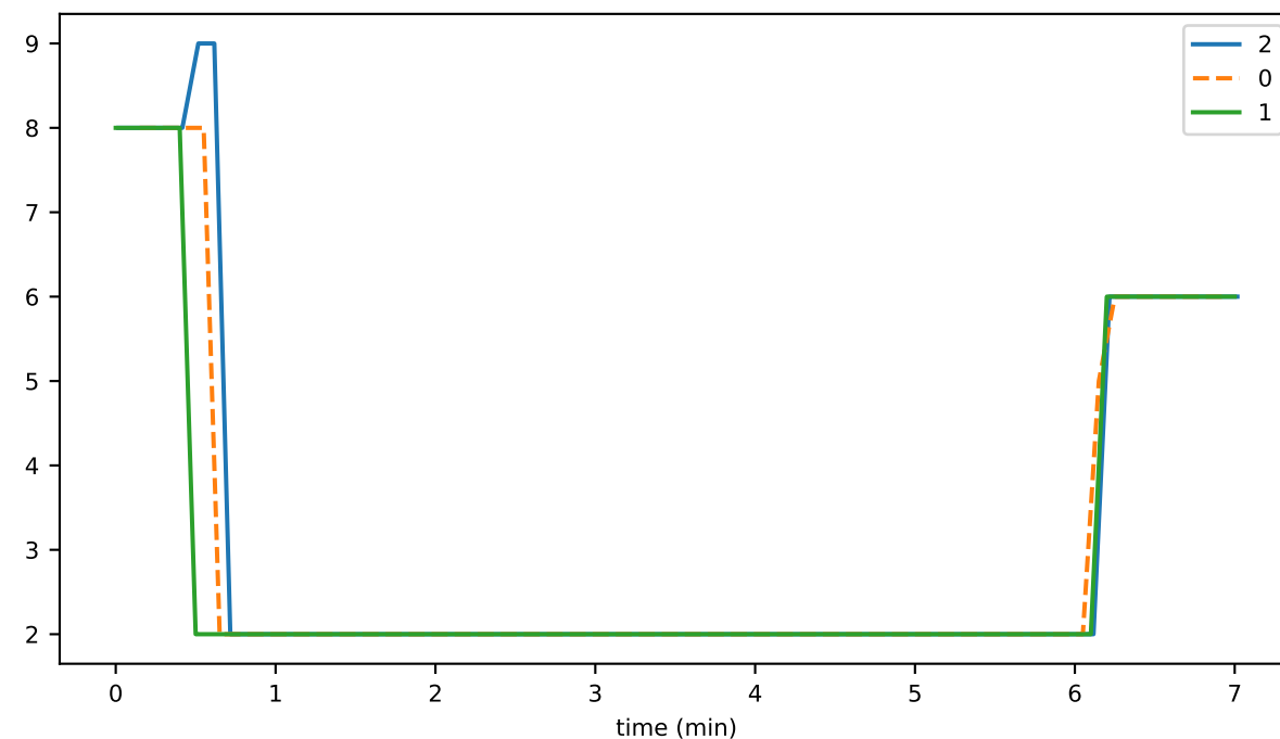
PlatSigExpandTime
