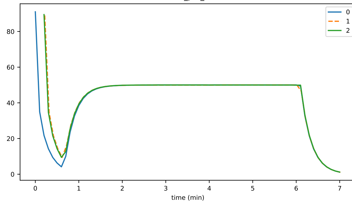
EventSignatureValidator_unhandled_task_count
