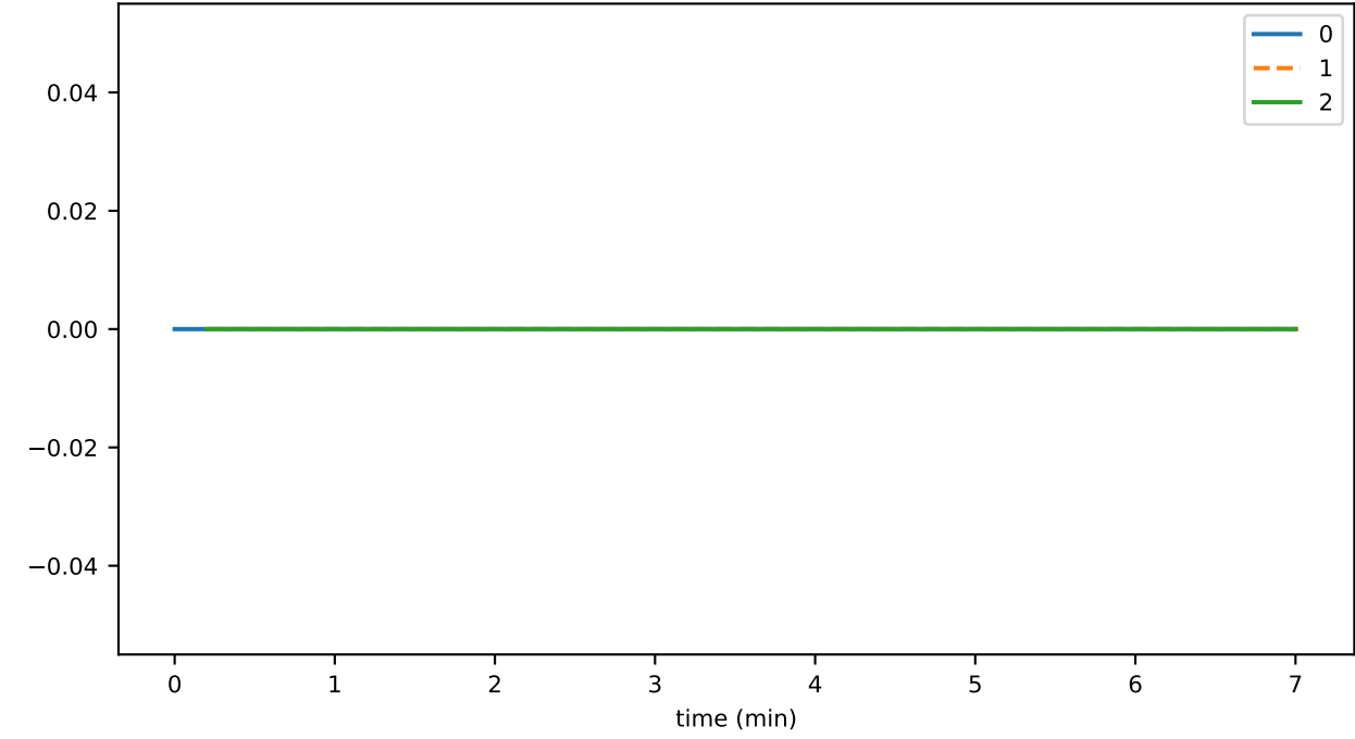
contractGetInfoThrottledTxns
