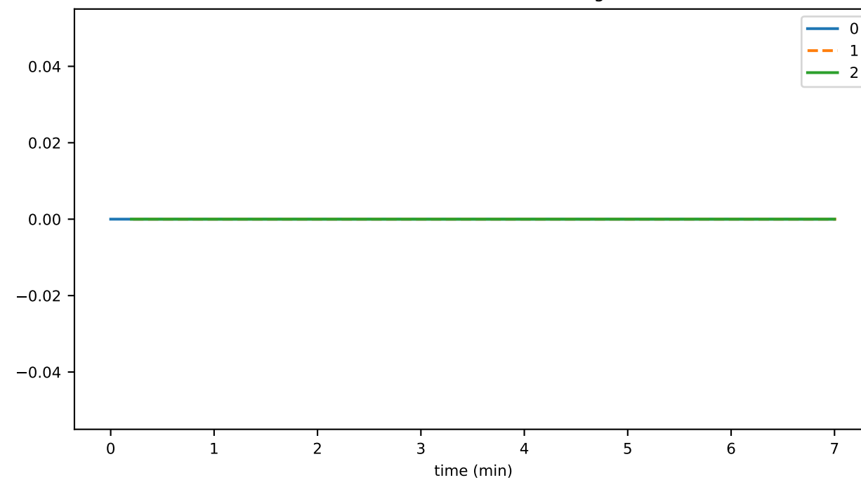
tokenGetNftInfosThrottledTxns
