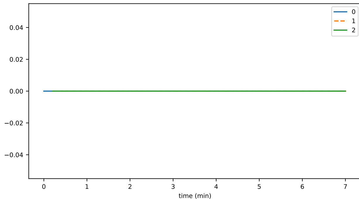
tokenGetNftInfosDurationMax
