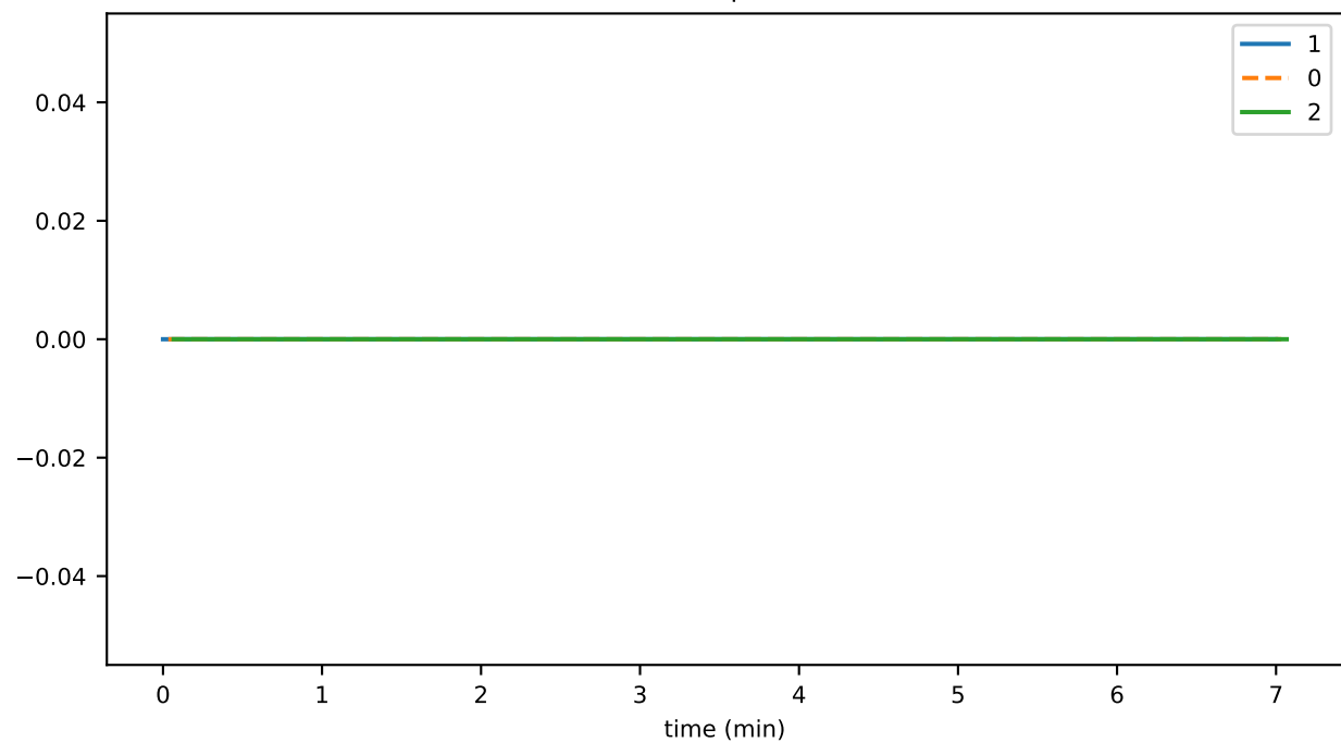
tokenAccountWipeDurationMax
