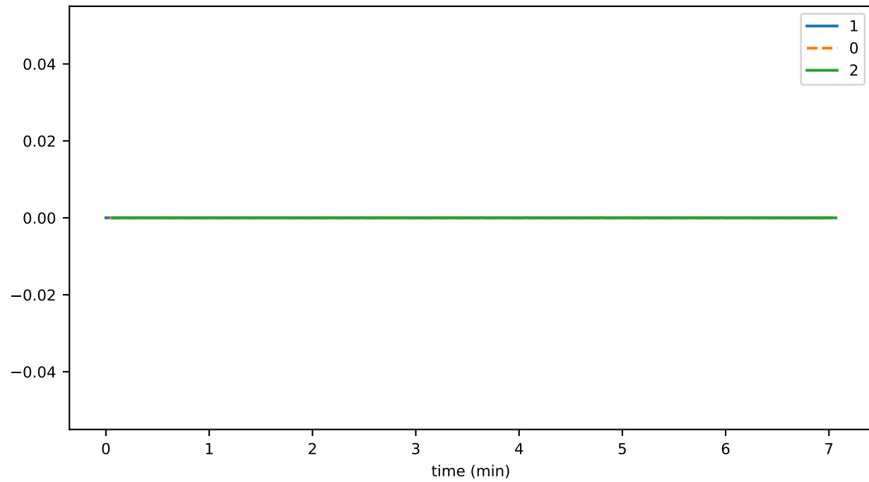
eventDelay_1_eventCreation_runtimeMAX
