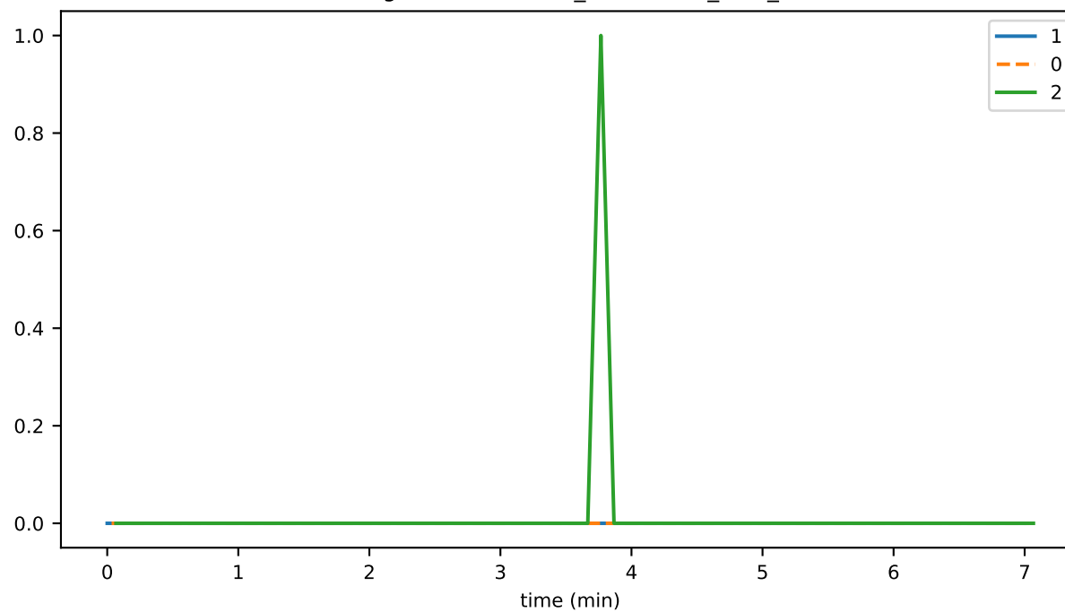
EventSignatureValidator_unhandled_task_count
