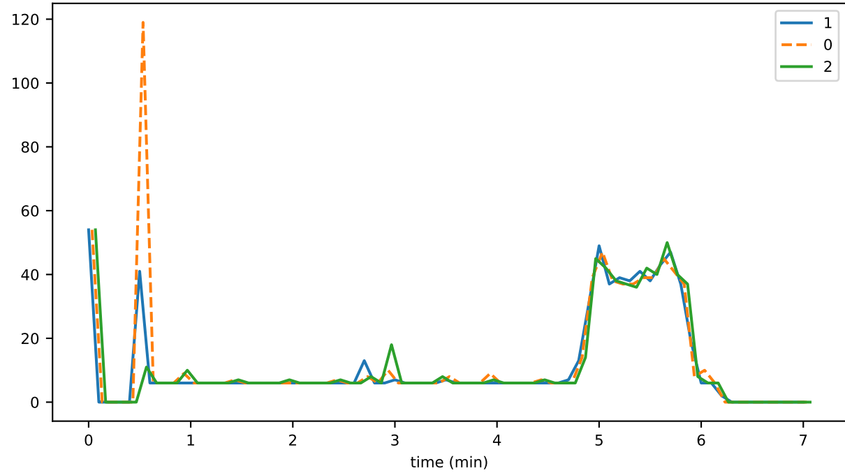
dupEv_per_sec
