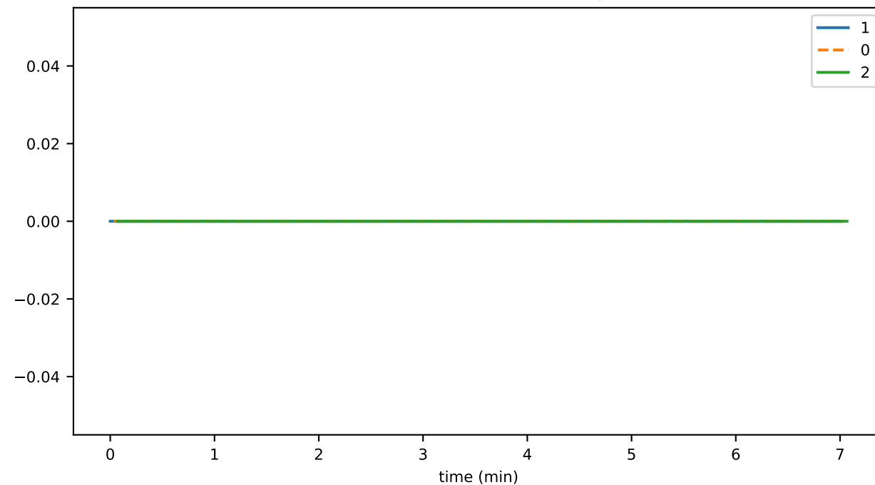
scheduleCreateThrottledTxns
