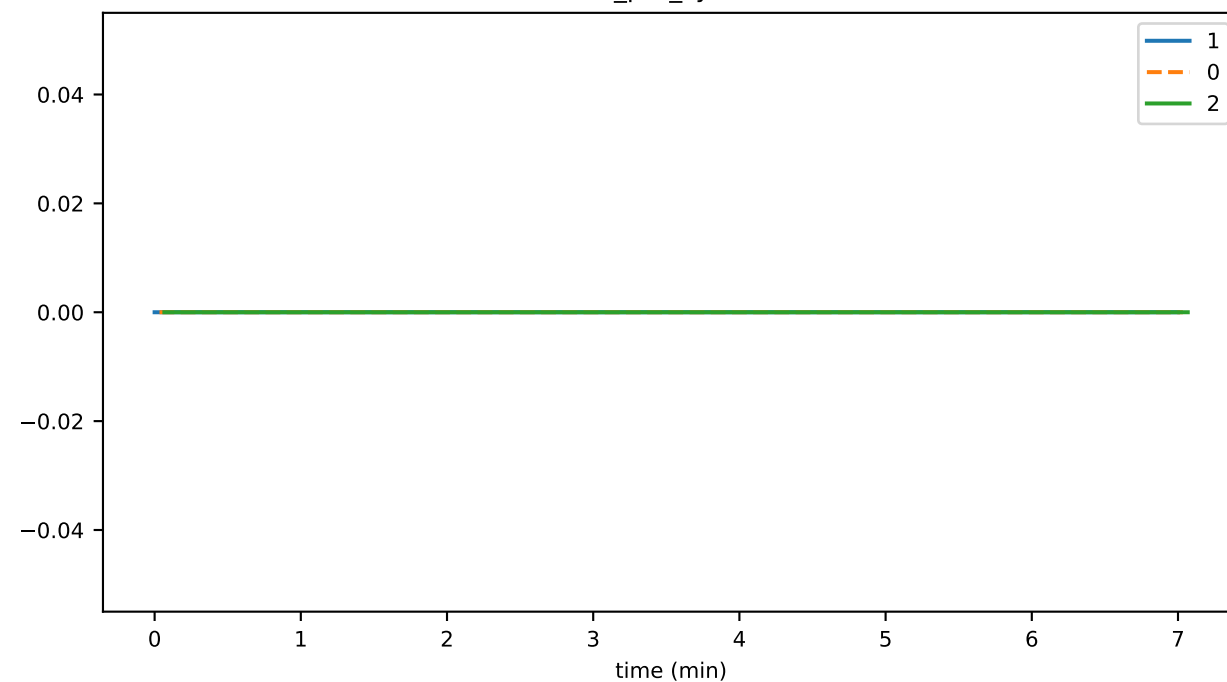
ev_per_syncS
