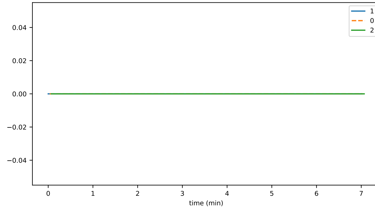
conn_connClose_periodicReset
