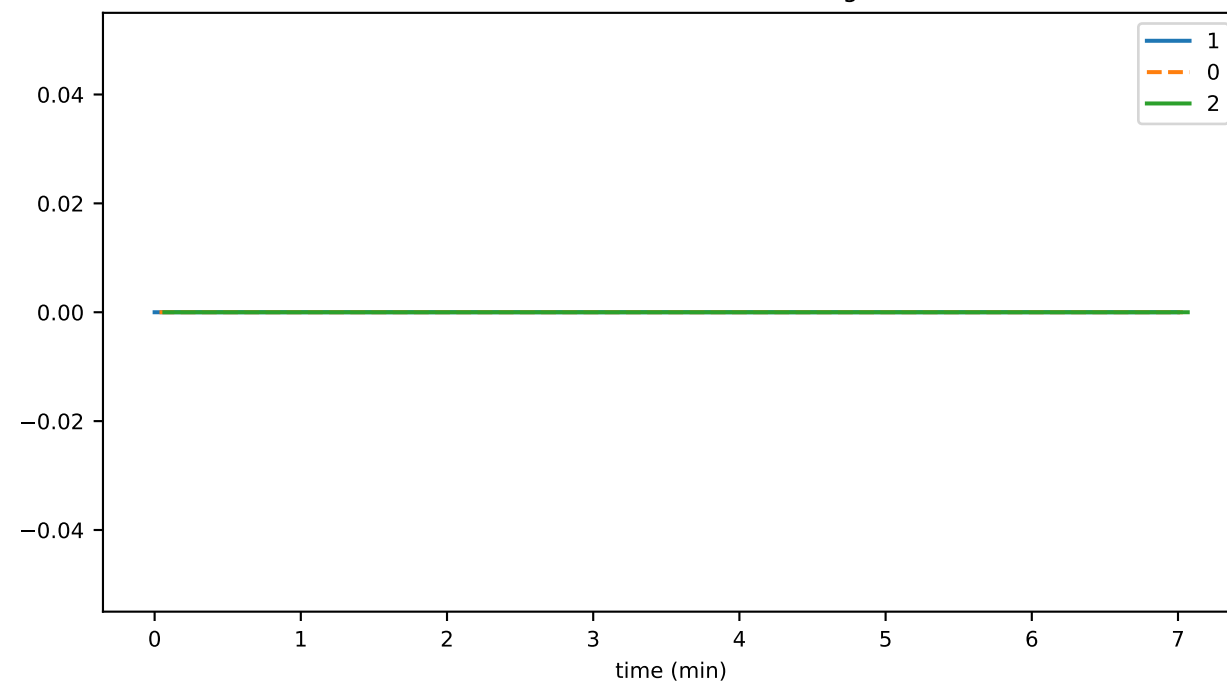
tokenGetNftInfosThrottledTxns
