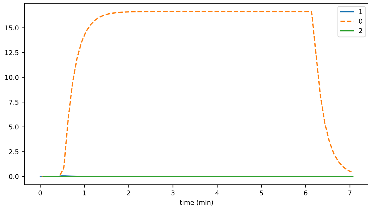
tokenAccountWipeDurationMax
