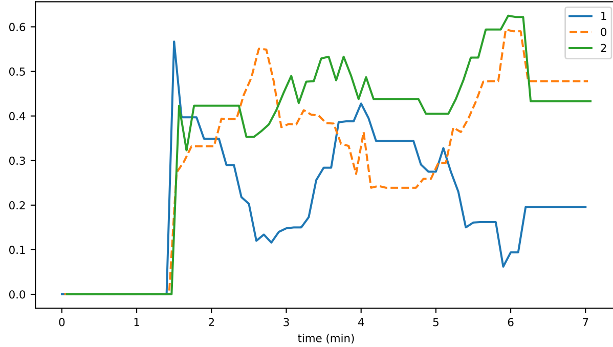
indicatorsWaitingForExpiry
