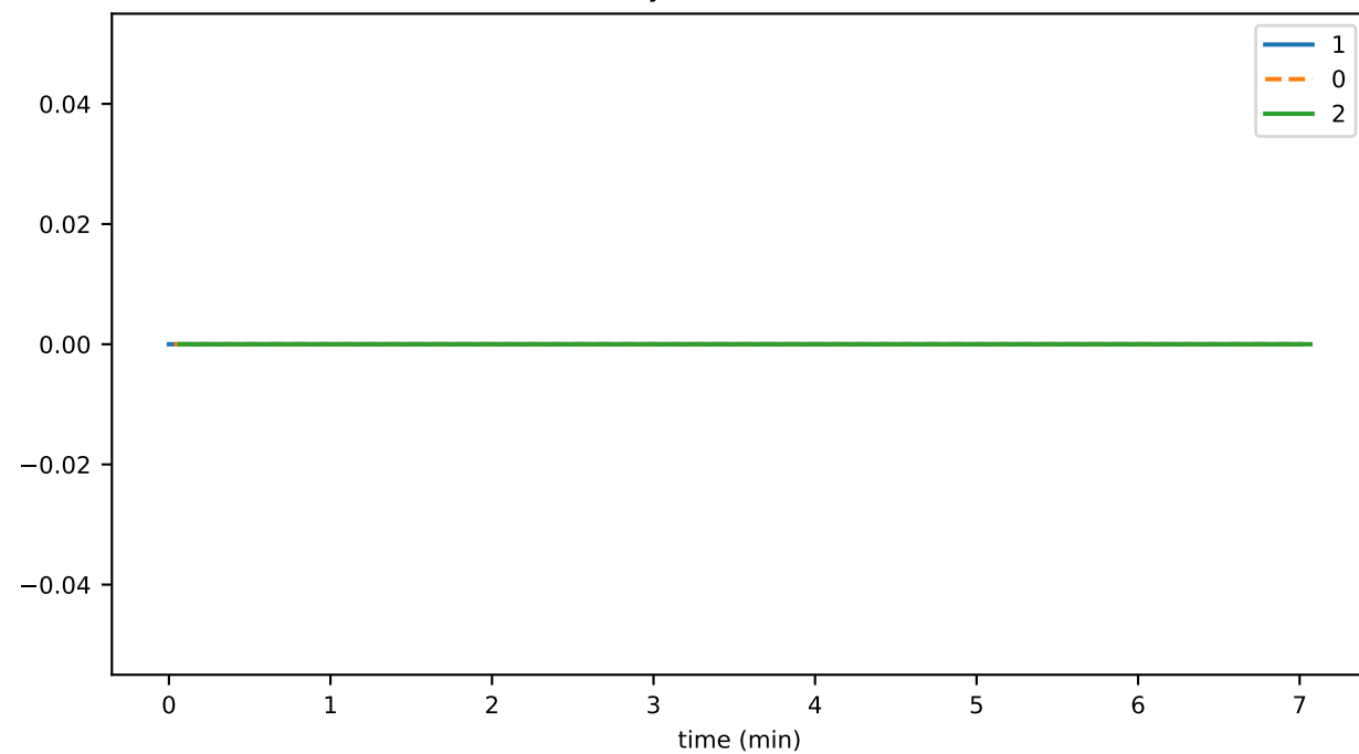
tokenGrantKycToAccountDurationMax
