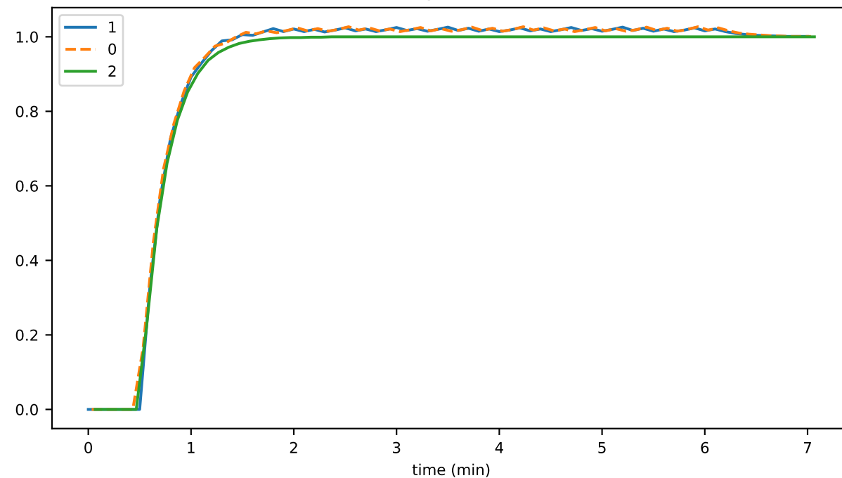
stateToDisk
