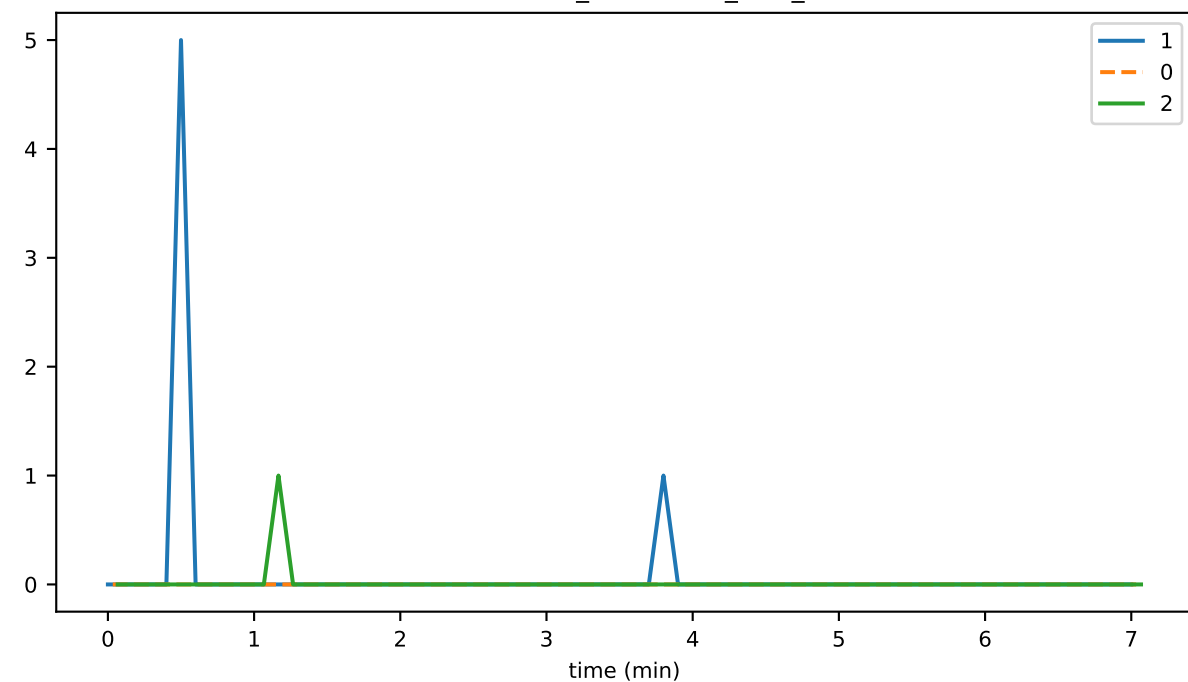
PlatSigEnqueueTime
