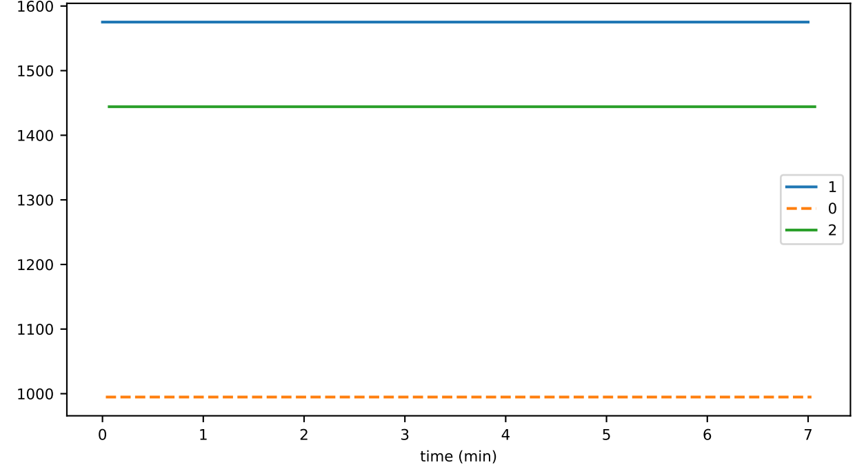
eventDelay_2_validation_gossip
