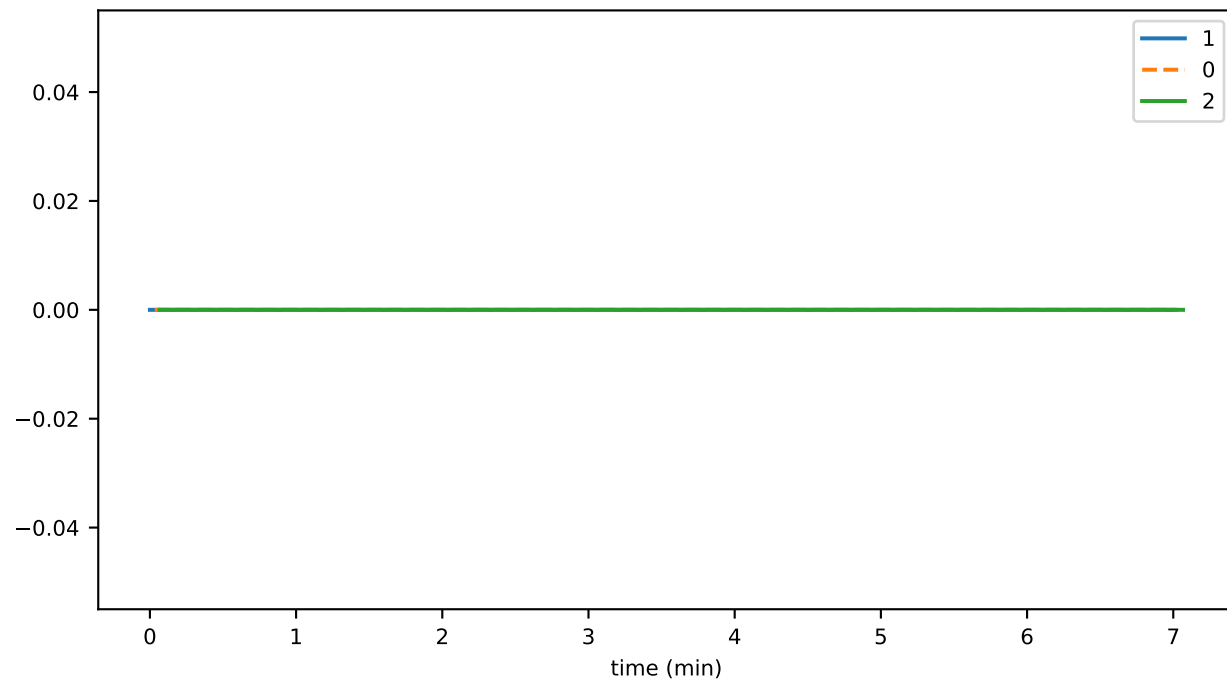
SigIntakeListSize
