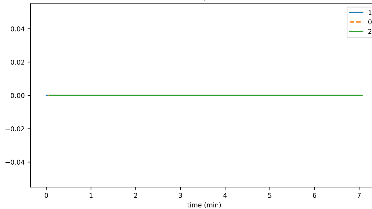
tokenAccountWipeThrottledTxns
