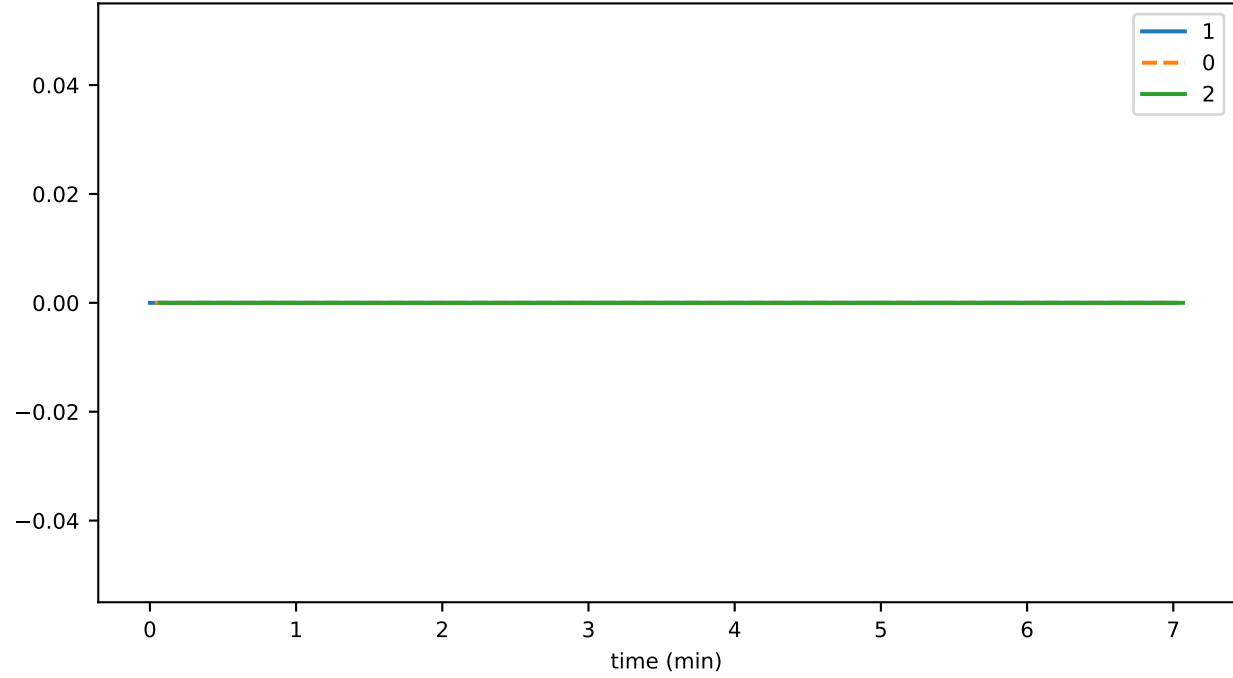
dupEv_per_sec
