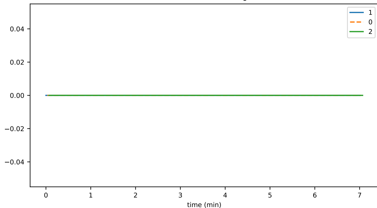
fileCreateThrottledTxns
