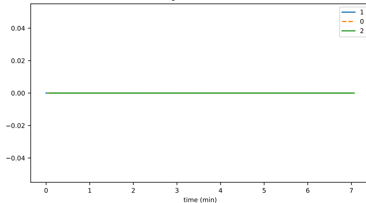
getAccountDetailsDurationMax
