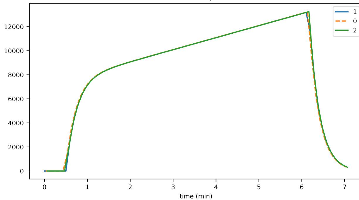
roundSup
