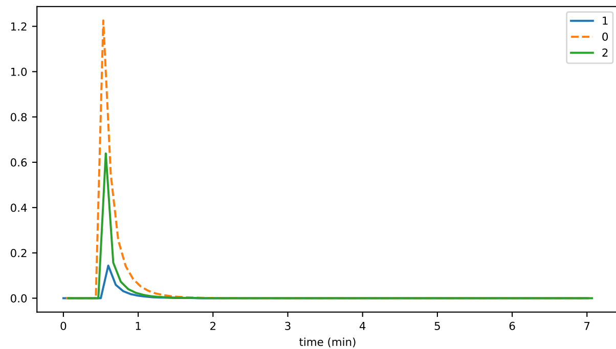
Sig_per_sec
