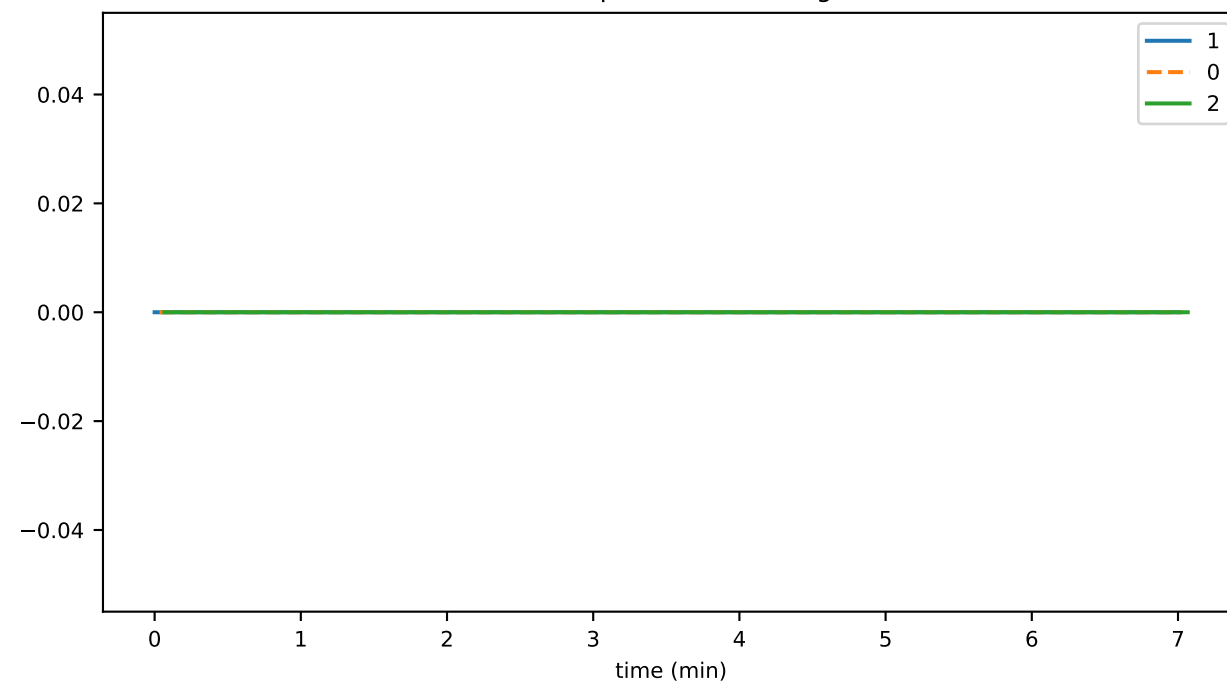
tokenUpdateNftsDurationAvg
