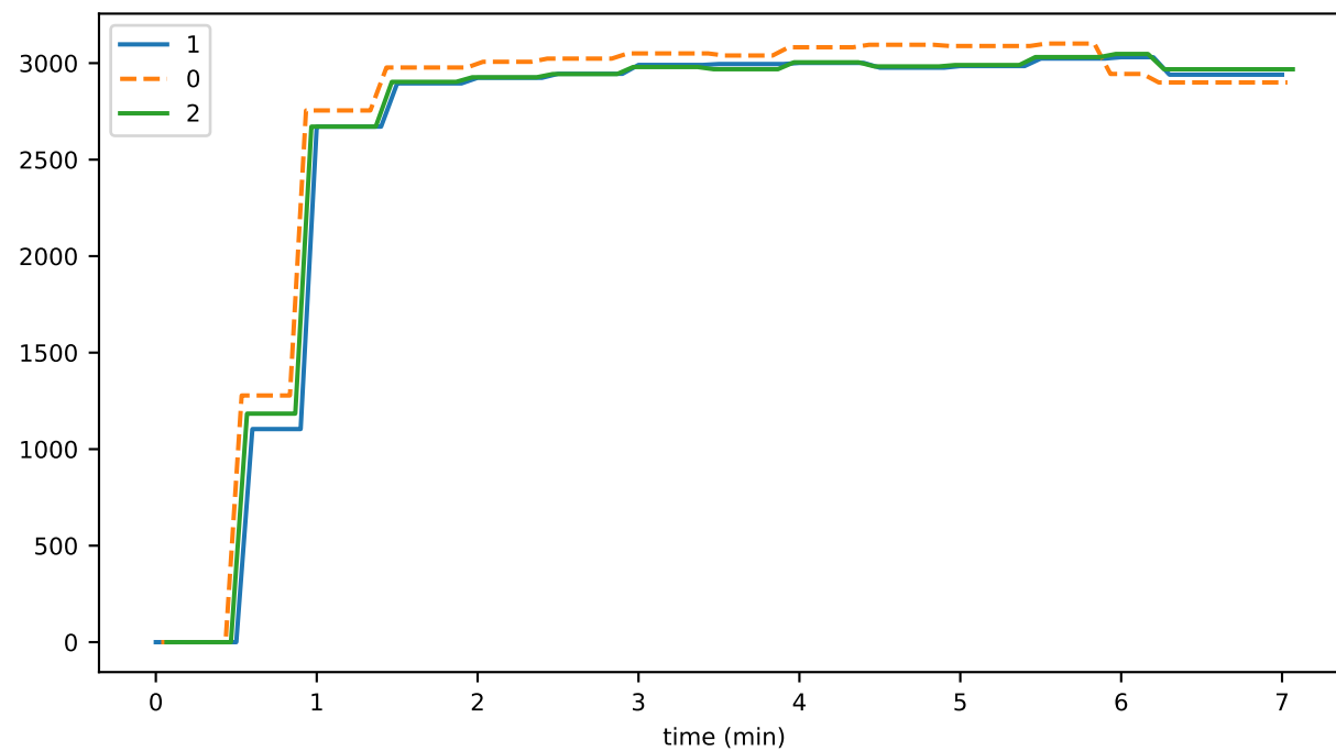
stateToDisk
