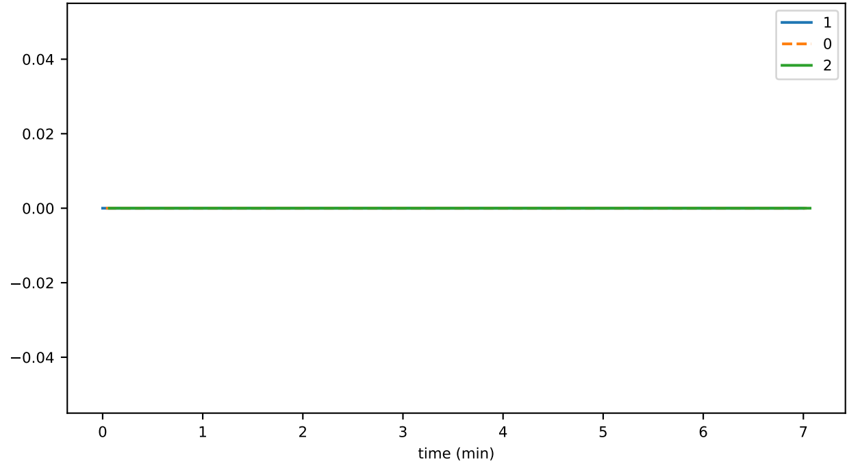
timeFracDot
