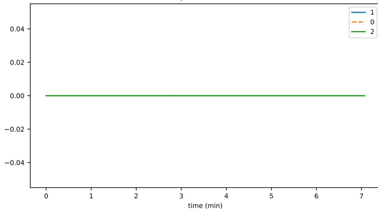
tokenUpdateThrottledTxns
