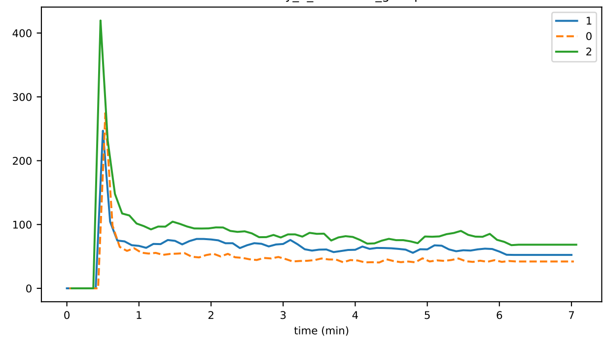
eventDelay_2_validation_gossip
