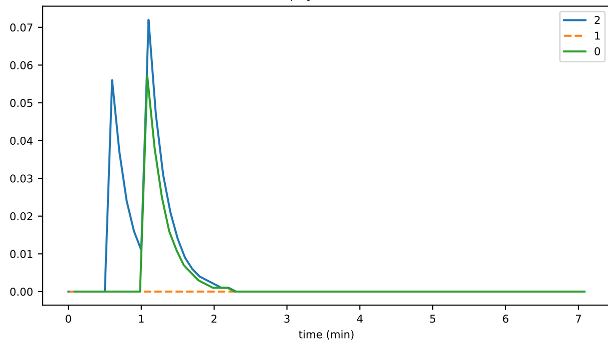
pityParent1
