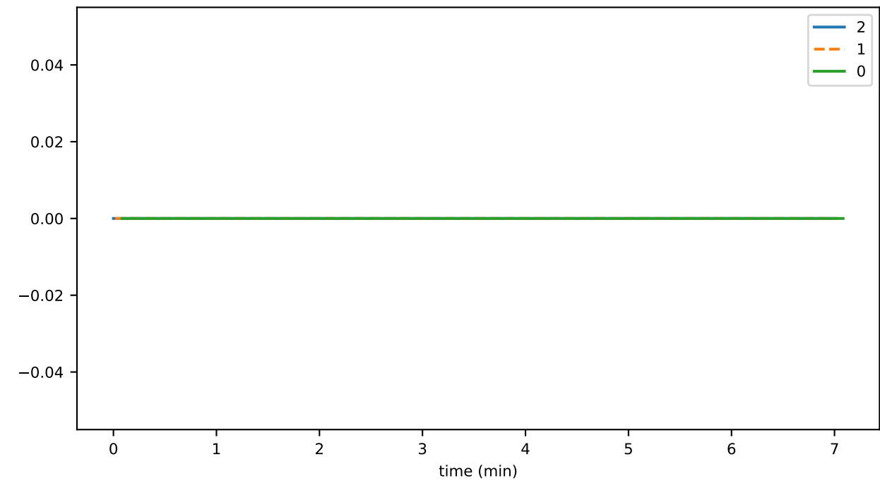
nftsUsed
