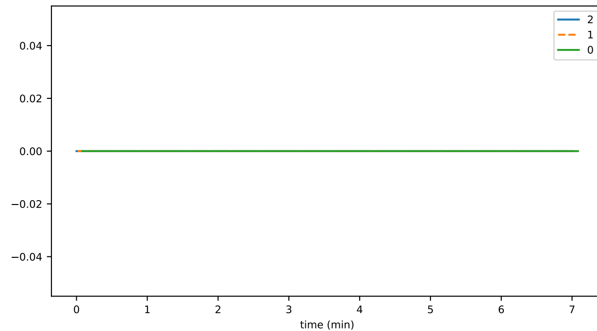
tokenBurnThrottledTxns
