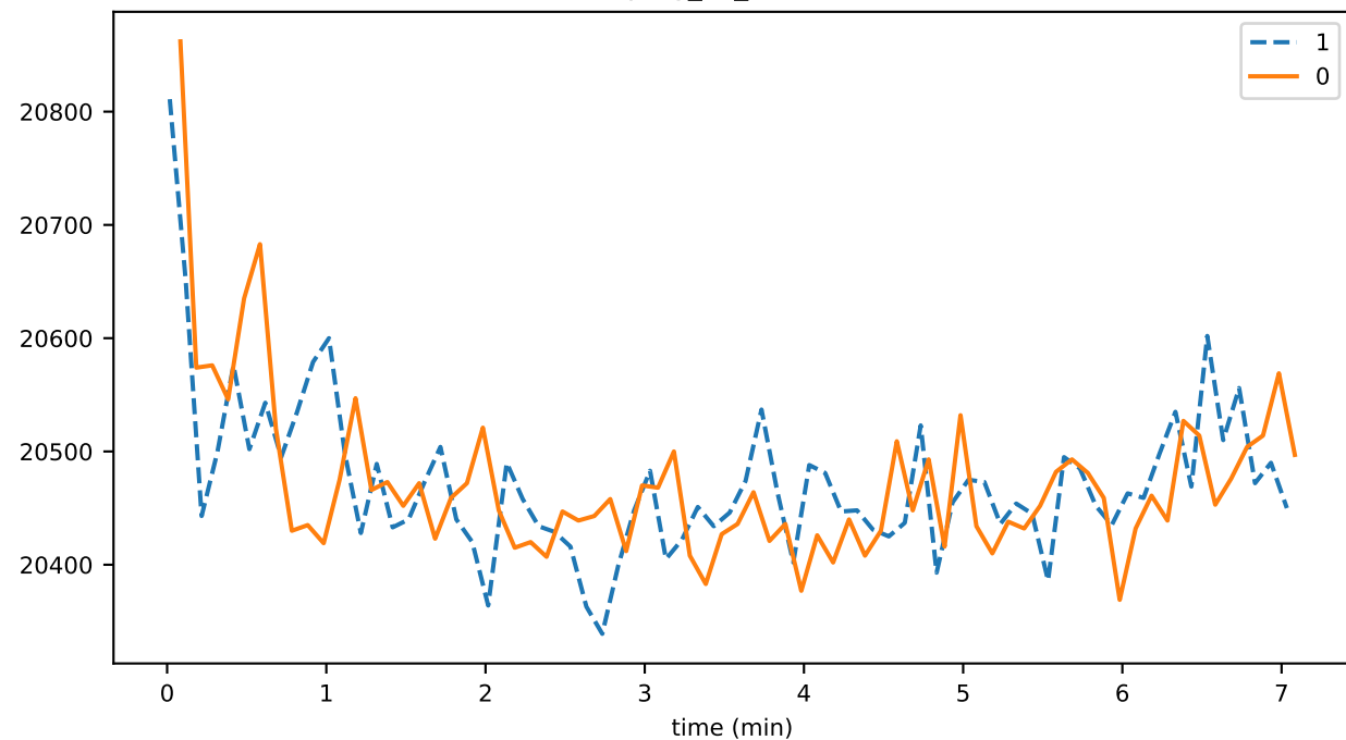
pityParent1
