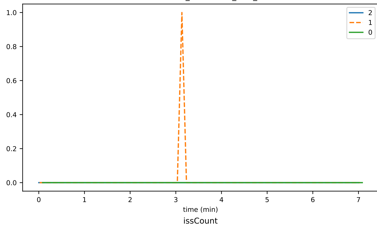
InlinePcesWriter_unhandled_task_count
