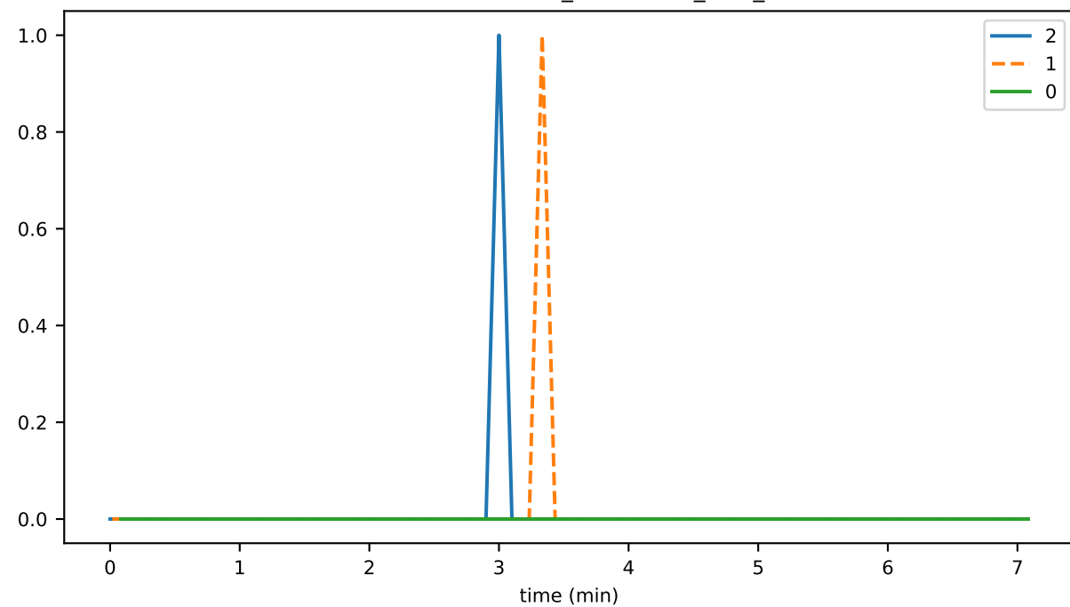
TransactionPrehandler_unhandled_task_count
