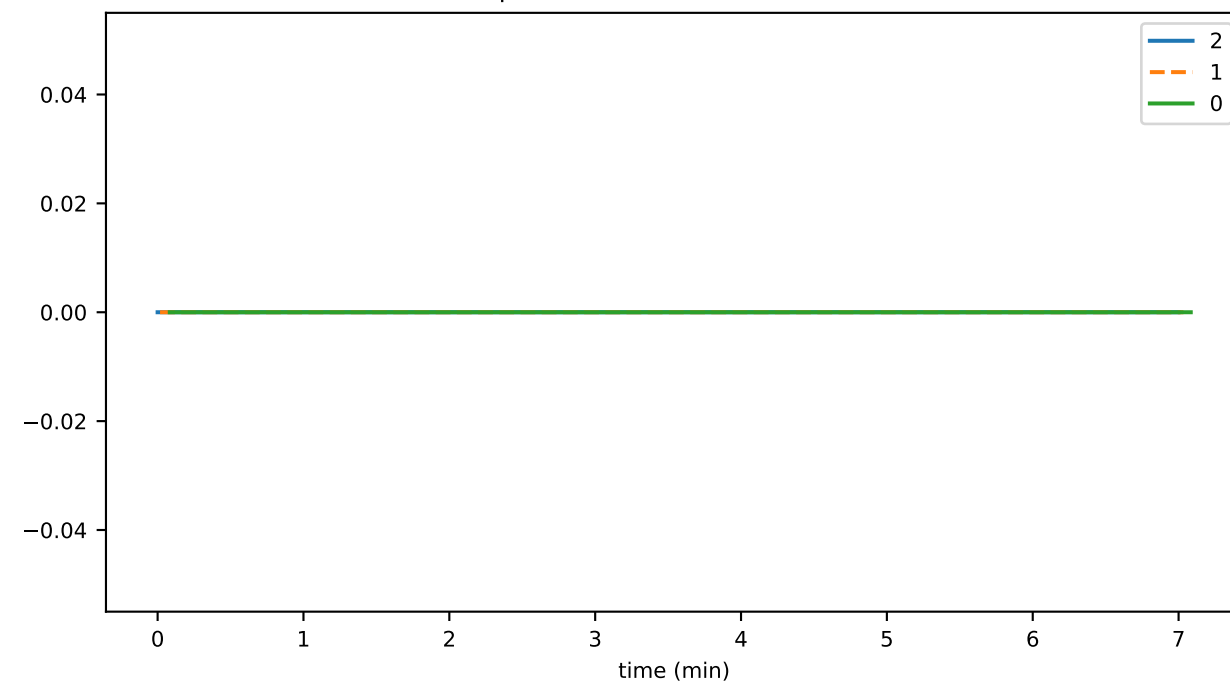
ParseErrOtherRcv
