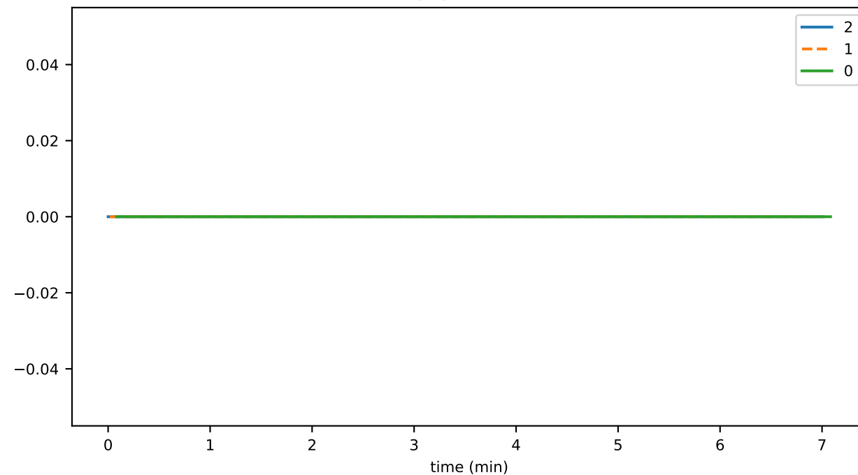
pityParent2
