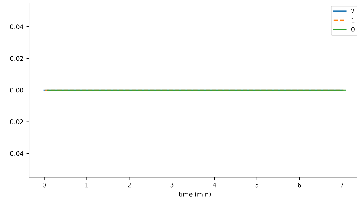
getByKeyThrottledTxns
