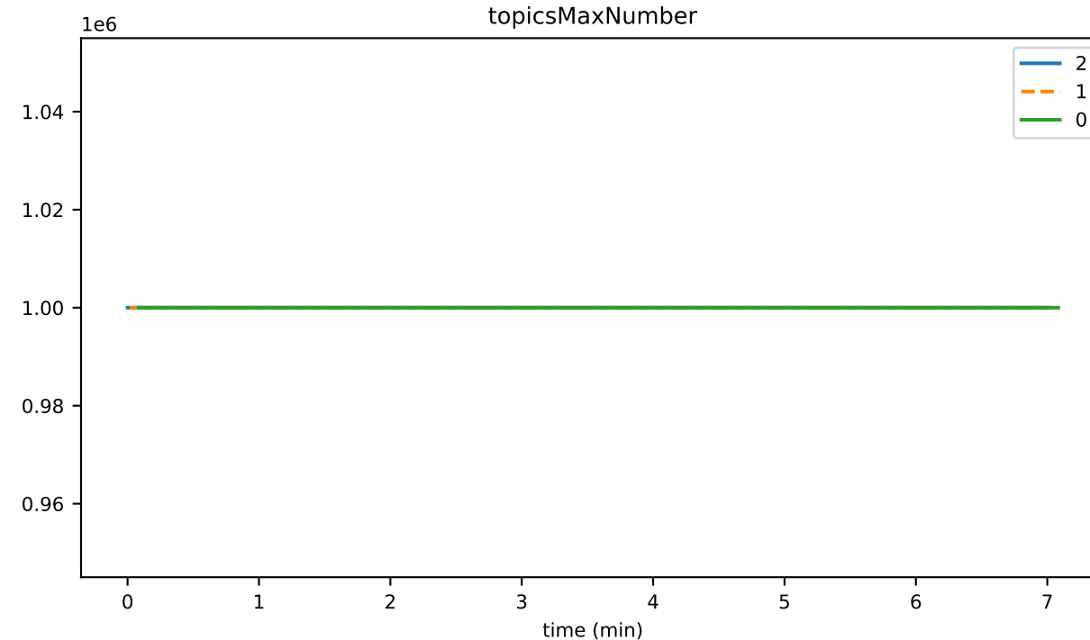
topicsMaxNumber
