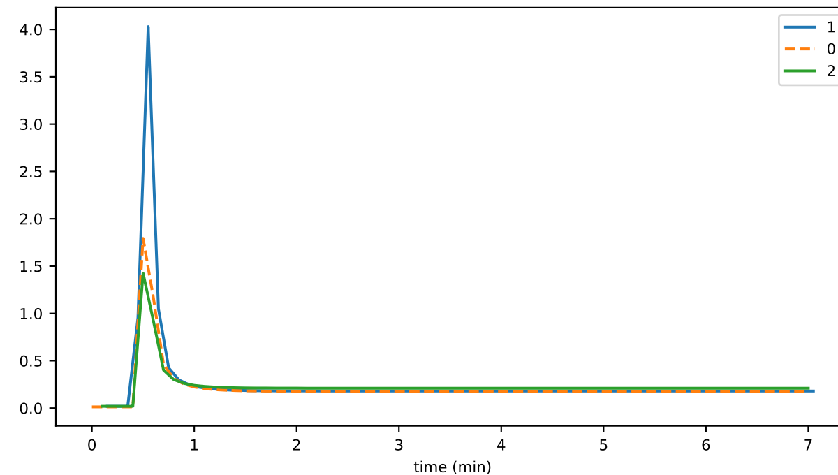
memFree (1e10)
