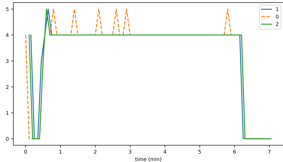
hapiBytesPercentUsed
