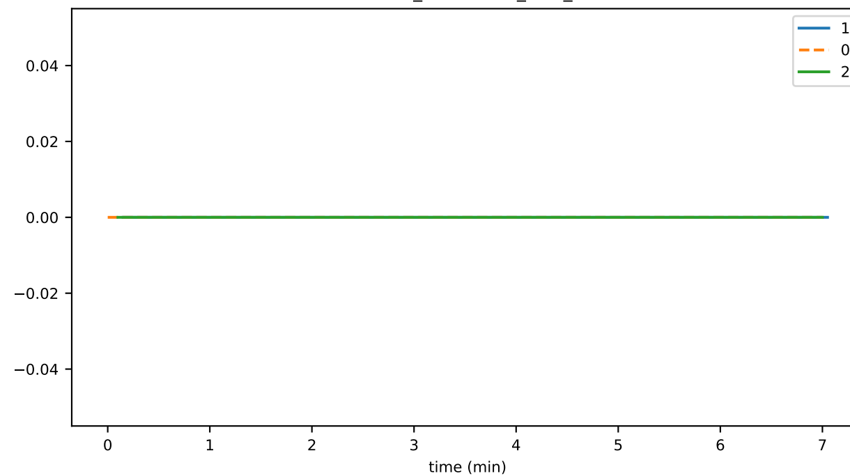
IssDetector_unhandled_task_count
