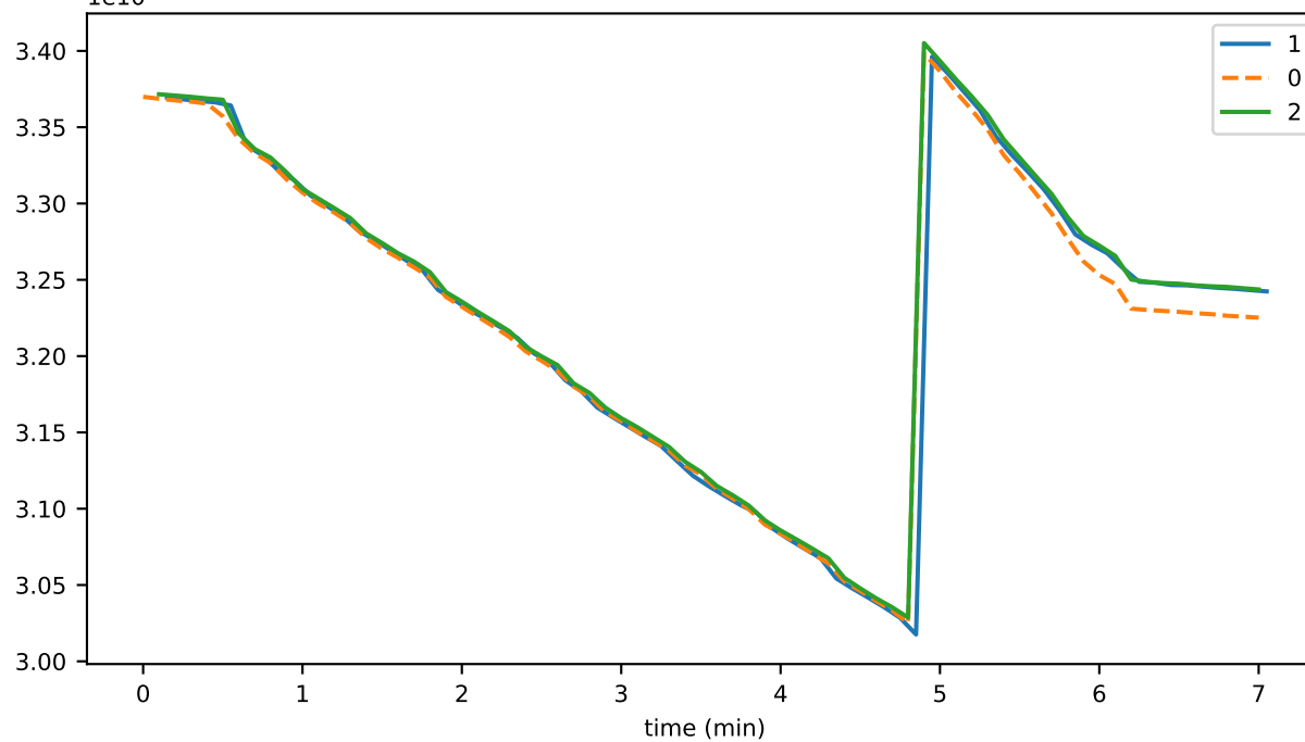
memFree (1e10)
