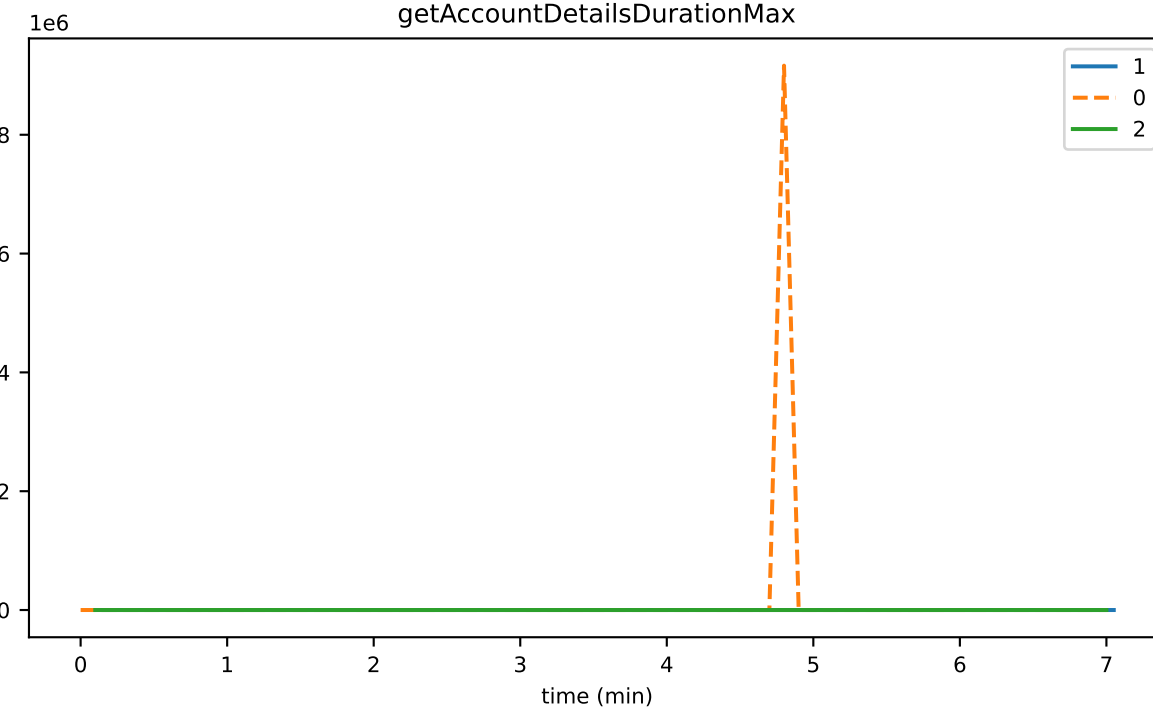
getAccountDetailsDurationMax
