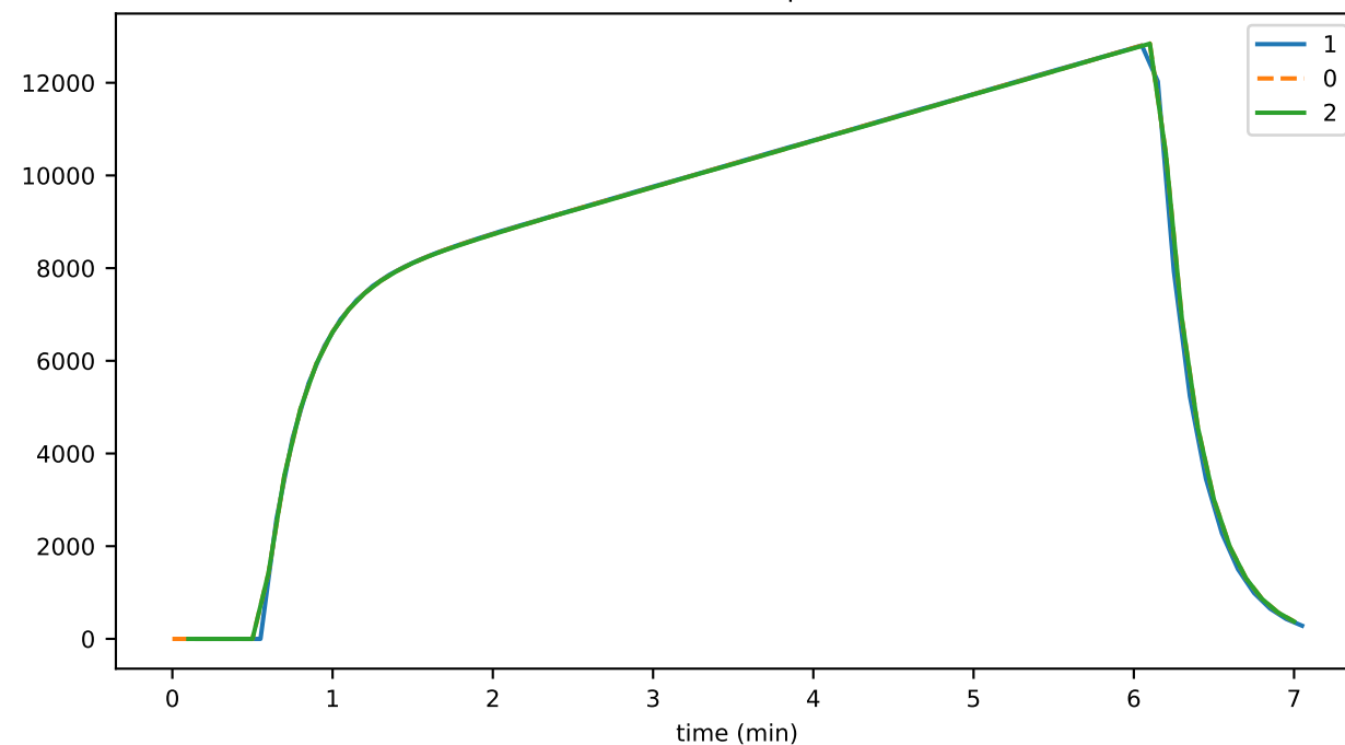
roundSup
