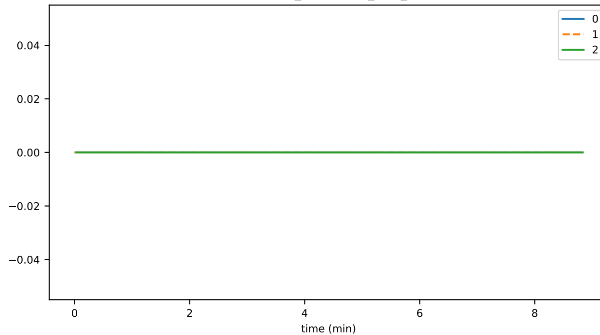
EventHasher_unhandled_task_count
