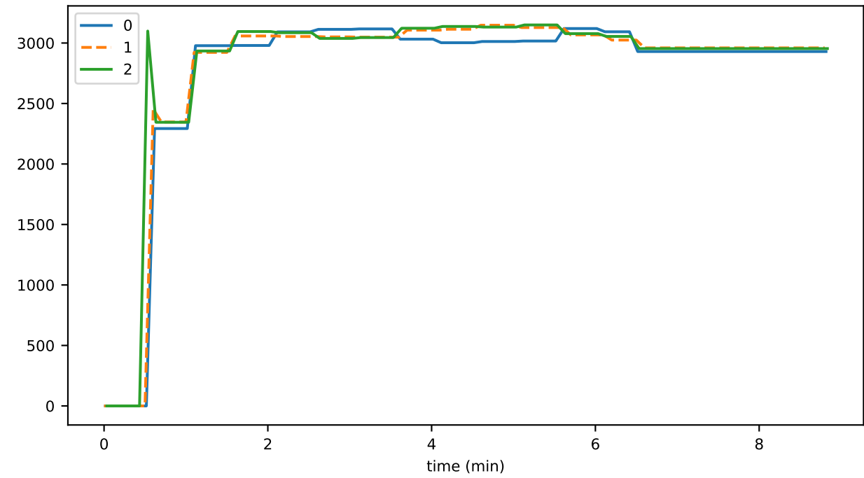
stateToDisk
