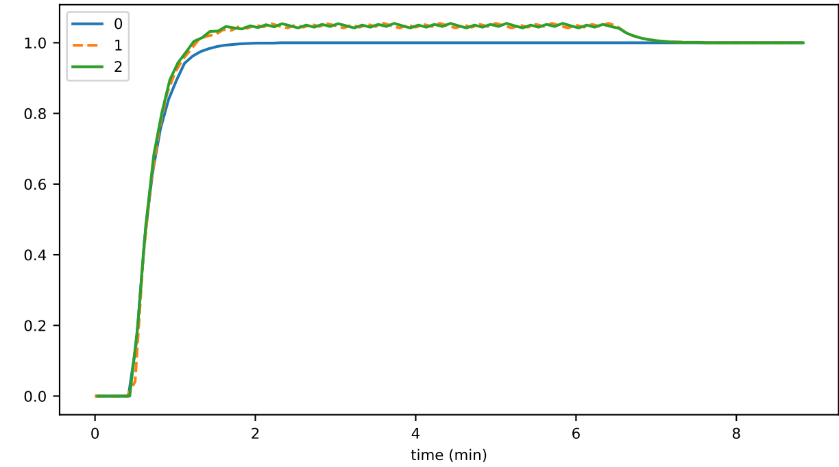
stateToDisk
