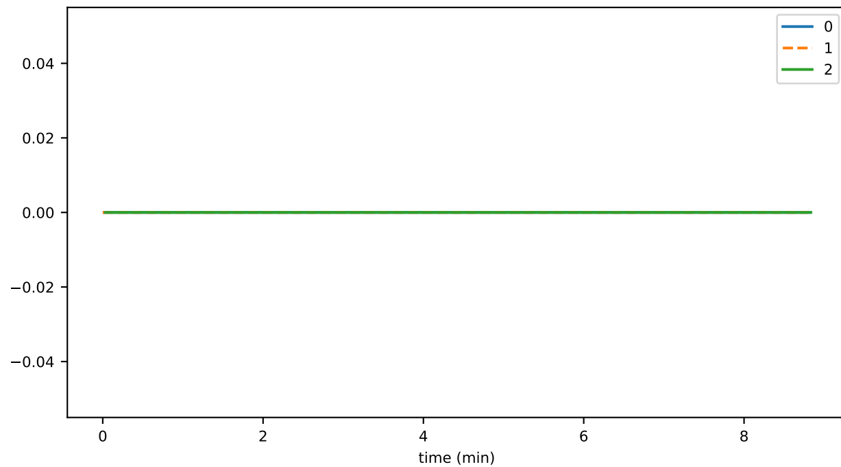
indicatorsWaitingForExpiry
