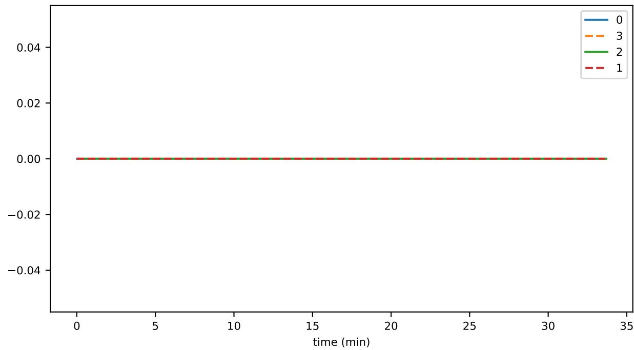
secC2R
