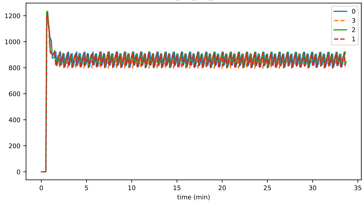
bytes_per_sec_trans
