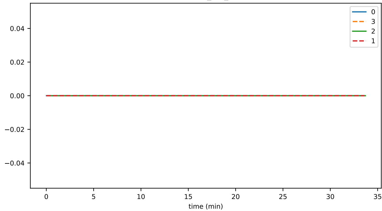
DigSpans_per_sec
