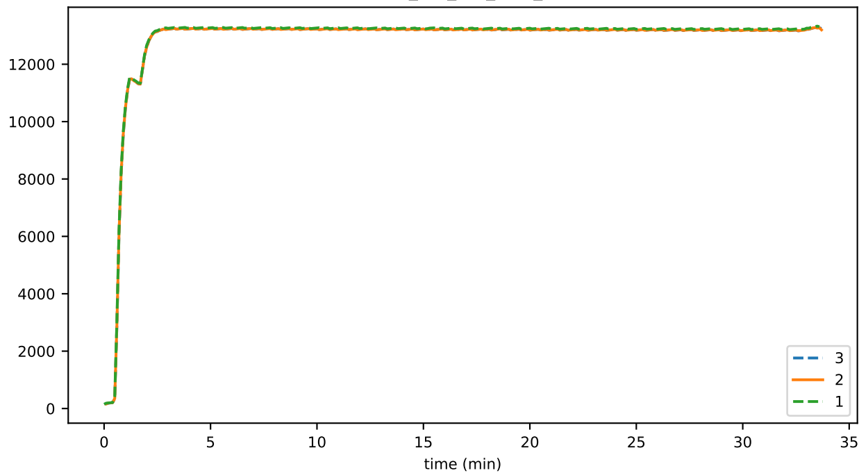
bytes_per_sec_sent_00
