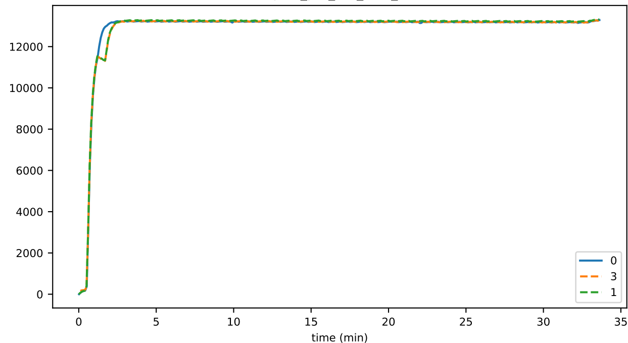
bytes_per_sec_trans
