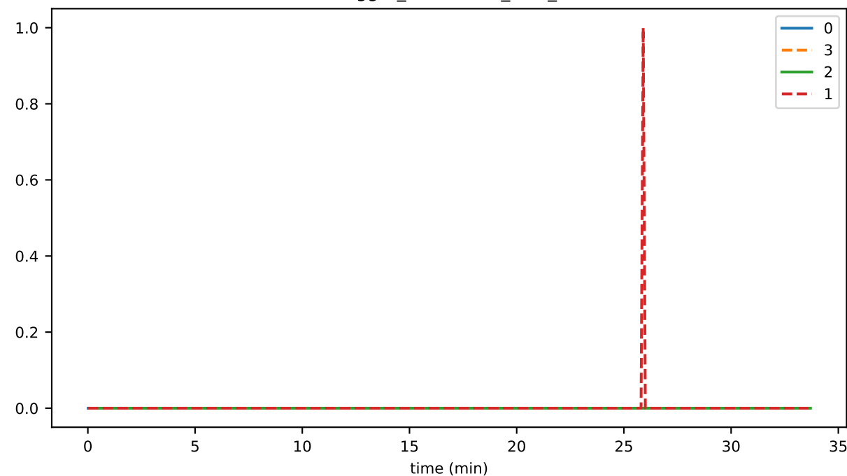
HashLogger_unhandled_task_count
