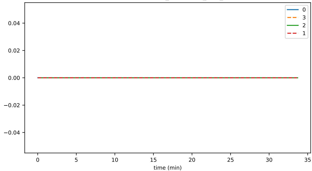
TransactionPrehandler_unhandled_task_count
