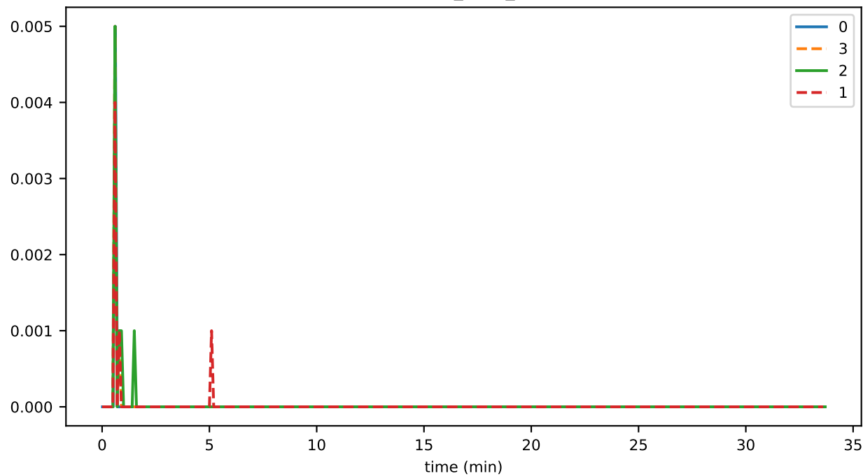
StateHasher_busy_fraction
