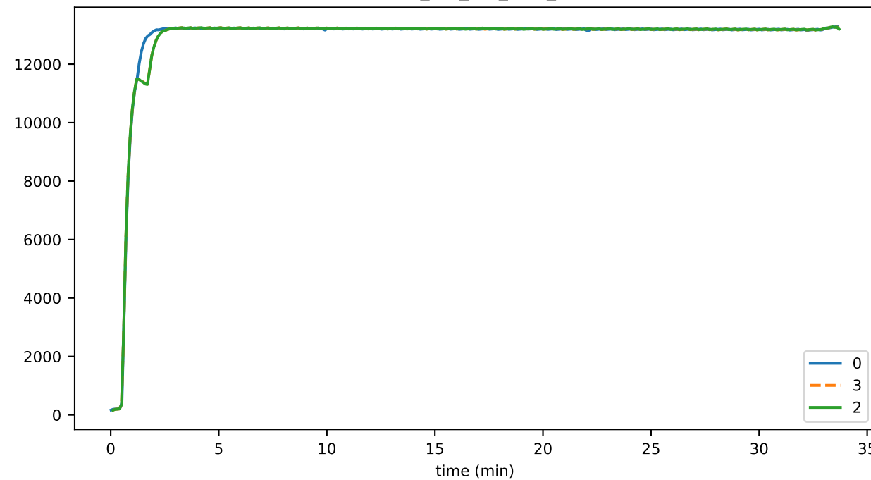
bytes_per_sec_sent_01
