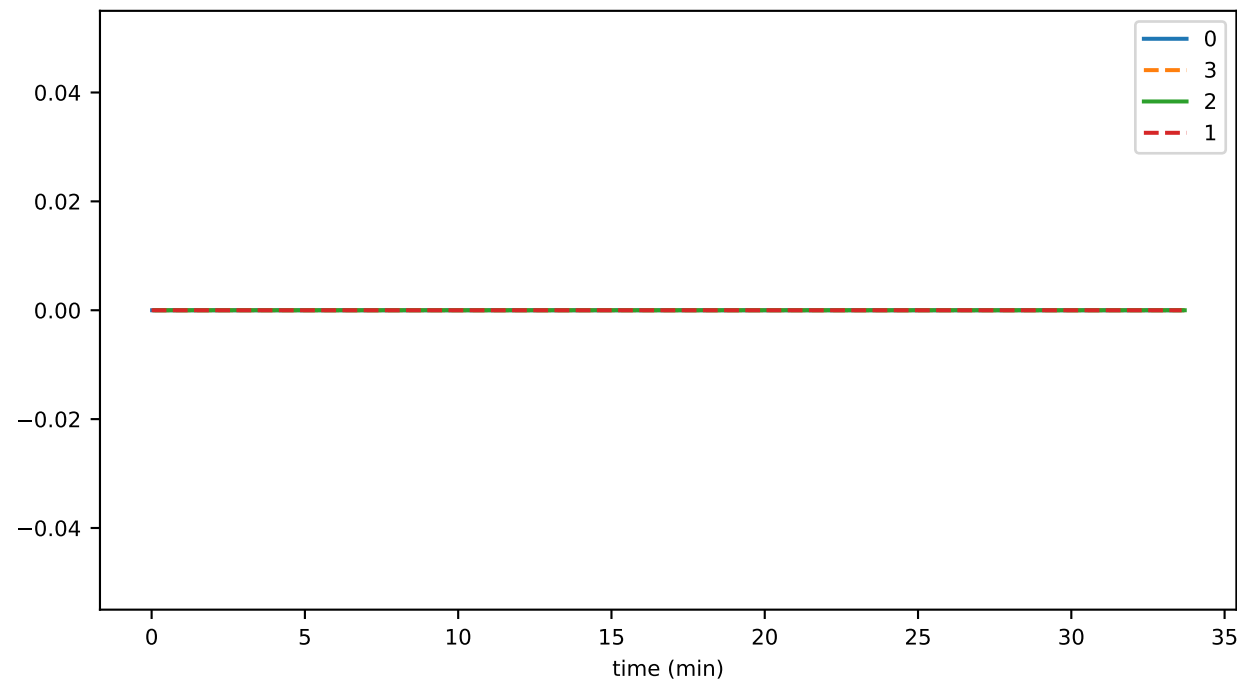
secC2RC
