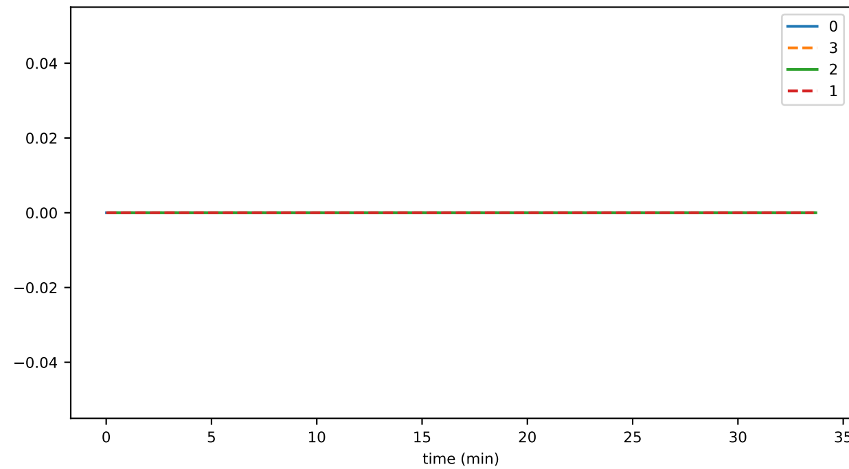
DigSubWrkItmTime
