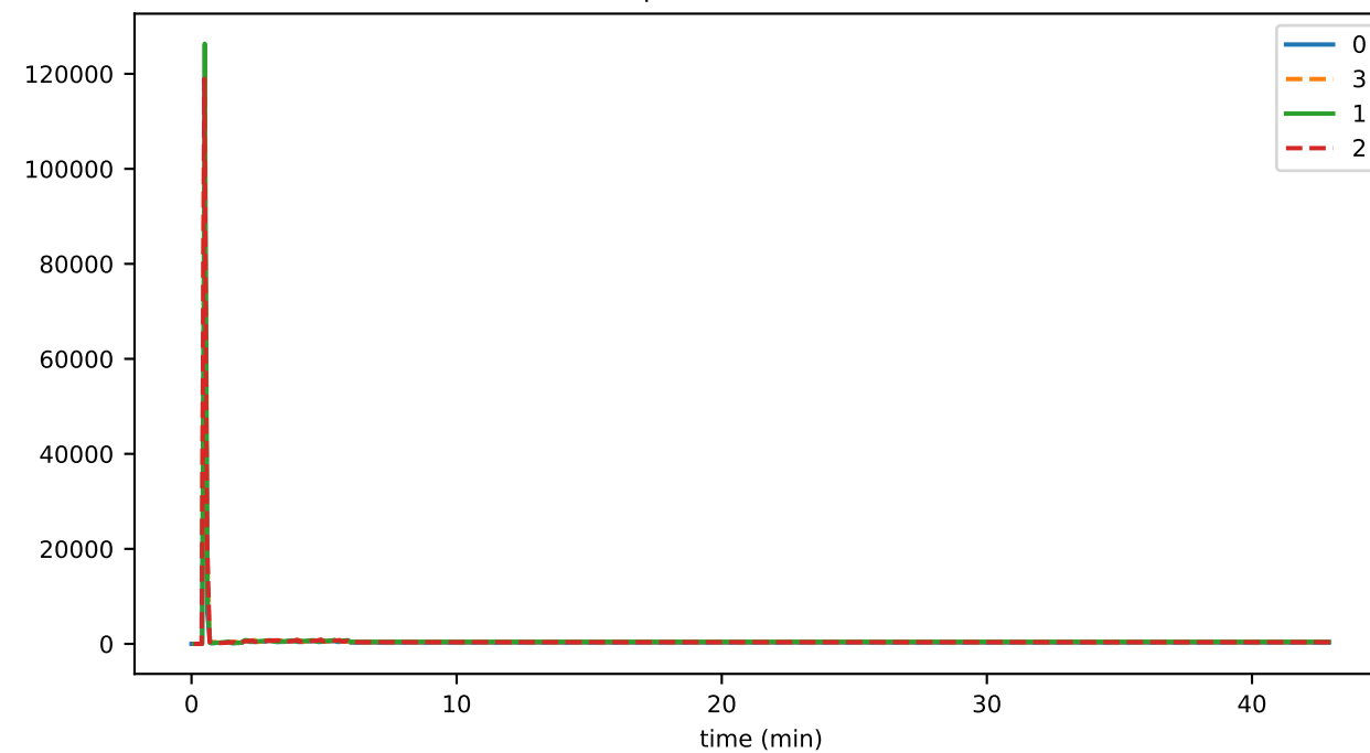
preHandleMicros
