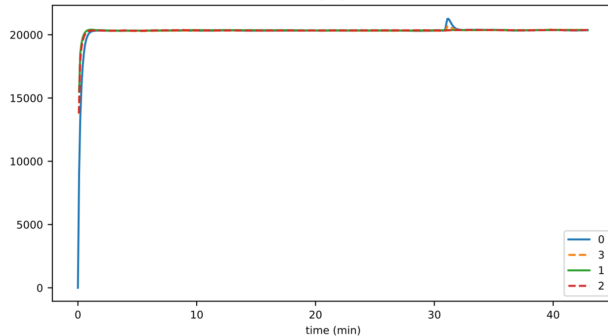
ping_us_00MIN
