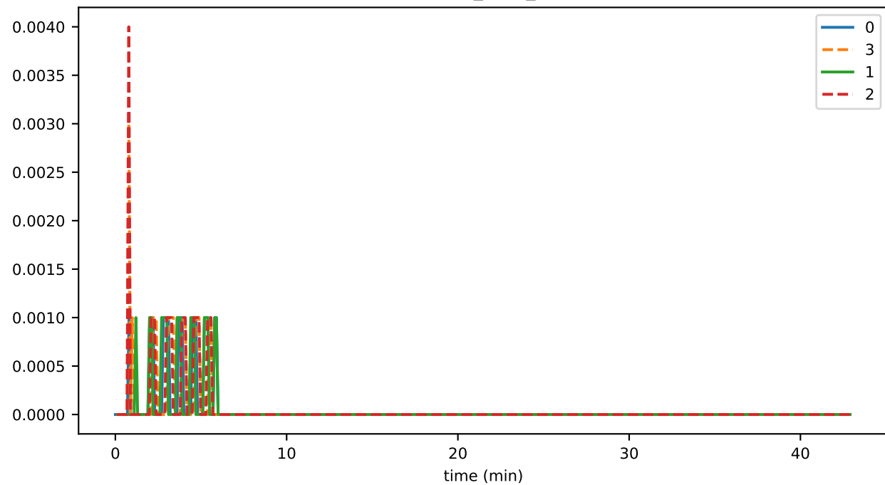
StateHasher_busy_fraction
