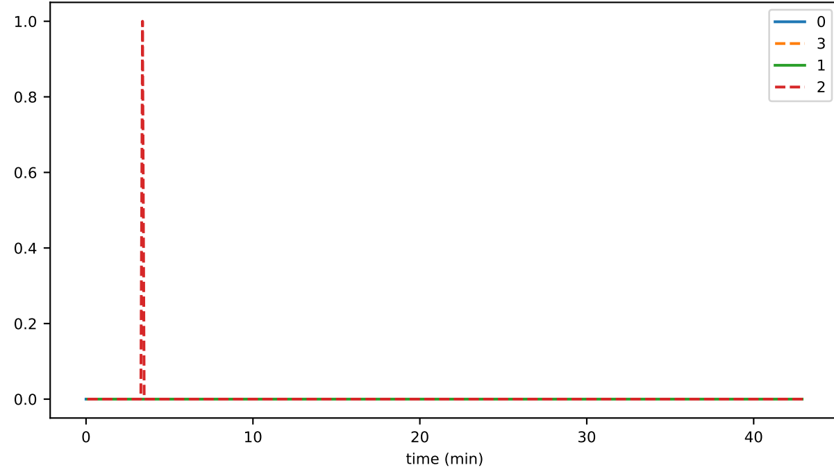
PlatformMonitor_unhandled_task_count
