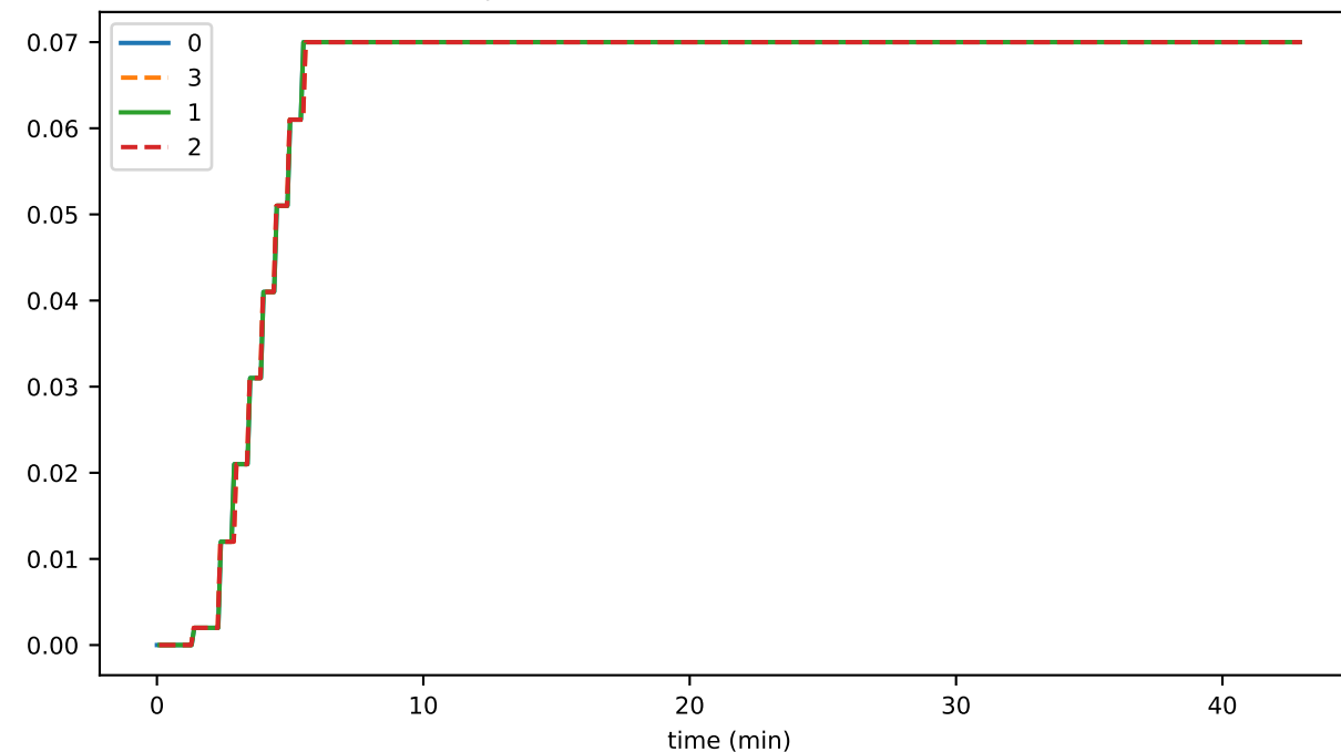
preHandleMicros
