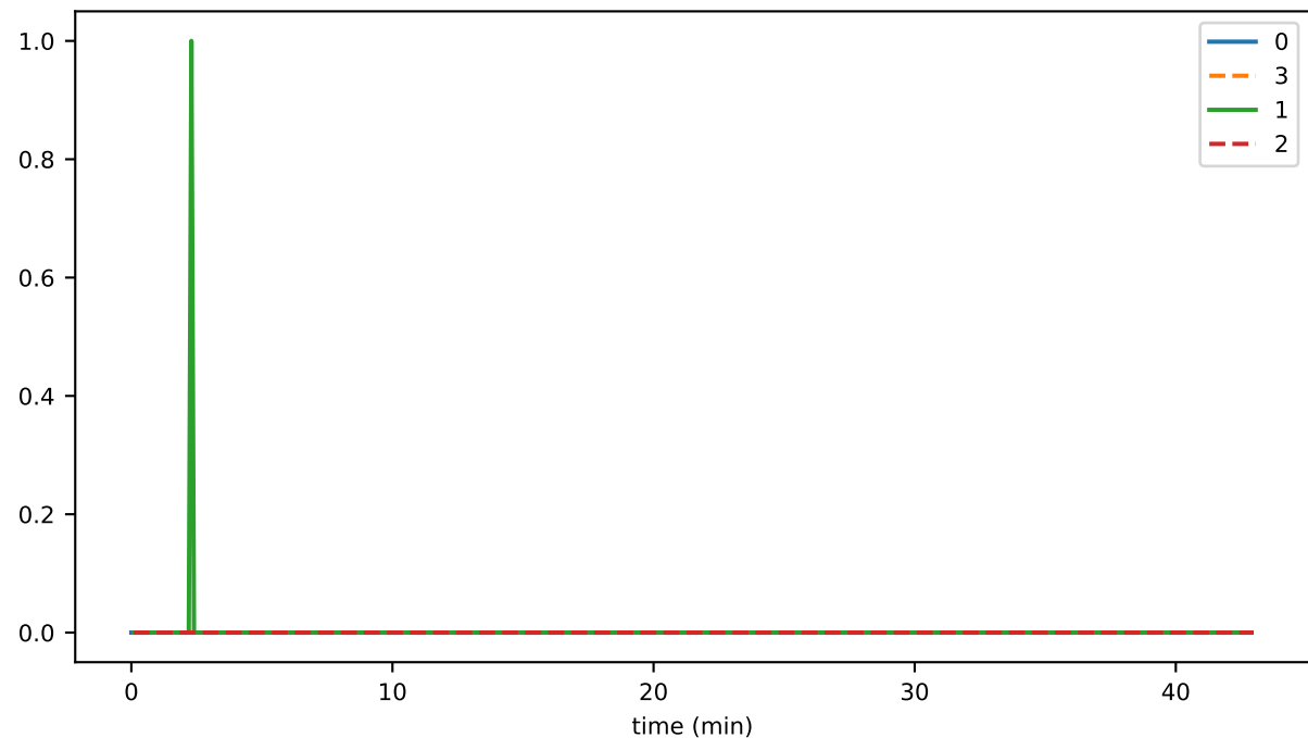
syncRoundLag
