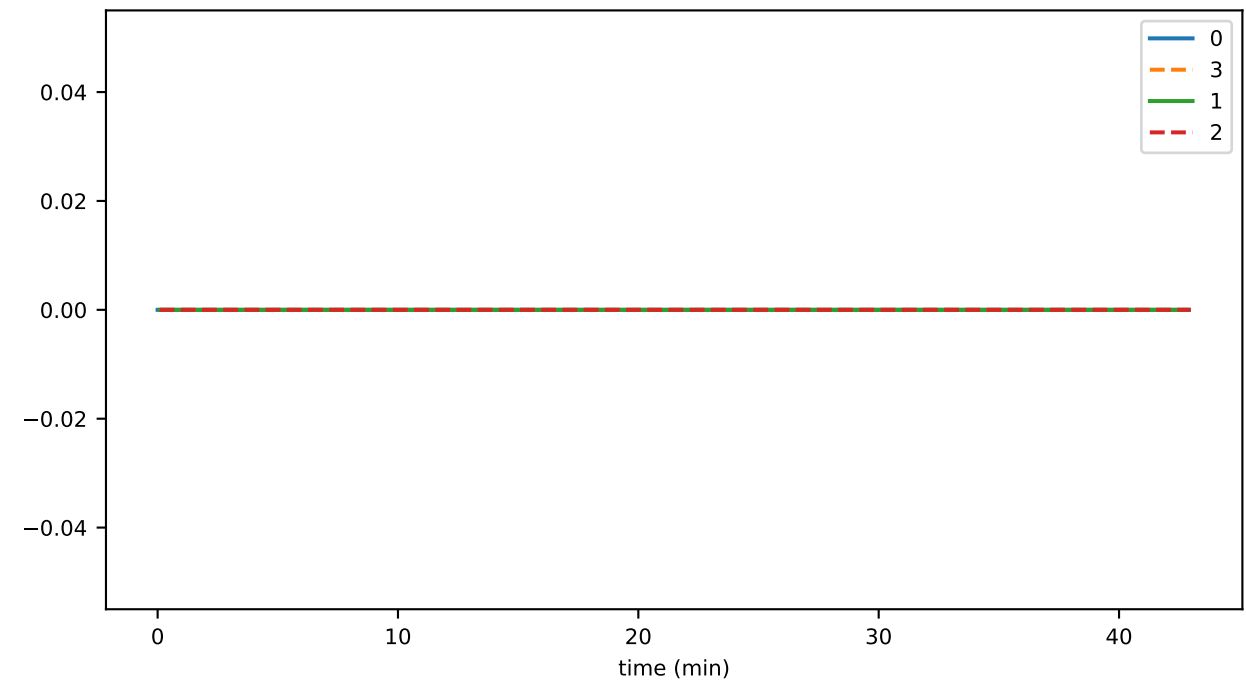
contractsUsed
