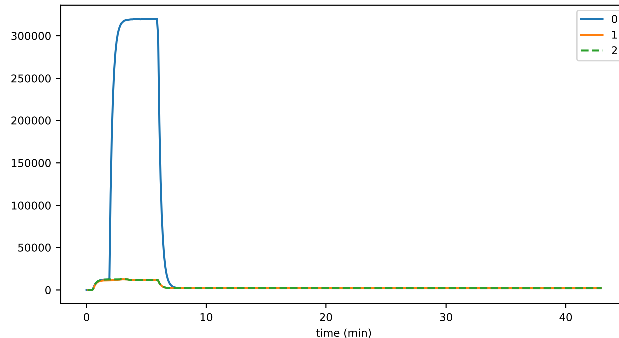
bytes_per_trans
