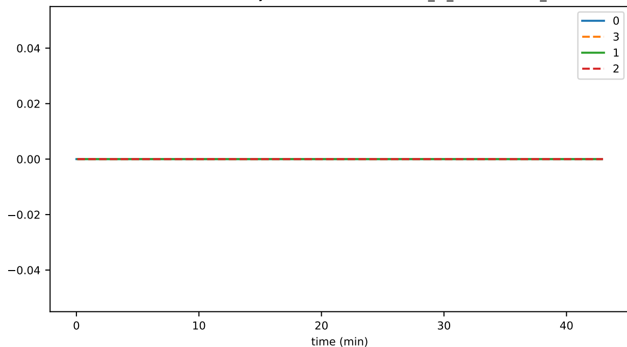
SmartContractService:SystemContractMethodCall_KYC_total
