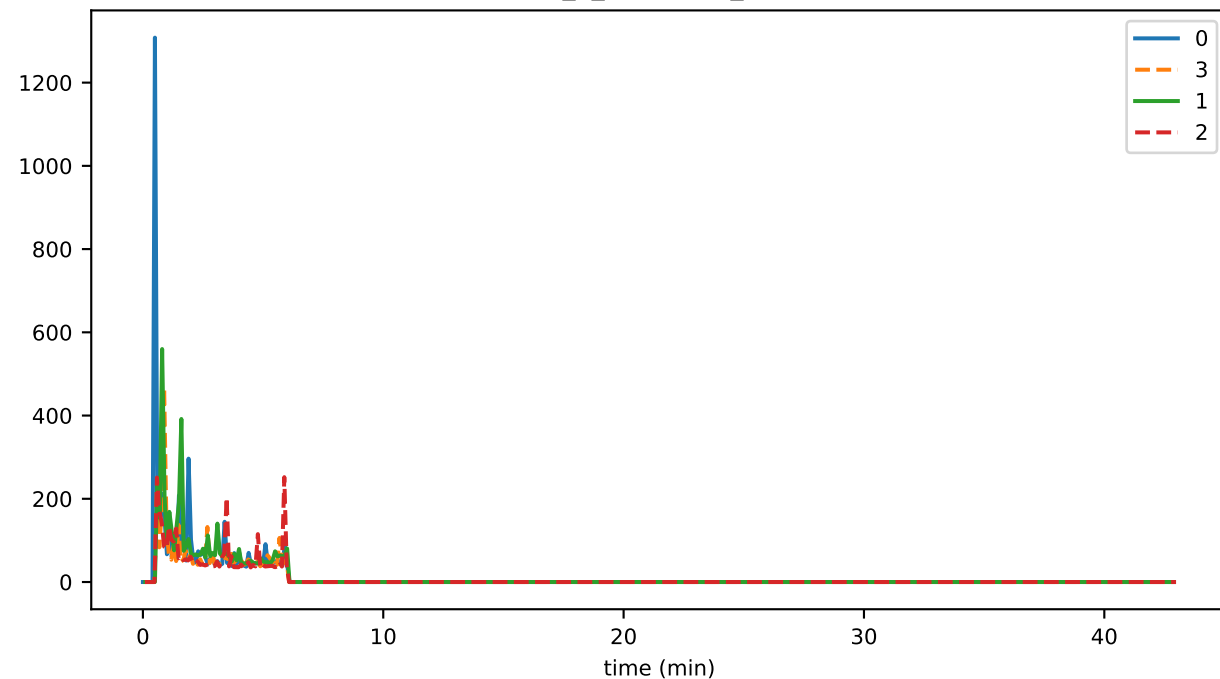
eventDelay_2_validation_runtimeMAX
