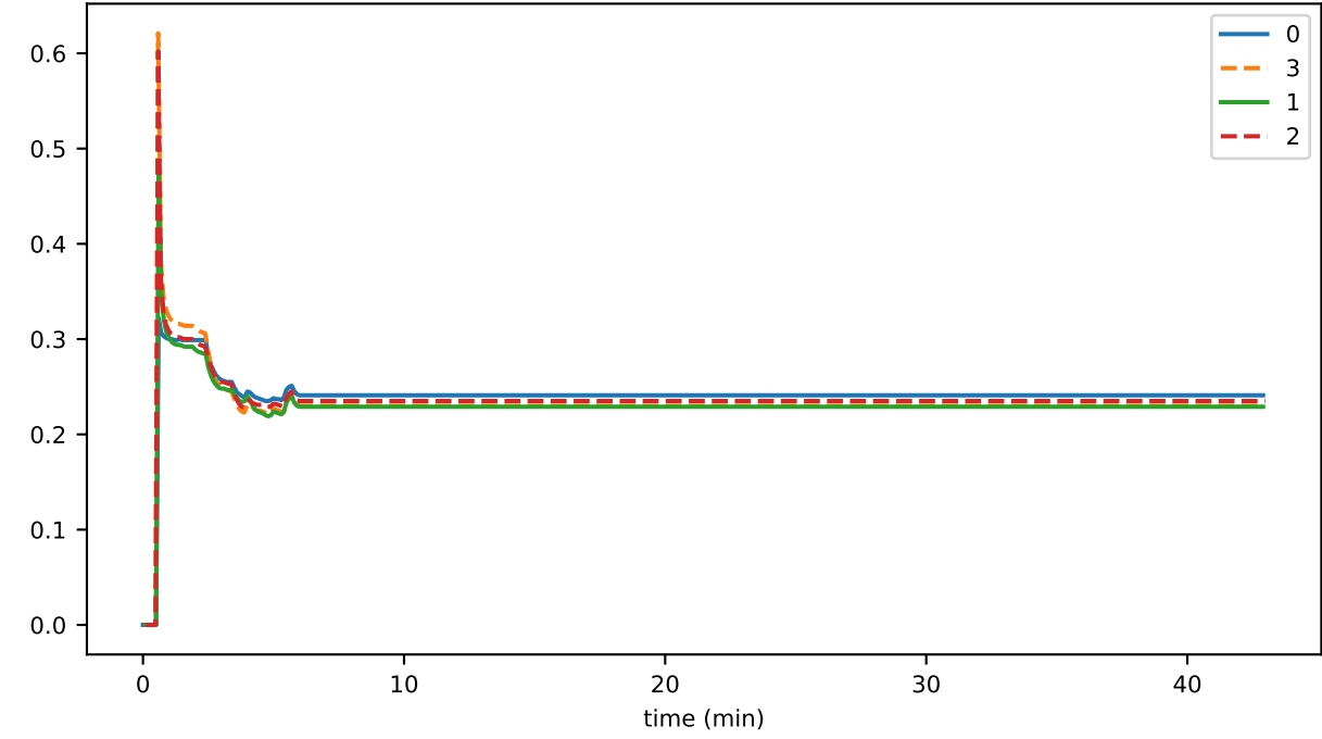
secC2RC
