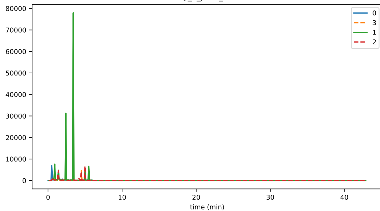
eventDelay_6_pces_runtimeMAX
