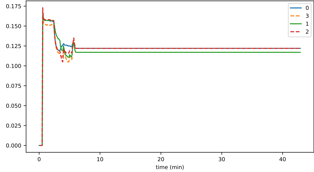
secR2F
