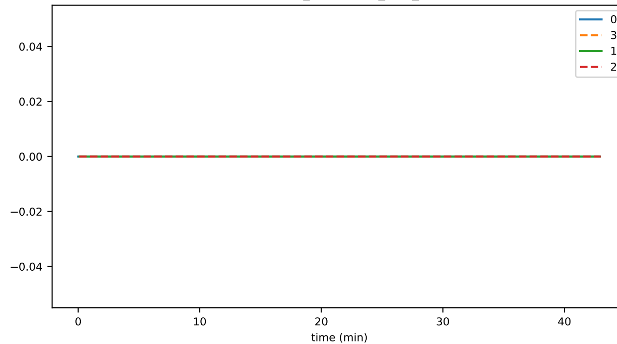
StateHasher_unhandled_task_count
