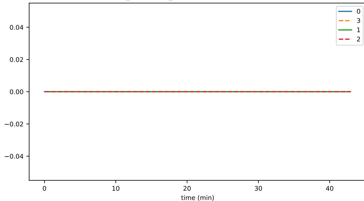
conn_connClose_tooManyEndStreamResponses
