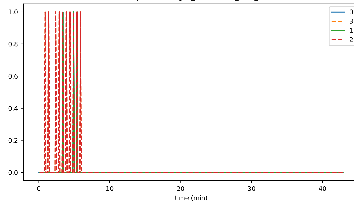
storageSlotsMaxNumber
