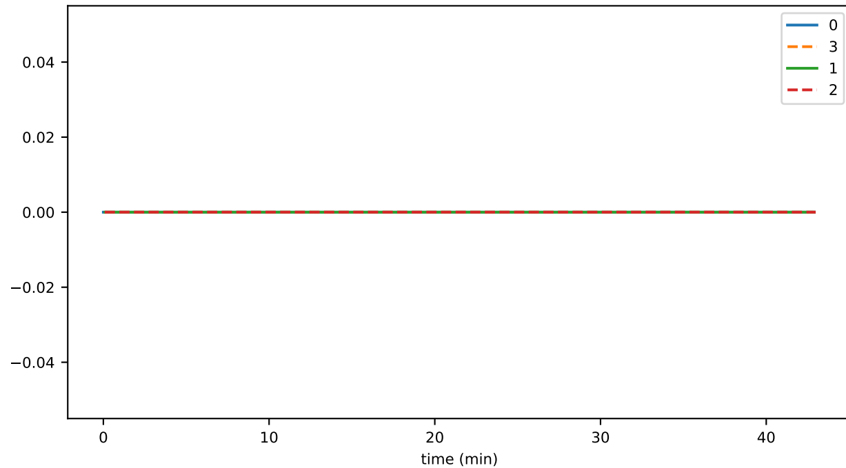
SmartContractService:SystemContractMethodCall_TOKEN_QUERY_total
