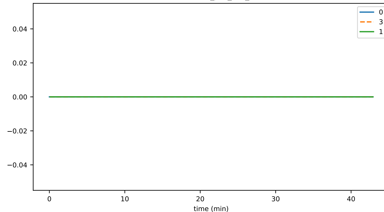
DiskspaceFree
