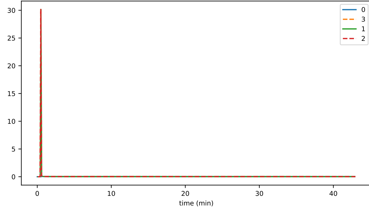
secC2R
