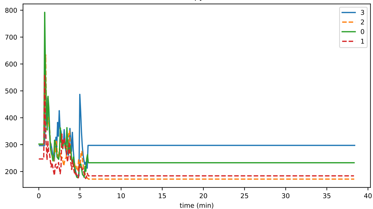
StateHasher_busy_fraction
