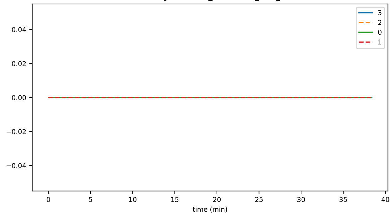
StateHasher_unhandled_task_count
