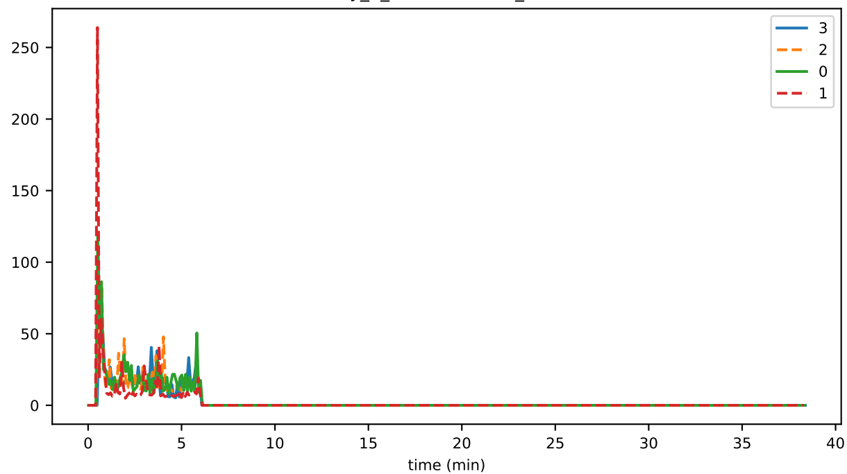
eventDelay_1_eventCreation_runtimeMAX
