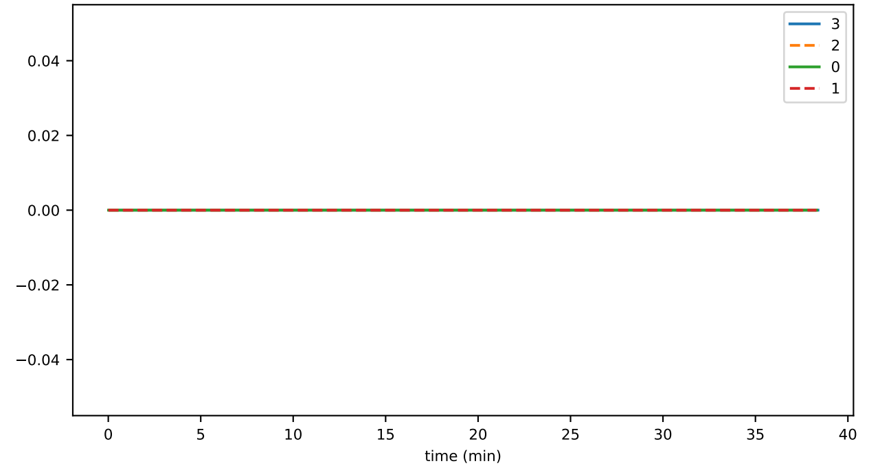
HashLogger_unhandled_task_count
