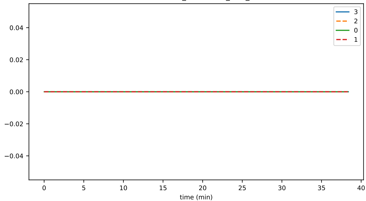
InlinePcesWriter_unhandled_task_count
