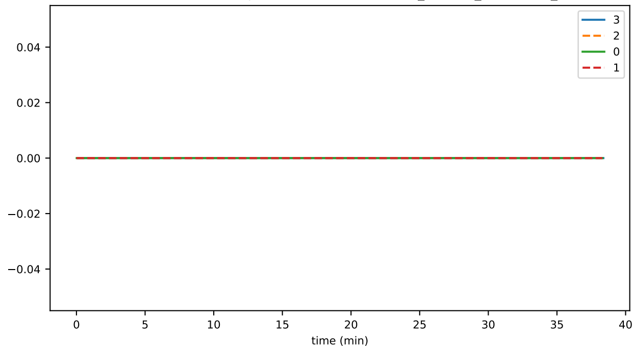
SmartContractService:SystemContractMethodCall_HAS_total
