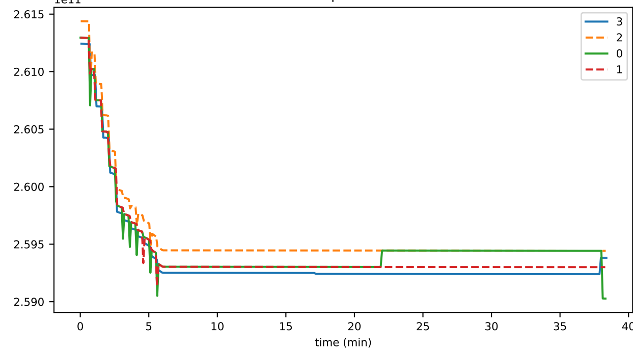
DiskspaceFree
