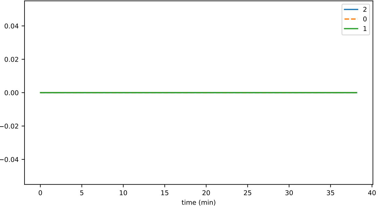
SmartContractService:SystemContractMethodCall_KYC_total
