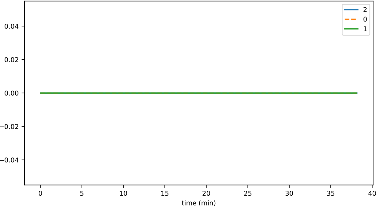
SmartContractService:SystemContractMethodCall_HTS_total
