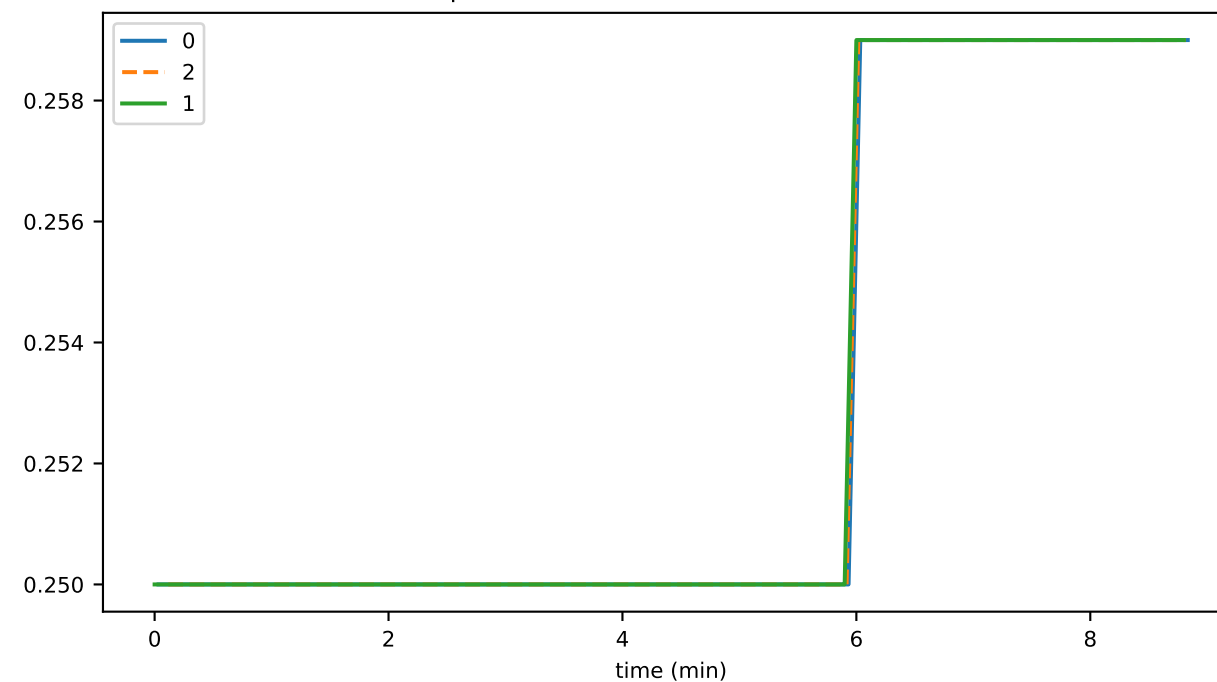
preHandleMicros
