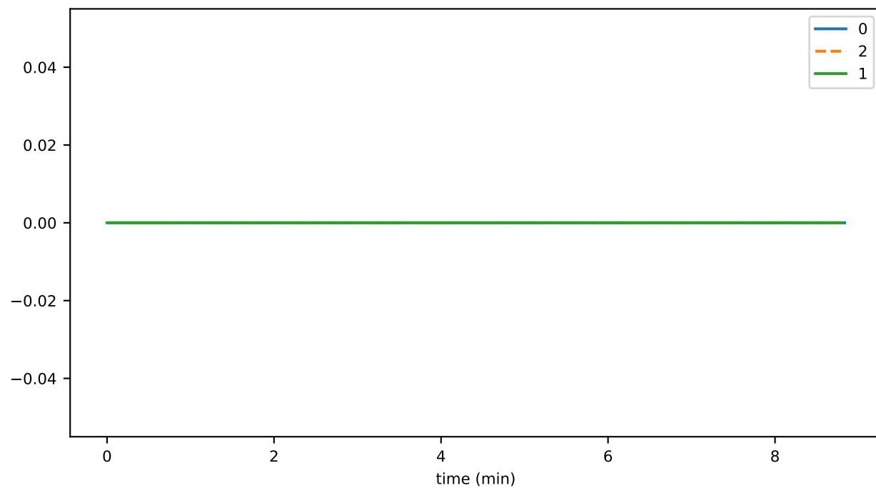
nodeCreateThrottledTxns
