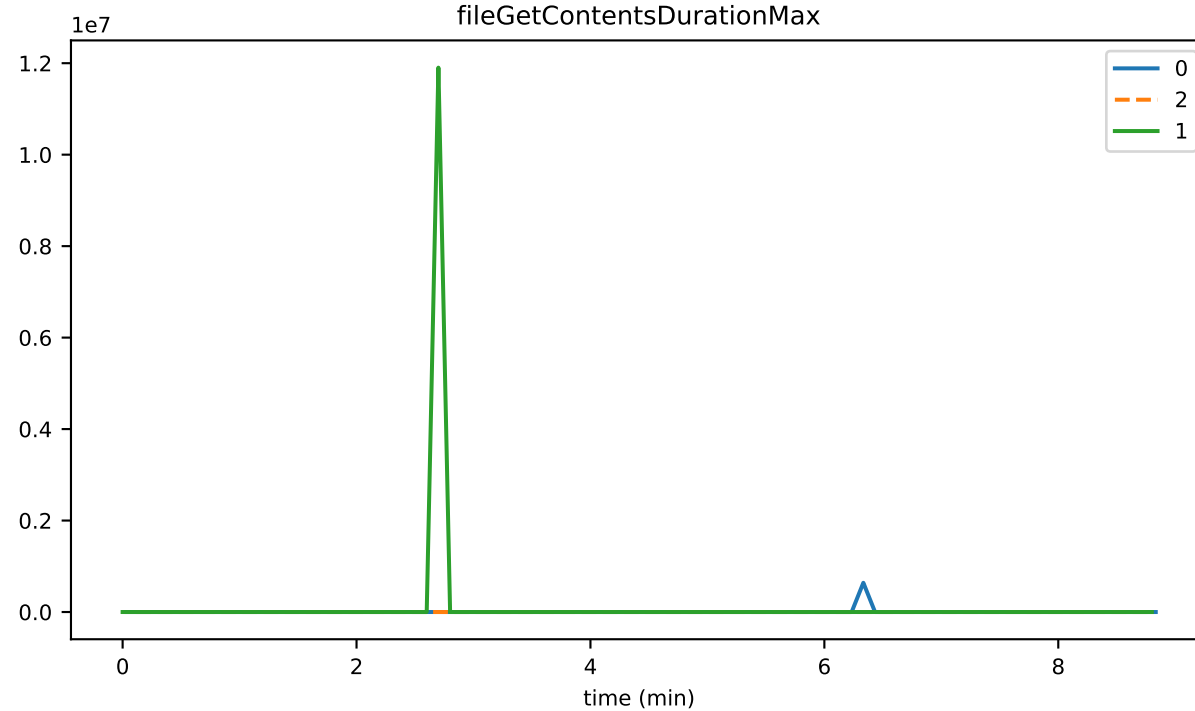
fileGetContentsDurationMax
