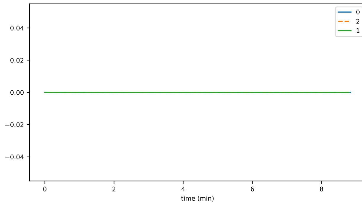
secC2RC
