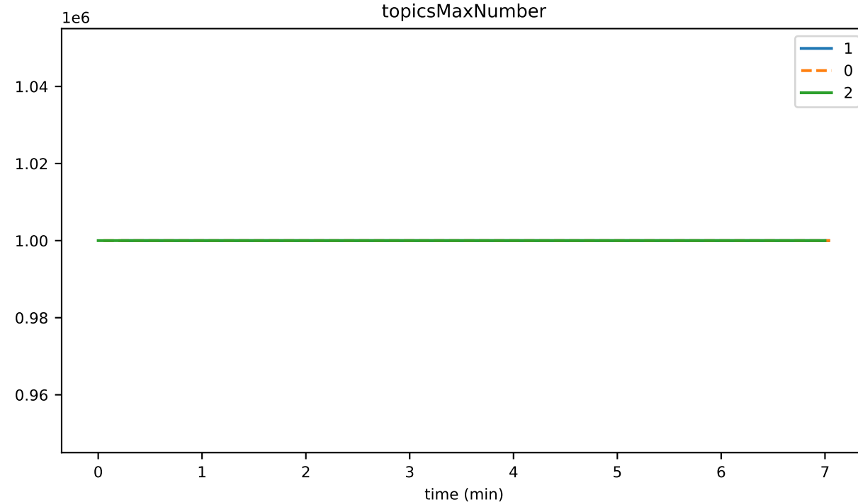
topicsMaxNumber
