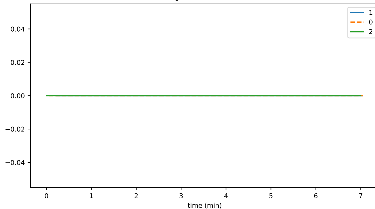
getAccountDetailsDurationMax
