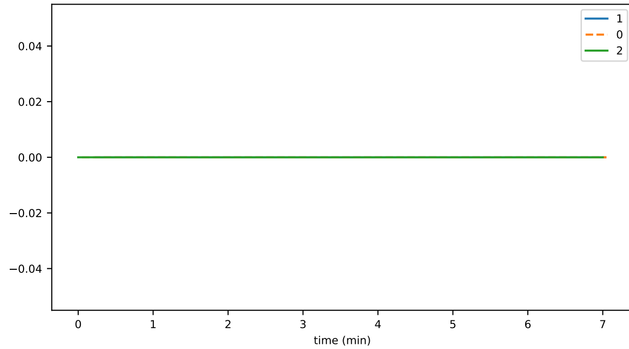
cryptoGetInfoThrottledTxns
