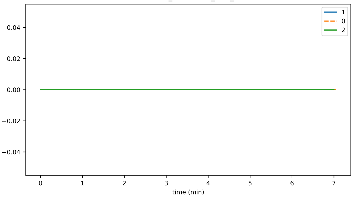
EventHasher_unhandled_task_count
