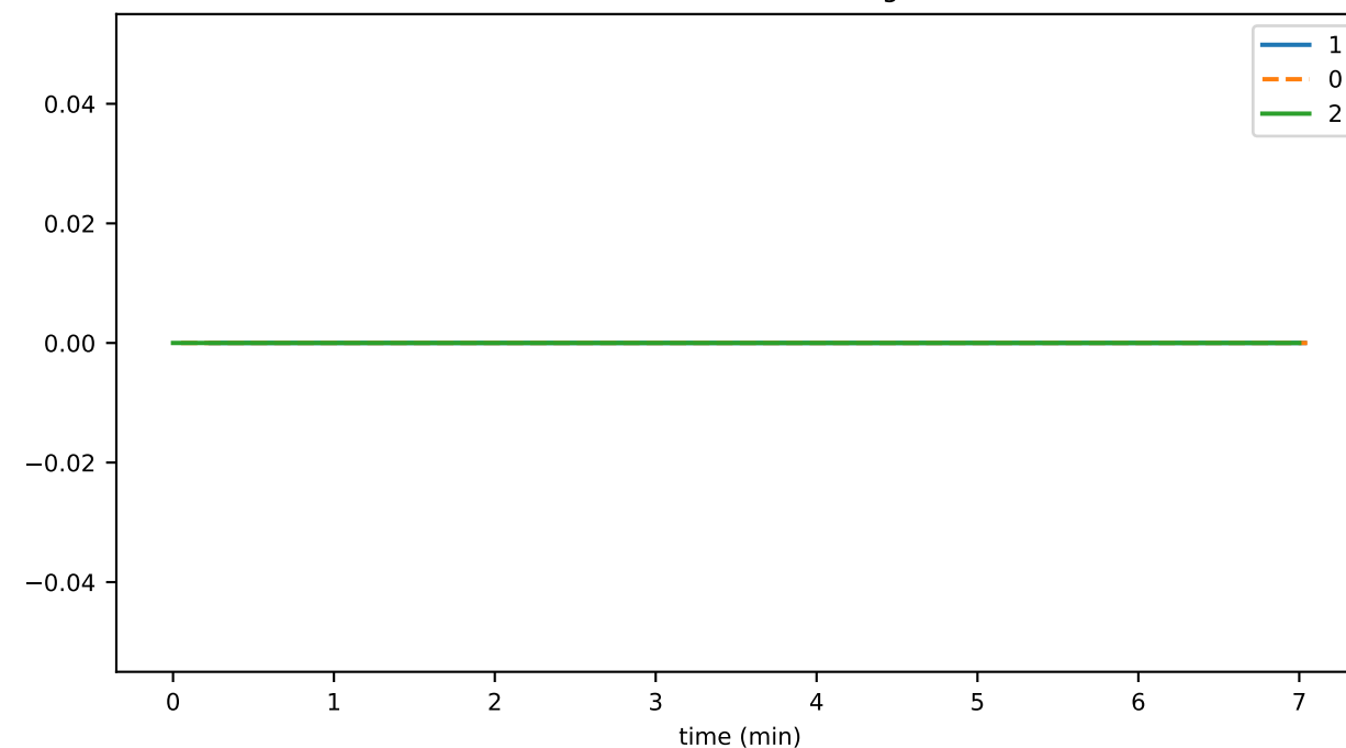
tokenBurnThrottledTxns
