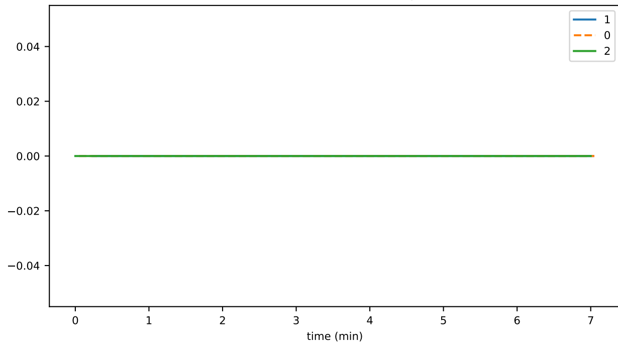
tokenGetInfoThrottledTxns
