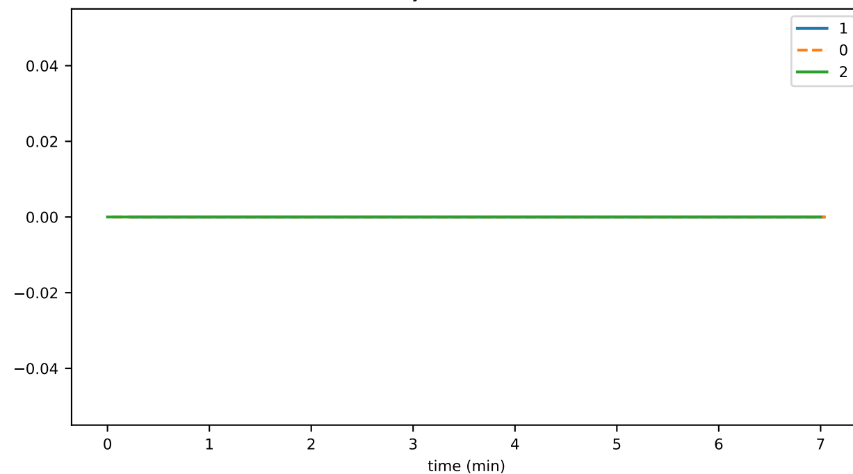
historyProofTransAggToDoneCnt
