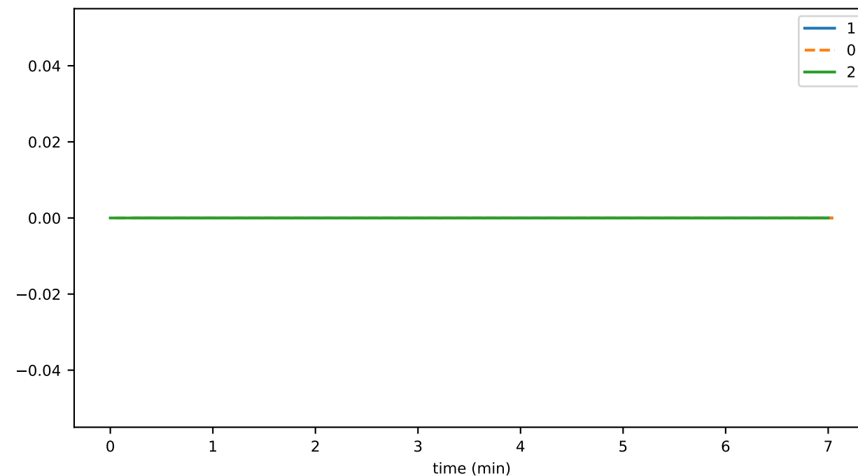
nodeDeleteThrottledTxns
