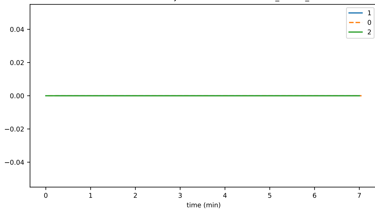
SmartContractService:SystemContractMethodCall_PROXY_total
