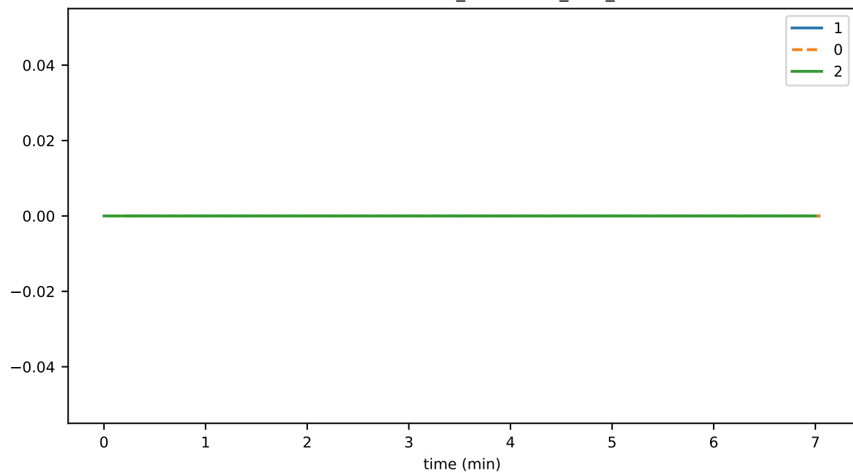
TransactionPrehandler_unhandled_task_count
