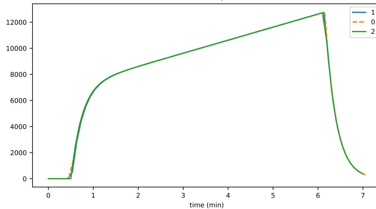
roundSup
