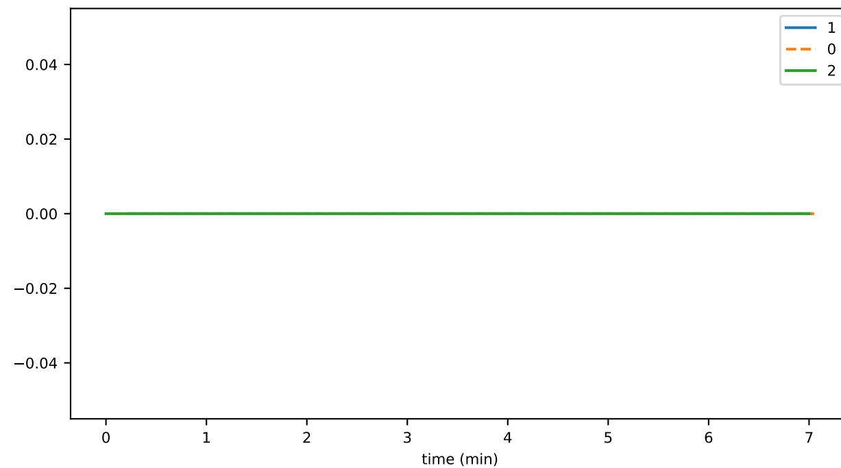
transactionGetRecordThrottledTxns
