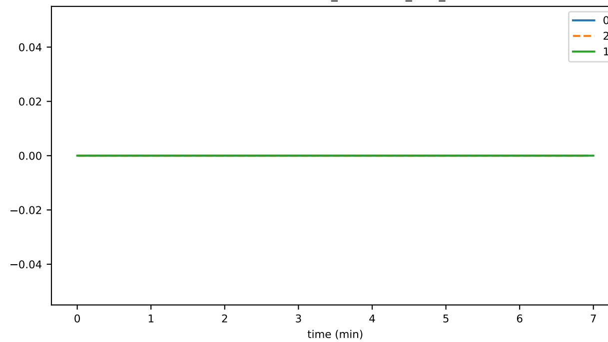
IssDetector_unhandled_task_count
