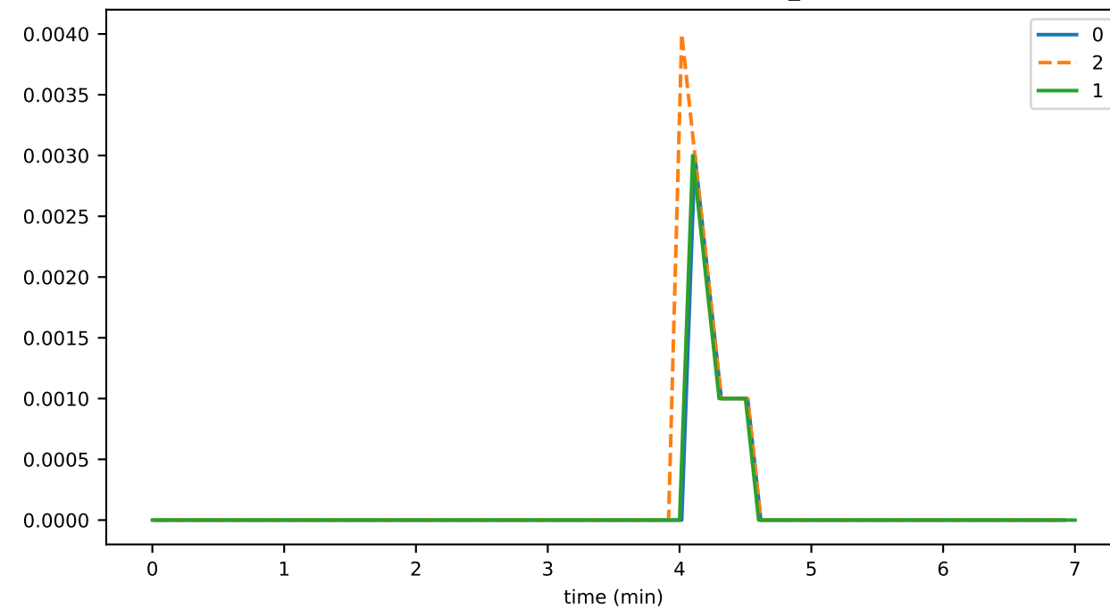
roundSup
