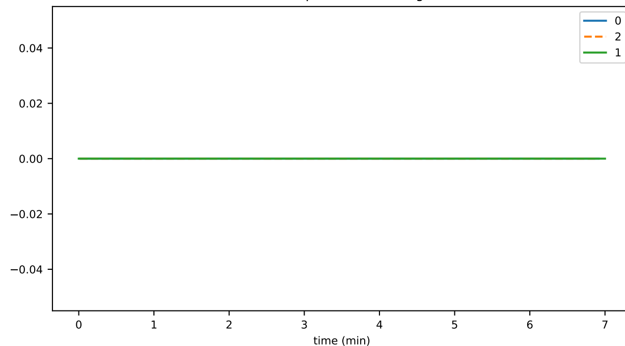
tokenUpdateNftsDurationAvg
