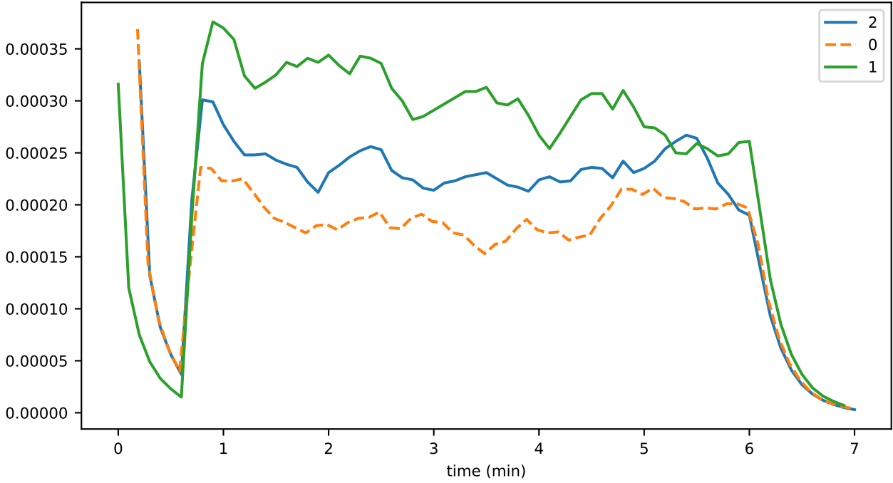
timeFracDot
