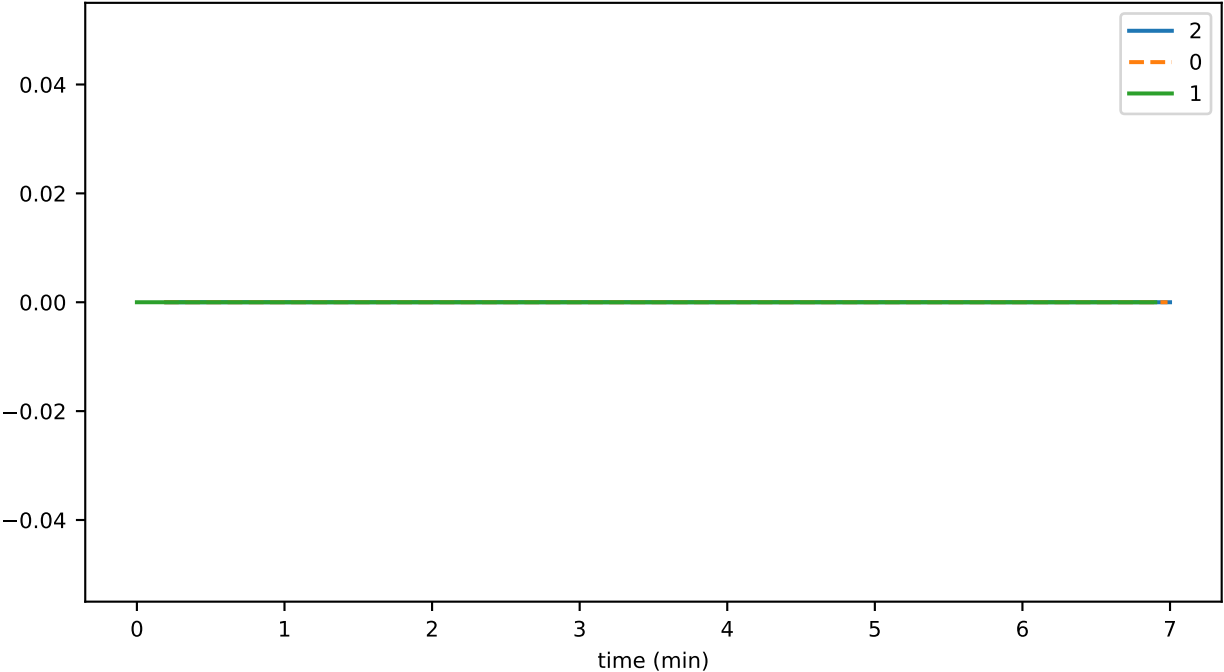
SmartContractService:SystemContractMethodCall_PROXY_total
