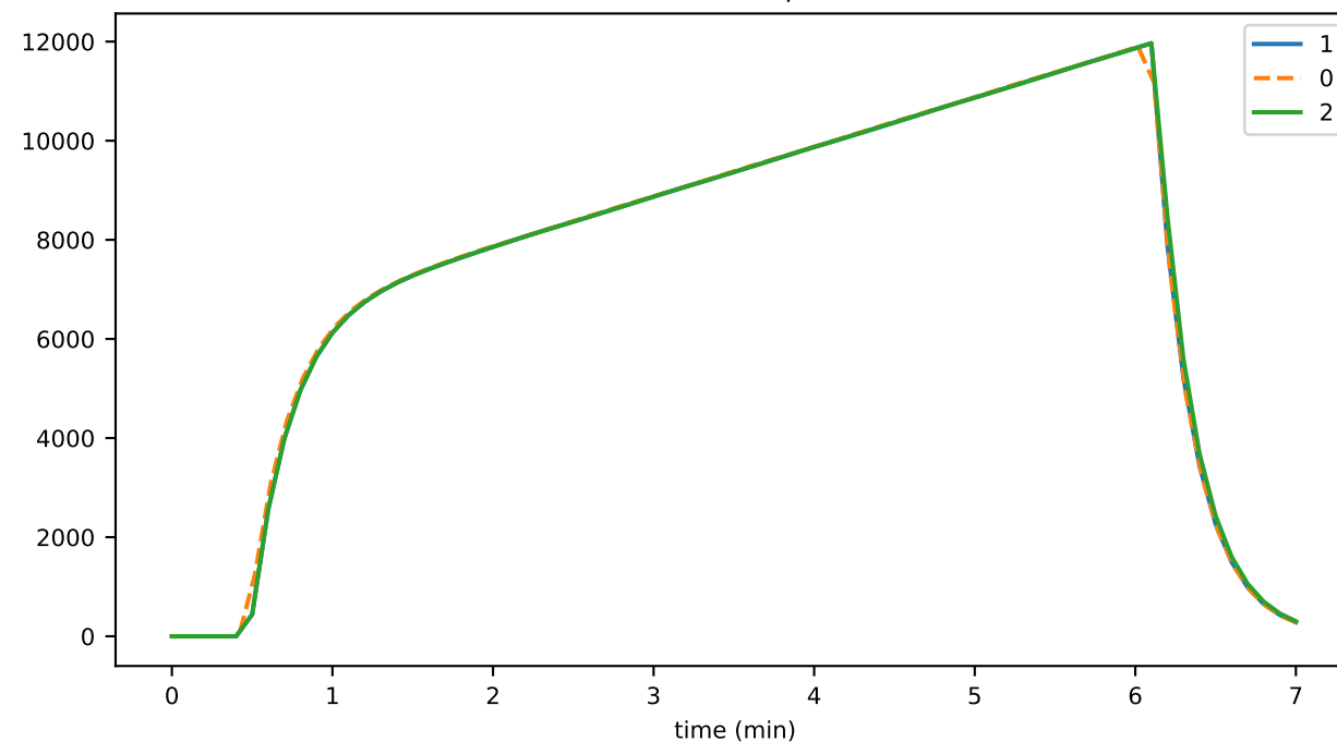
roundSup
