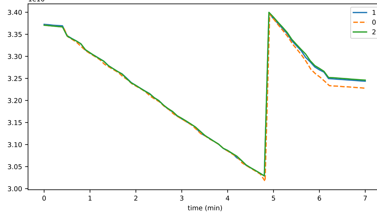
1e10 memFree
