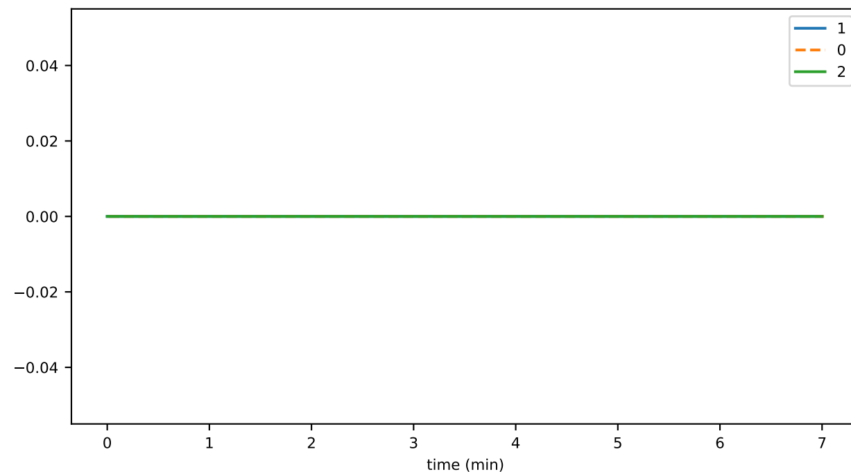
fileGetContentsDurationMax
