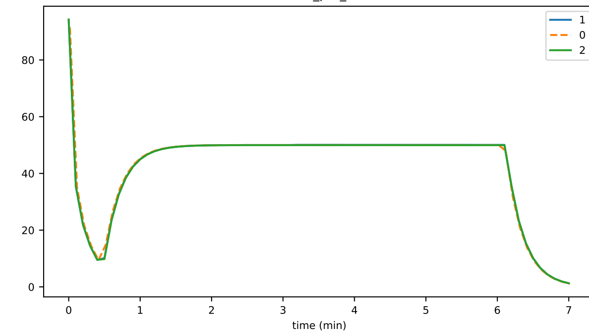
EventSignatureValidator_unhandled_task_count
