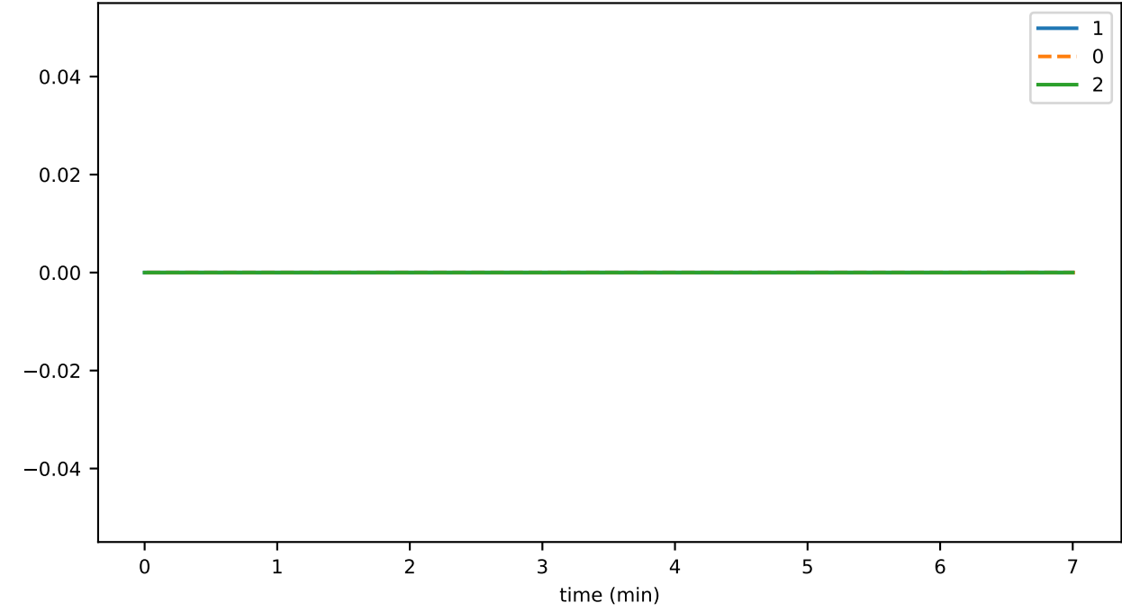
tokenGrantKycToAccountThrottledTxns
