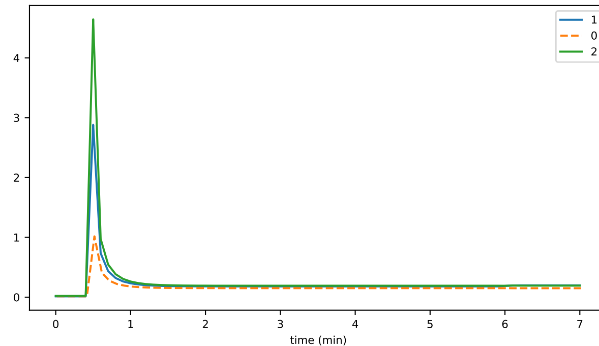
1e10 memFree
