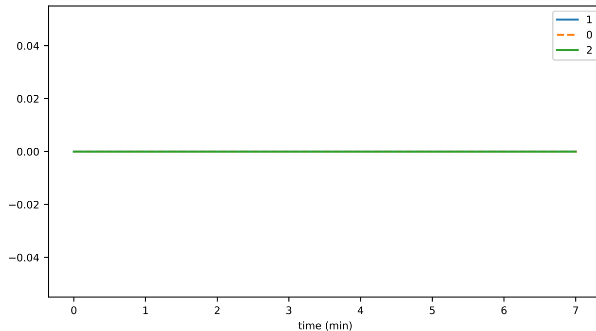
contractCallThrottledTxns
