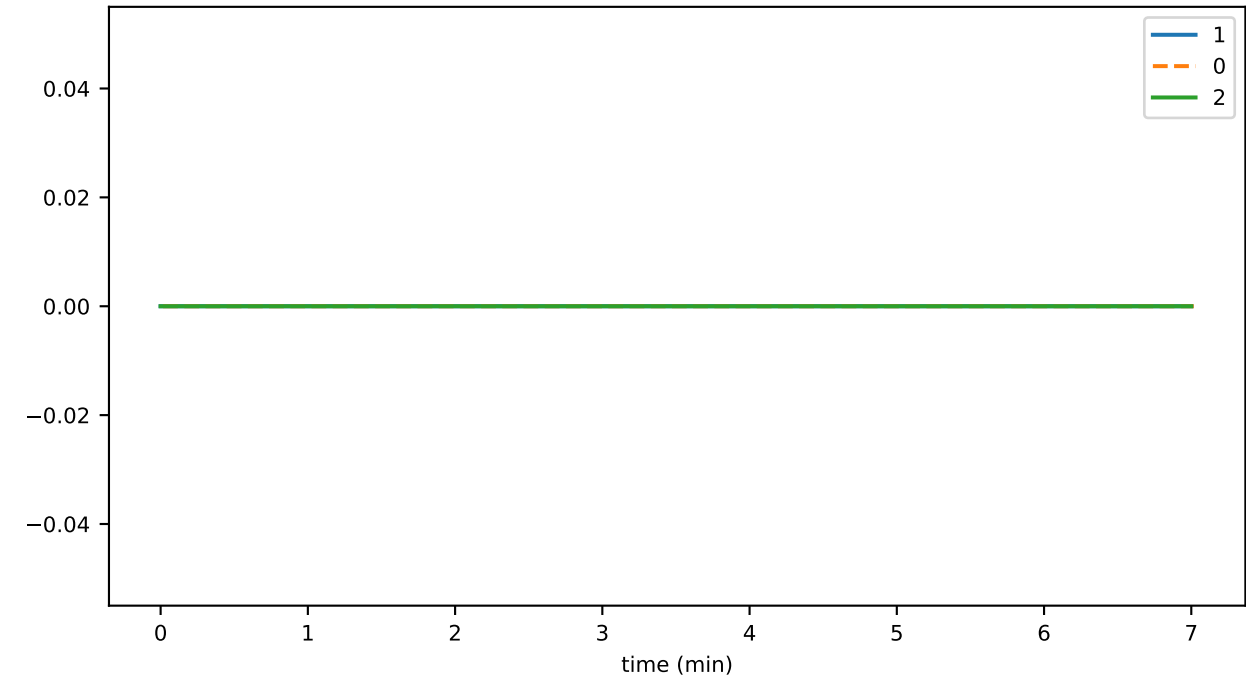
tokenGrantKycToAccountThrottledTxns
