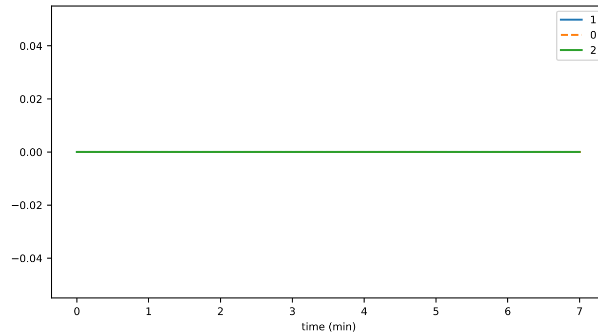
transactionGetRecordThrottledTxns
