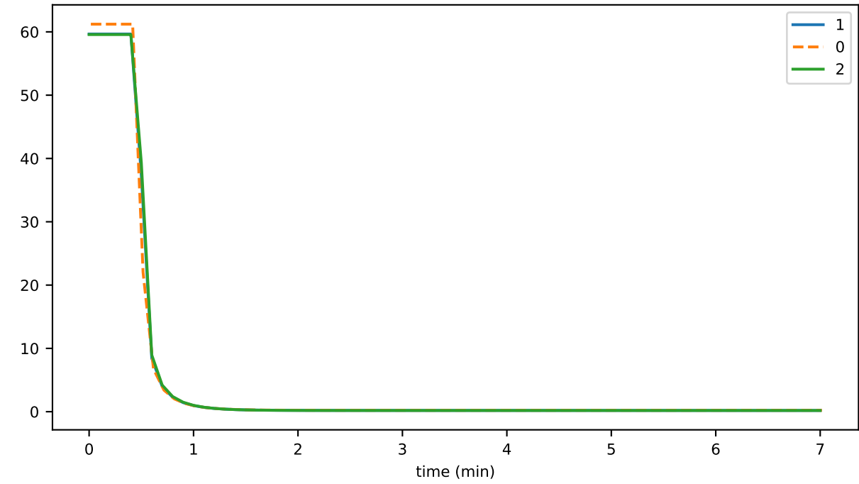
secOR2T
