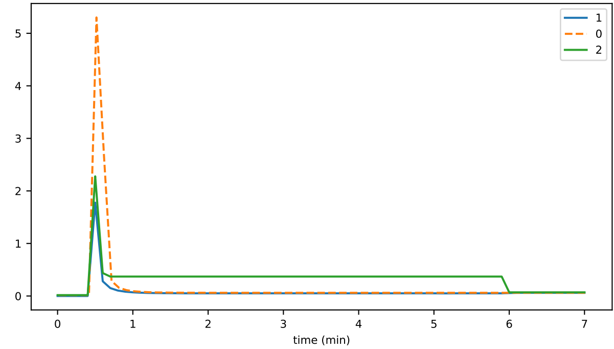
secSC2T
