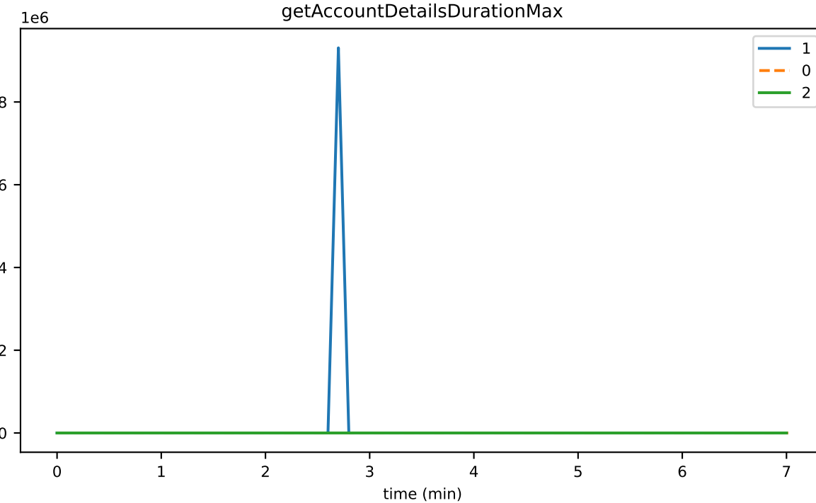
getAccountDetailsDurationMax
