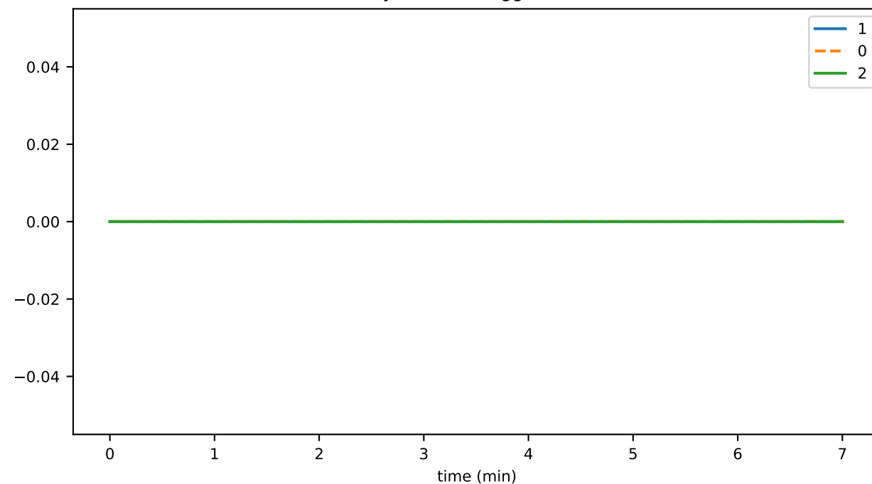
historyProofTransAggToDoneCnt
