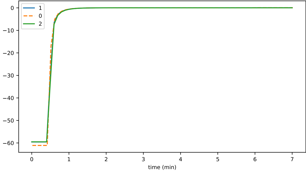
secOR2T
