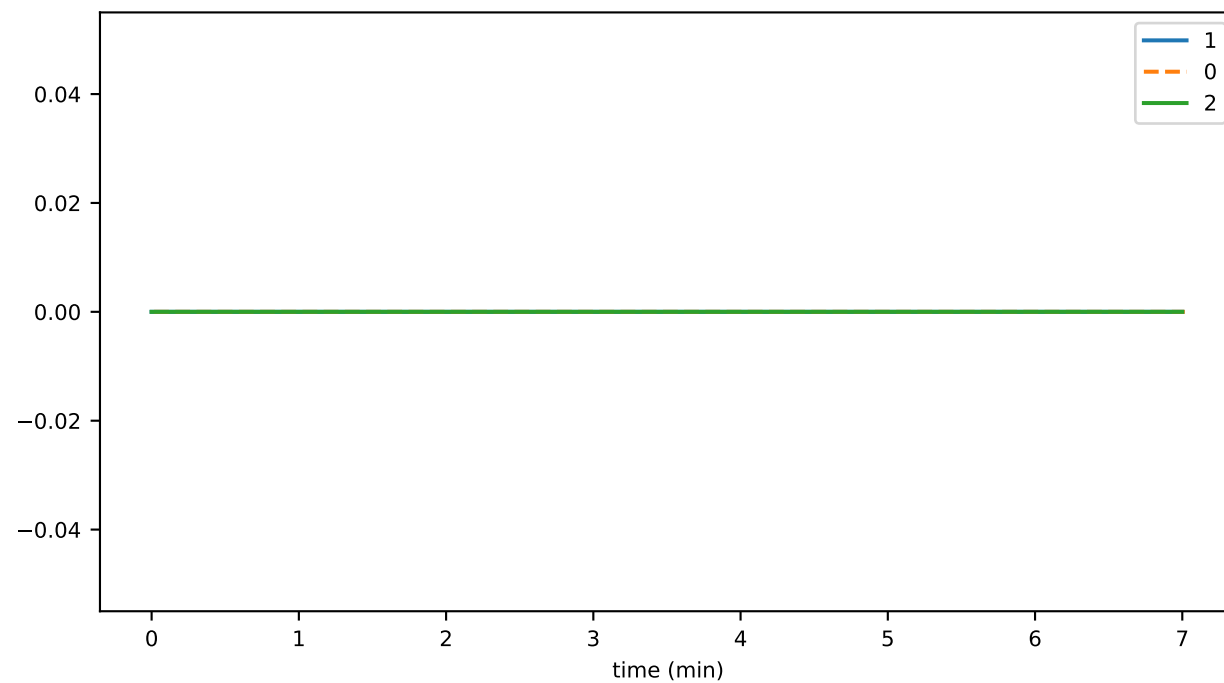
nftsUsed
