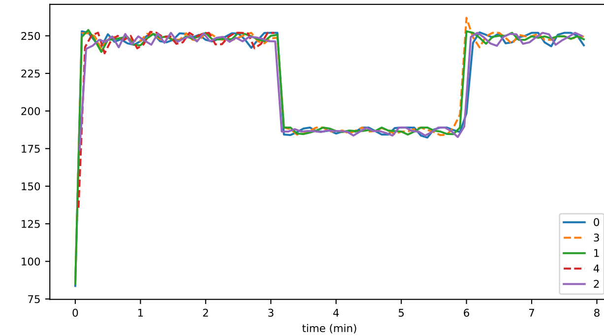
doNotSyncFairSelector
