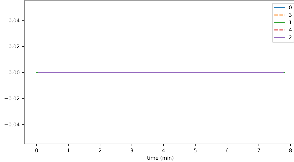
doNotSyncFairSelector
