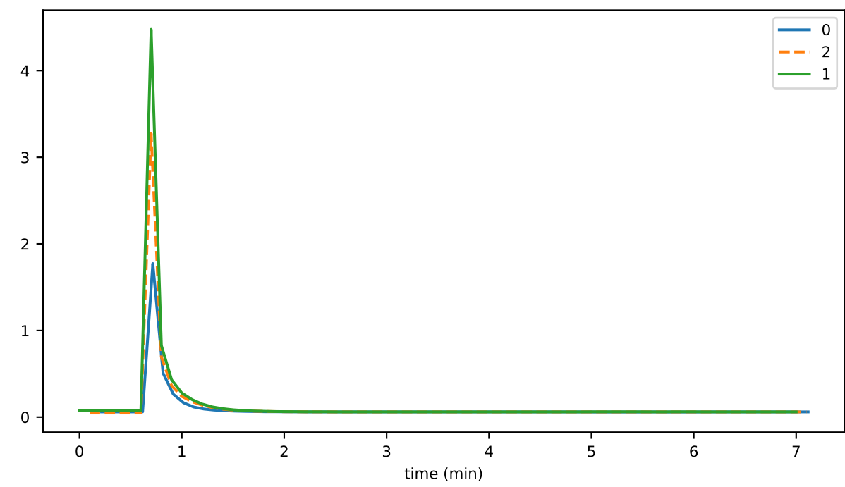
secSC2T
