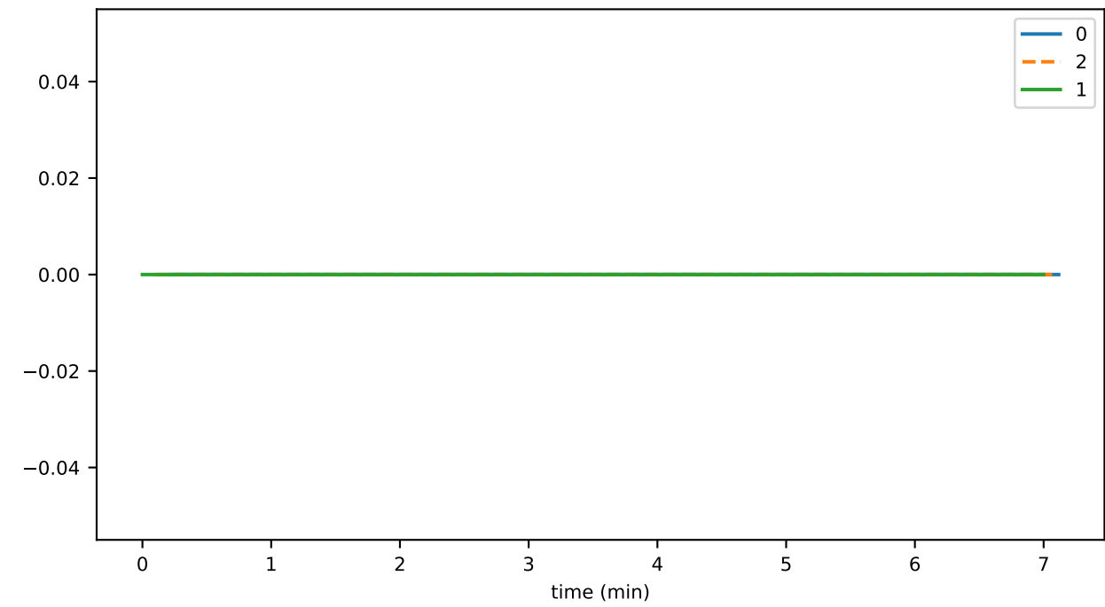
tokenRejectDurationMax
