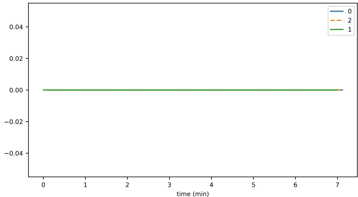
hintsPreprocessingVoteThrottledTxns
