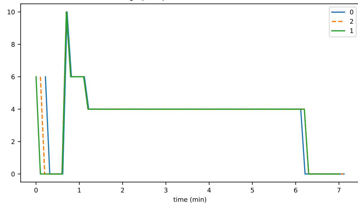
hapiBytesPercentUsed
