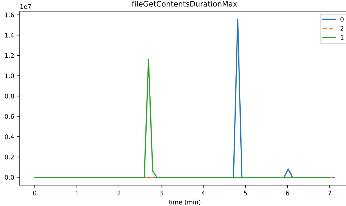
fileGetContentsDurationMax
