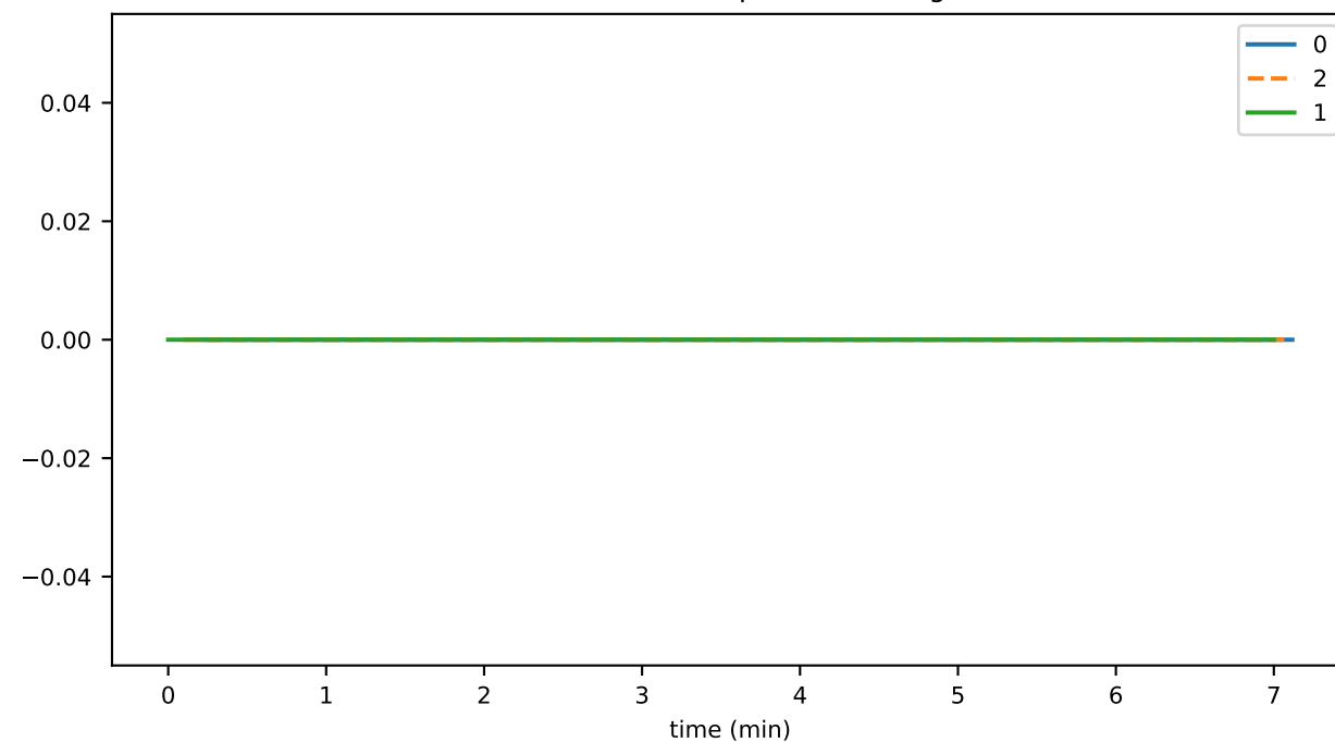
tokenAccountWipeThrottledTxns
