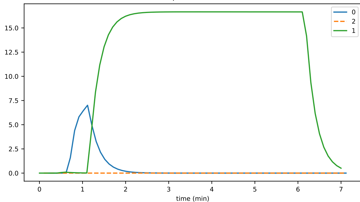
tokenAccountWipeDurationMax
