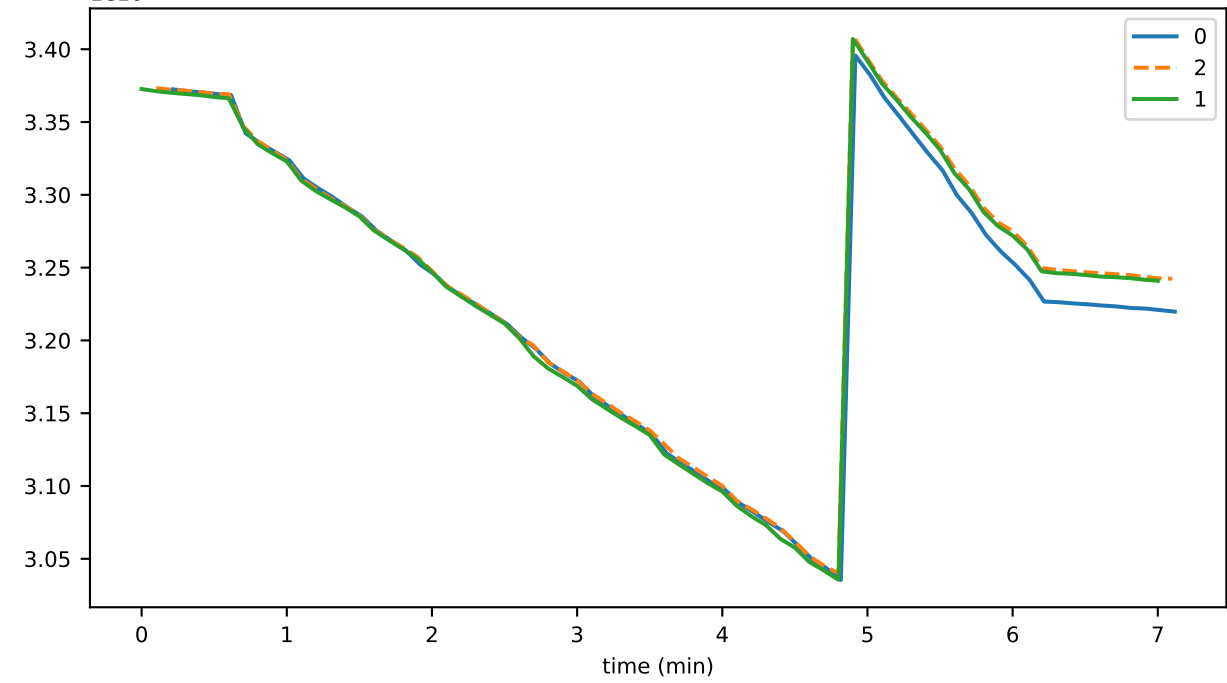
memFree (1e10)
