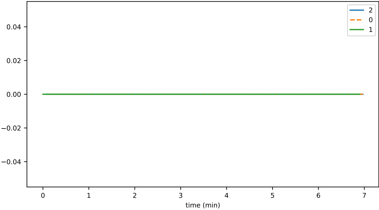
SmartContractService:SystemContractMethodCall_PAUSE_UNPAUSE_total
