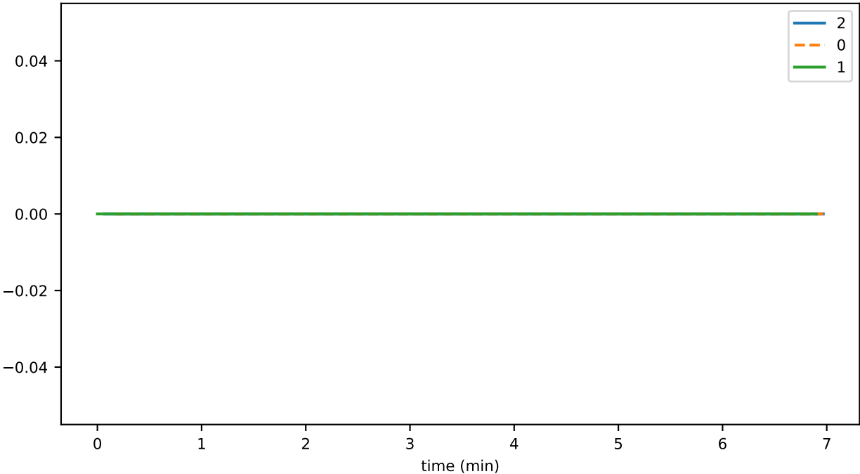
SmartContractService:SystemContractMethodCall_UPDATE_total
