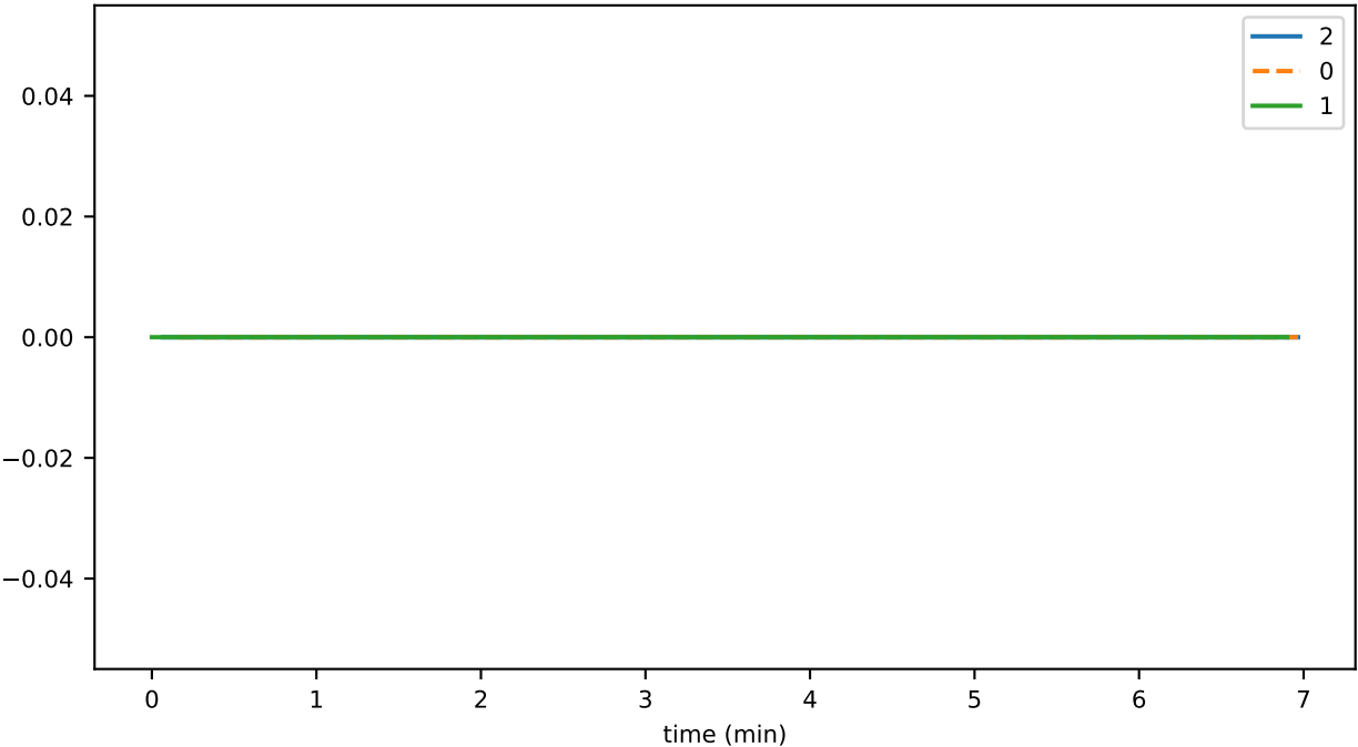
SmartContractService:SystemContractMethodCall_UPDATE_failed
