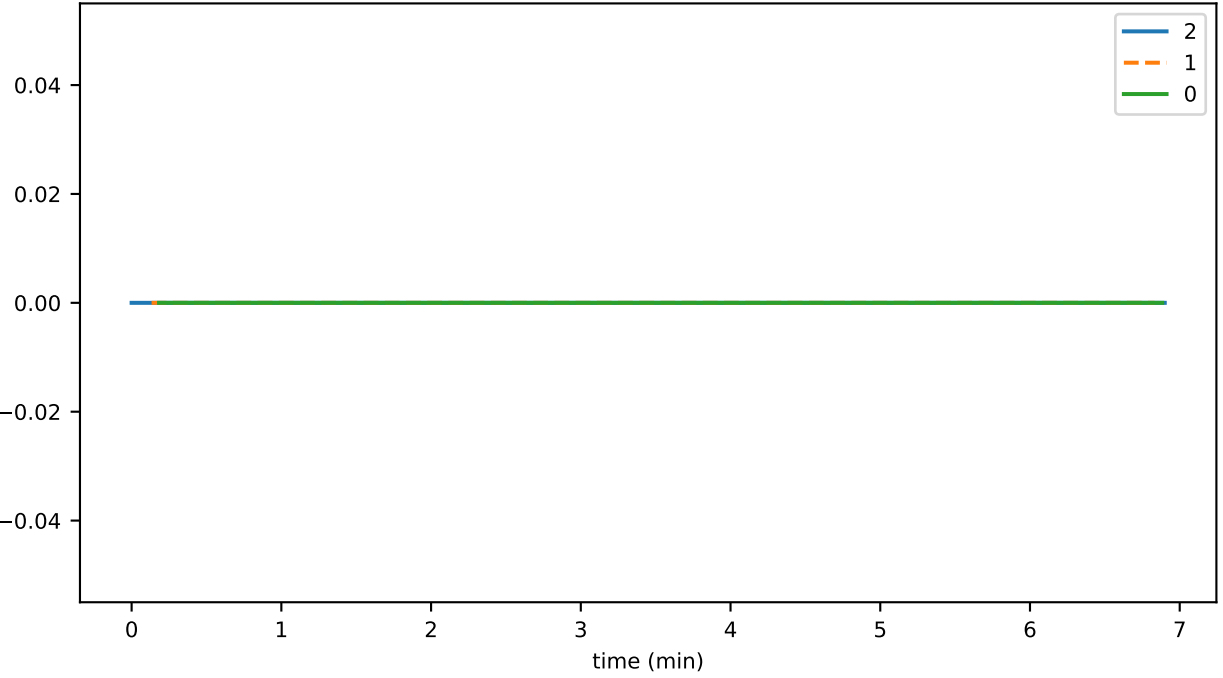
SmartContractService:SystemContractMethodCall_HAS_total
