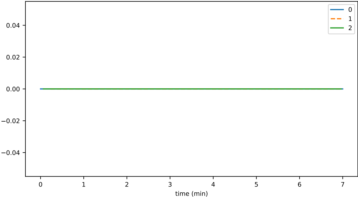
SmartContractService:SystemContractMethodCall_HTS_total
