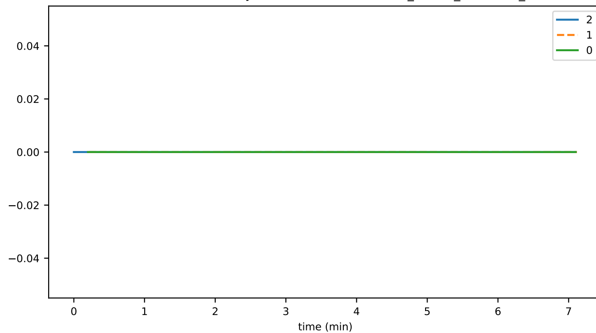
SmartContractService:SystemContractMethodCall_PAUSE_UNPAUSE_total
