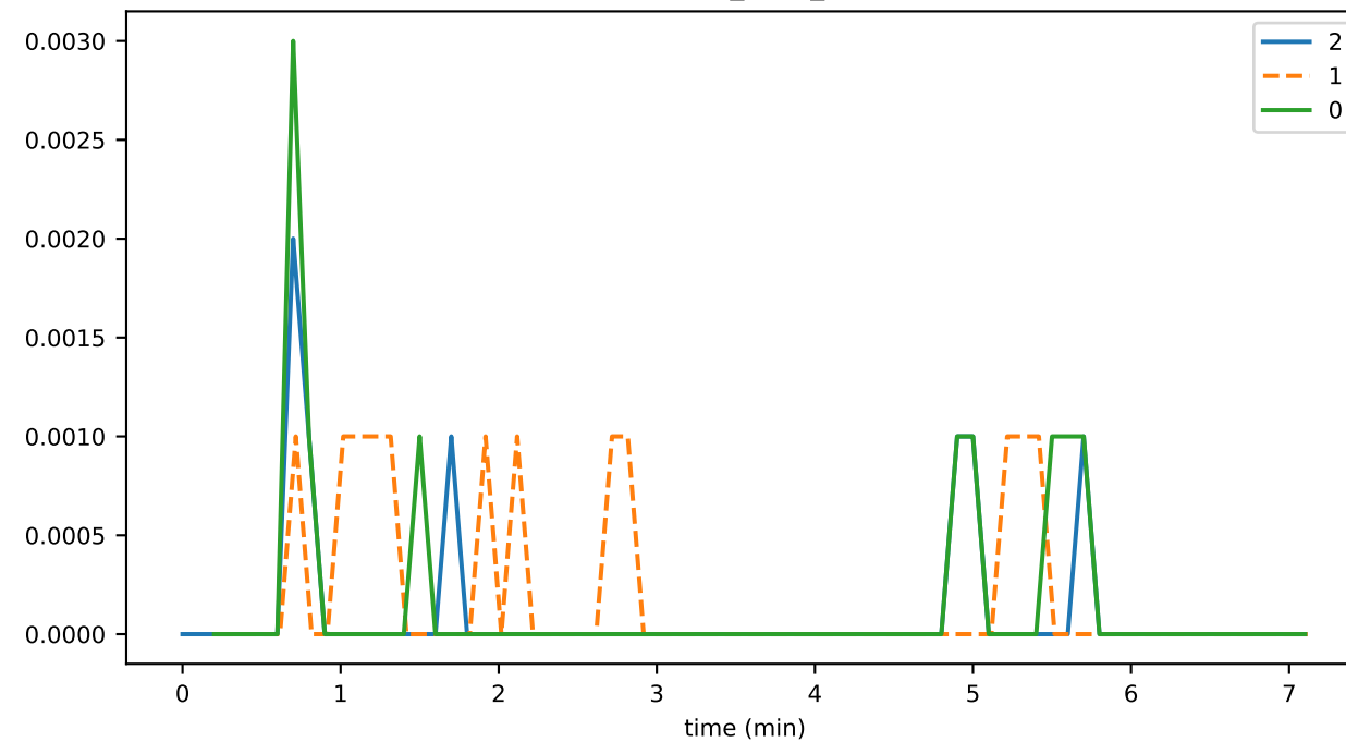
StateHasher_busy_fraction
