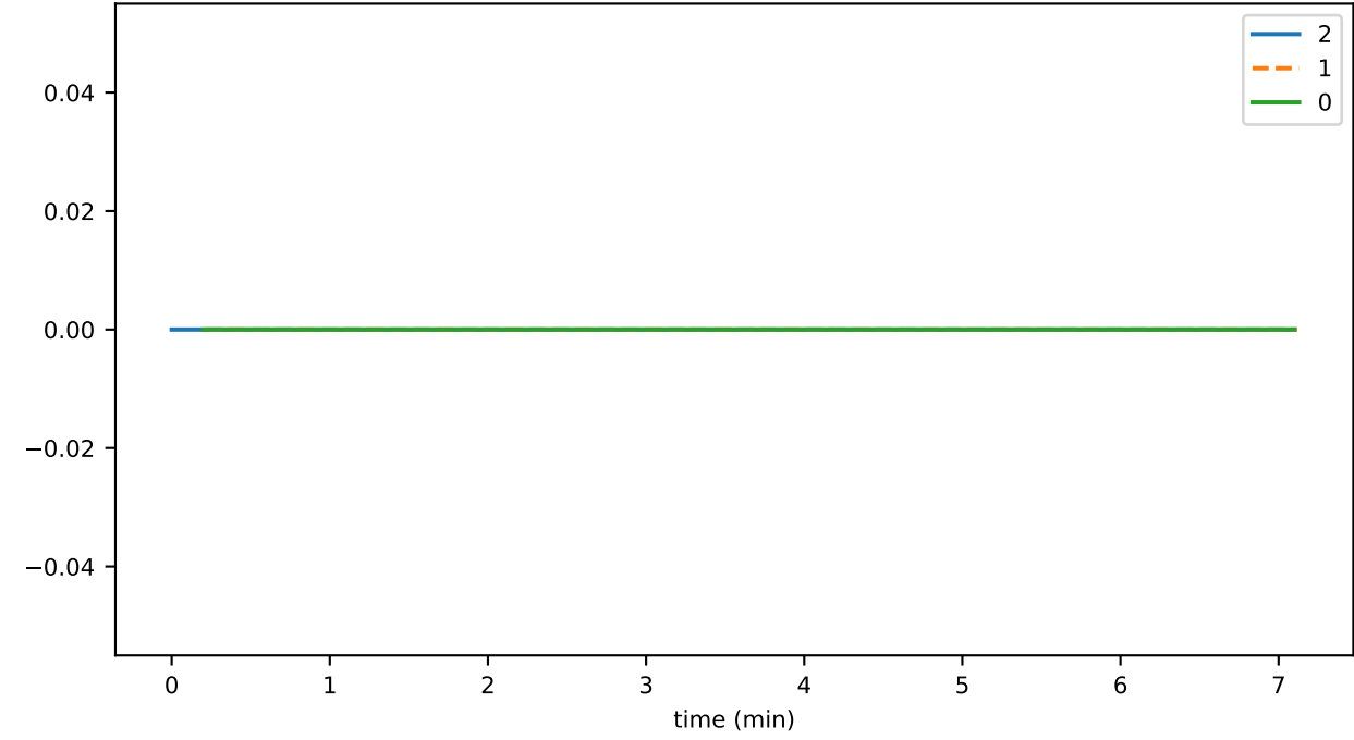
SigBatchSz
