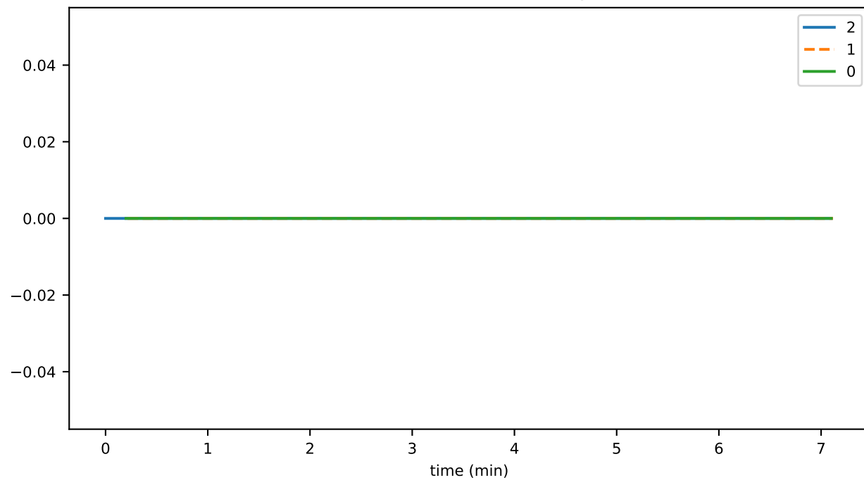
lambdaSStoreThrottledTxns
