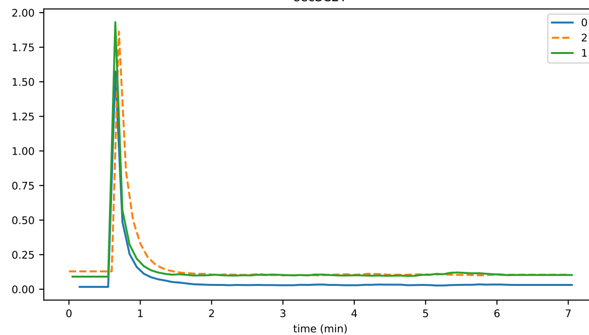
secSC2T
