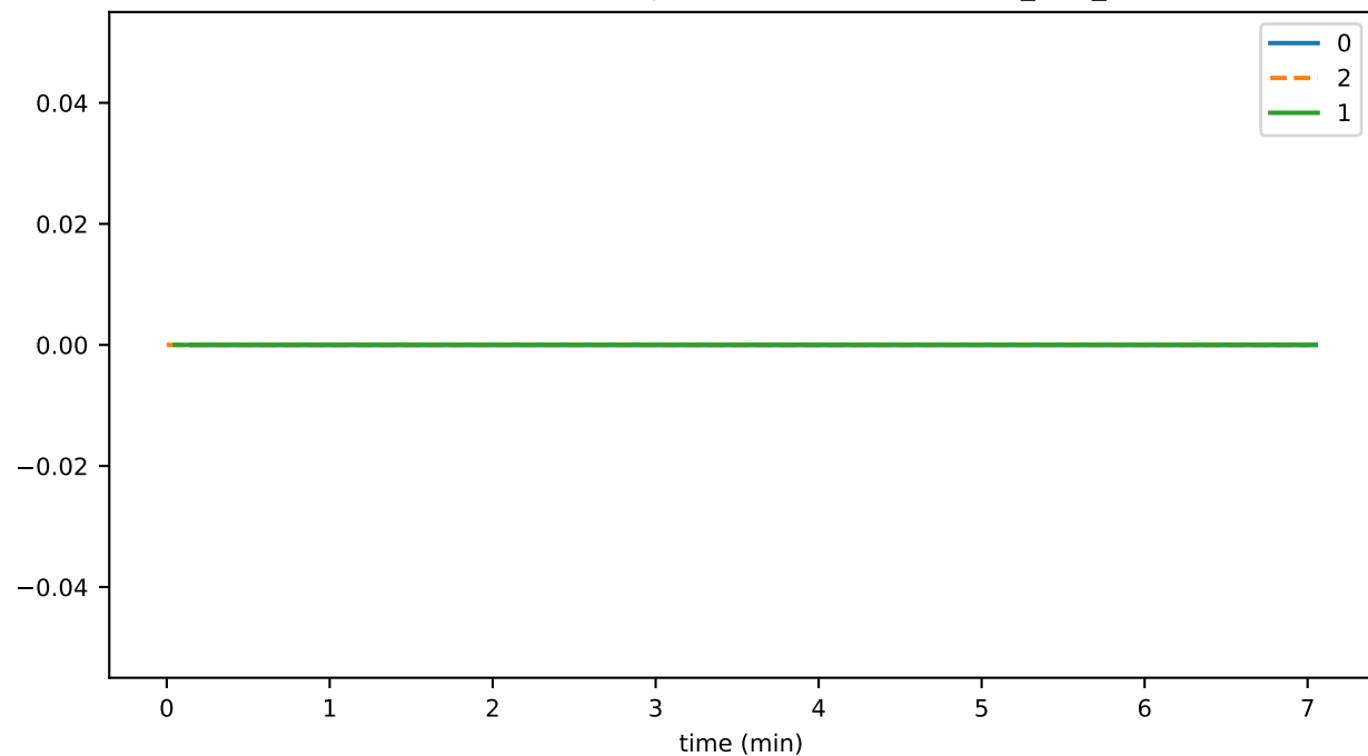
SmartContractService:SystemContractMethodCall_IS_AUTHORIZED_total
