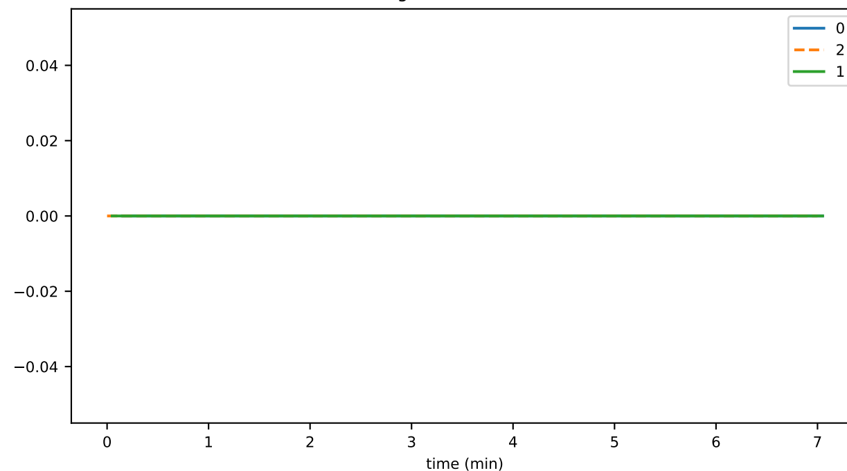
getAccountDetailsDurationMax
