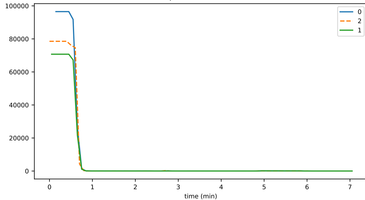
preHandleMicros
