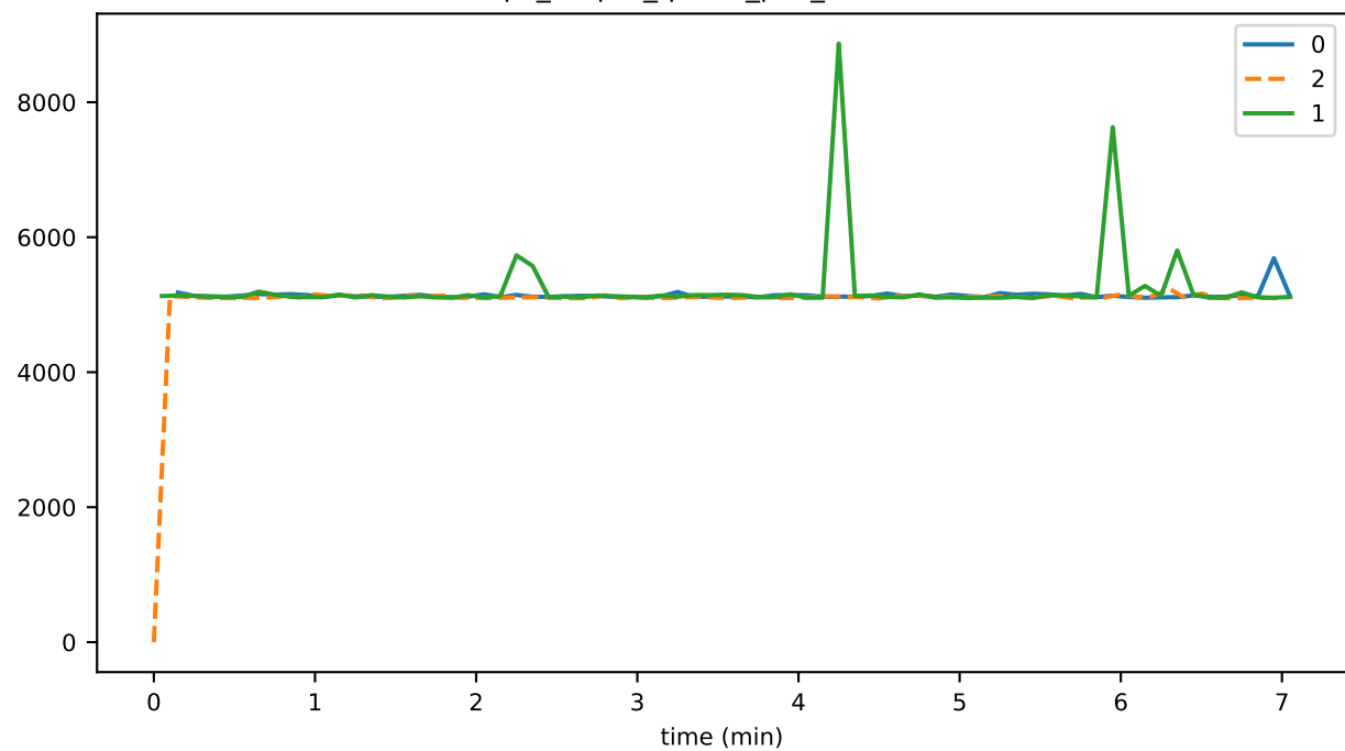
rpc_output_queue_poll_timeMAX
