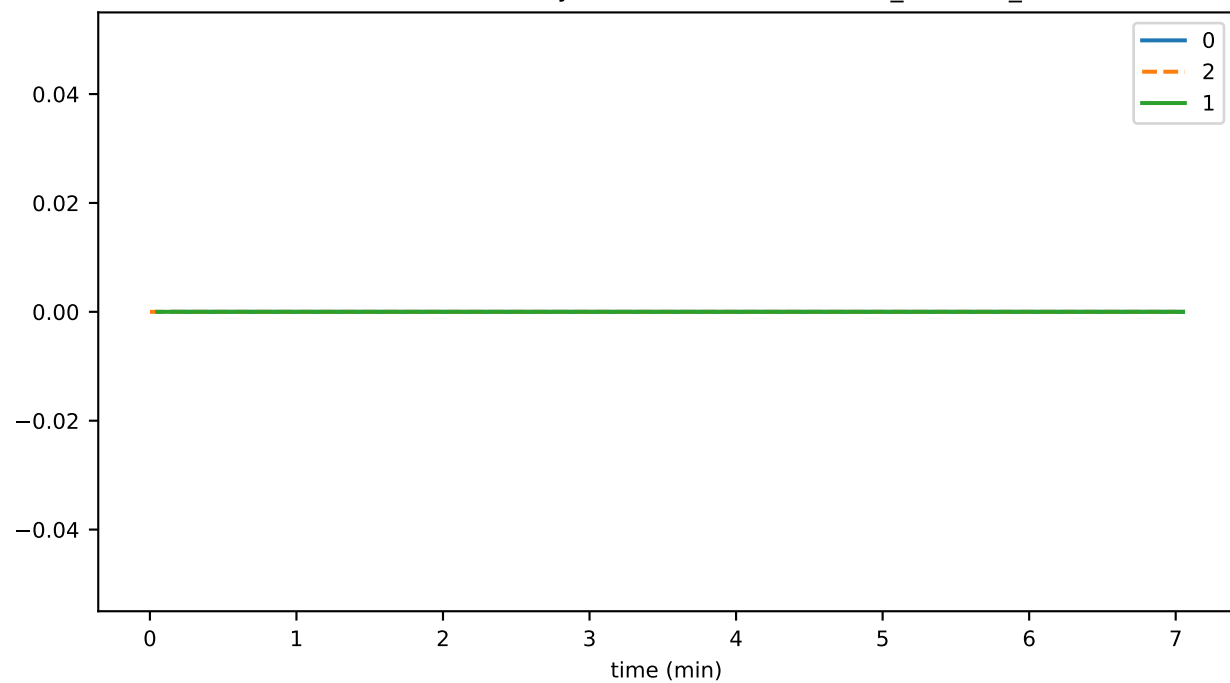
SmartContractService:SystemContractMethodCall_ALIASES_total
