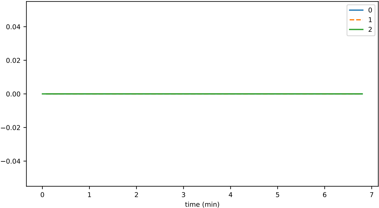
SmartContractService:SystemContractMethodCall_PAUSE_UNPAUSE_total
