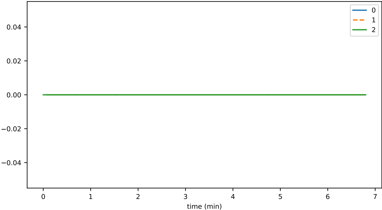
SmartContractService:SystemContractMethodCall_PROXY_failed
