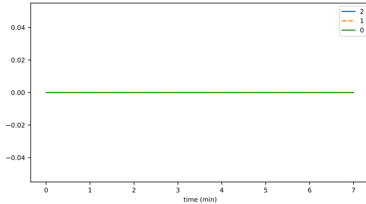
scheduleCreateThrottledTxns
