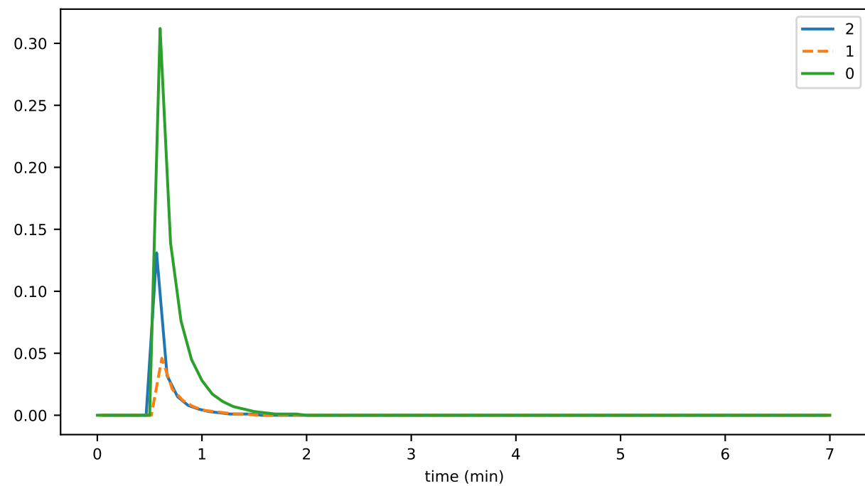
Sig_per_sec
