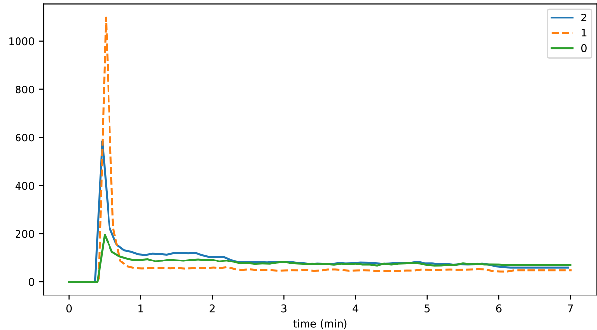
eventDelay_2_validation_gossip
