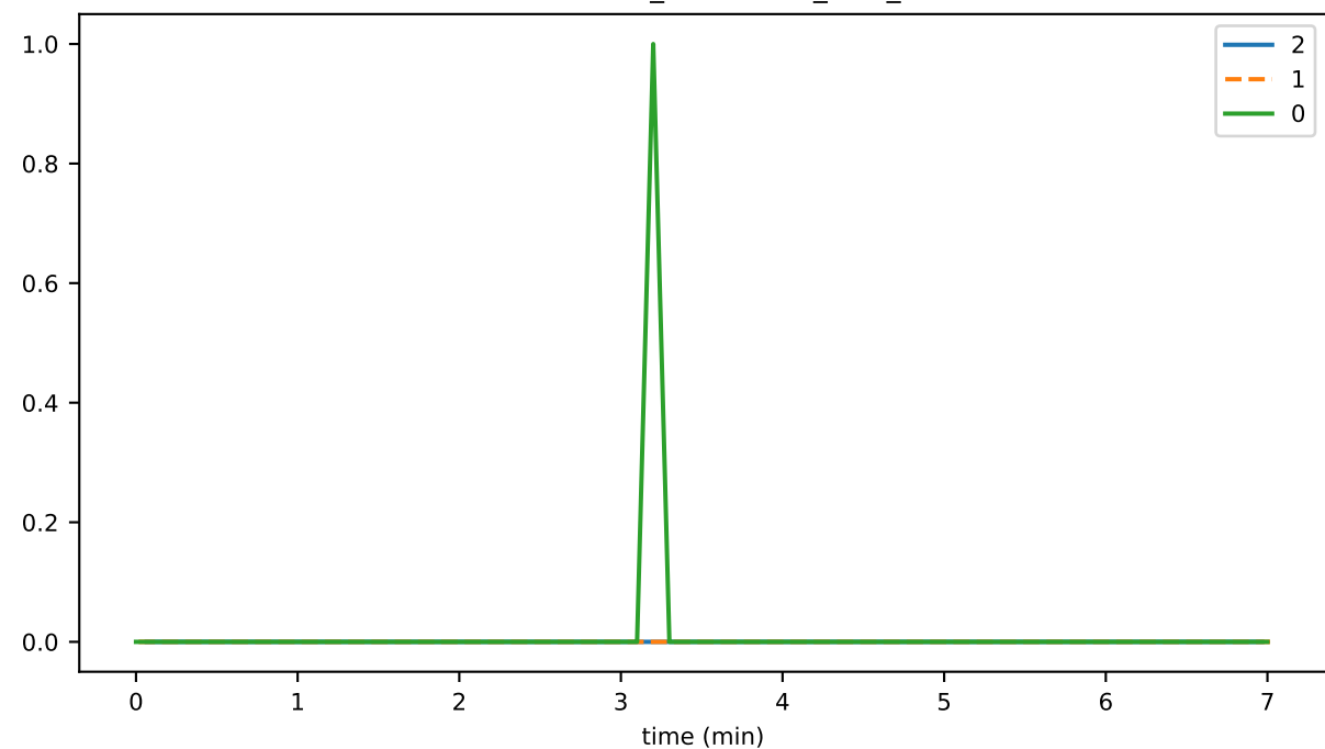
PlatSigEnqueueTime
