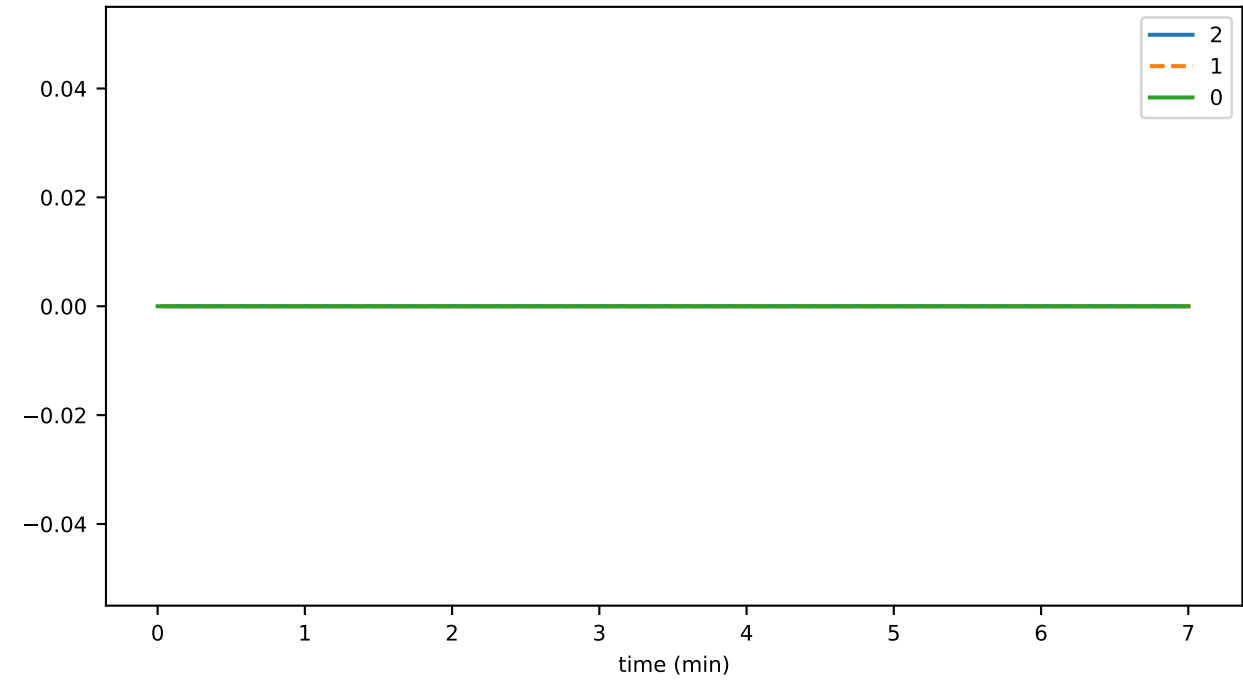
ParseErrOtherRcv
