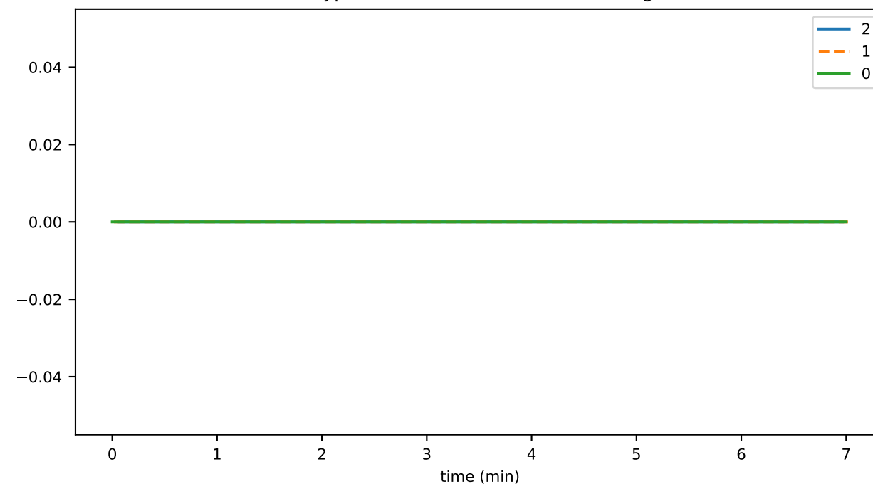
cryptoAccountAutoRenewThrottledTxns
