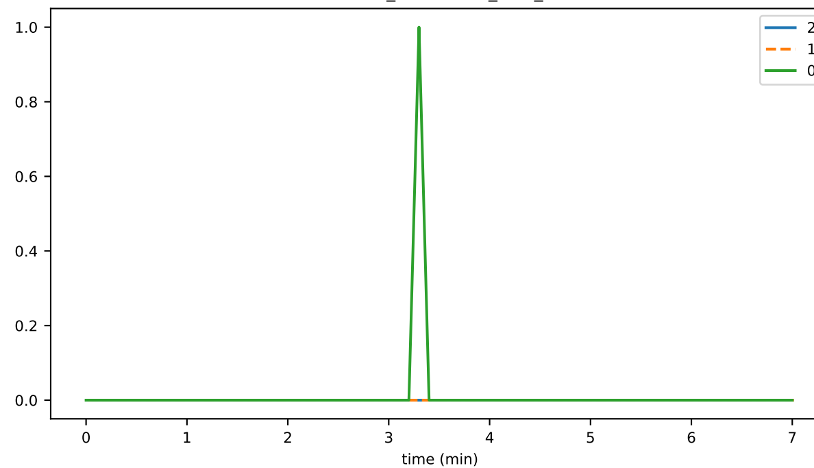
IssDetector_unhandled_task_count
