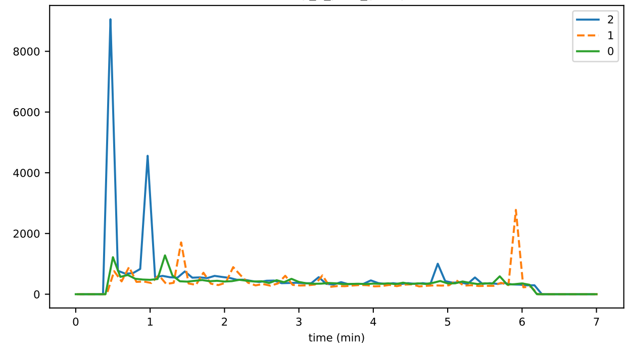
eventDelay_6_pces_runtimeMAX
