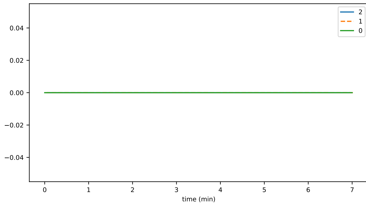
nftsPercentUsed
