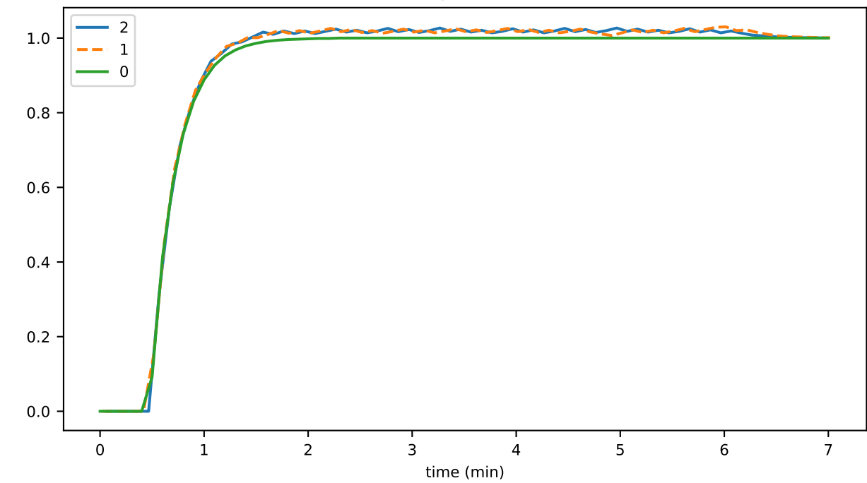
stateToDisk
