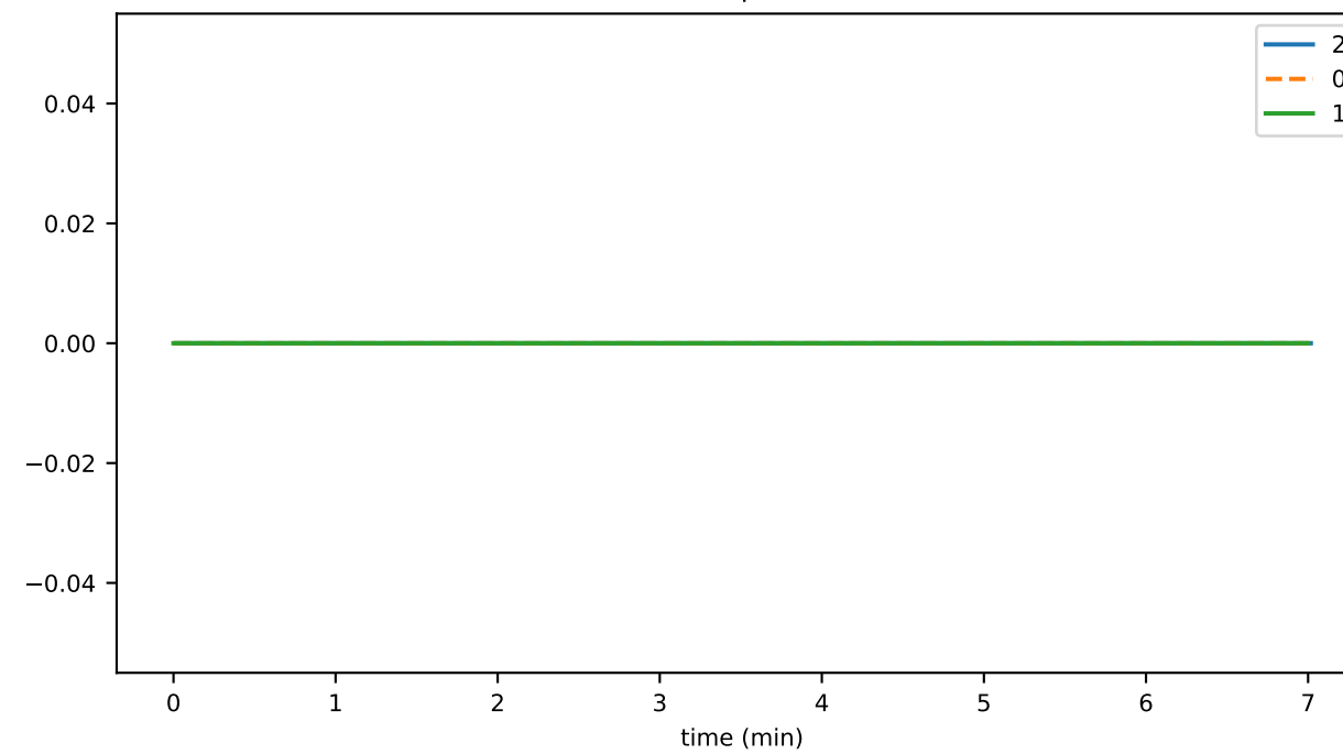
tokenAccountWipeThrottledTxns
