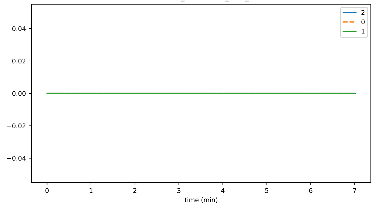
EventHasher_unhandled_task_count
