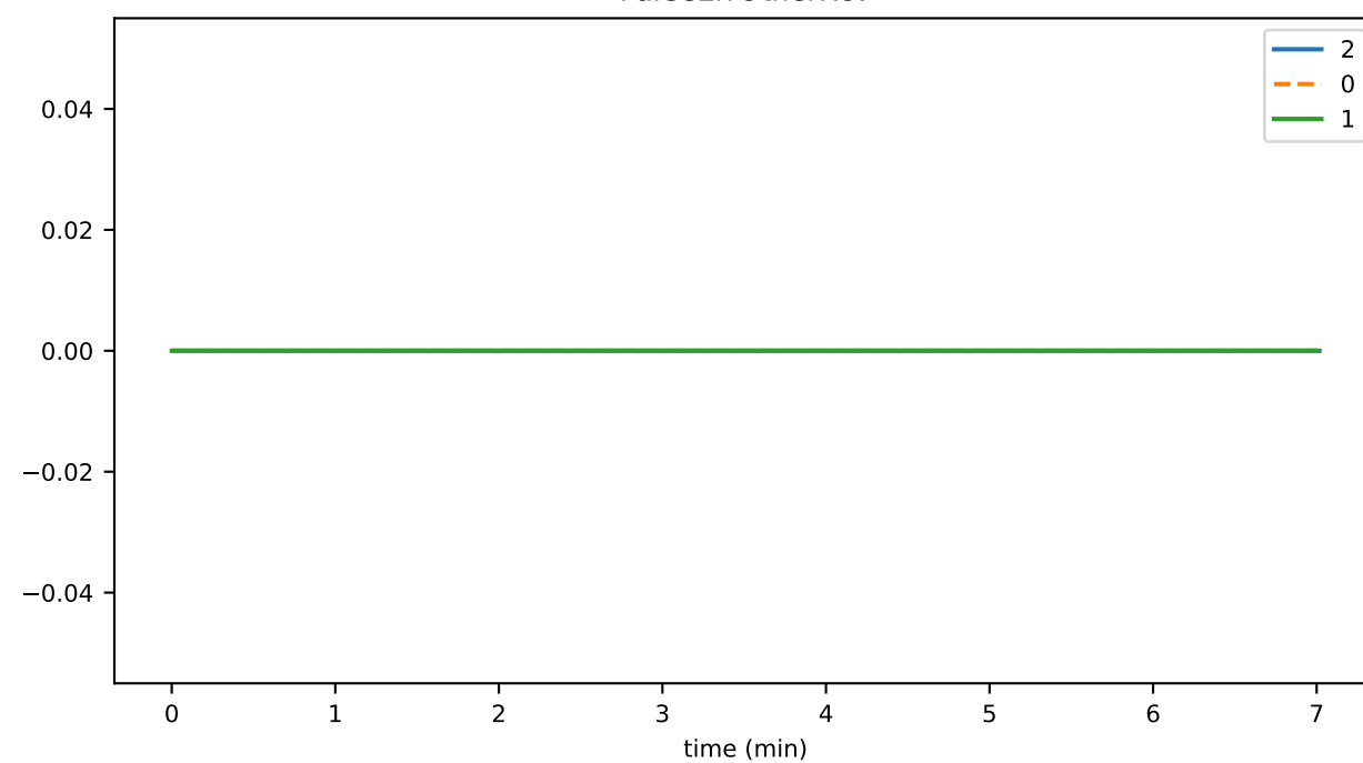
ParseErrOtherRcv
