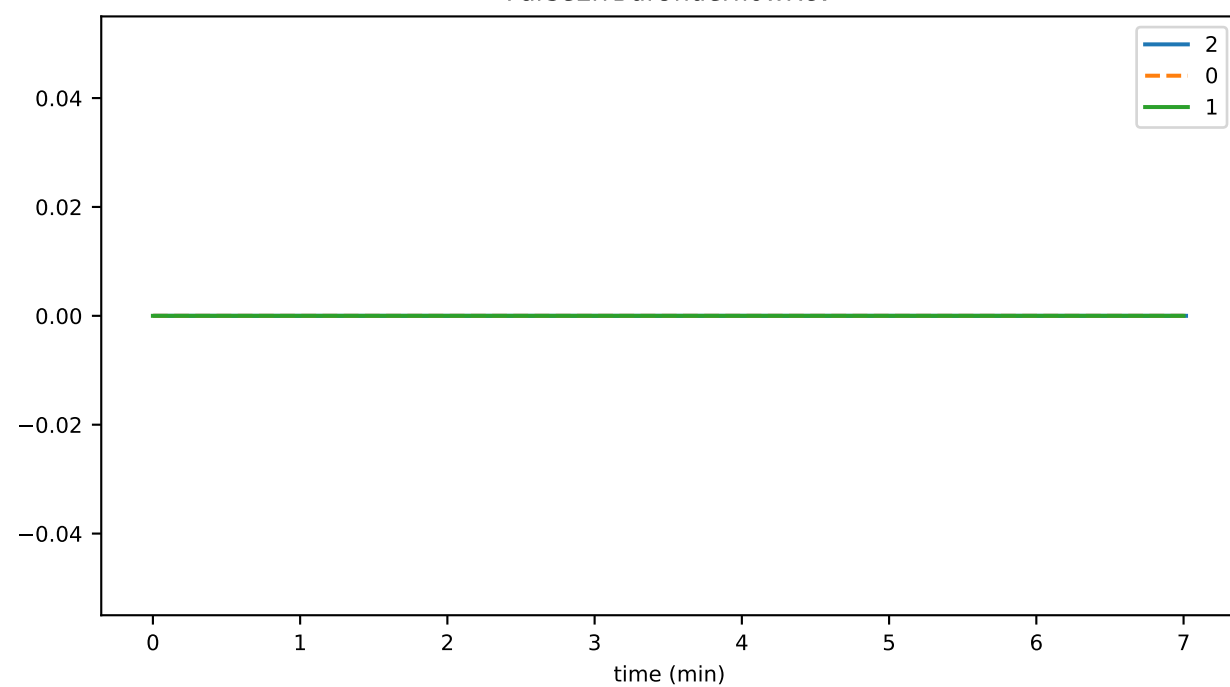
ParseErrBufUnderflowRcv
