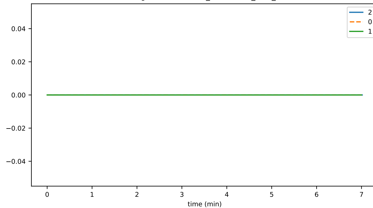
EventSignatureValidator_unhandled_task_count
